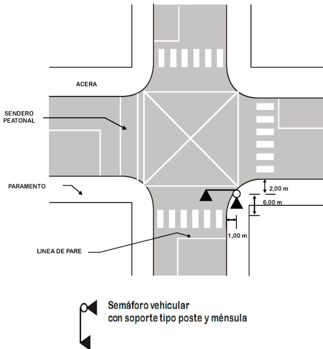
Figura 2.9. Localización de las caras del semáforo en el lado más cercano del acceso de la intersección
