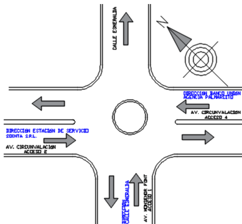
Figura 3.16. Croquis de la intersección – punto de estudio 15
