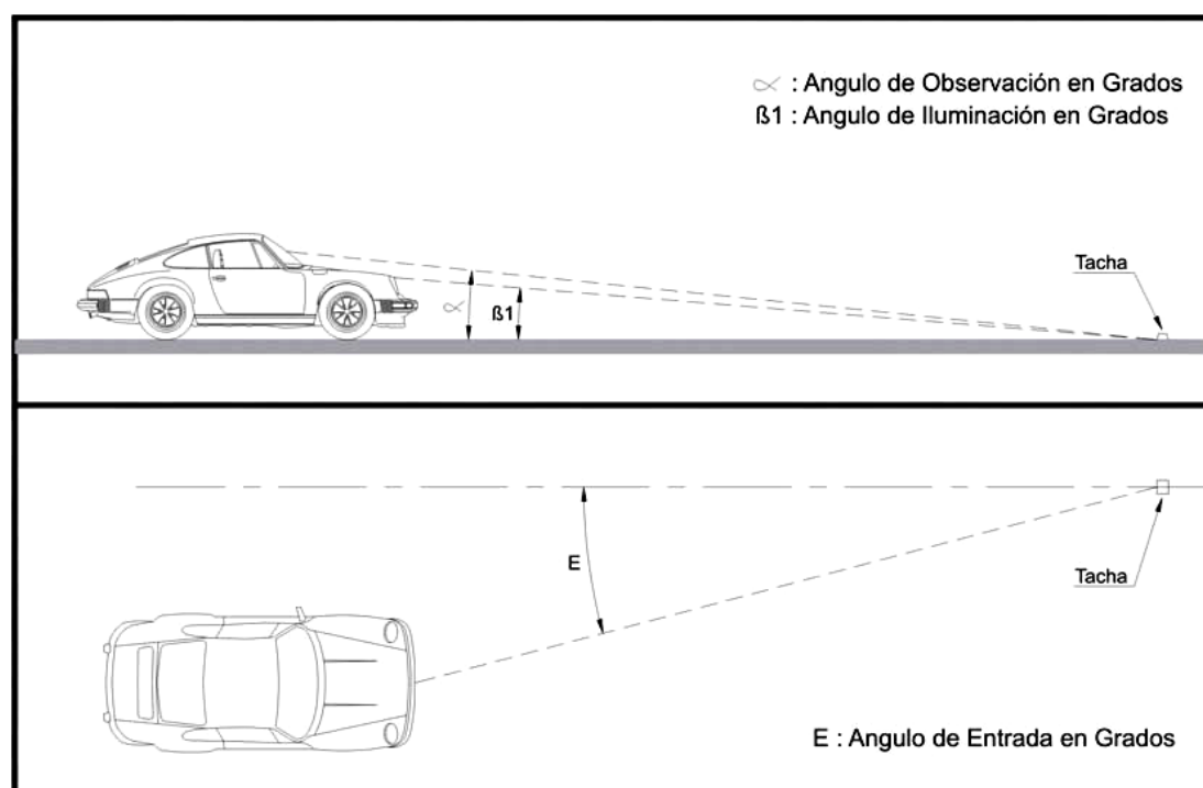
Figura 2.7. Ángulo de entrada y observación de las demarcaciones (Señalización horizontal)
