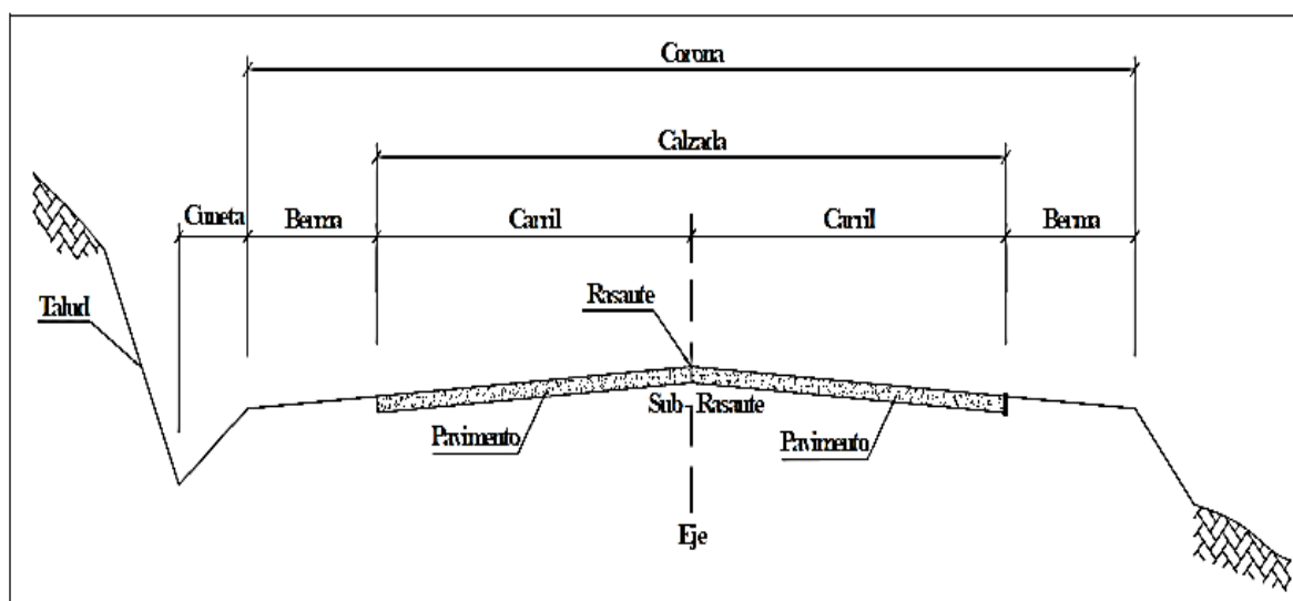
Figura 2.1. Partes integrantes de una vía
