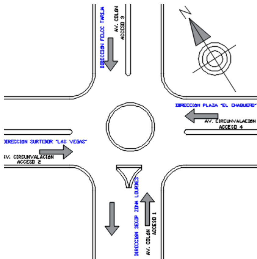
Figura 3.6. Croquis de la intersección – punto de estudio 5
