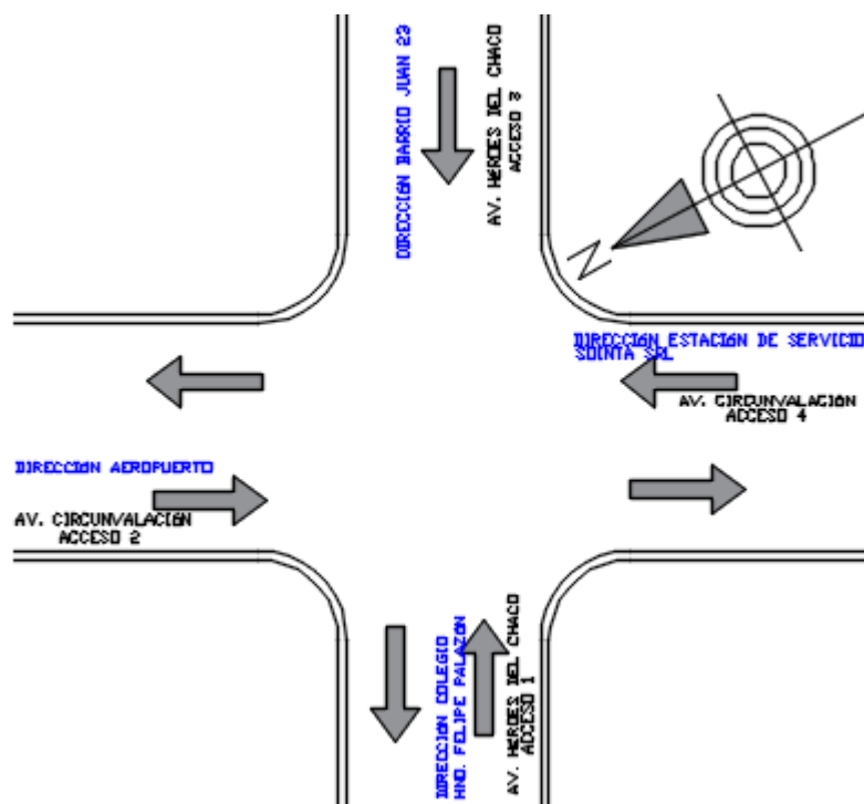
Figura 3.19. Croquis de la intersección – punto de estudio 18
