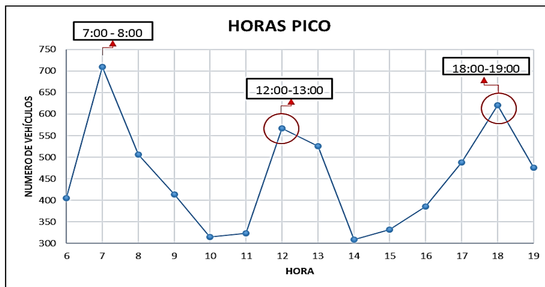
Figura 3.20. Horas pico – Avenida Circunvalación
