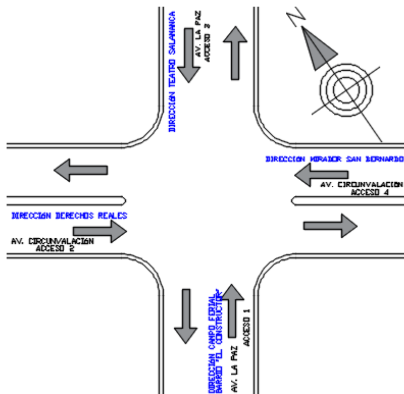
Figura 3.11. Croquis de la intersección – punto de estudio 10
