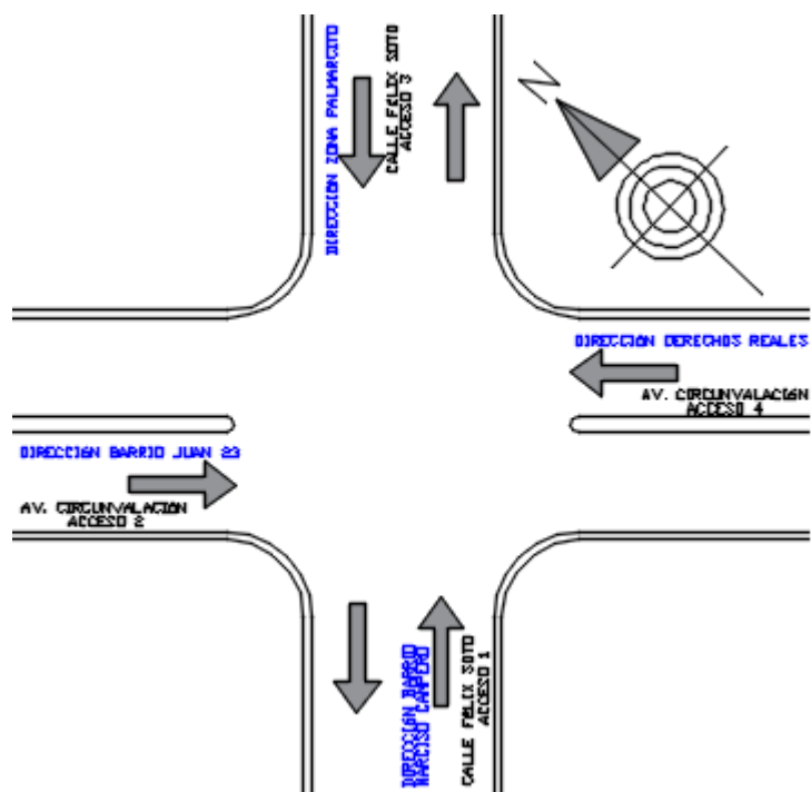
Figura 3.14. Croquis de la intersección – punto de estudio 13
