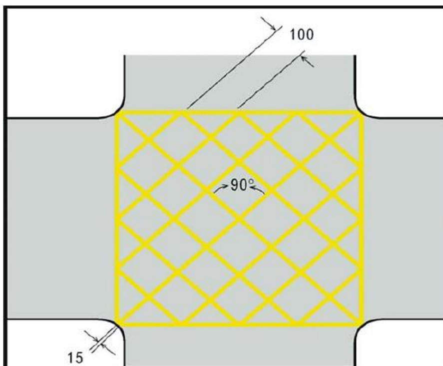
Figura 3.48. Demarcación tipo “bloqueo de cruces”
