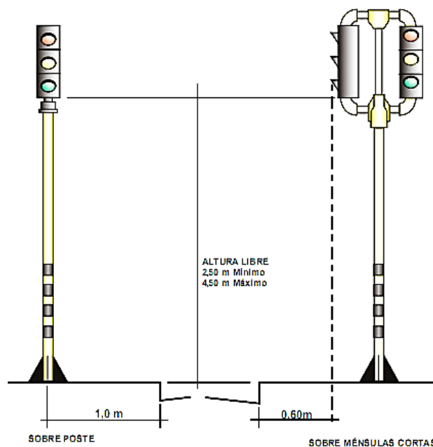
Figura 2.11. Semáforos montados en postes o en ménsula corta
