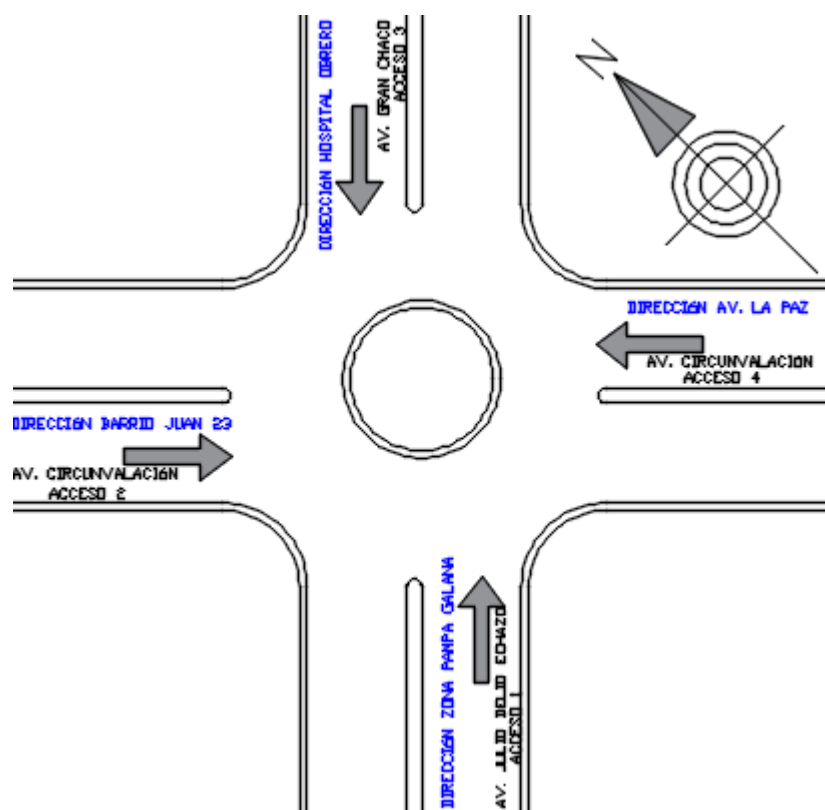
Figura 3.12. Croquis de la intersección – punto de estudio 11
