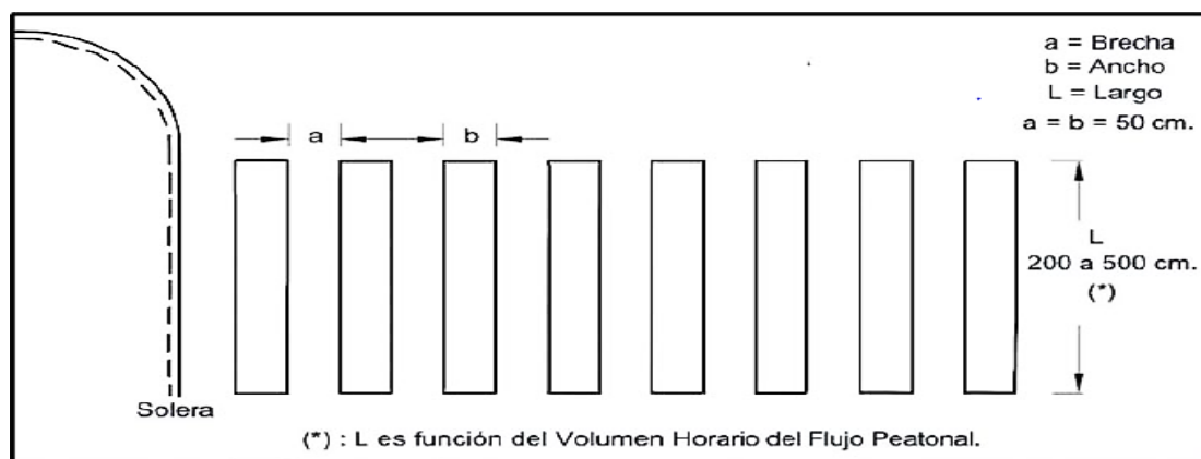
Figura 3.47. Pasos de cebra
