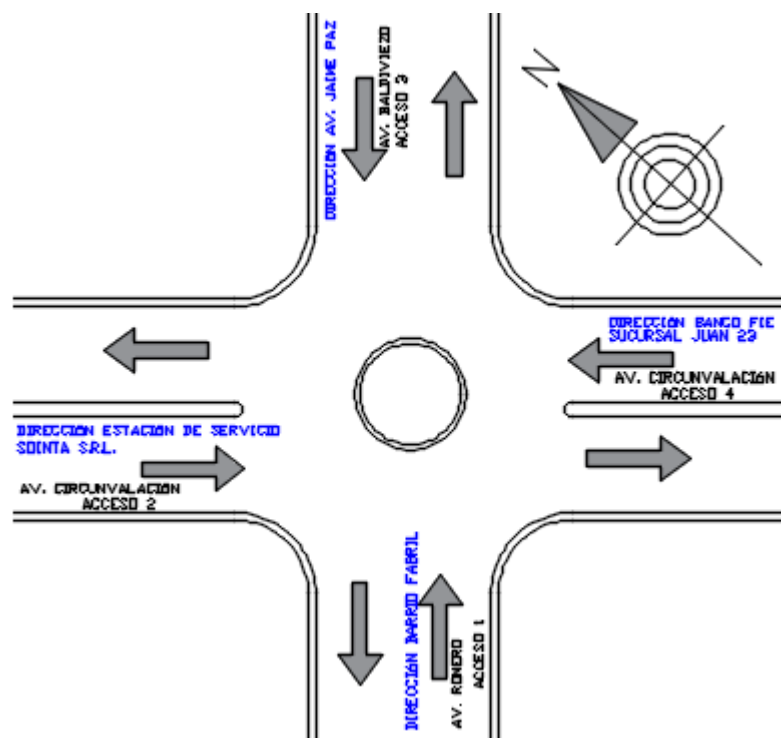
Figura 3.17. Croquis de la intersección – punto de estudio 16
