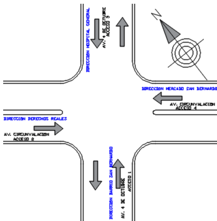
Figura 3.10. Croquis de la intersección – punto de estudio 9
