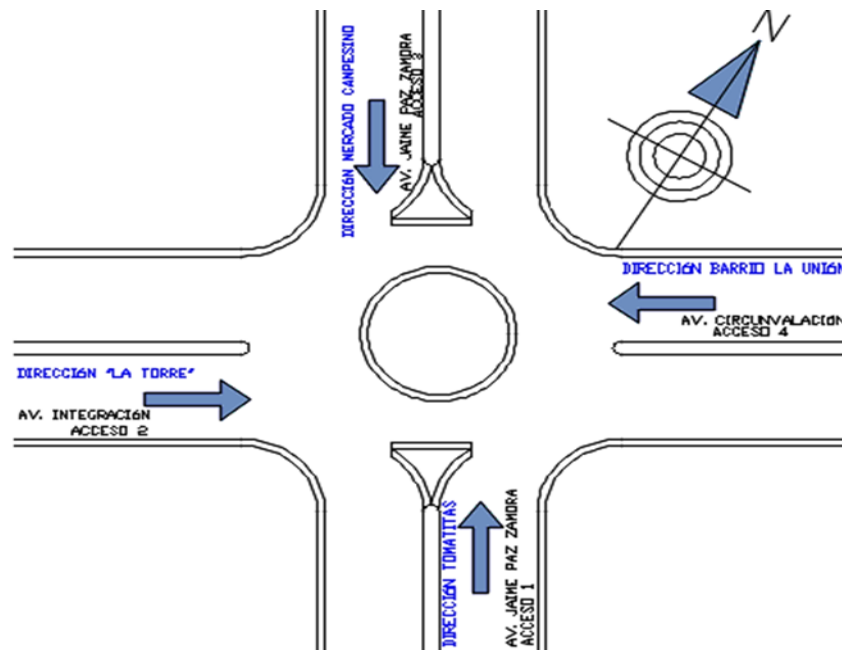
Figura 3.42. Croquis de la intersección - punto de estudio 1
