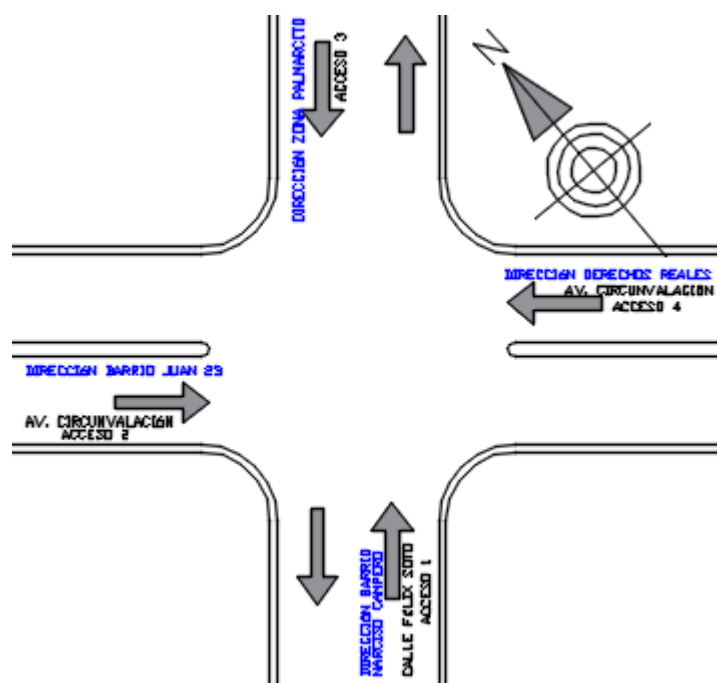
Figura 3.15. Croquis de la intersección – punto de estudio 14
