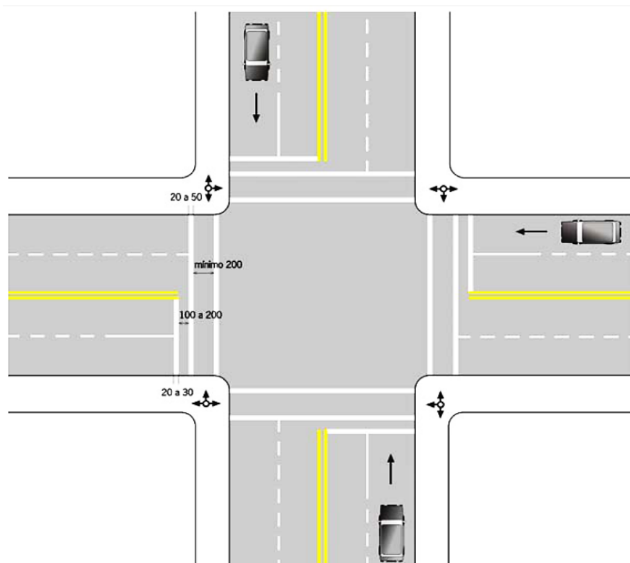
Figura 3.45. Demarcación paso peatonal regulado por semáforo
