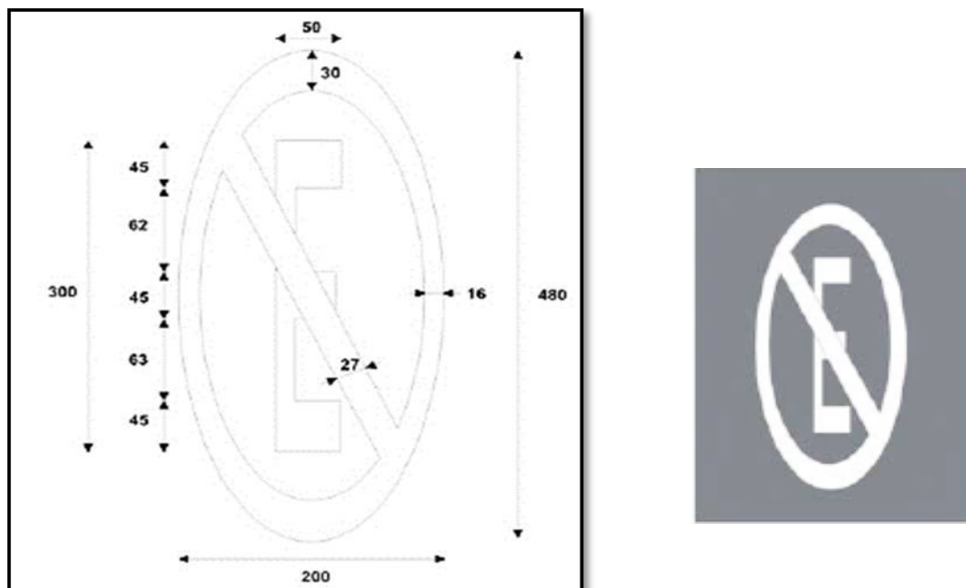
Figura 3.46. Prohibido estacionar
