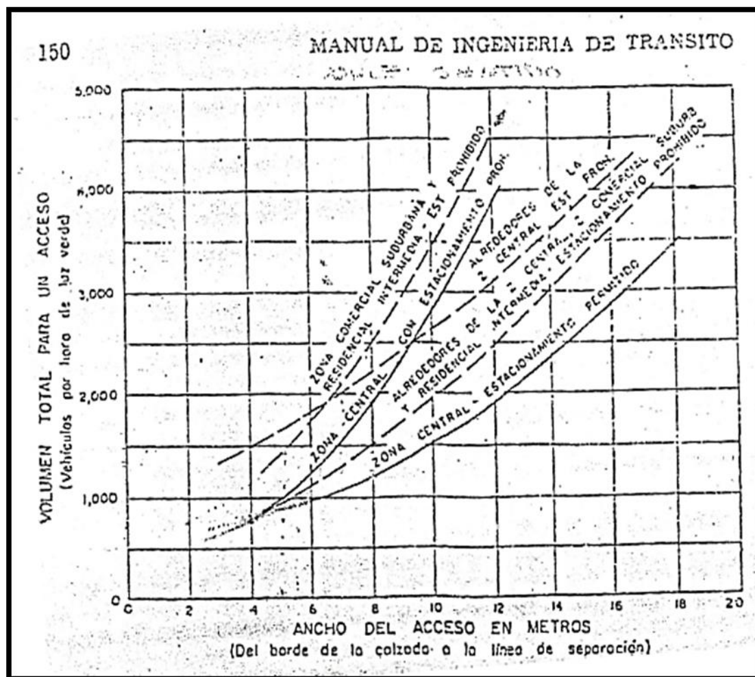
Figura 3.40. Ábaco para capacidad teórica en vías interrumpidas de doble sentido
