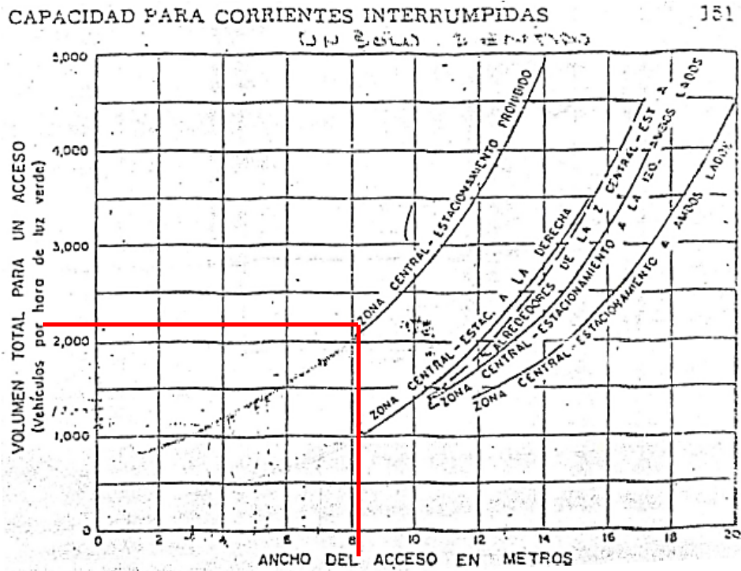
Figura 3.41. Capacidad teórica del acceso 1 del punto de estudio 1
