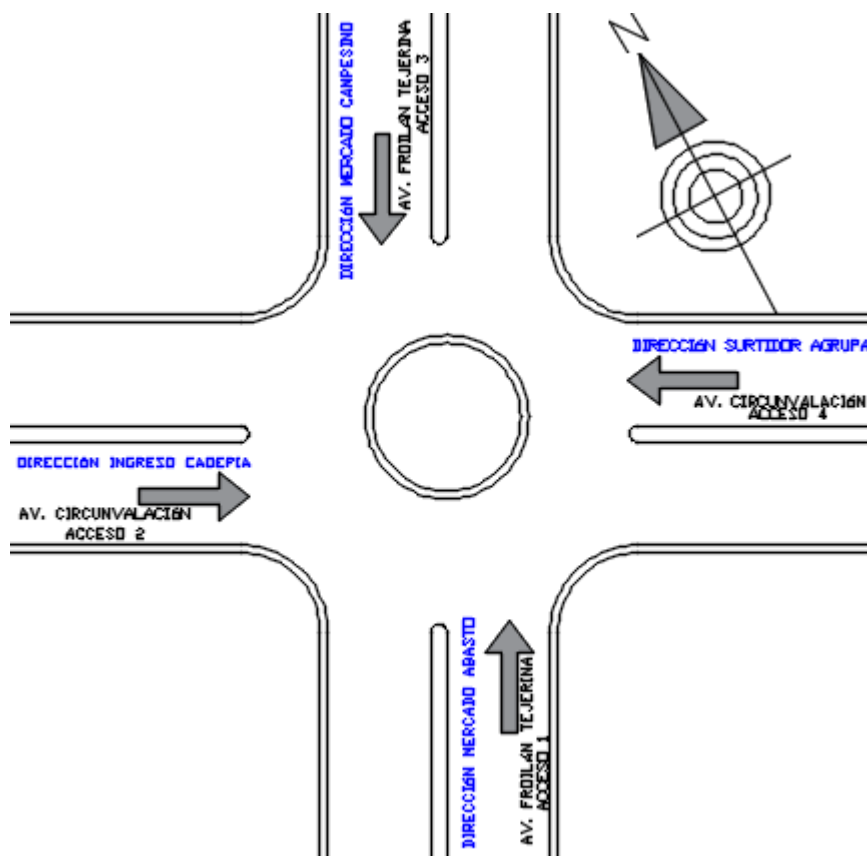
Figura 3.3. Croquis de la intersección – punto de estudio 2
