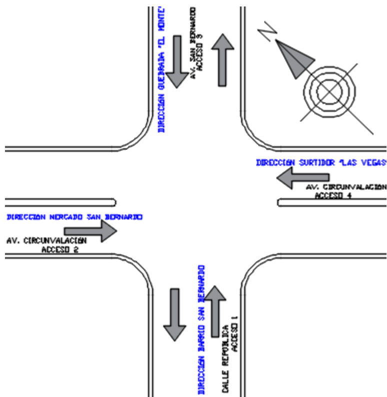
Figura 3.9. Croquis de la intersección – punto de estudio 8
