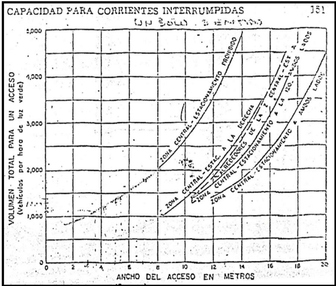
Figura 3.39. Ábaco para capacidad teórica en vías interrumpidas en un solo sentido
