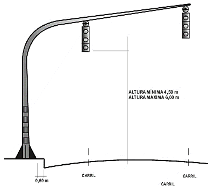
Figura 2.10. Semáforos montados en ménsula sujeta a poste lateral
