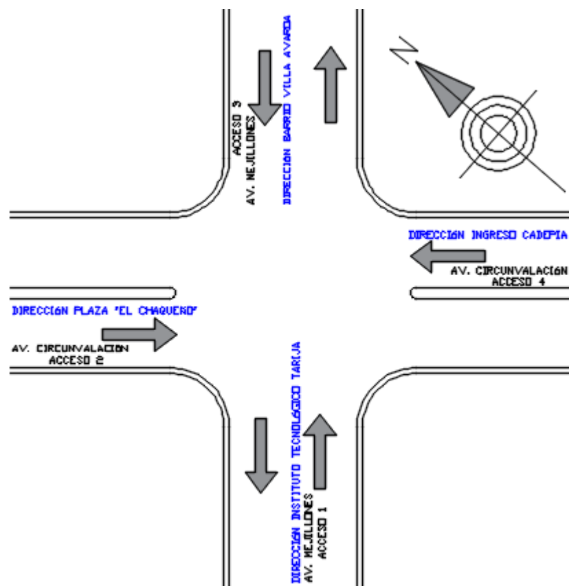
Figura 3.4. Croquis de la intersección – punto de estudio 3
