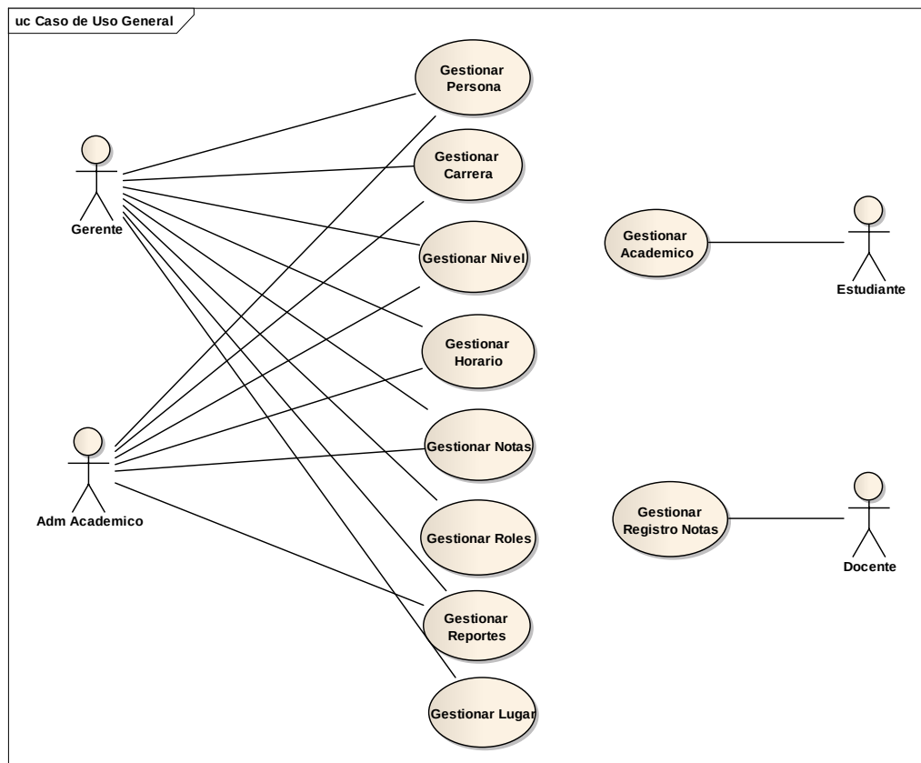
Figura 9 Caso de Uso General
