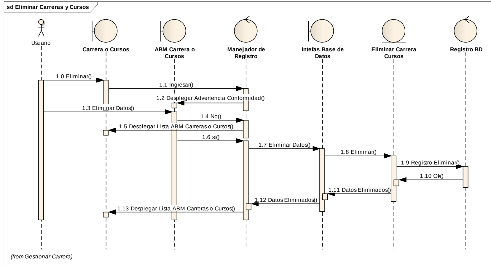
Figura 32 Eliminar Carrera o Cursos
