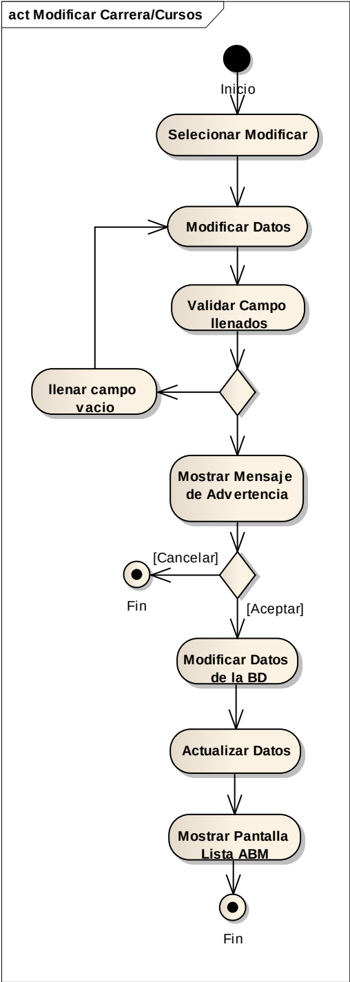
Figura 71 Modificar Carrera y Cursos
