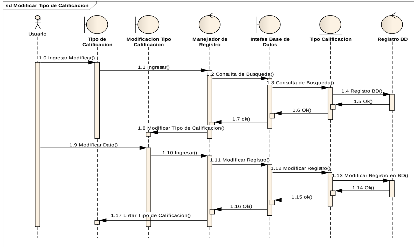
Figura 41 Modificar Tipo de Calificación
