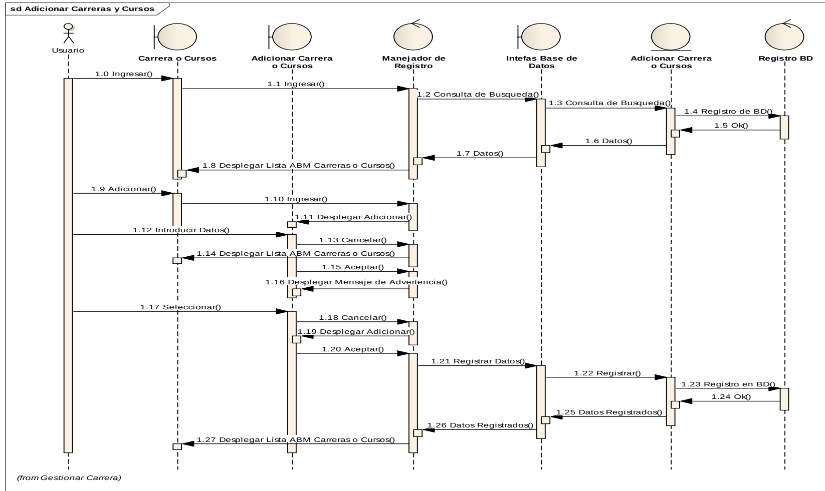
Figura 30 Adicionar Carrera o Cursos
