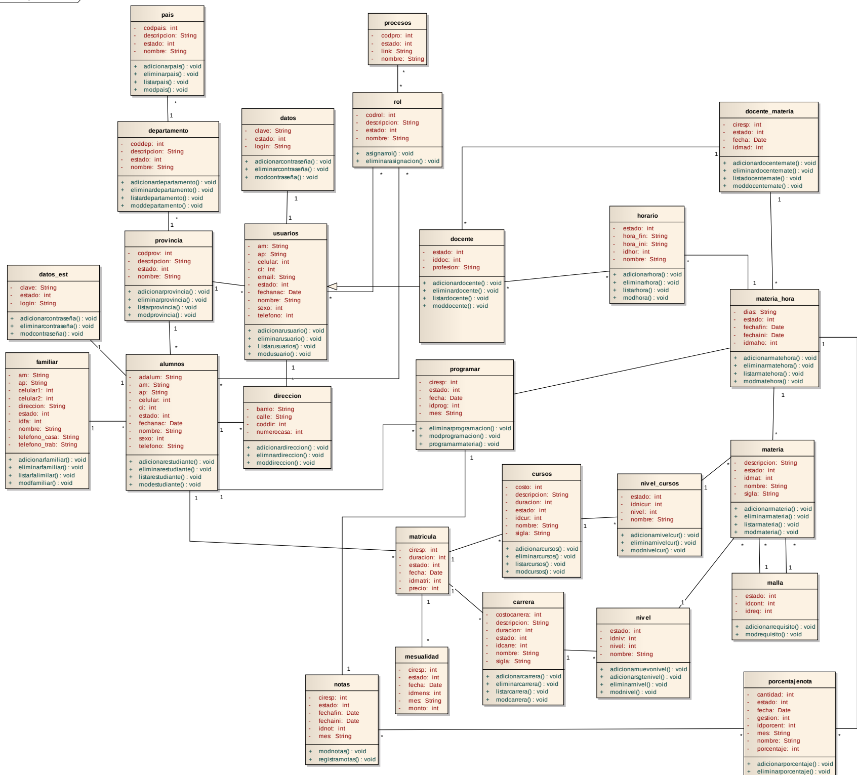
Figura 148 Diagrama de Clases
