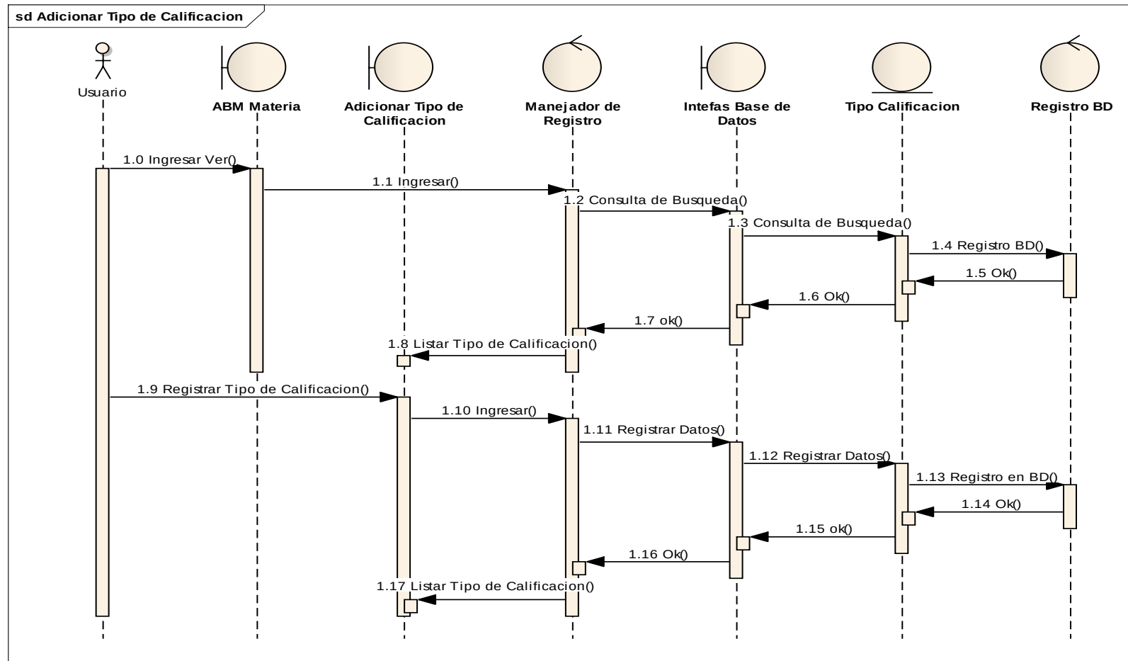
Figura 40 Adicionar tipo de Calificación
