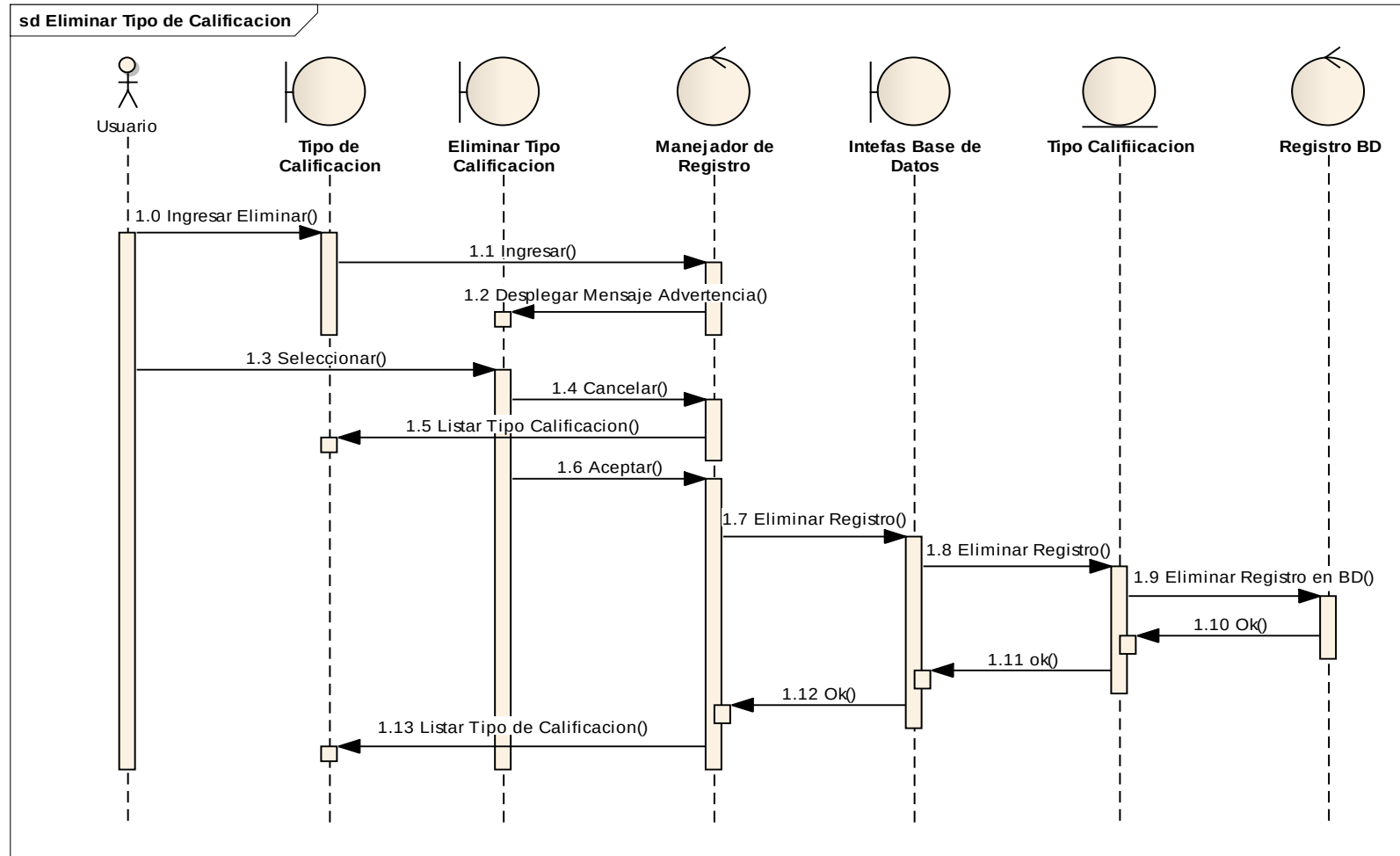
Figura 42 Eliminar Tipo de Calificación
