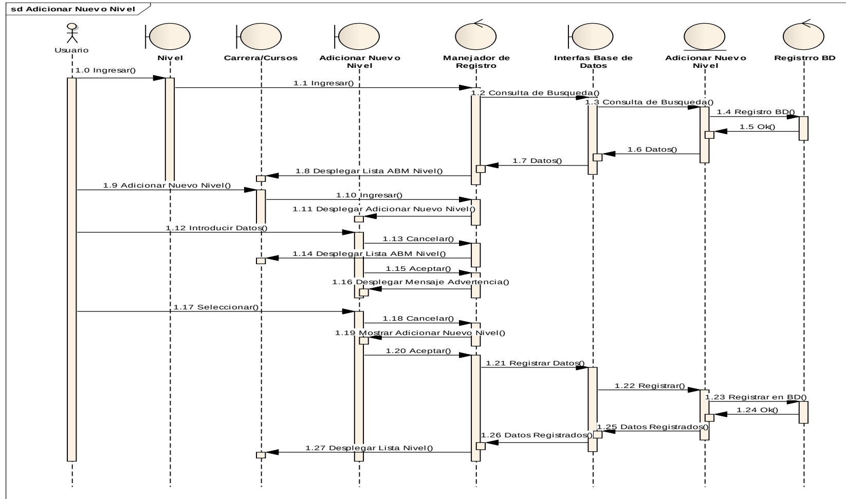
Figura 49 Adicionar Nuevo Nivel
