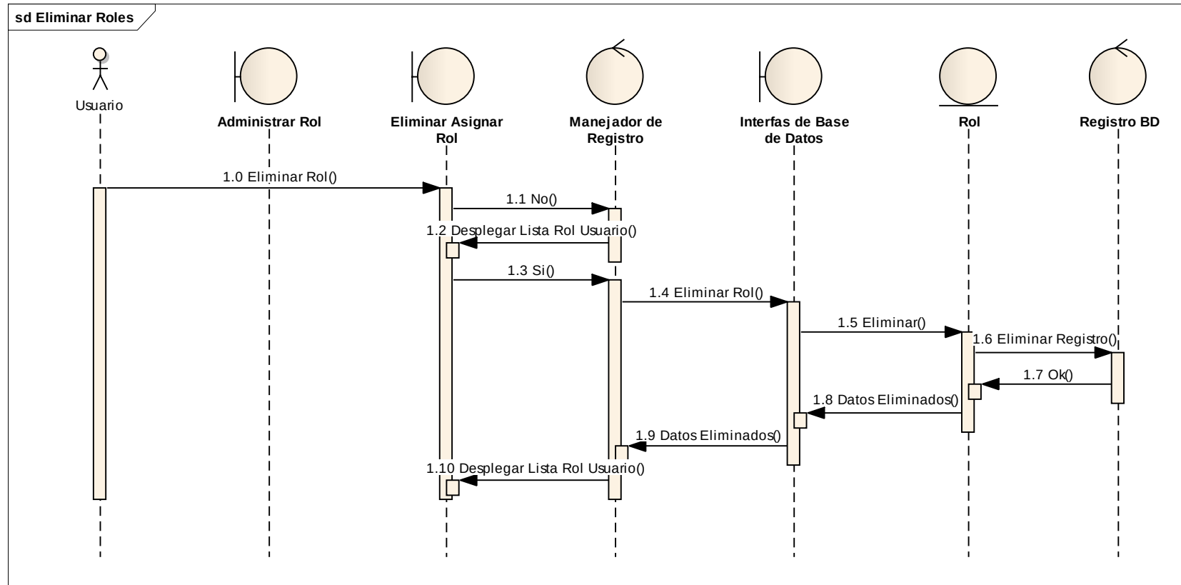
Figura 59 Eliminar Asignar Rol
