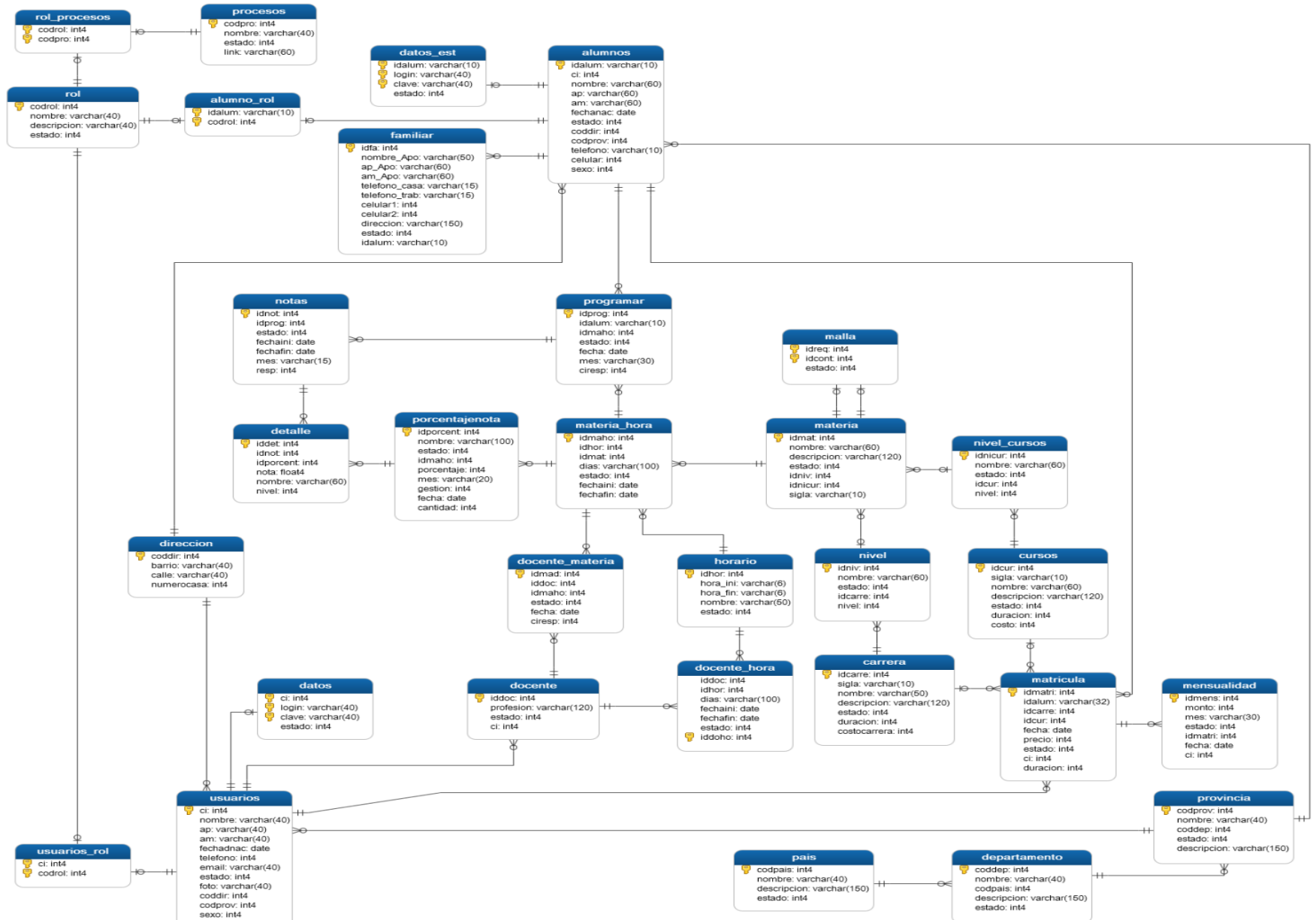
Figura 149 Diagrama de Entidad Relación
