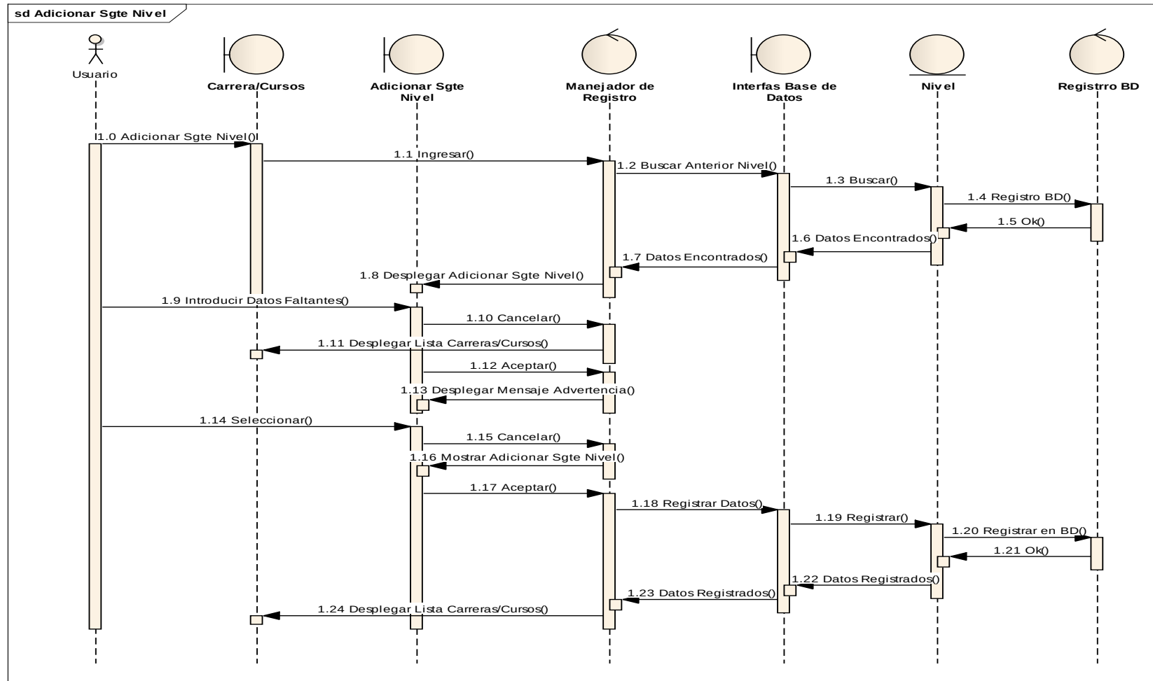
Figura 50 Adicionar sgte. Nivel
