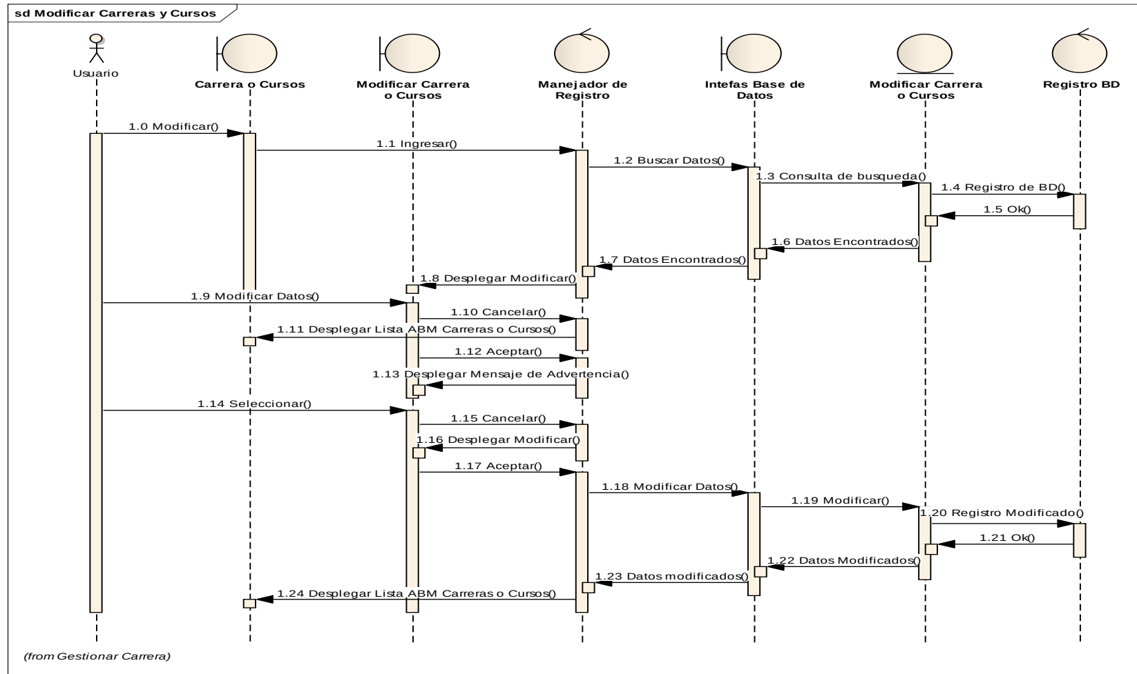
Figura 31 Modificar Carrera o Cursos
