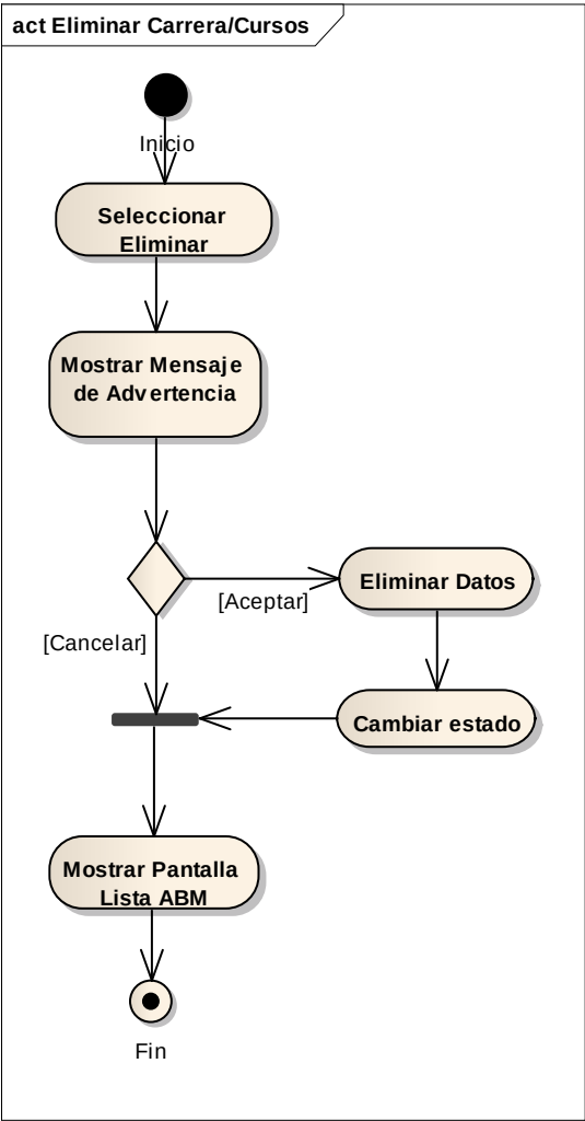
Figura 72 Eliminar Carrera y Cursos
