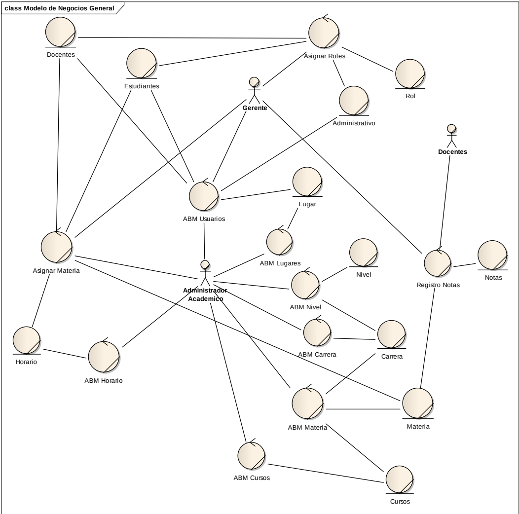
Figura 8 Caso de Uso de Negocios General
