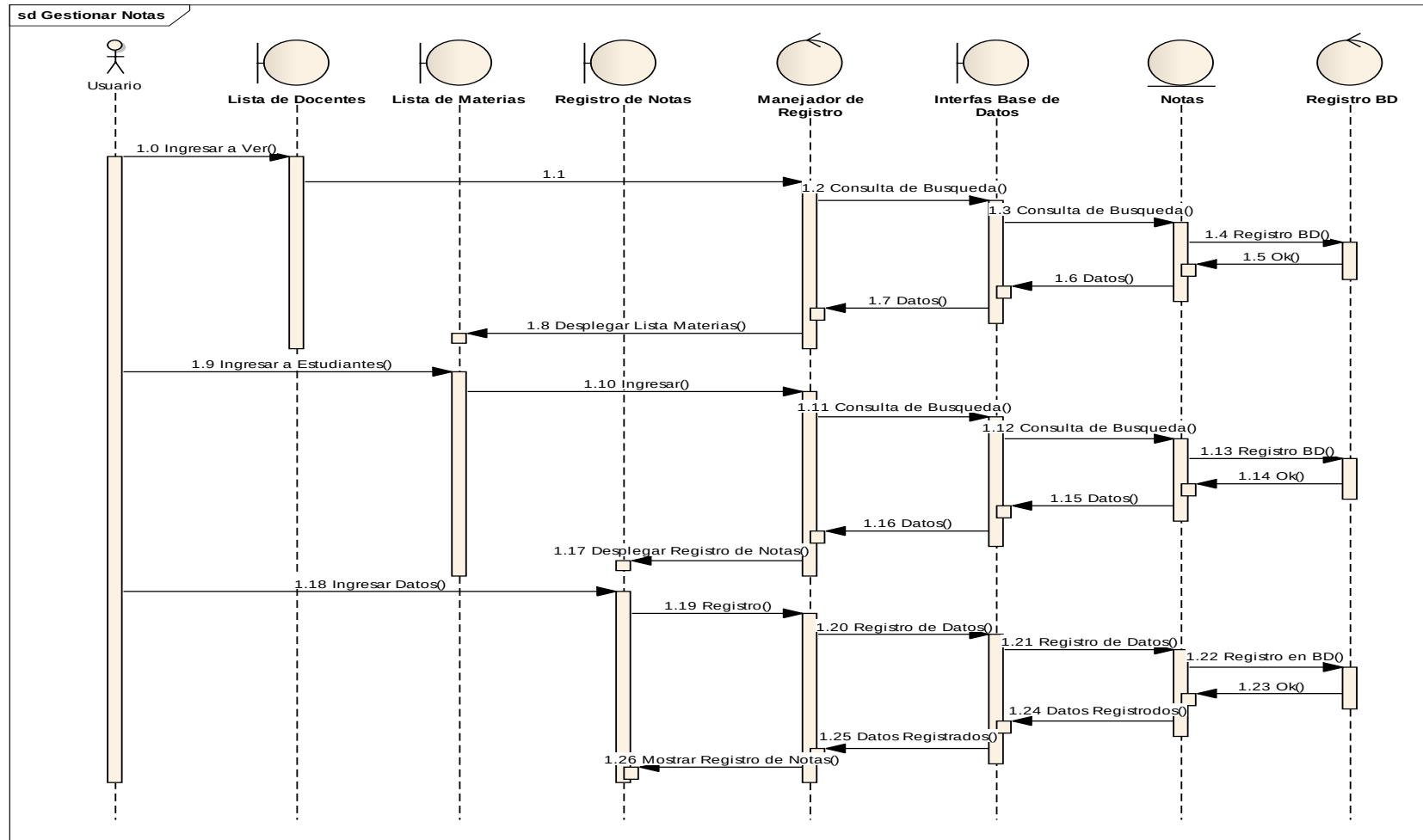
Figura 54 Registro de Notas
