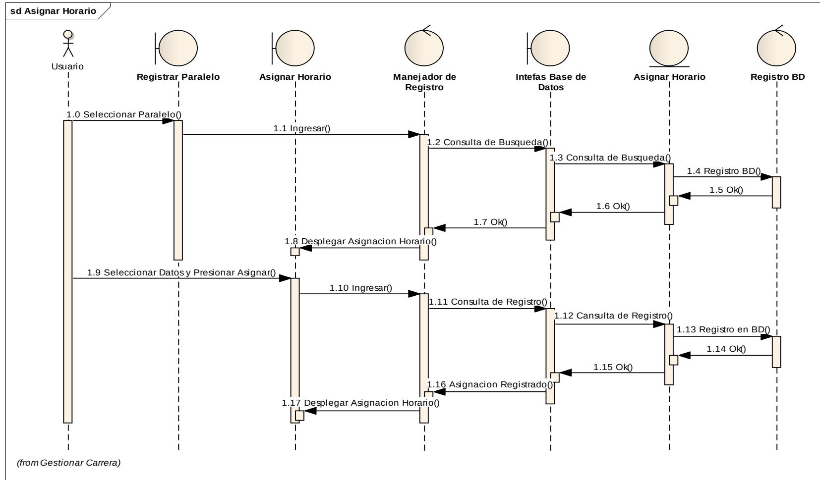
Figura 37 Asignar Horario a Paralelo
