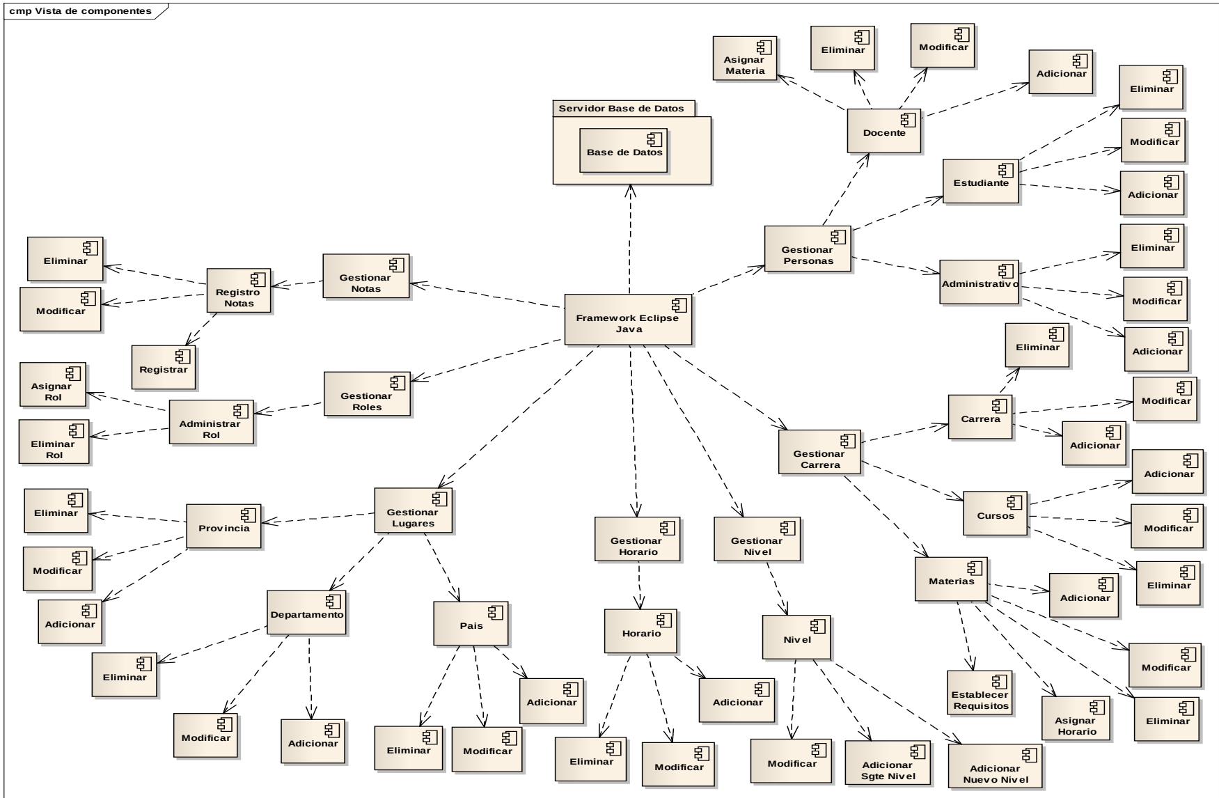
Figura 150 Diagrama de Componentes
