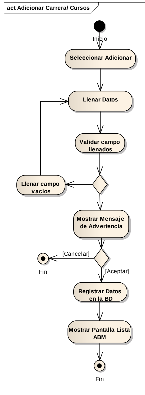
Figura 70 Adicionar Carrera y Cursos
