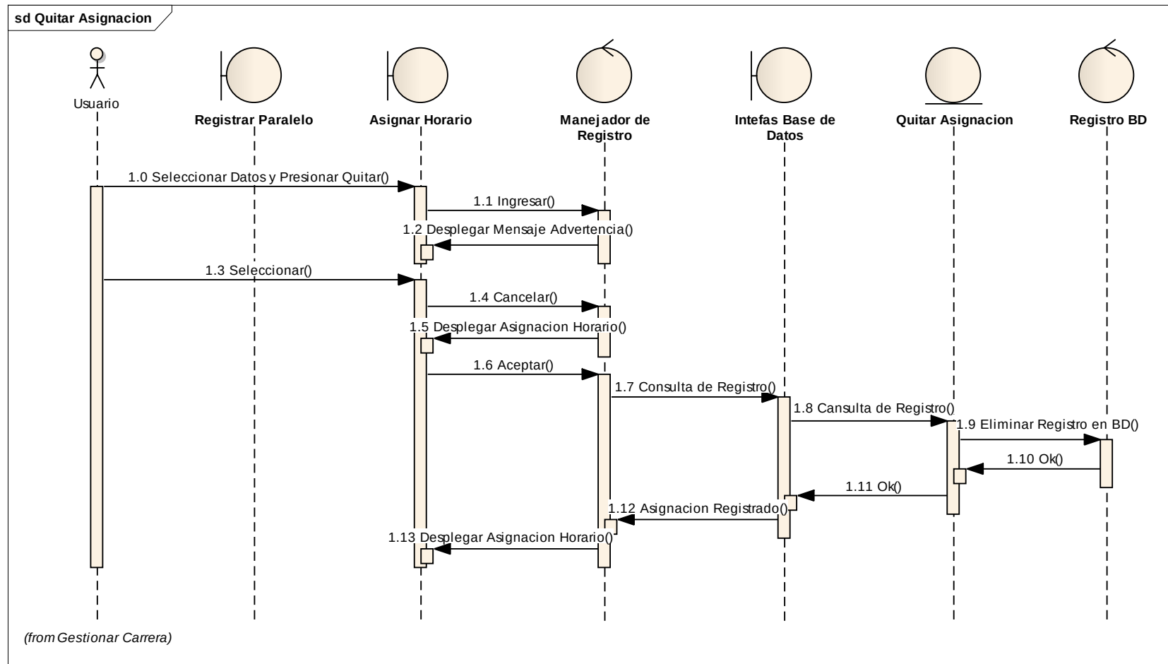
Figura 38 Quitar Asignar Horario de Paralelo
