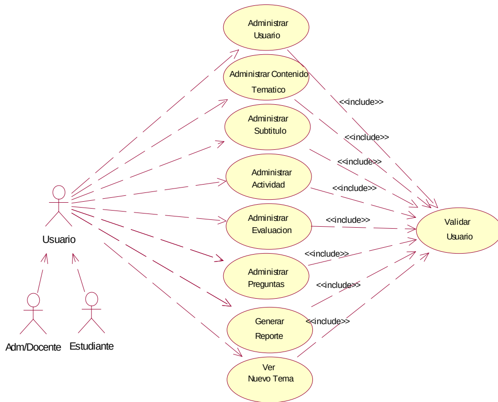
Figura 5. Diagrama de Caso de Uso General
