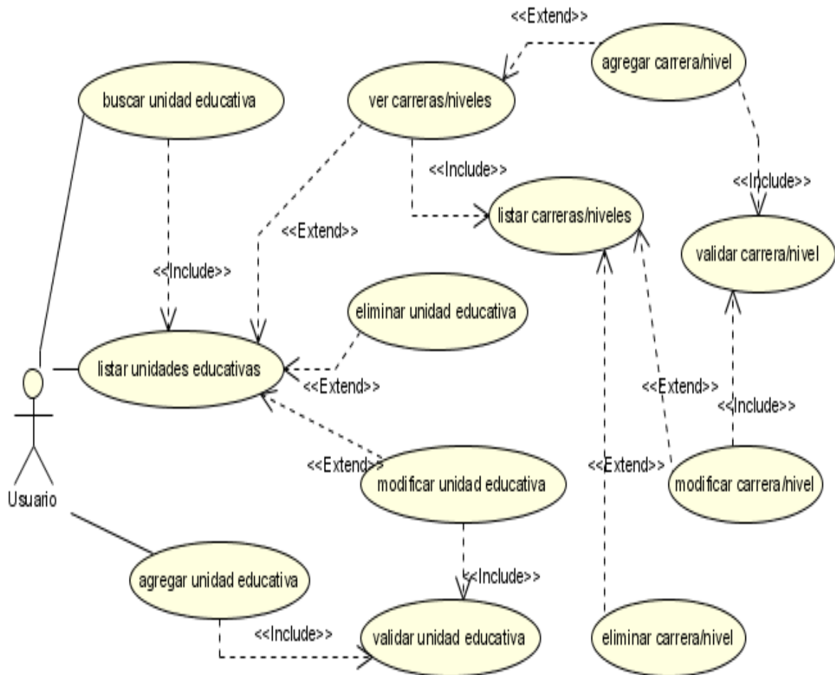
Figura N°6. Diagrama de Caso de Uso Gestionar Unidades Educativas.
