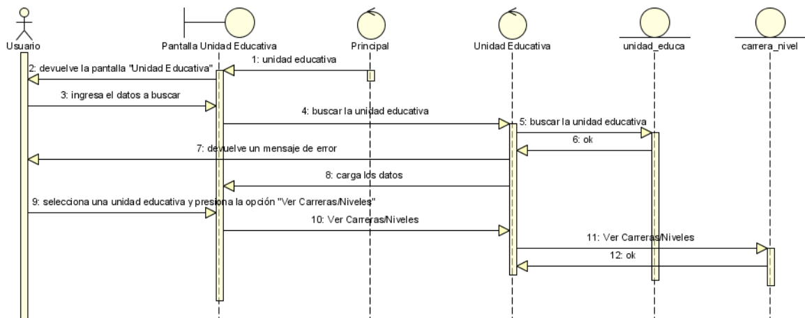
Figura N°88. Diagrama de Secuencia Ver Carreras/Niveles.
