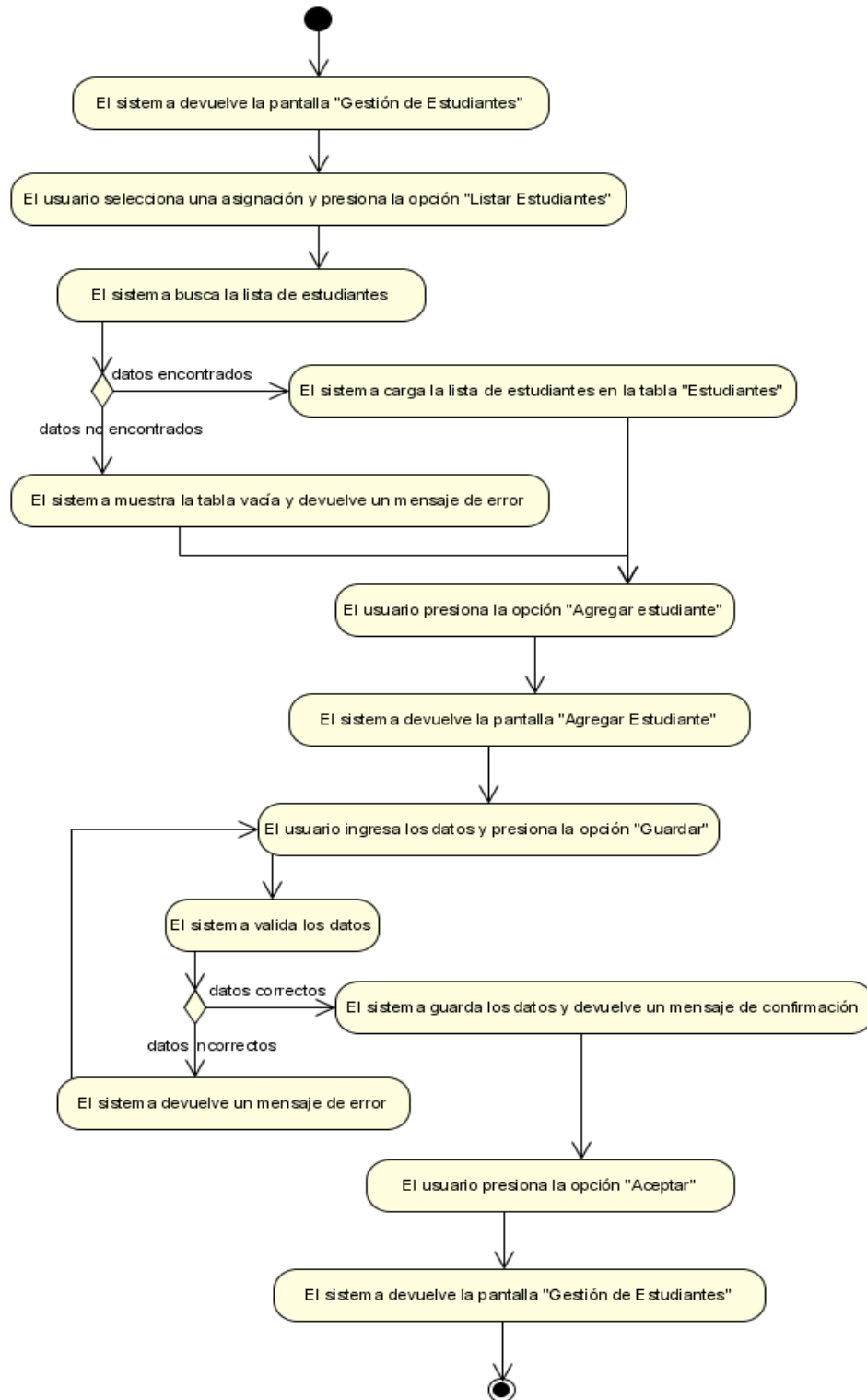
Figura N°60. Diagrama de Actividad Agregar Estudiante.
