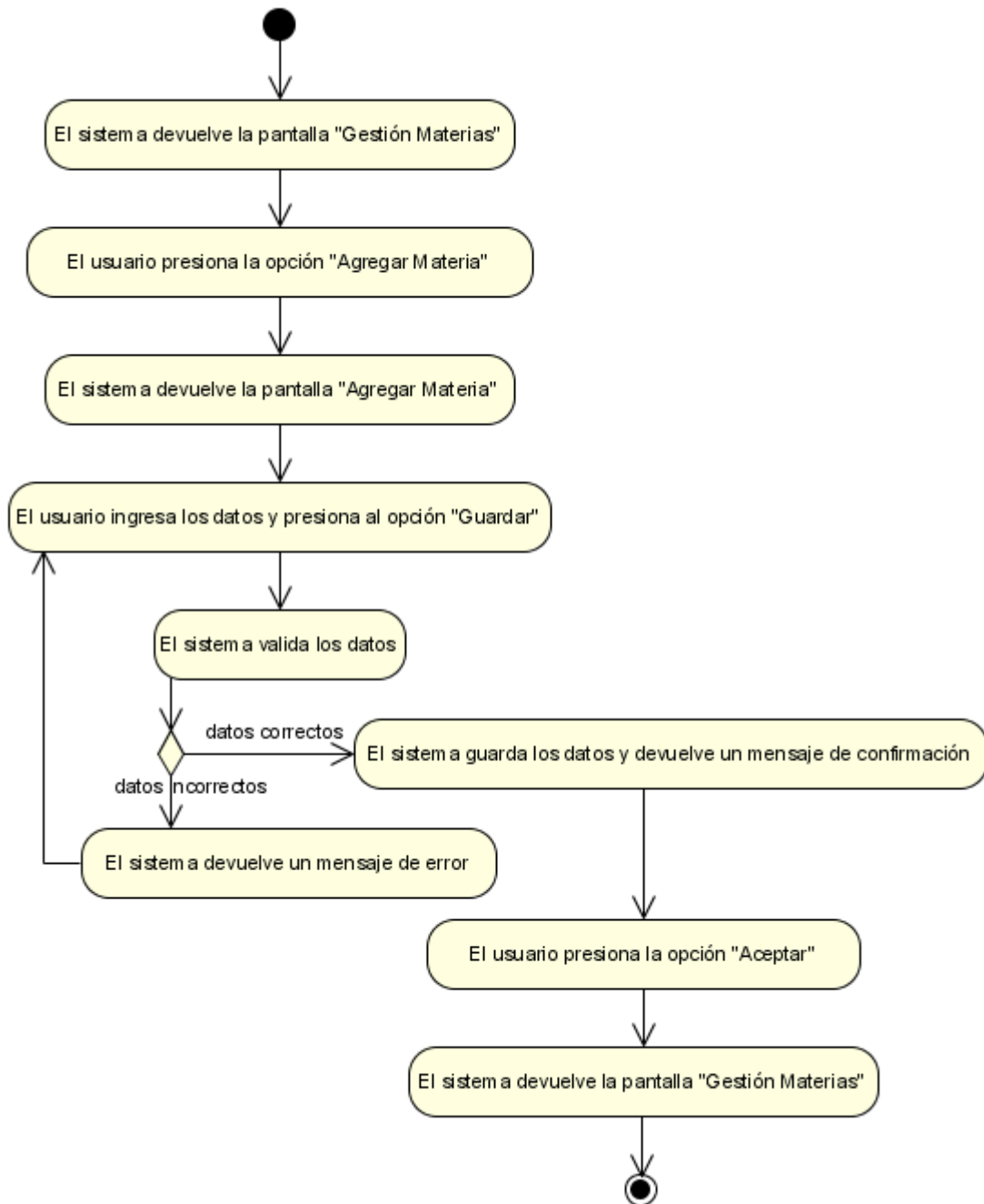
Figura N°34. Diagrama de Actividad Agregar Materia.
