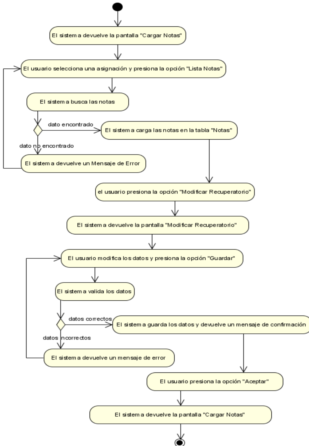
Figura N°68. Diagrama de Actividad Modificar Recuperatorio.
