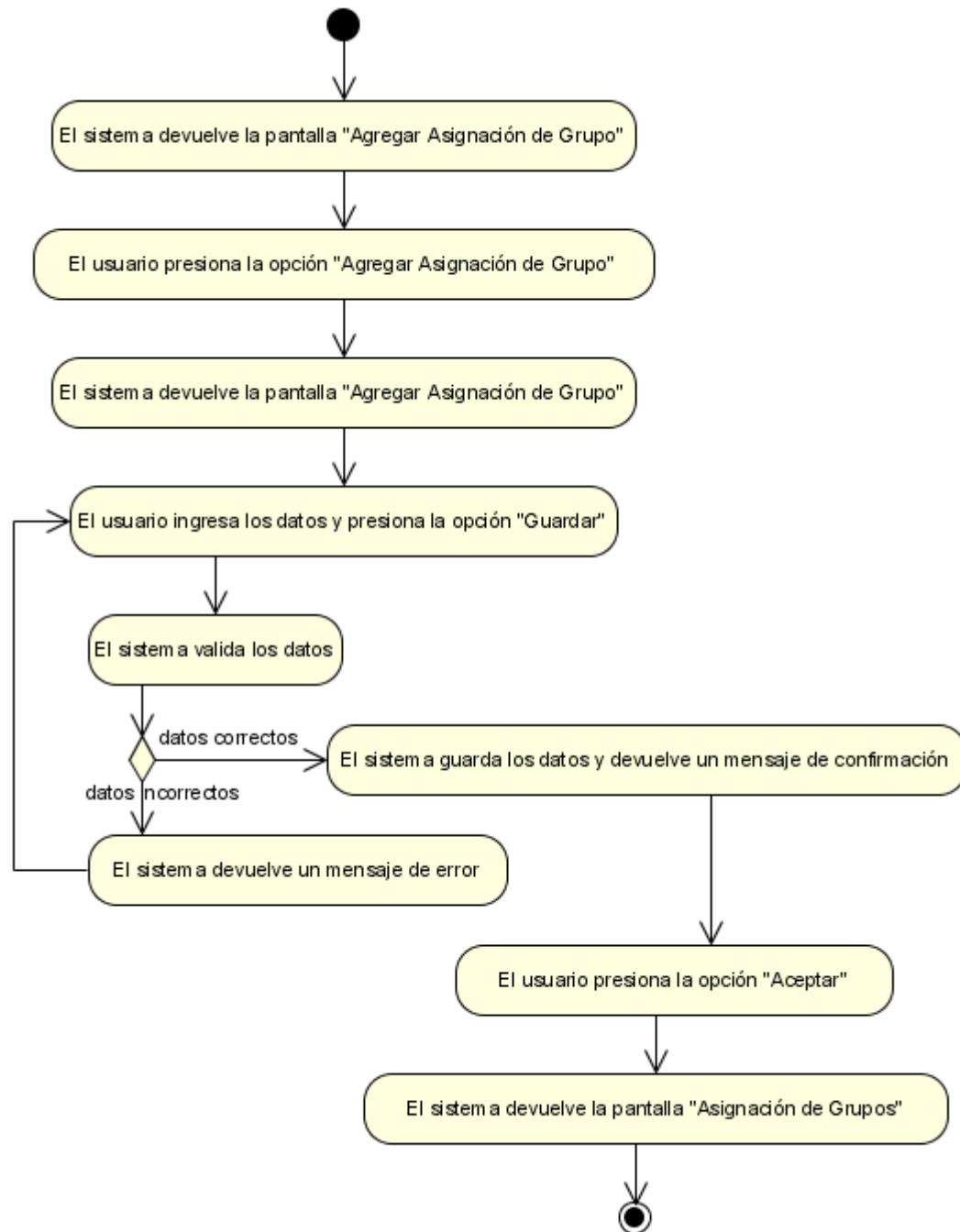
Figura N°39. Diagrama de Actividad Agregar Asignación de Grupo.
