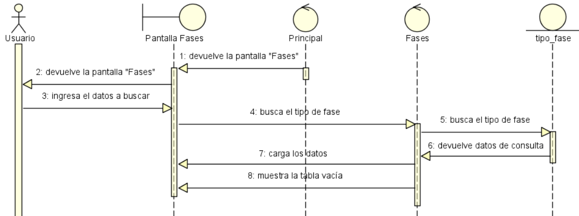
Figura N°74. Diagrama de Secuencia Listar Modelos Educativos.
