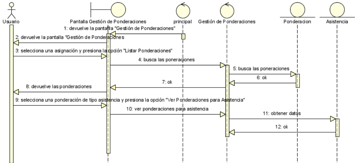
Figura N°114. Diagrama de Secuencia Ver Ponderaciones para asistencia.
