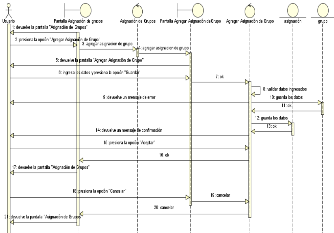
Figura N°99. Diagrama de Secuencia Agregar Asignación de Grupo.
