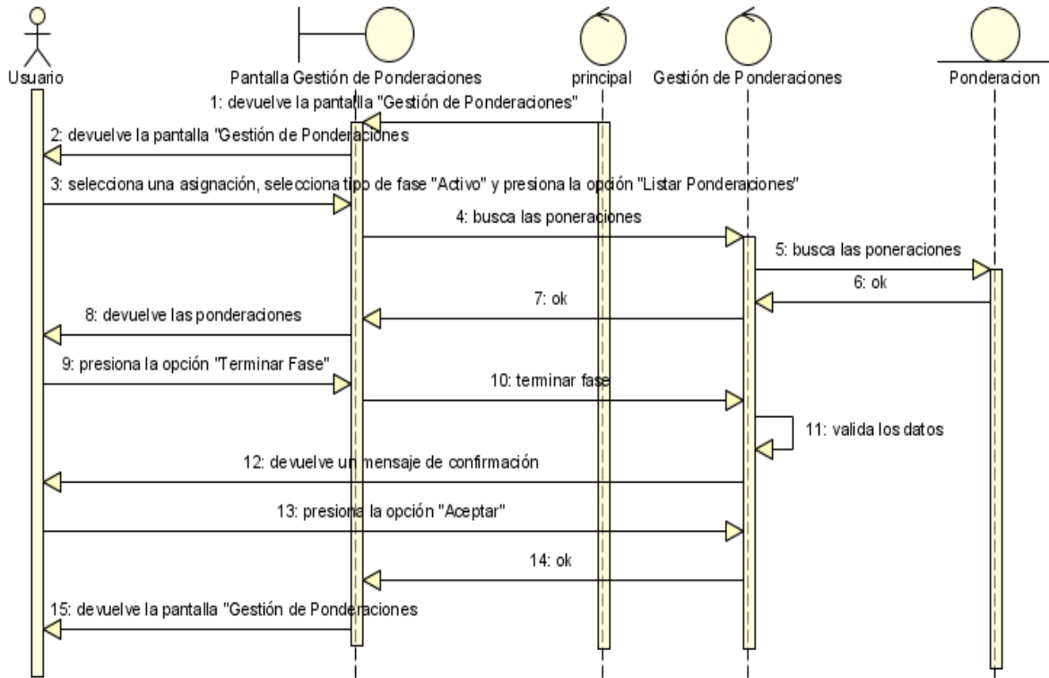
Figura N°108. Diagrama de Secuencia Terminar Fase.
