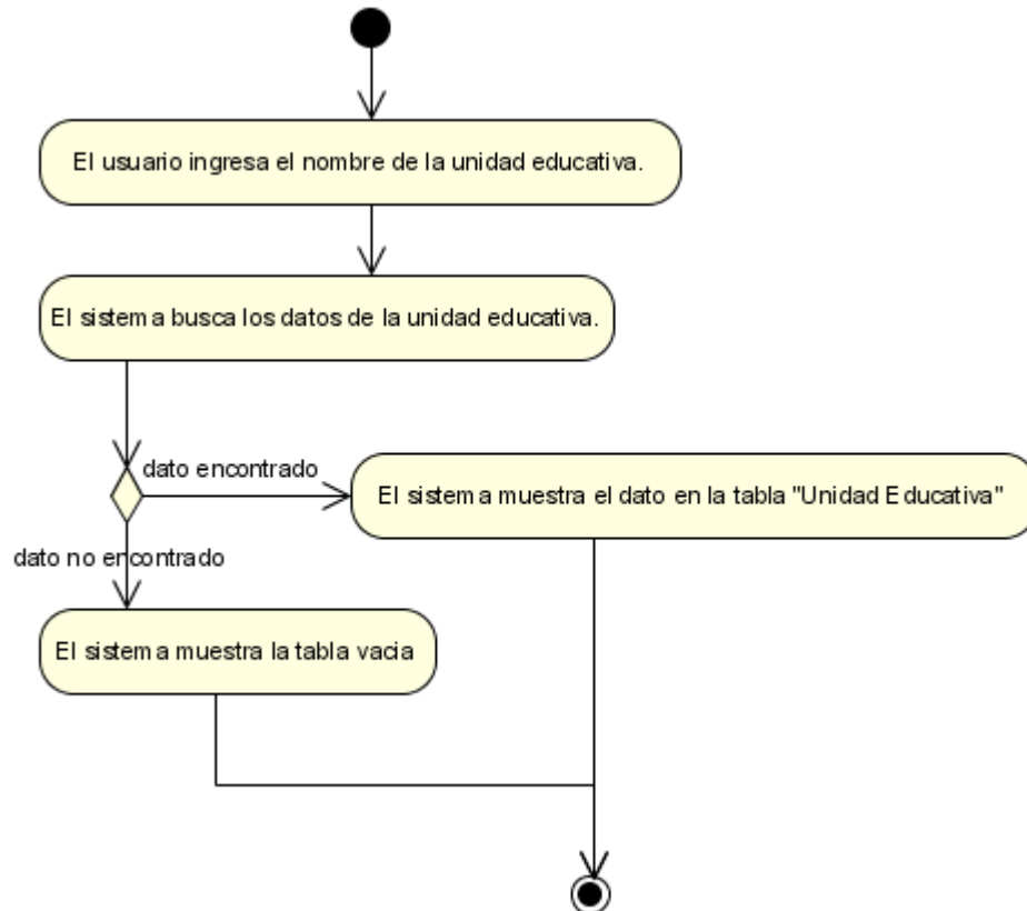
Figura N°23. Diagrama de Actividad Listar Unidades Educativas.
