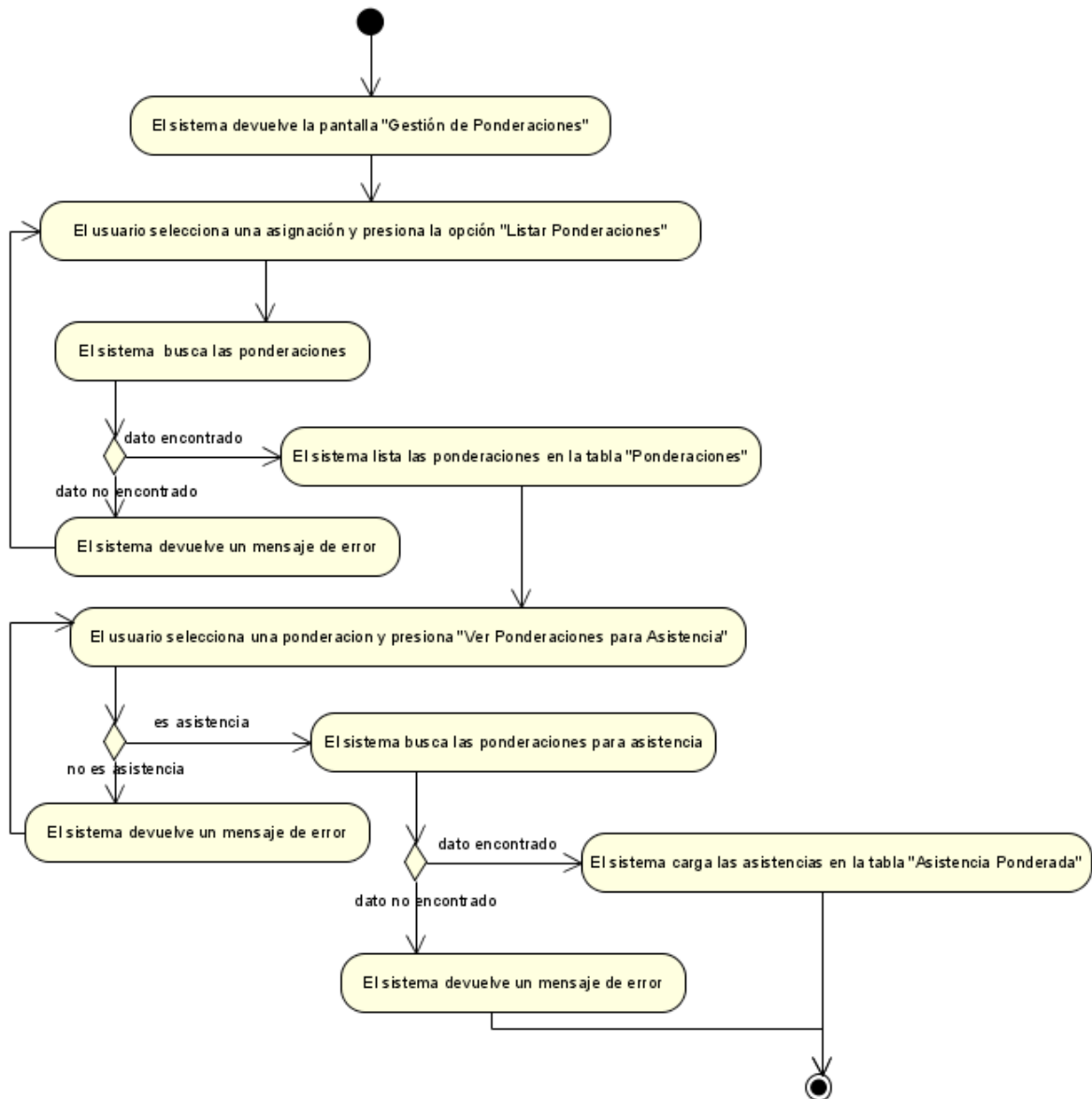
Figura N°55. Diagrama de Actividad Listar Ponderaciones de Asistencia.
