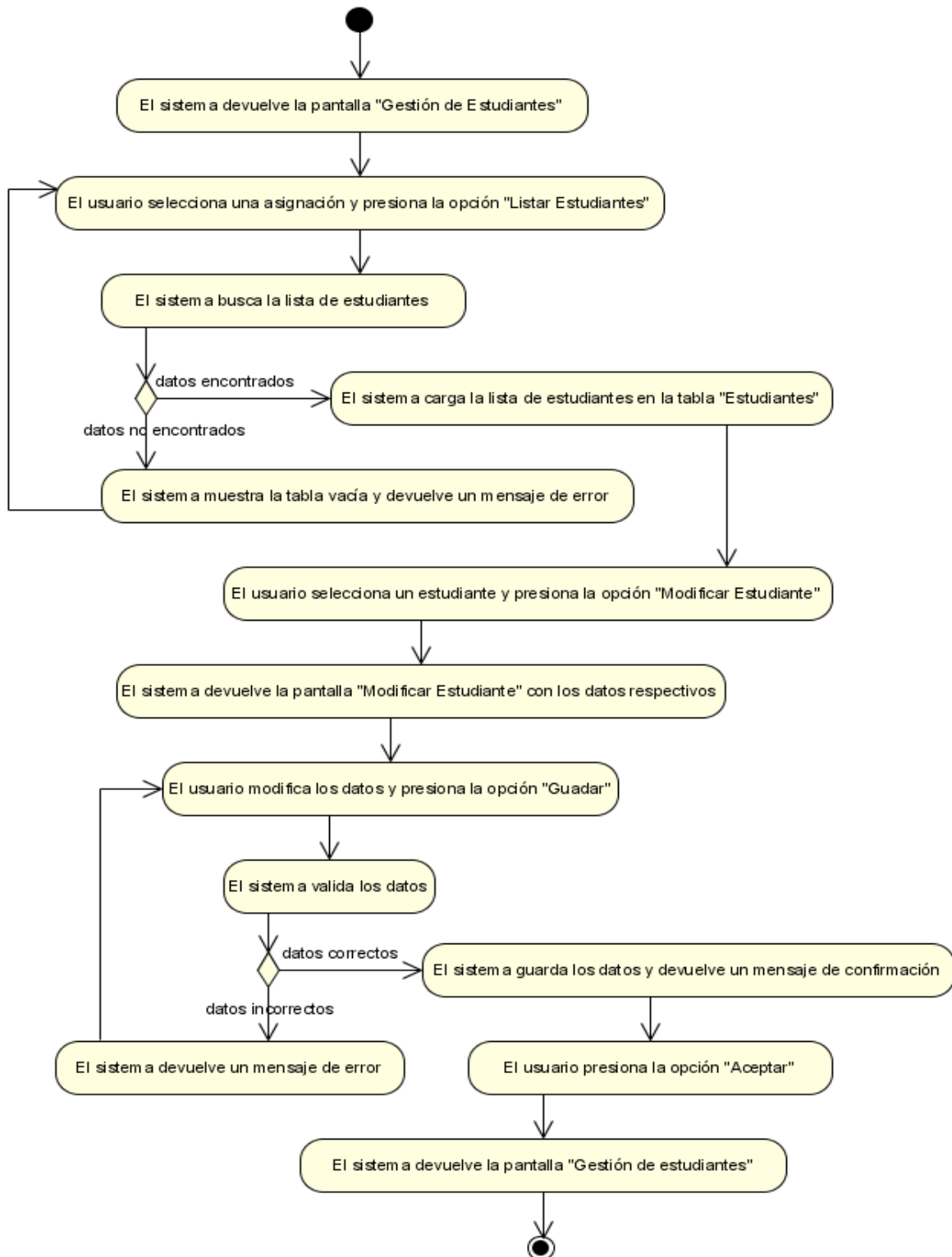
Figura N°61. Diagrama de Actividad Modificar Estudiante.
