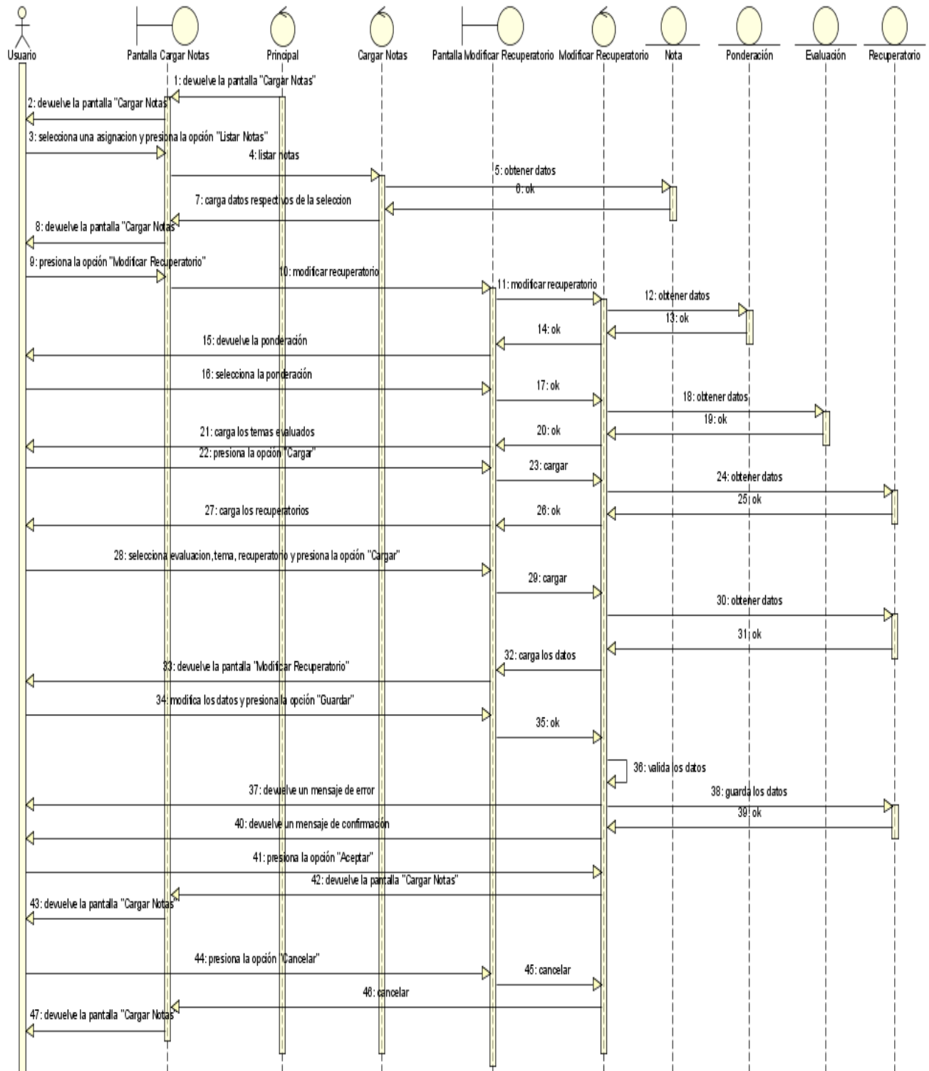
Figura N°128. Diagrama de Secuencia Modificar Recuperatorio.
