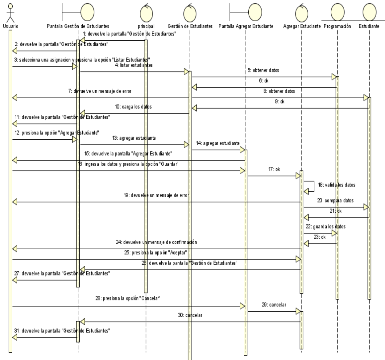
Figura N°120. Diagrama de Secuencia Agregar Estudiante.
