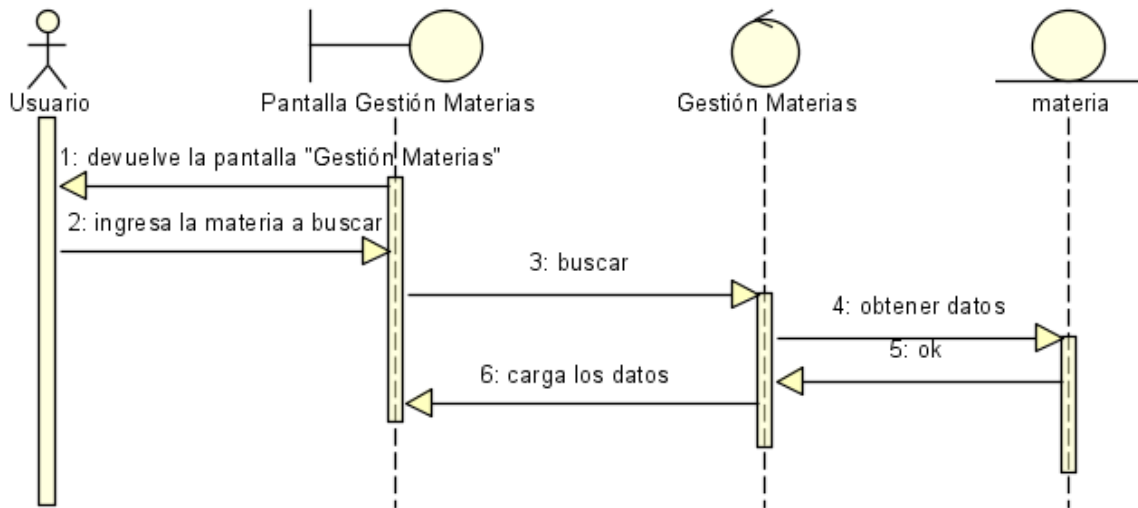
Figura N°93. Diagrama de Secuencia Listar Materias.
