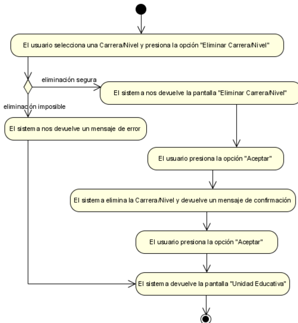
Figura N°31. Diagrama de Actividad Eliminar Carrera/Nivel.
