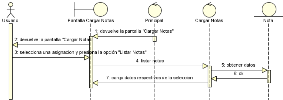
Figura N°123. Diagrama de Secuencia Listar Notas.
