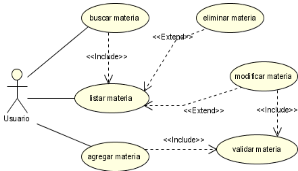
Figura N°7. Diagrama de Caso de Uso Gestionar Materias.
