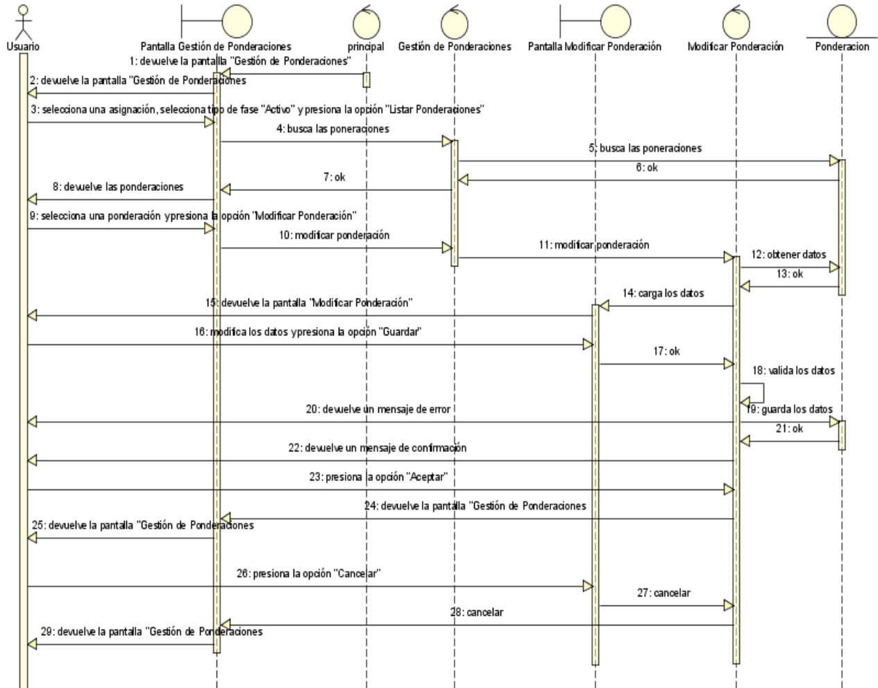
Figura N°111. Diagrama de Secuencia Modificar Ponderación.
