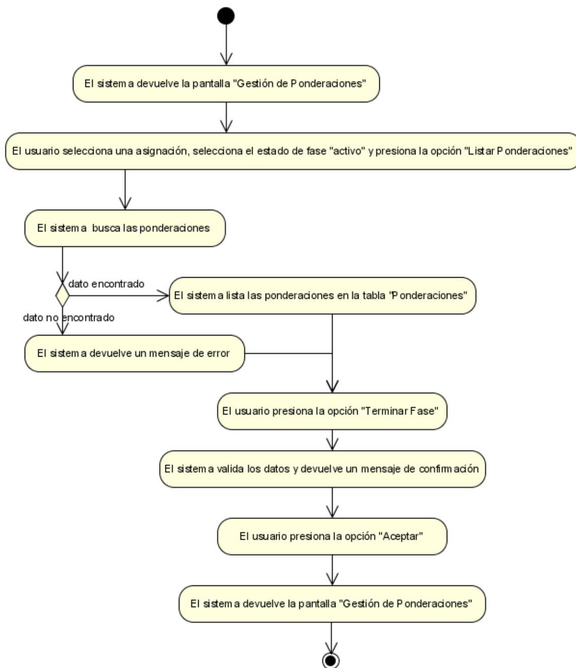
Figura N°49. Diagrama de Actividad Terminar Fase.
