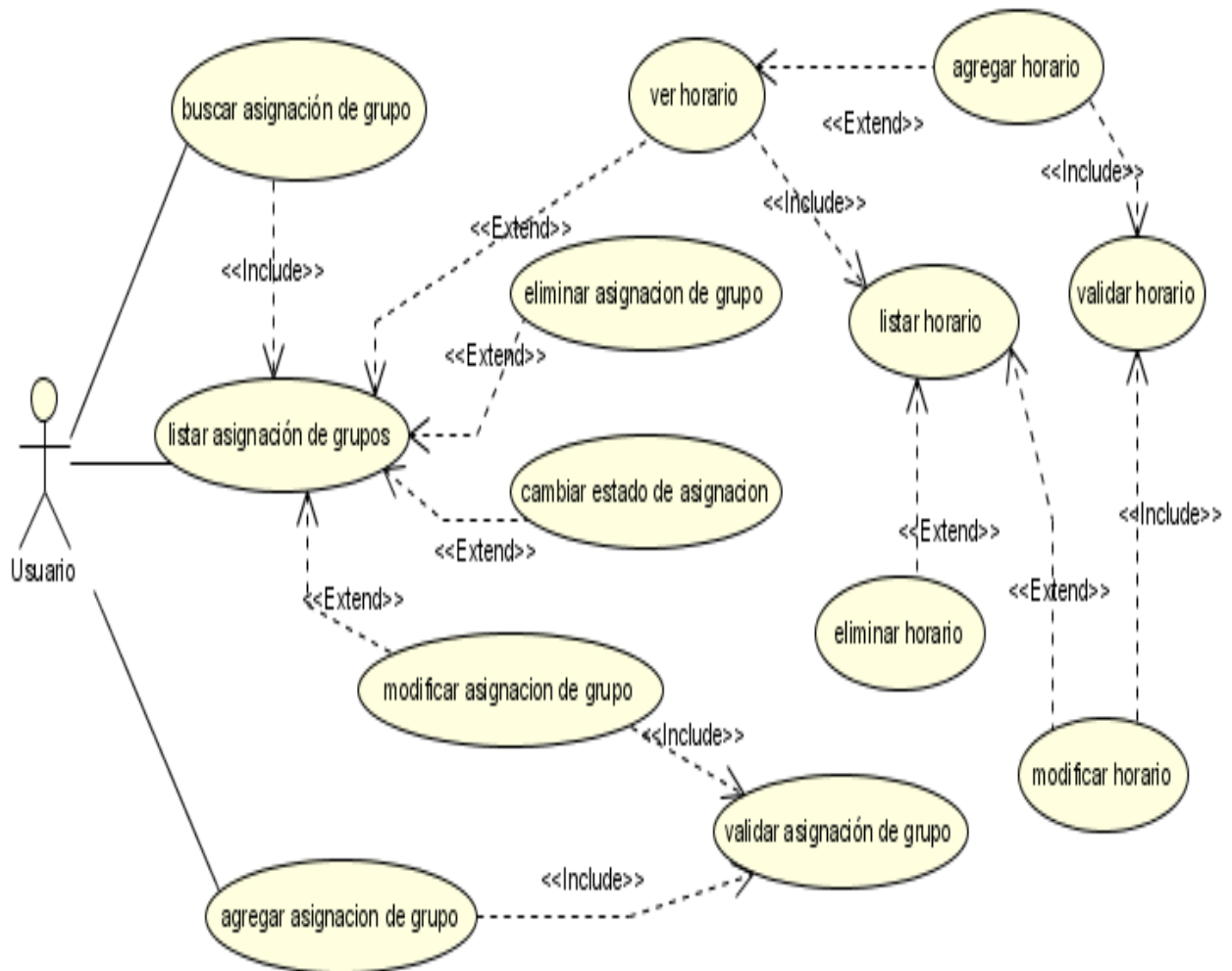
Figura N°8. Diagrama de Caso de Uso Gestionar Asignación de Grupos.
