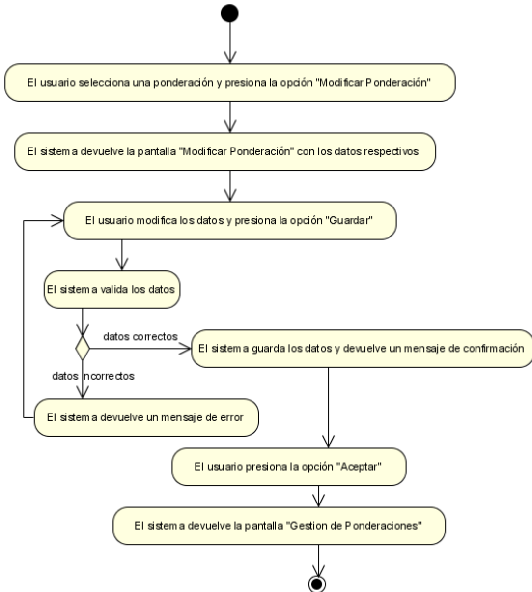
Figura N°51. Diagrama de Actividad Modificar Ponderación.
