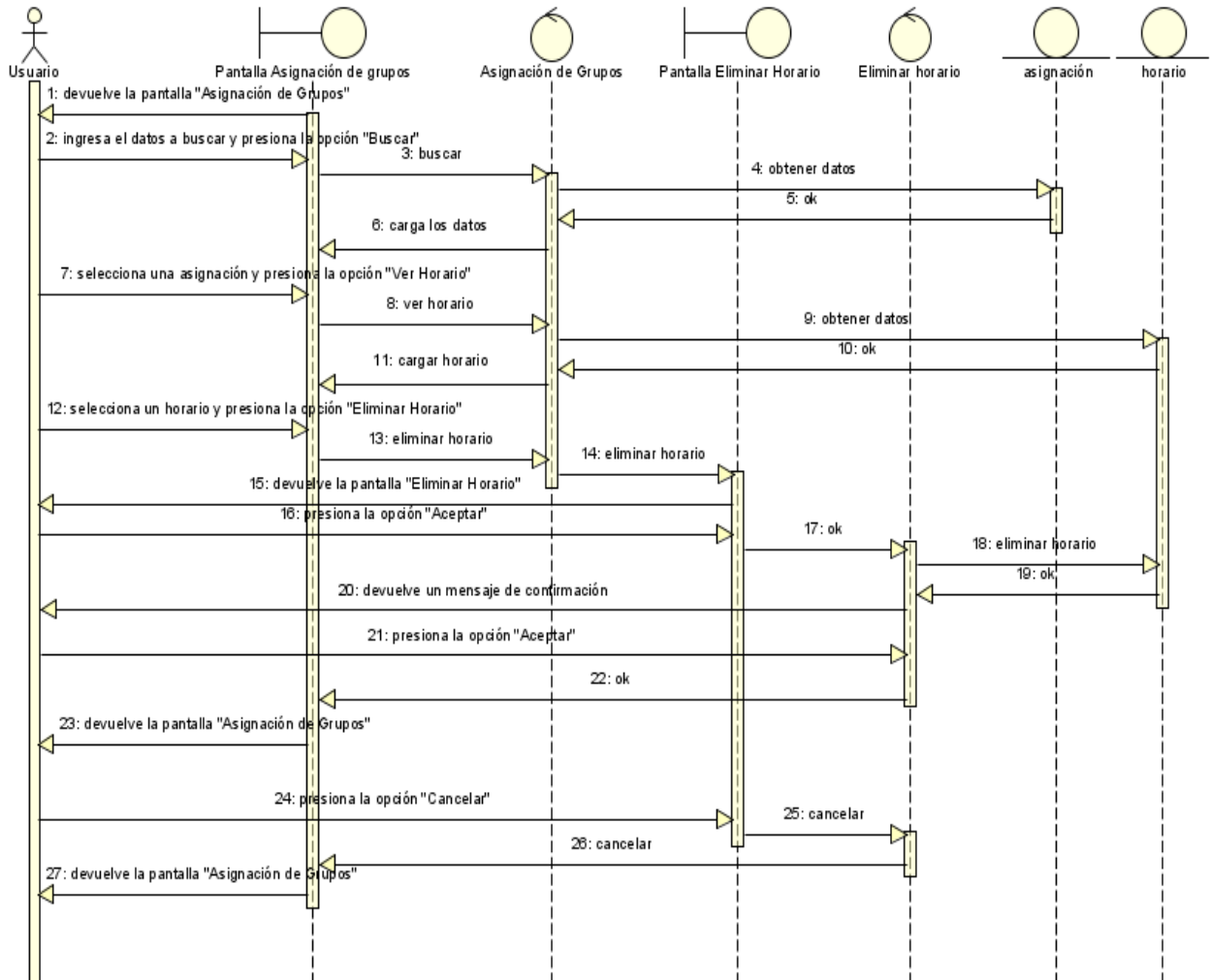
Figura N°107. Diagrama de Secuencia Eliminar horario.
