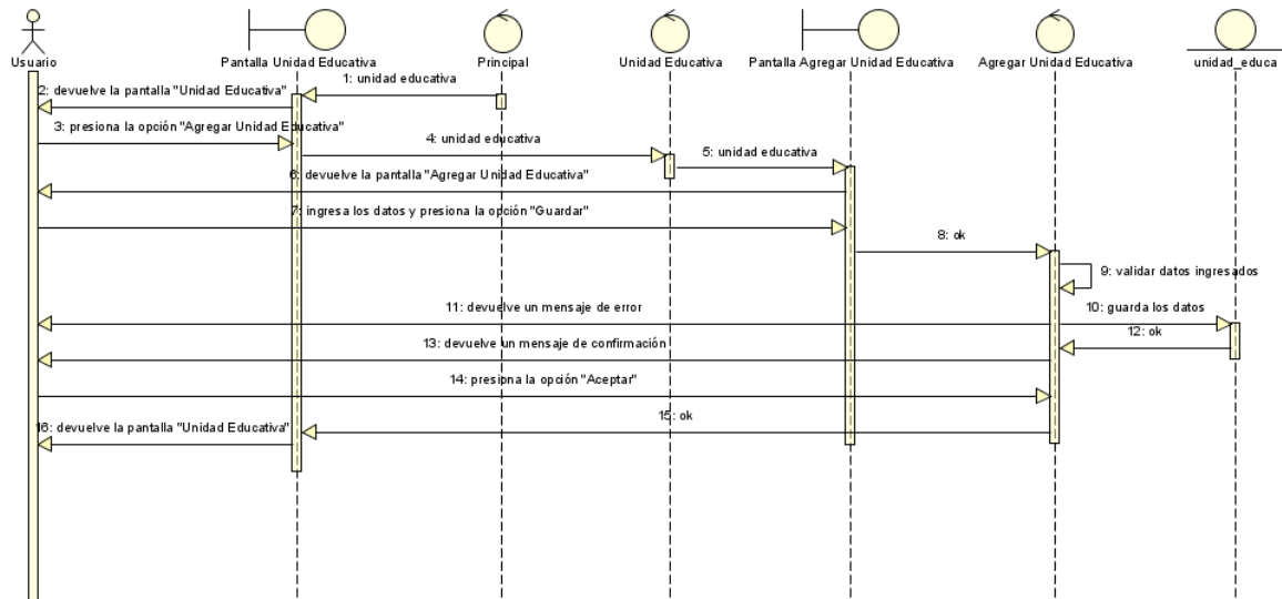
Figura N°85. Diagrama de Secuencia Agregar Unidad Educativa.
