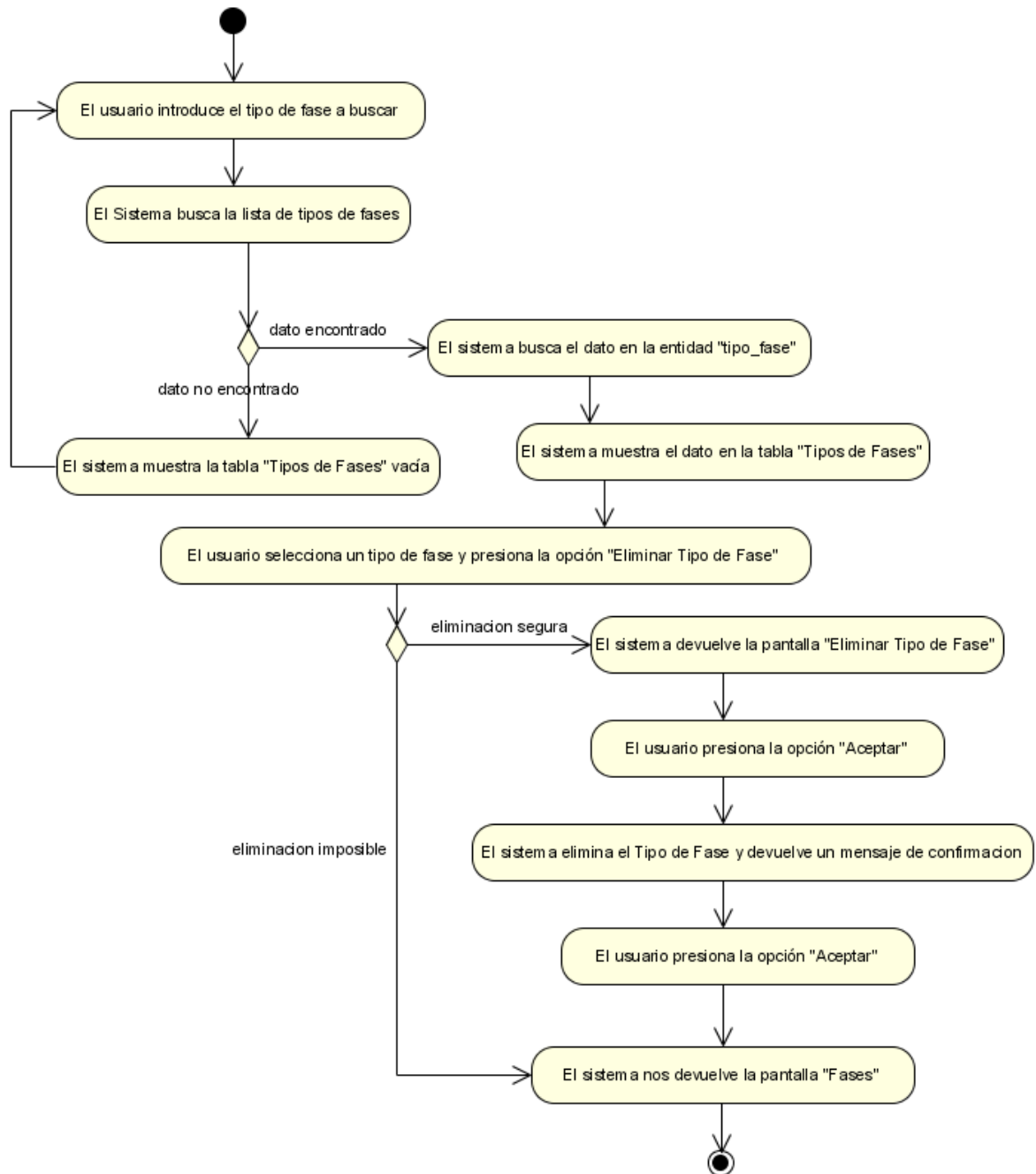
Figura N°16. Diagrama de Actividad Eliminar Modelo Educativo.
