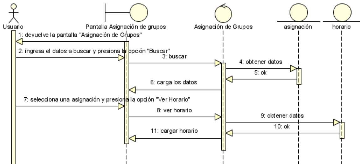
Figura N°104. Diagrama de Secuencia Listar Horario.
