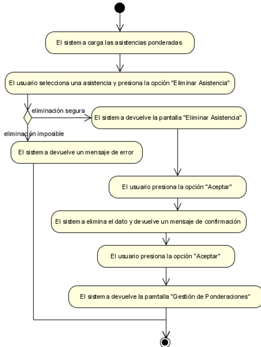
Figura N°57. Diagrama de Actividad .Eliminar Asistencia.
