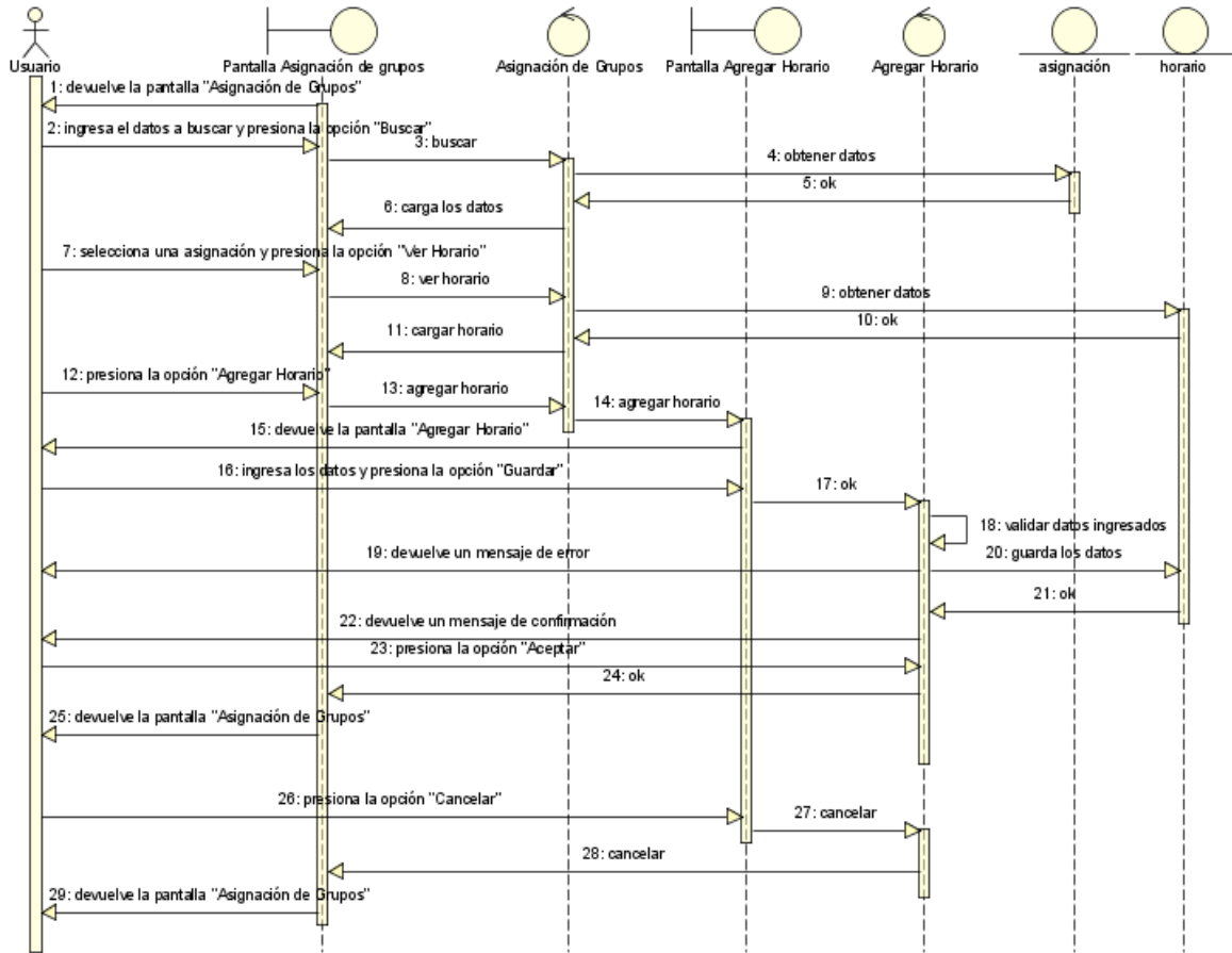
Figura N°105. Diagrama de Secuencia Agregar Horario.
