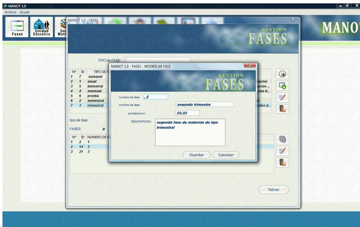
Figura N°142. Pantalla Modificar Fase.
