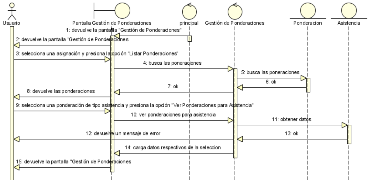
Figura N°115. Diagrama de Secuencia Listar Ponderaciones de Asistencia.
