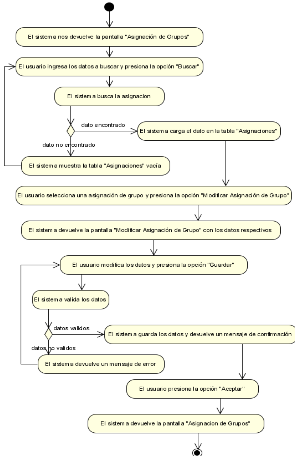
Figura N°40. Diagrama de Actividad Modificar Asignación de Grupo.
