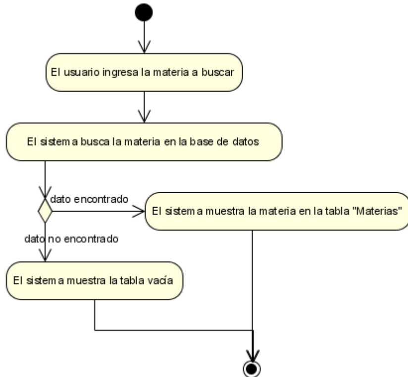
Figura N°33. Diagrama de Actividad Listar Materia.
