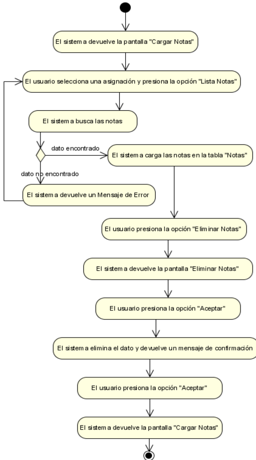
Figura N°66. Diagrama de Actividad Eliminar Notas.
