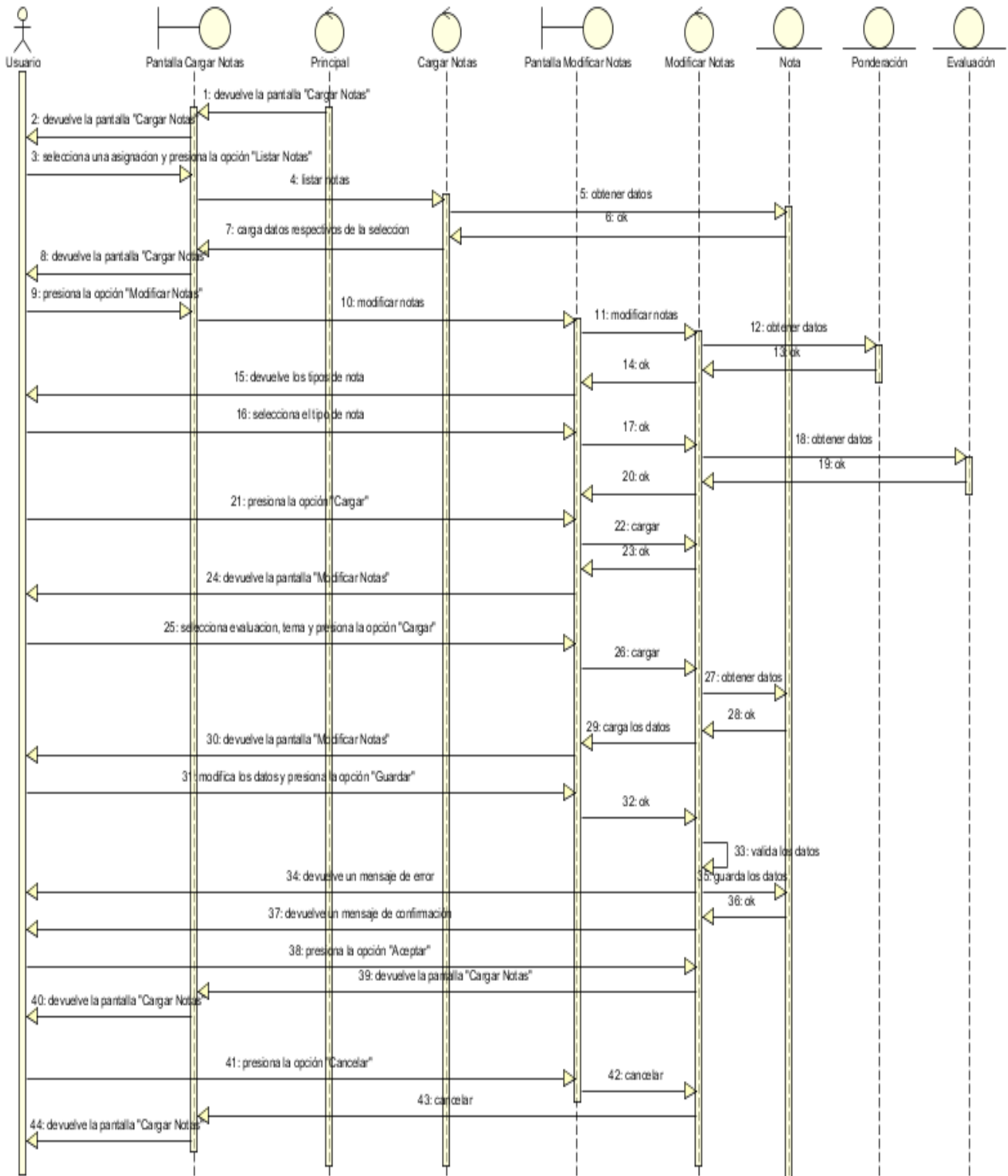
Figura N°125. Diagrama de Secuencia Modificar Notas.
