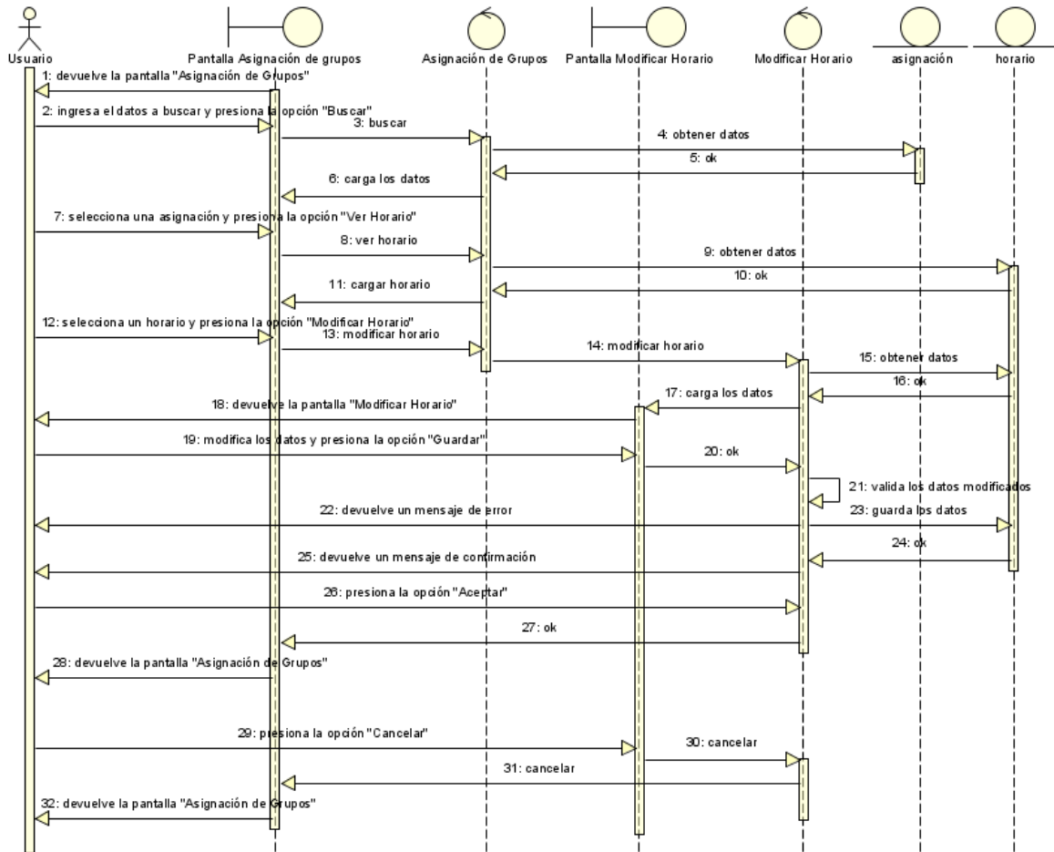
Figura N°106. Diagrama de Secuencia Modificar Horario.
