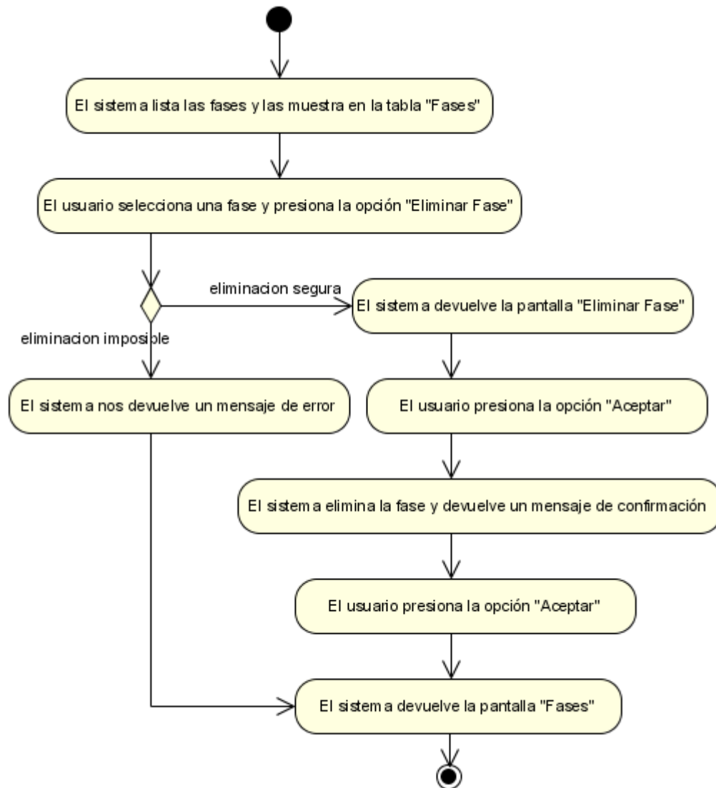
Figura N°21. Diagrama de Actividad Eliminar Fase.
