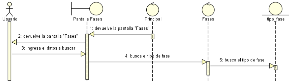
Figura N°73. Diagrama de Secuencia Buscar Modelos Educativos.
