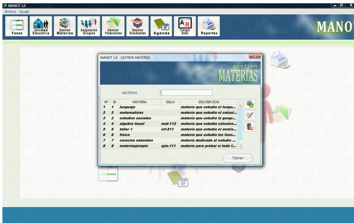
Figura N°152. Pantalla: Gestion Materias.
