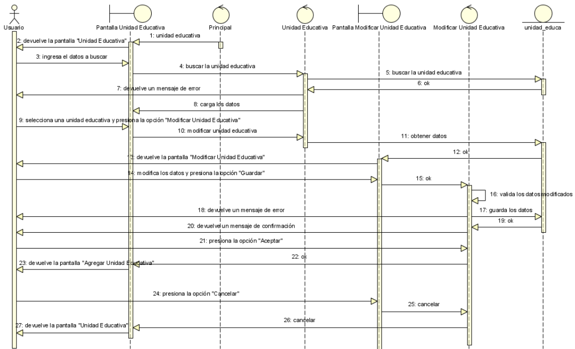
Figura N°86. Diagrama de Secuencia Modificar Unidad Educativa.
