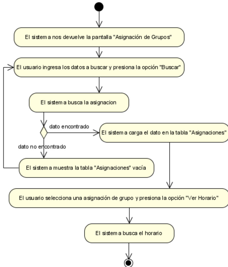
Figura N°43. Diagrama de Actividad Ver Horario.
