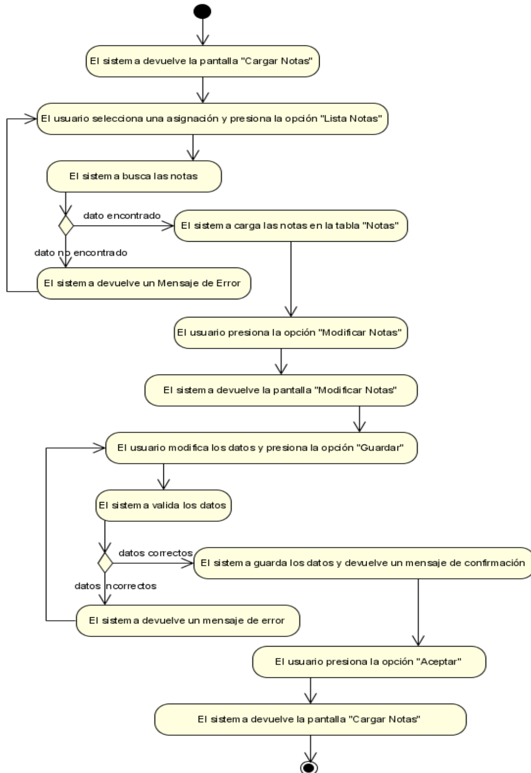
Figura N°65. Diagrama de Actividad Modificar Notas.
