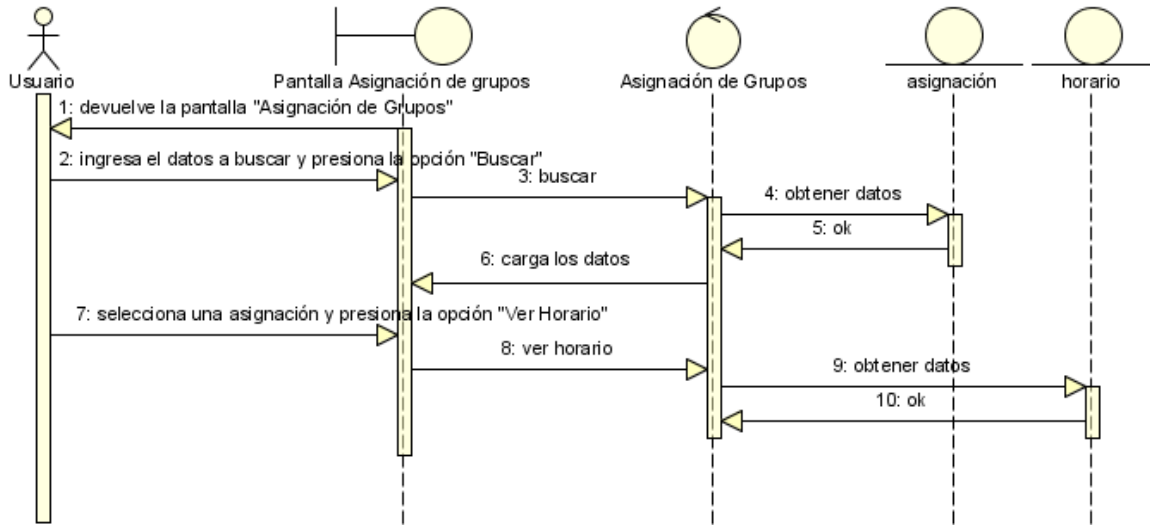
Figura N°103. Diagrama de Secuencia Ver Horario.
