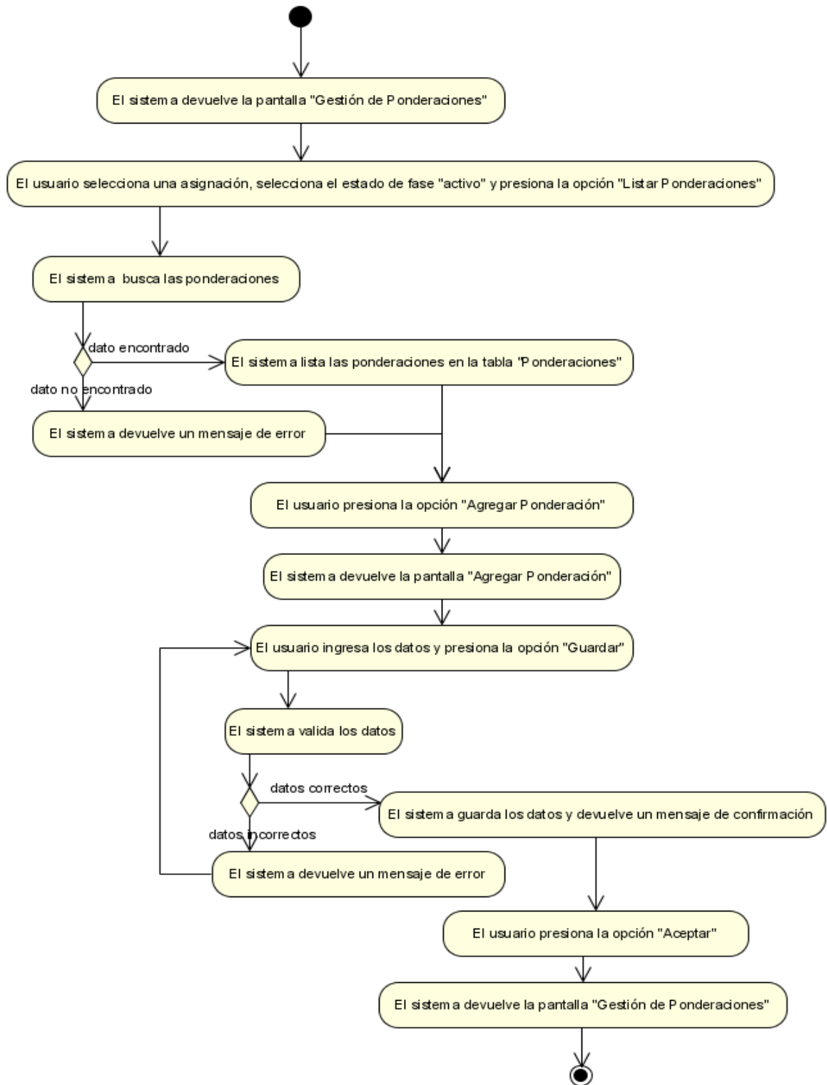
Figura N°50. Diagrama de Actividad Agregar Ponderación.
