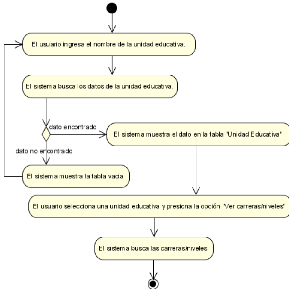
Figura N°27. Diagrama de Actividad Ver Carreras/Niveles.
