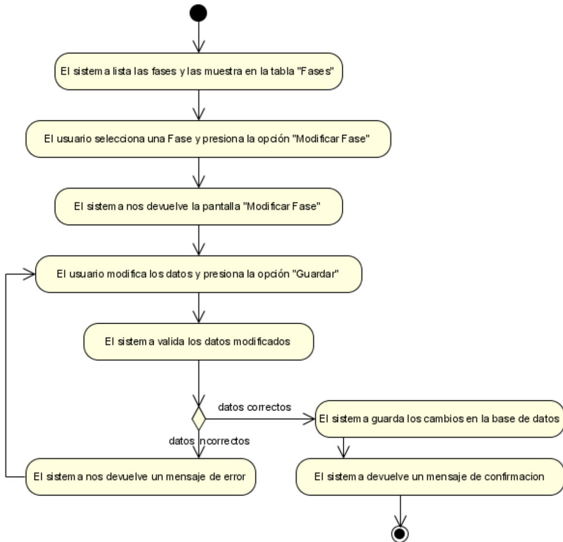
Figura N°20. Diagrama de Actividad Modificar Fase.
