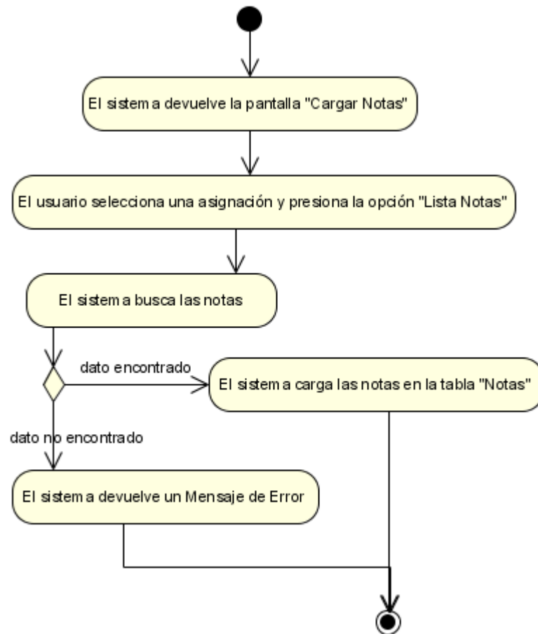
Figura N°63. Diagrama de Actividad Listar Notas.
