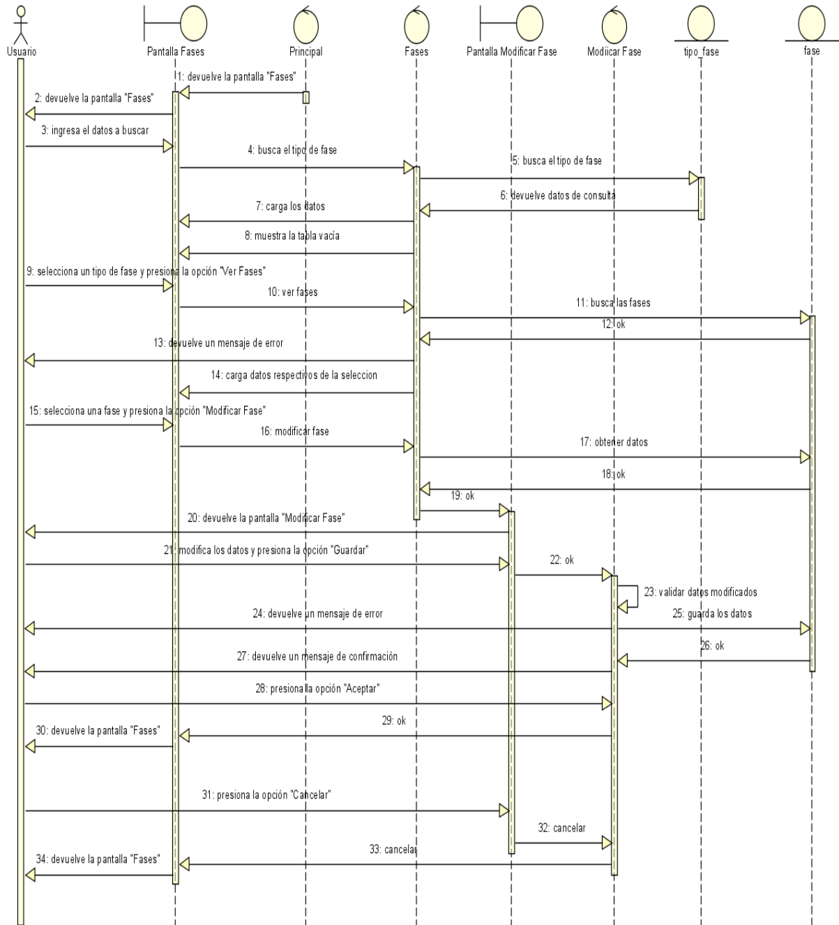
Figura N°81. Diagrama de Secuencia Modificar Fase.
