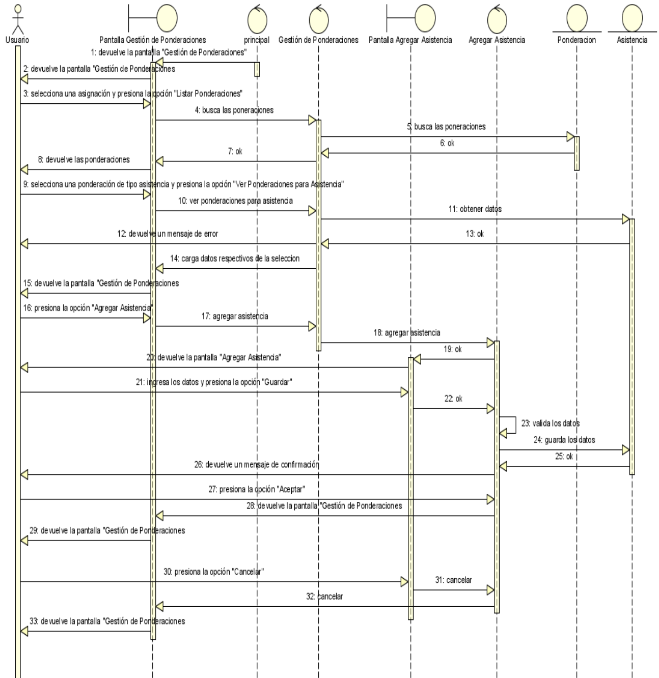
Figura N°113. Diagrama de Secuencia Agregar Asistencia.
