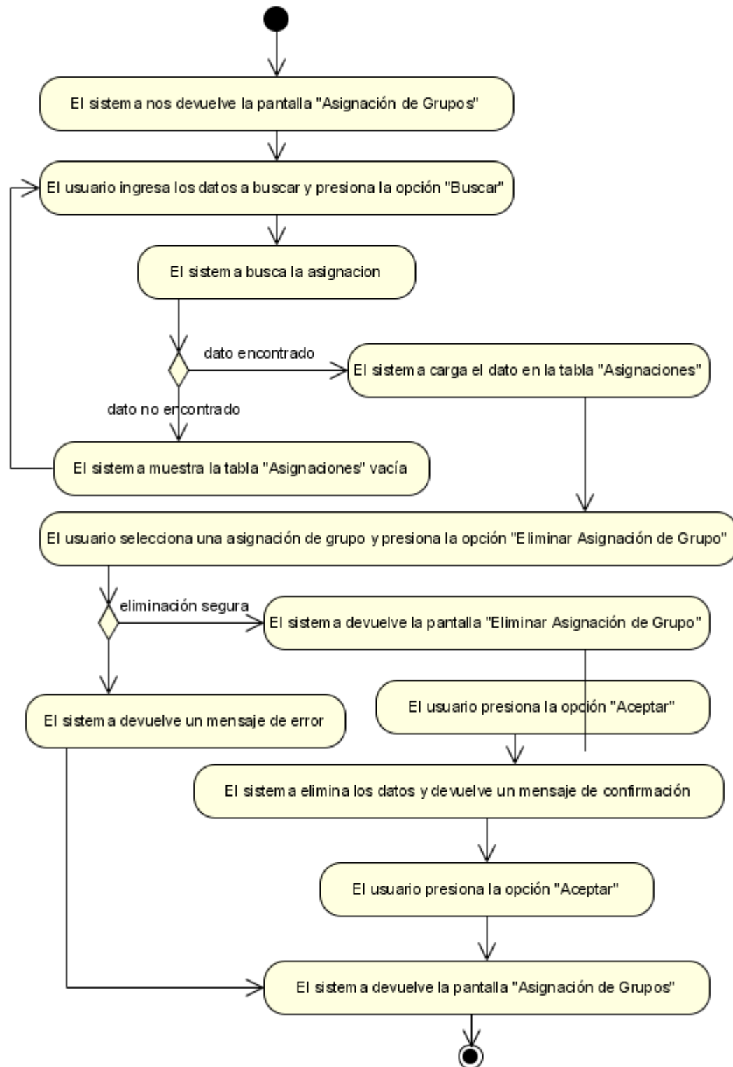
Figura N°41. Diagrama de Actividad Eliminar Asignación de Grupo.
