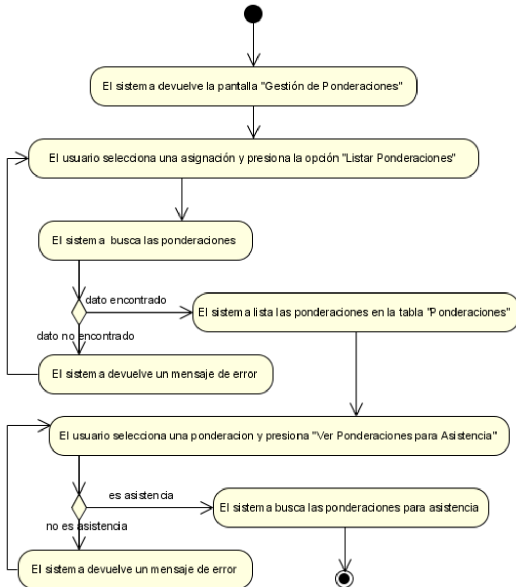
Figura N°53. Diagrama de Actividad Ver Ponderaciones para Asistencia.
