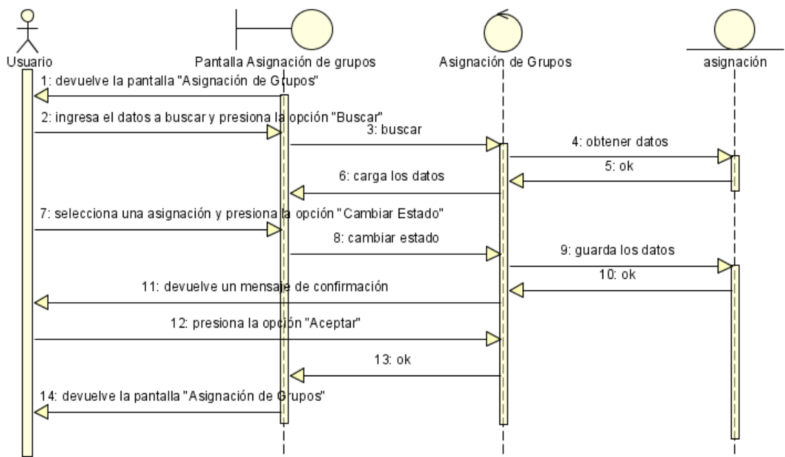
Figura N°102. Diagrama de Secuencia Cambiar Estado de Asignación.
