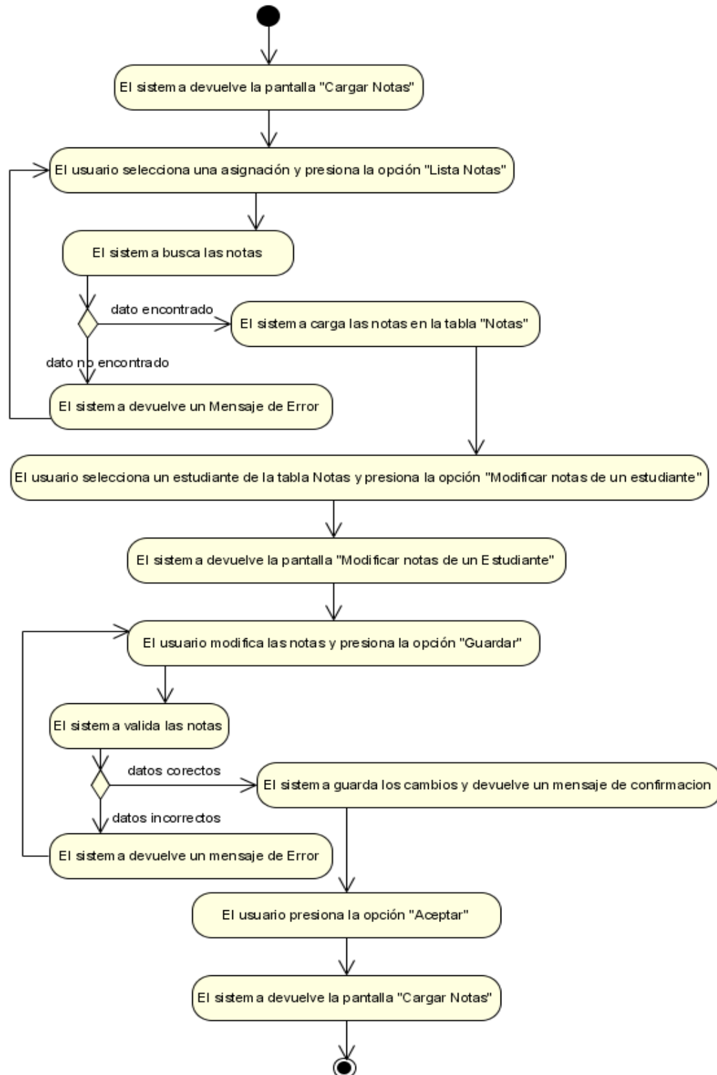
Figura N°72. Diagrama de Actividad Modificar Notas de un Estudiante.
