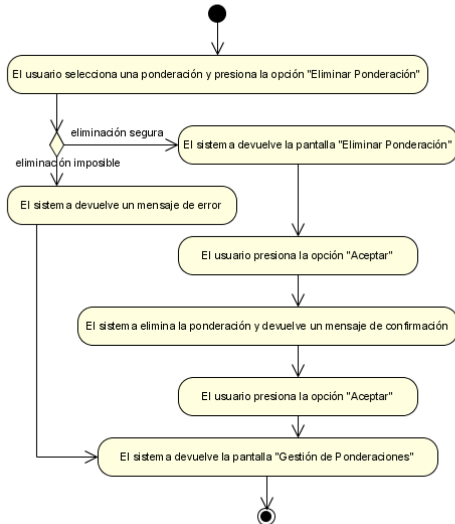
Figura N°52. Diagrama de Actividad Eliminar Ponderación.
