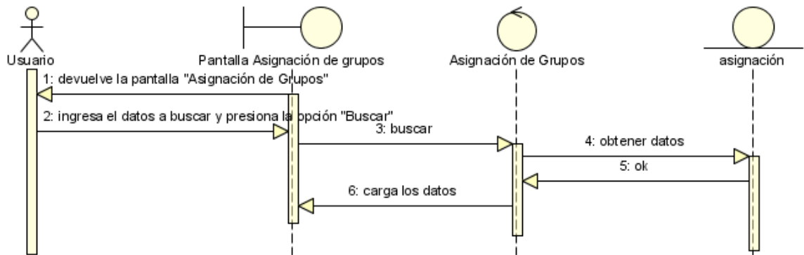
Figura N°98. Diagrama de Secuencia Listar Asignación de Grupo.
