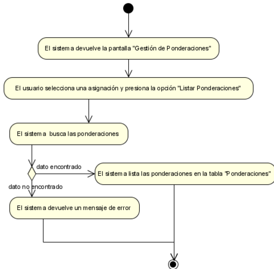
Figura N°48. Diagrama de Actividad Listar Ponderaciones.
