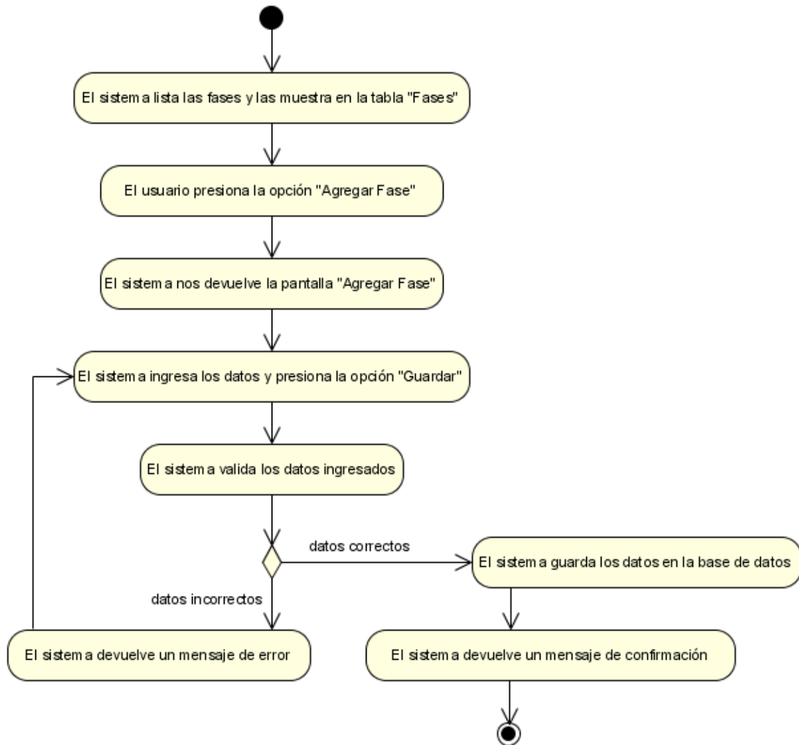
Figura N°19. Diagrama de Actividad Agregar Fase.
