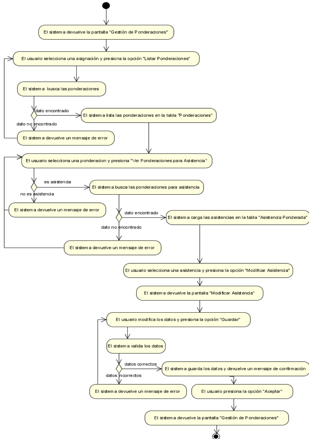
Figura N°56. Diagrama de Actividad Modificar Asistencia.
