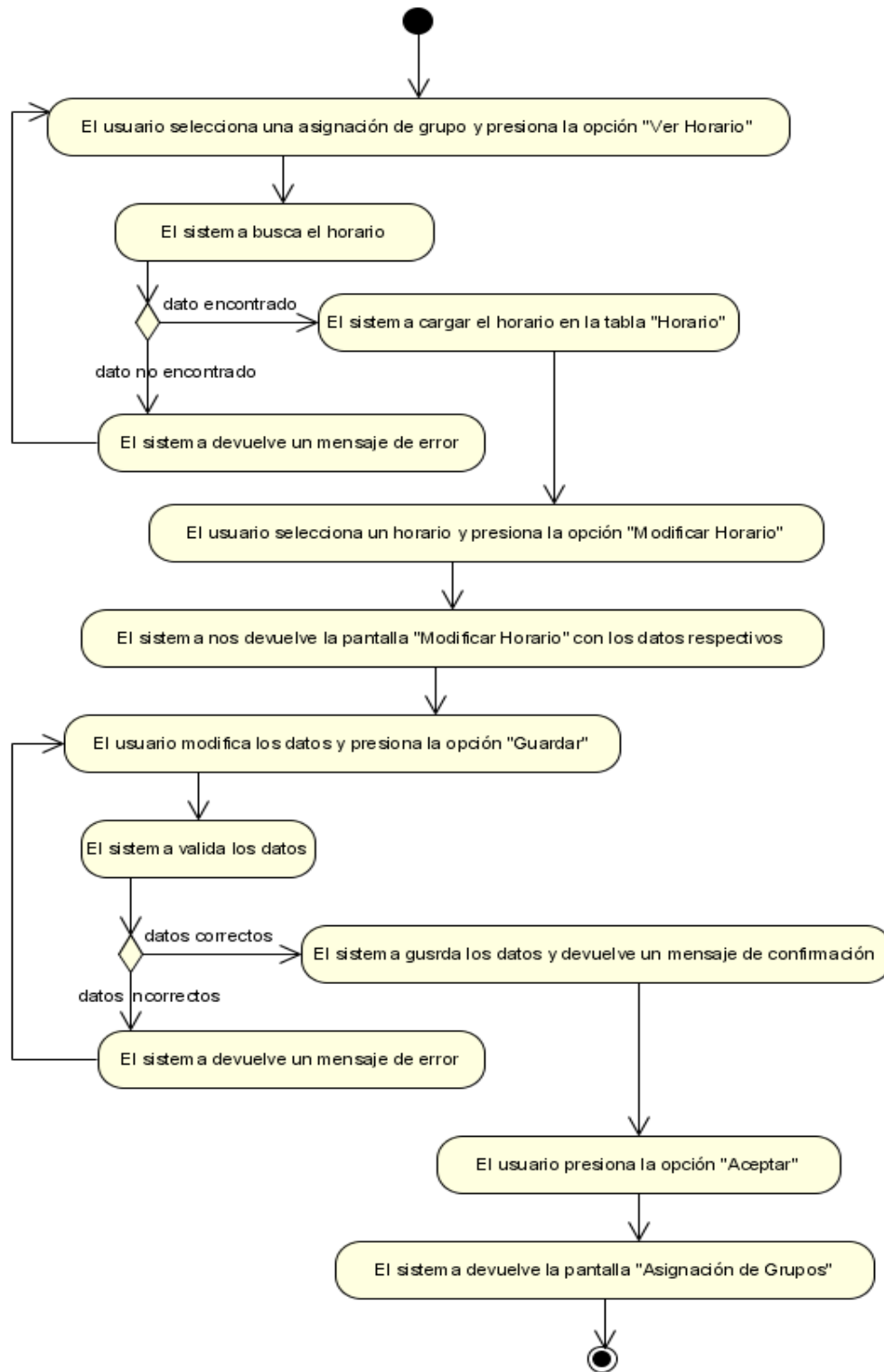
Figura N°46. Diagrama de Actividad Modificar Horario.
