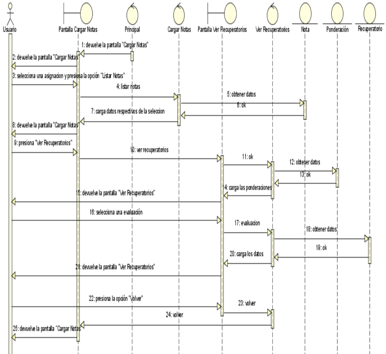
Figura N°131. Diagrama de Secuencia Ver Recuperatorios.
