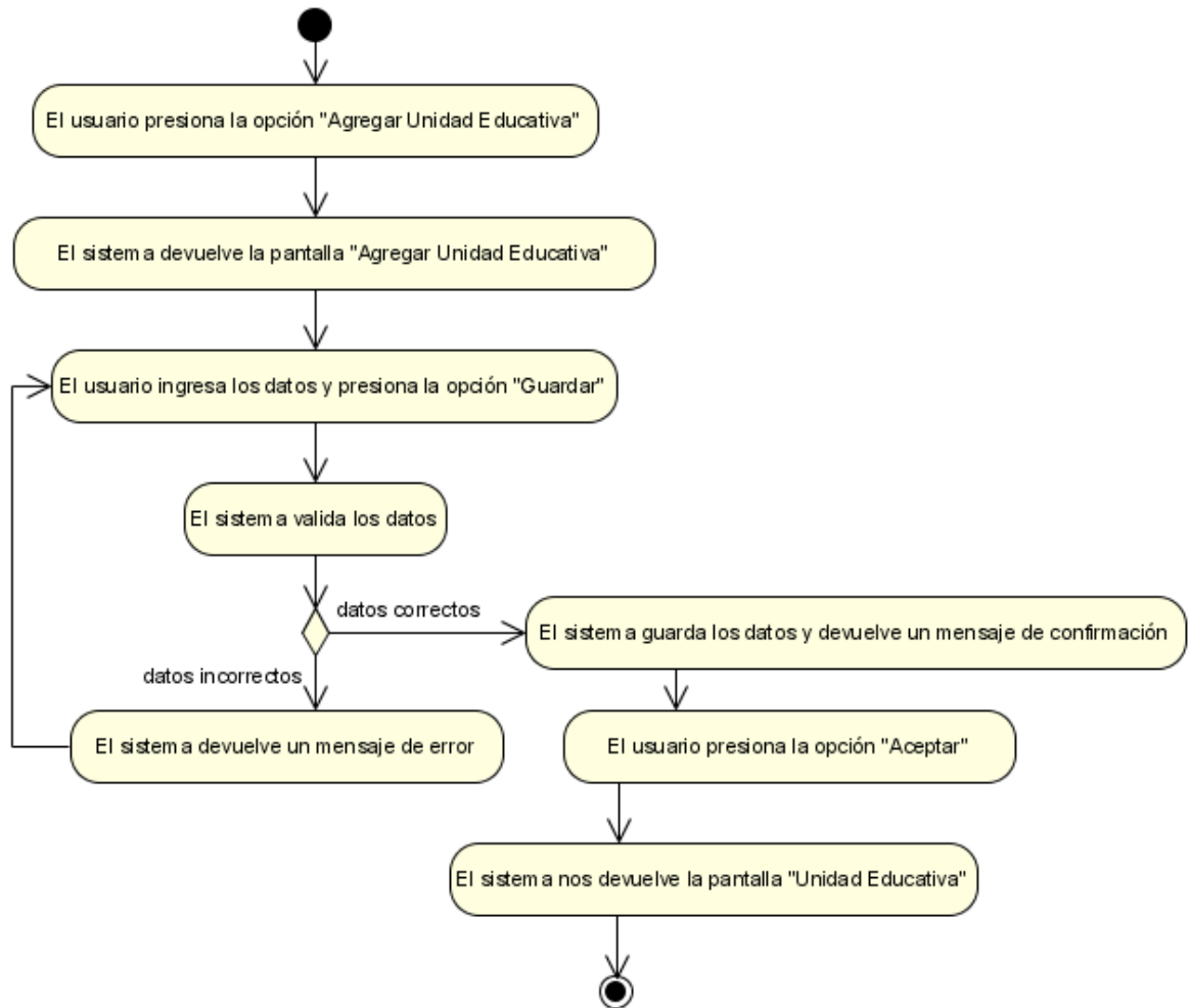
Figura N°24. Diagrama de Actividad Agregar Unidad Educativa.
