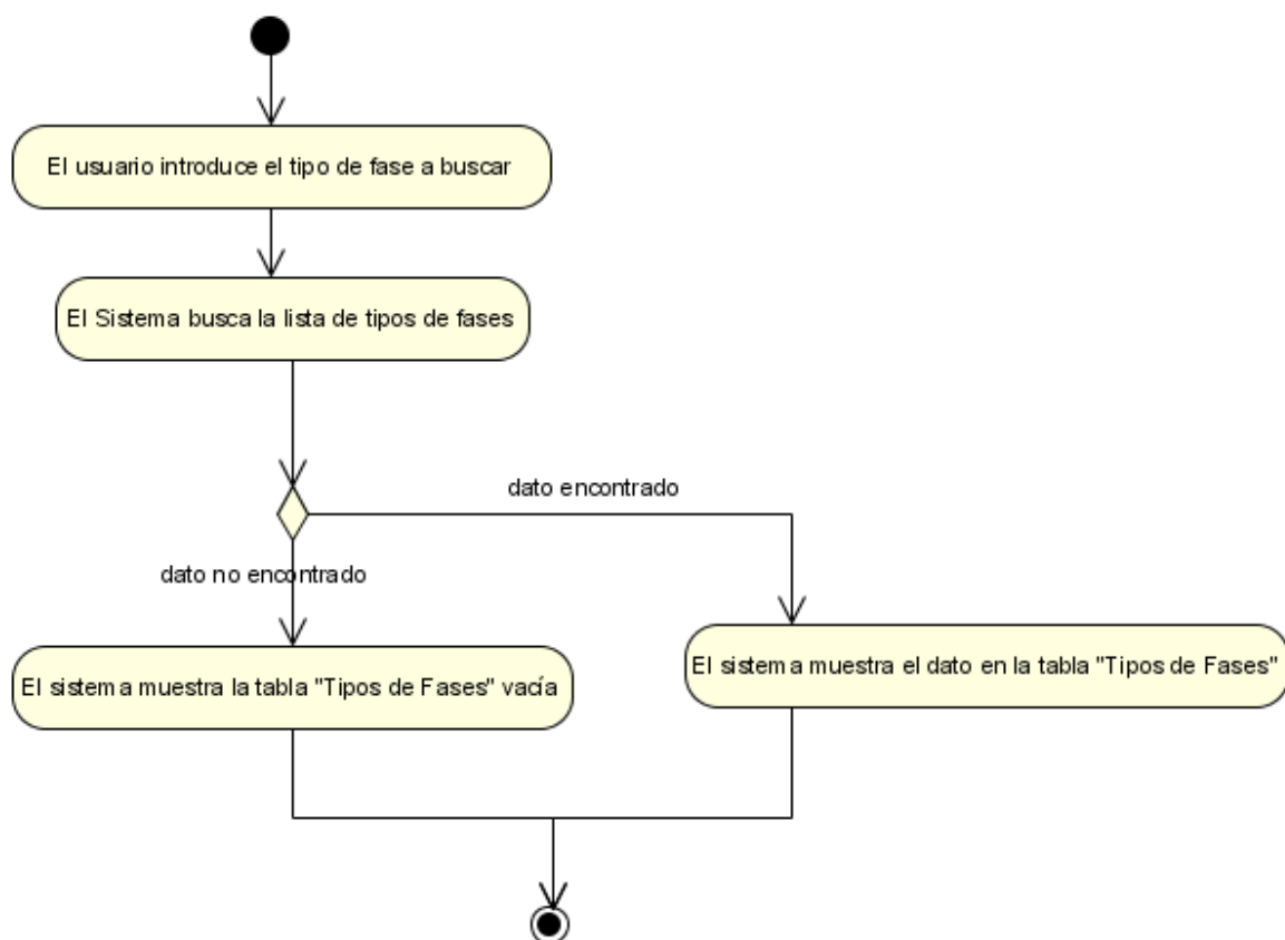
Figura N°13. Diagrama de Actividad Listar Modelos Educativos.
