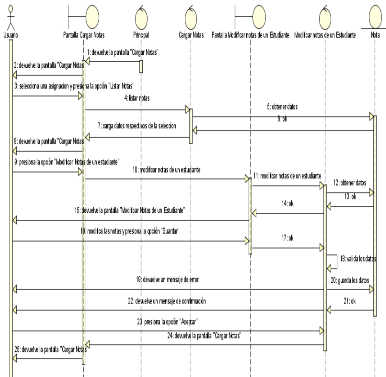
Figura N°132. Diagrama de Secuencia Modificar Notas de un Estudiante.
