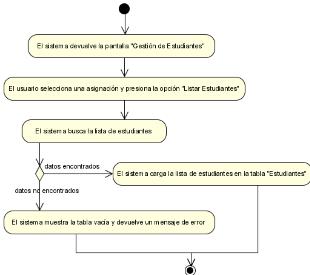
Figura N°58. Diagrama de Actividad Listar Estudiantes.
