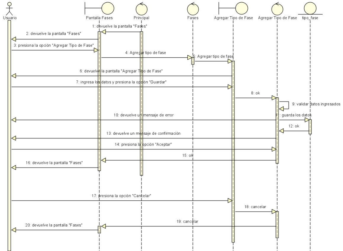
Figura N°75. Diagrama de Secuencia Agregar Modelo Educativo.
