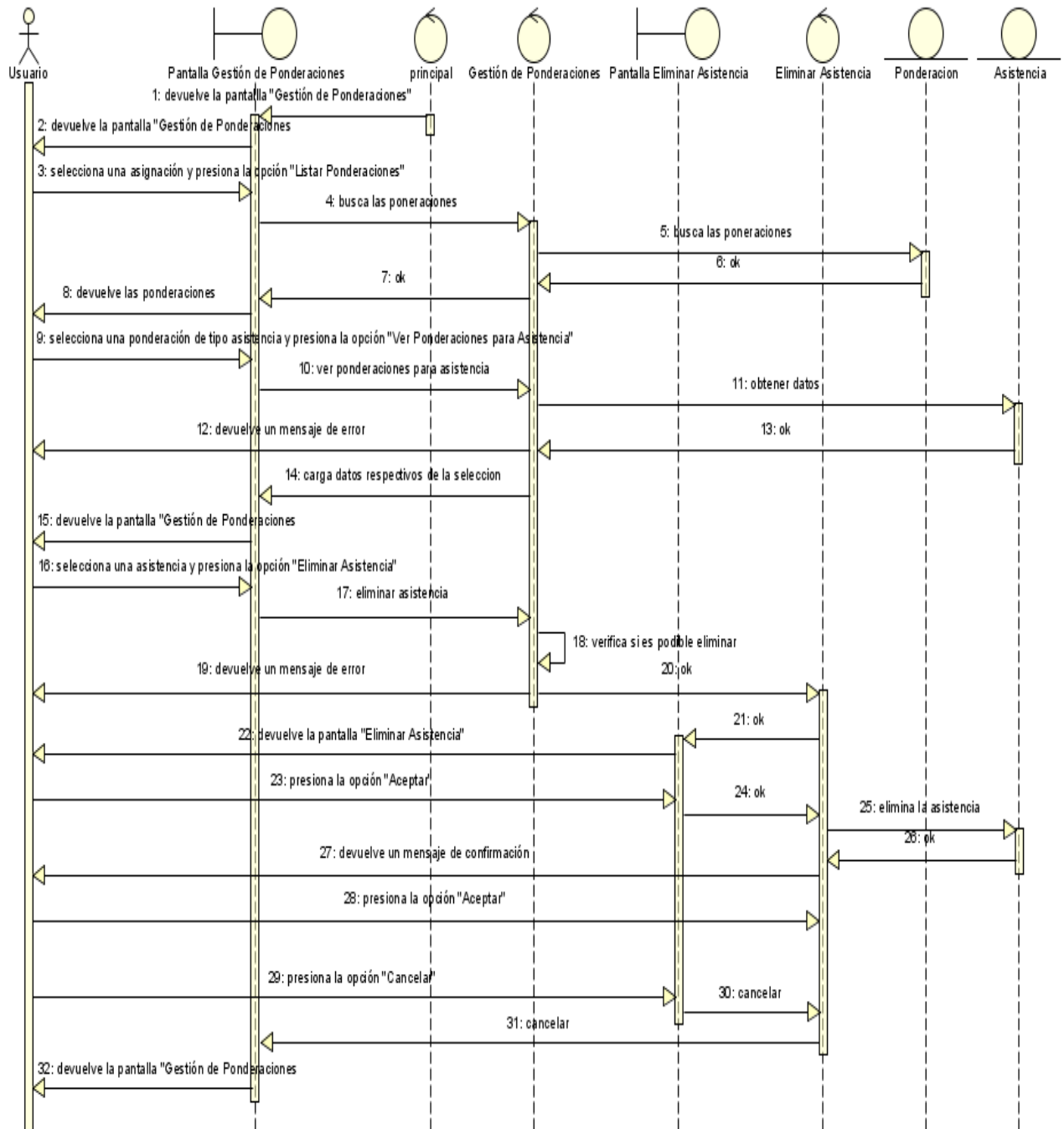
Figura N°117. Diagrama de Secuencia Eliminar Asistencia.
