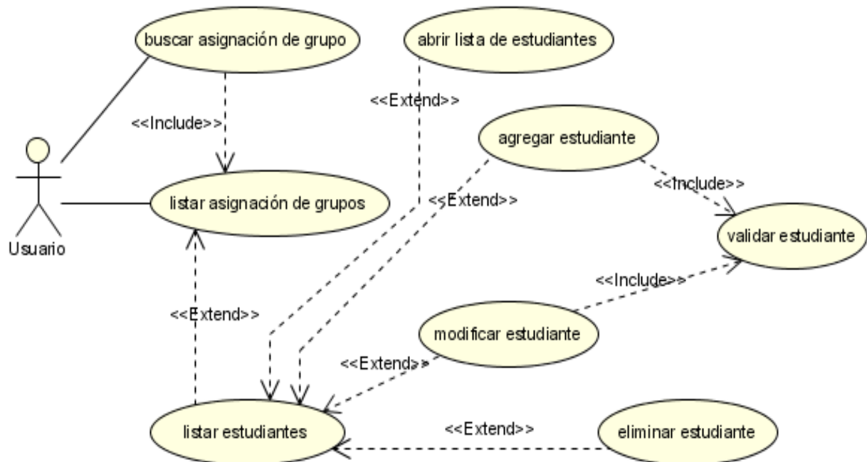
Figura N°10. Diagrama de Caso de Uso Gestionar Estudiantes.
