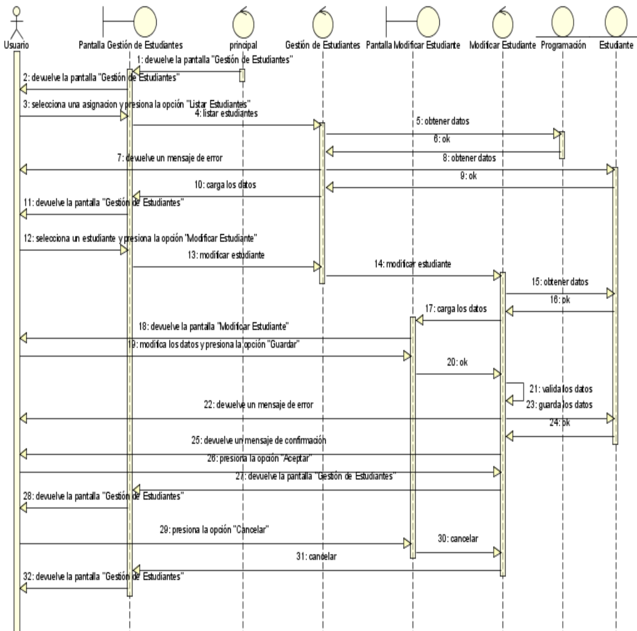
Figura N°121. Diagrama de Secuencia Modificar Estudiante.
