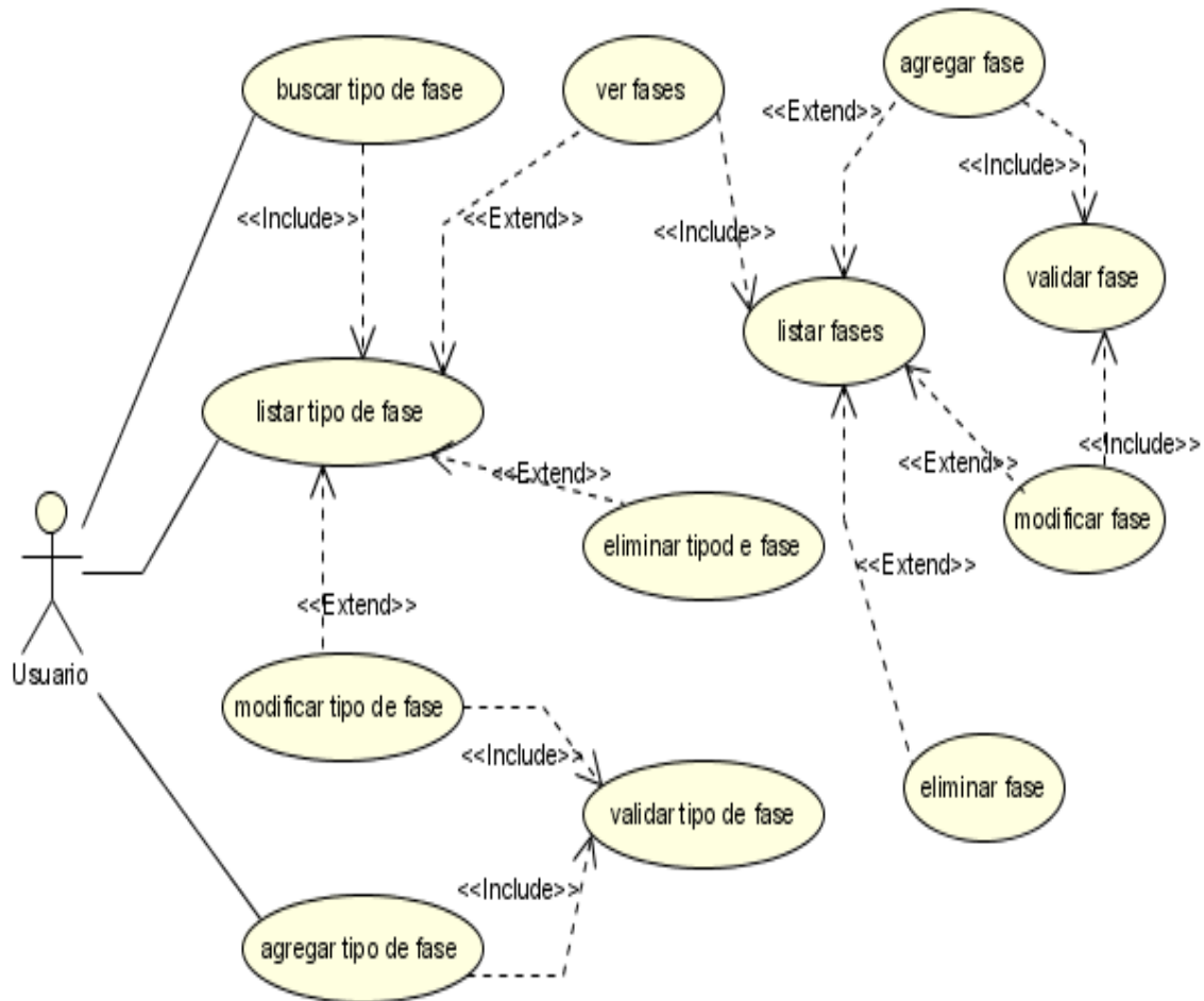
Figura N°5. Diagrama de Caso de Uso Gestionar Fases.
