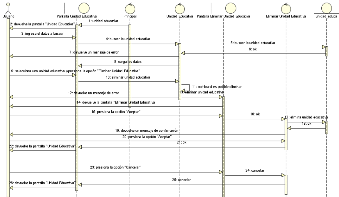
Figura N°87. Diagrama de Secuencia Eliminar Unidad Educativa.
