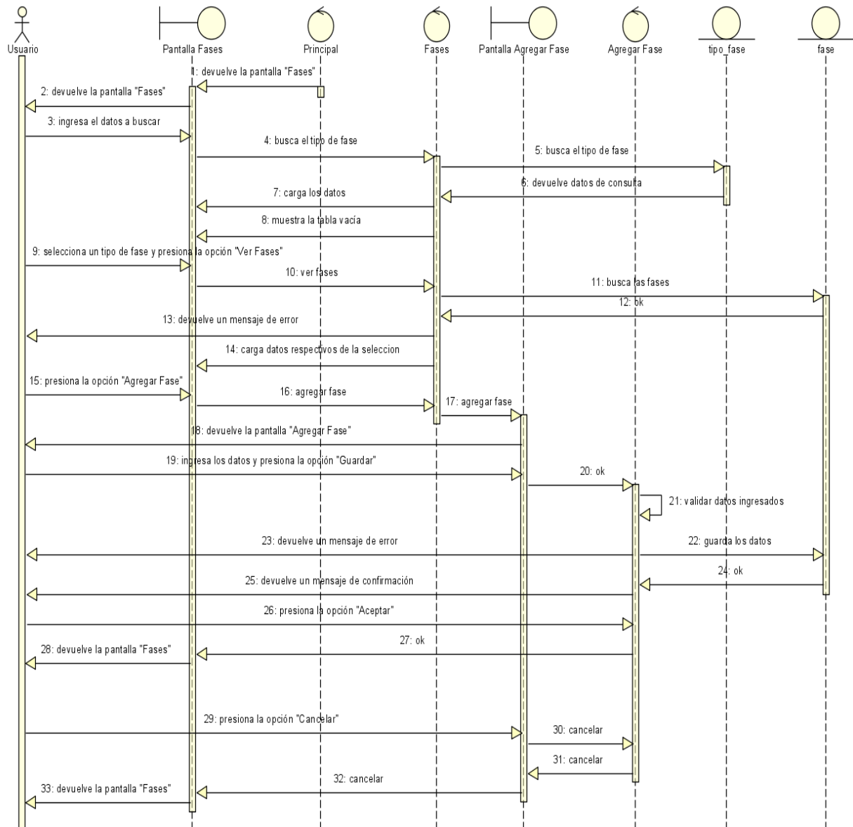
Figura N°80. Diagrama de Secuencia Agregar Fase.
