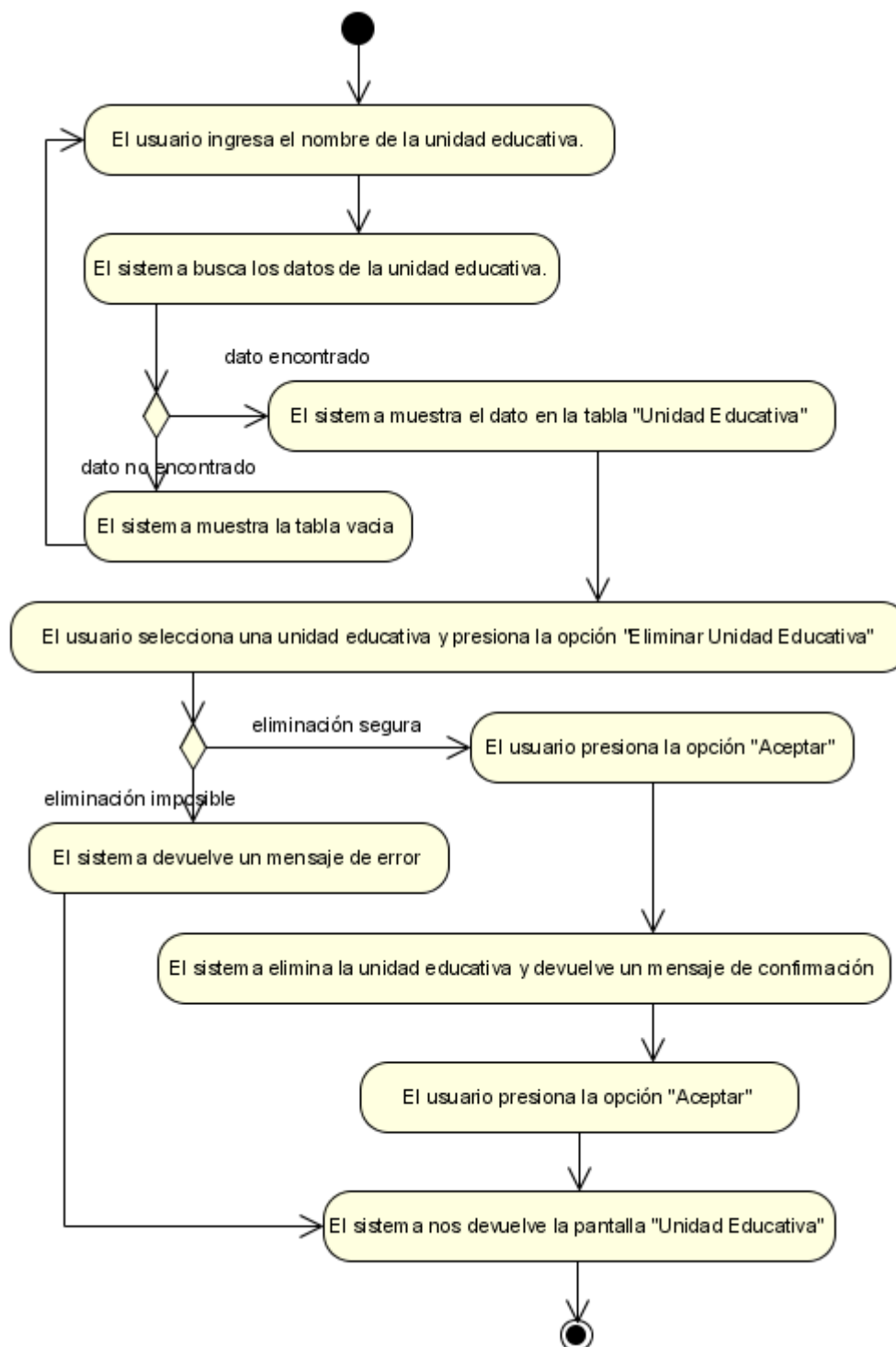
Figura N°26. Diagrama de Actividad Eliminar Unidad Educativa.
