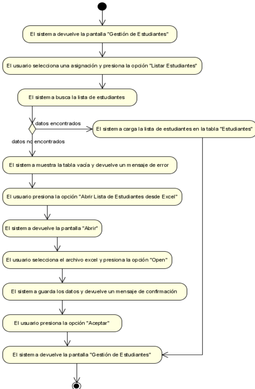
Figura N°59. Diagrama de Actividad Abrir Lista de Estudiantes.
