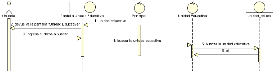
Figura N°83. Diagrama de Secuencia Buscar Unidad Educativa.
