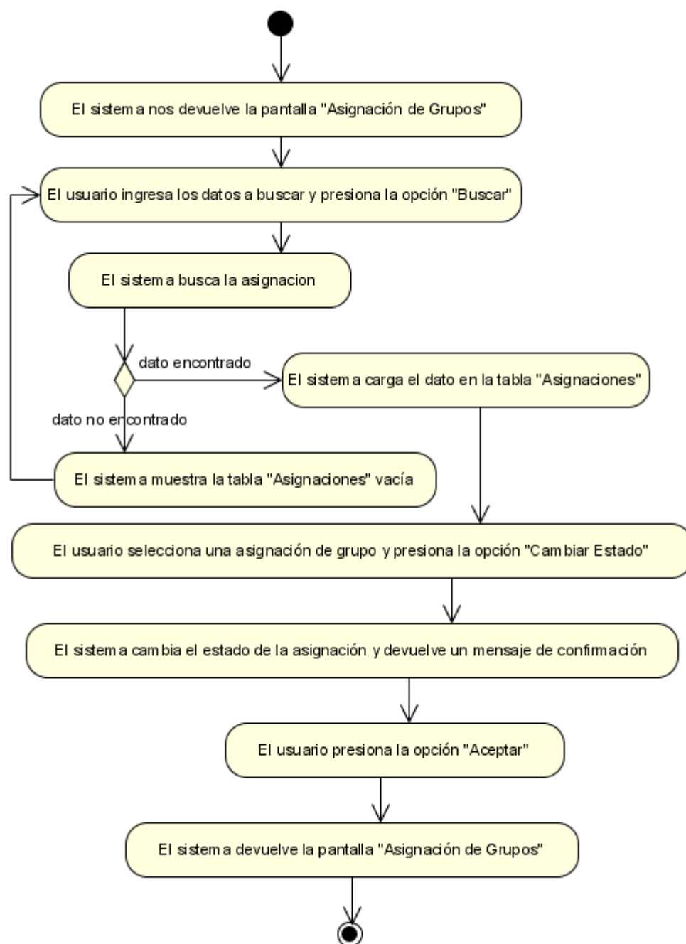
Figura N°42. Diagrama de Actividad Cambiar Estado de Asignación.
