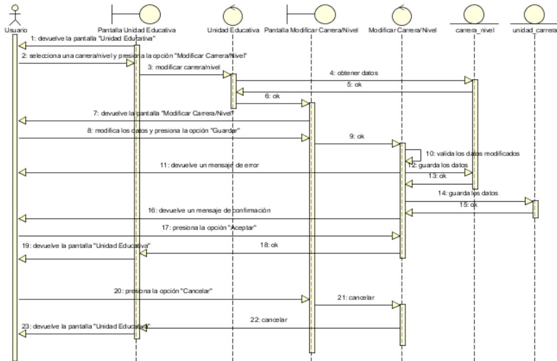
Figura N°90. Diagrama de Secuencia Modificar Carrera/Nivel.
