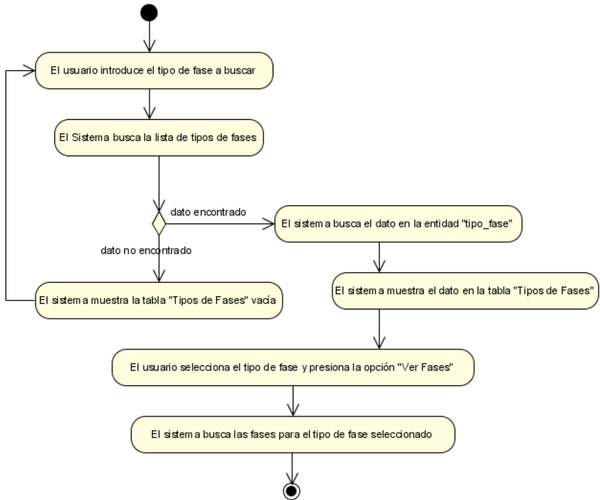
Figura N°17. Diagrama de Actividad Ver Fases.
