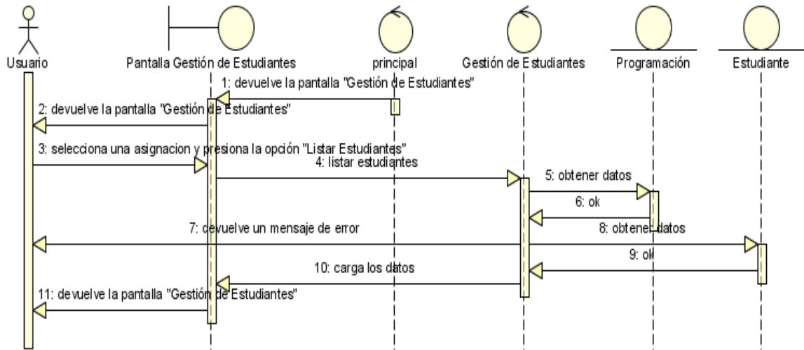
Figura N°118. Diagrama de Secuencia Listar Estudiantes.
