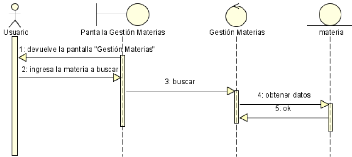
Figura N°92. Diagrama de Secuencia Buscar Materia.
