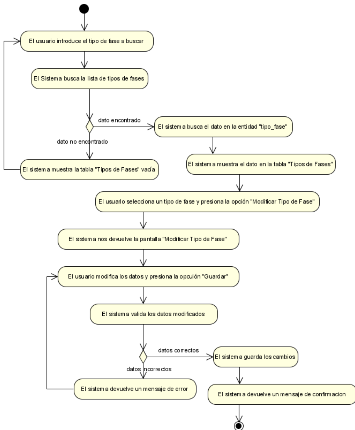
Figura N°15. Diagrama de Actividad Modificar Modelo educativo.
