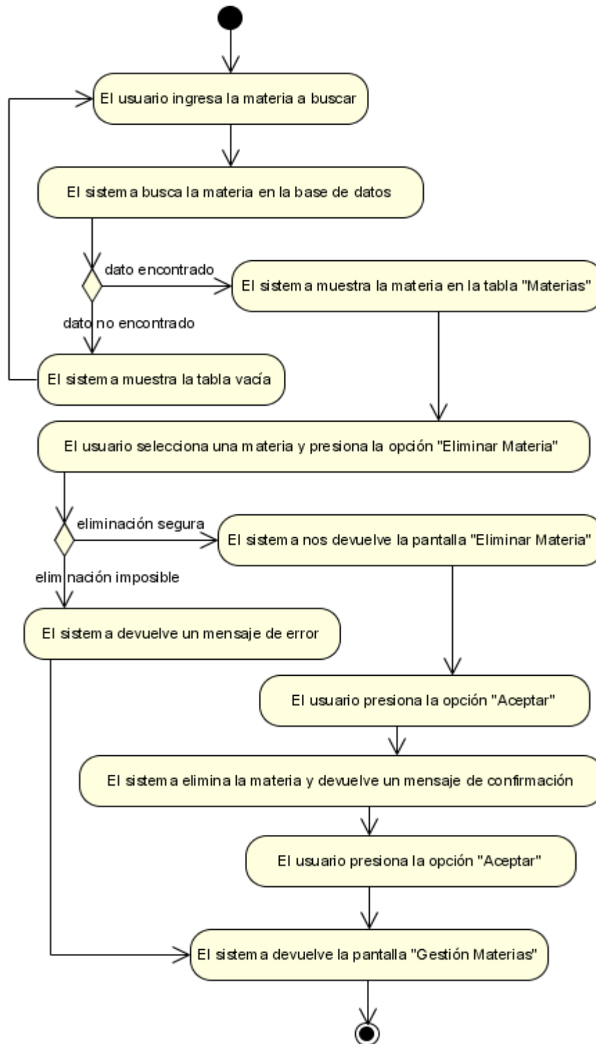
Figura N°36. Diagrama de Actividad Eliminar Materia.
