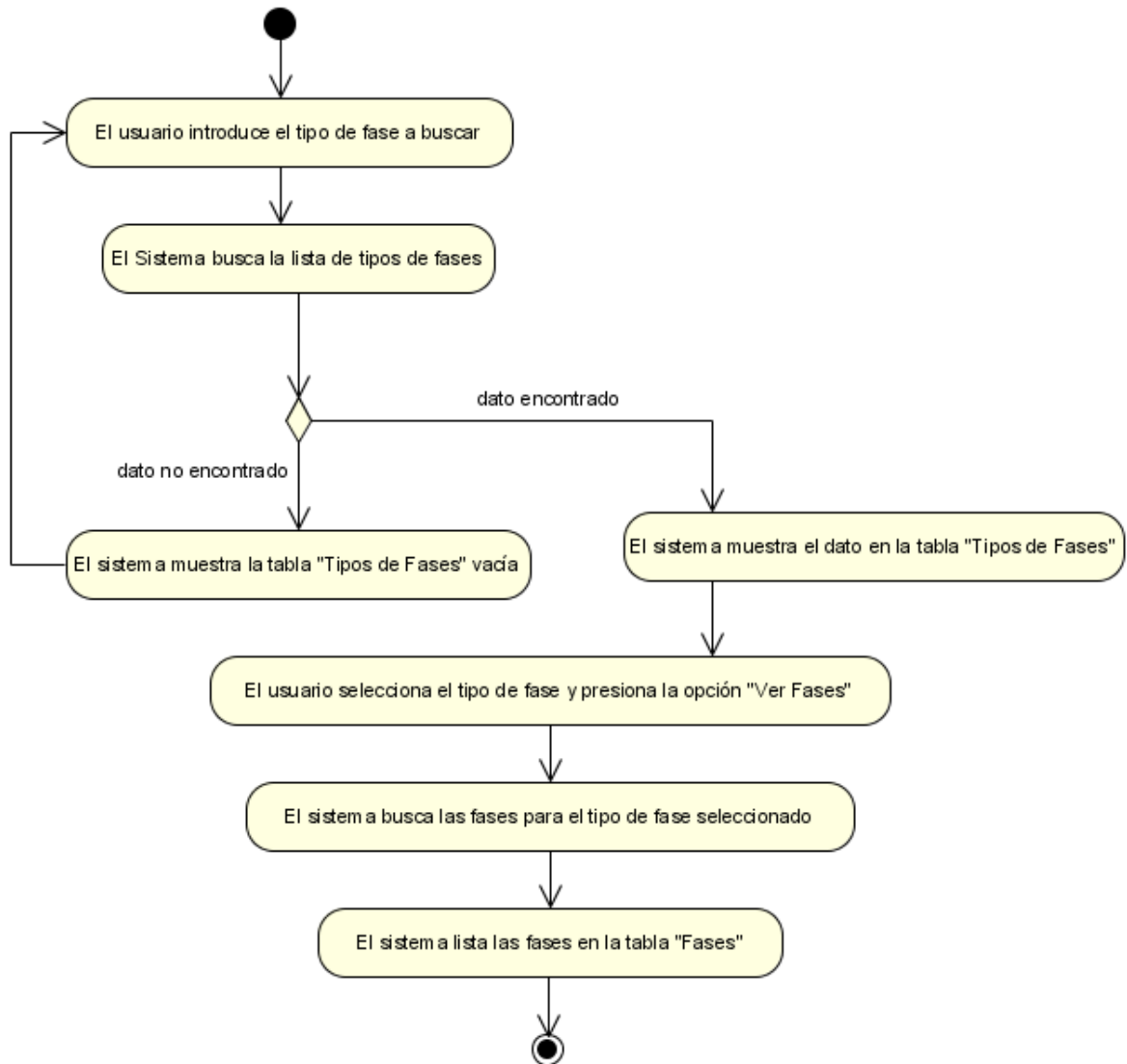
Figura N°18. Diagrama de Actividad Listar Fases.
