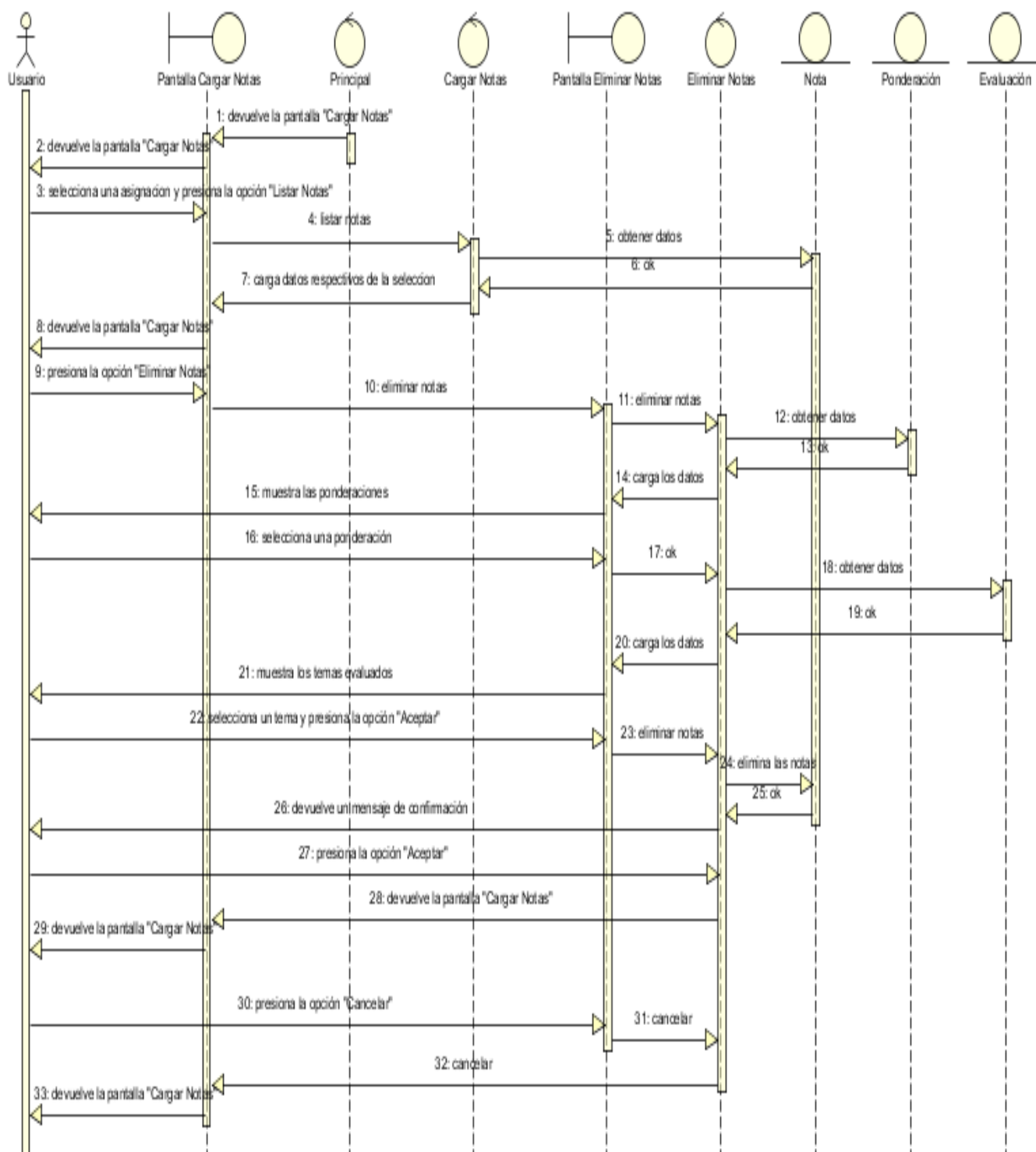
Figura N°126. Diagrama de Secuencia Eliminar Notas.
