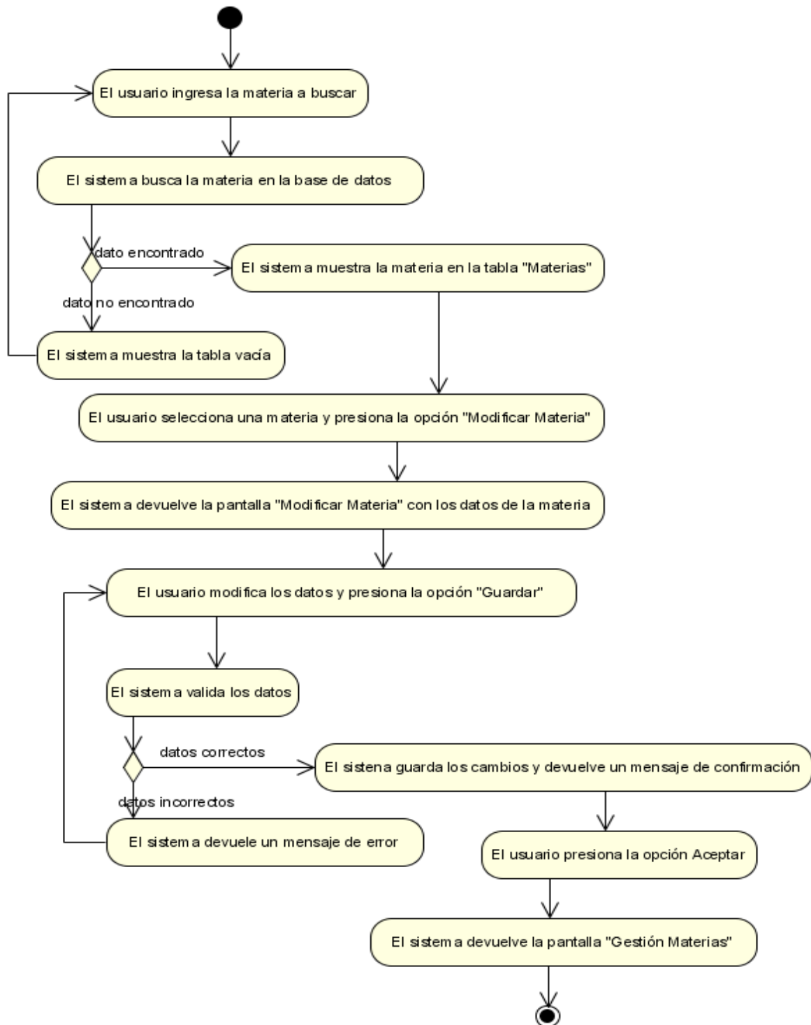
Figura N°35. Diagrama de Actividad Modificar Materia.
