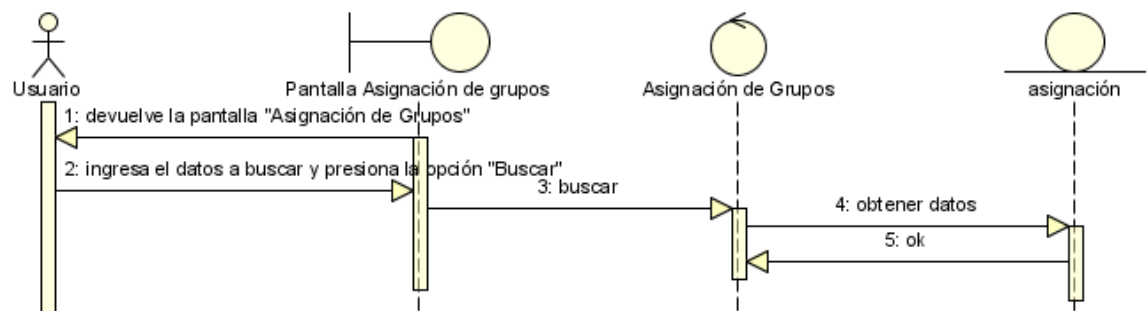
Figura N°97. Diagrama de Secuencia Buscar Asignación de Grupo.
