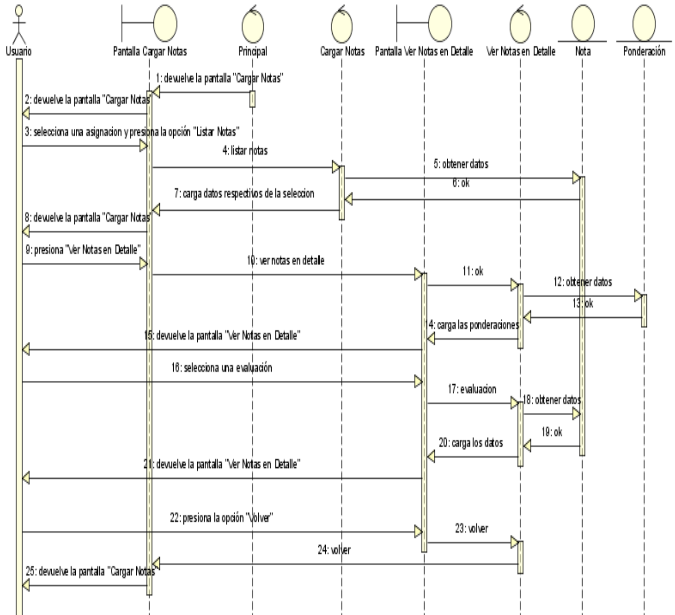
Figura N°130. Diagrama de Secuencia Ver Notas en Detalle.
