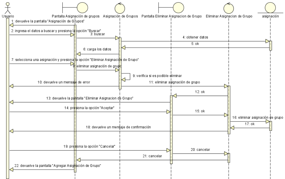
Figura N°101. Diagrama de Secuencia Eliminar Asignación de Grupo.
