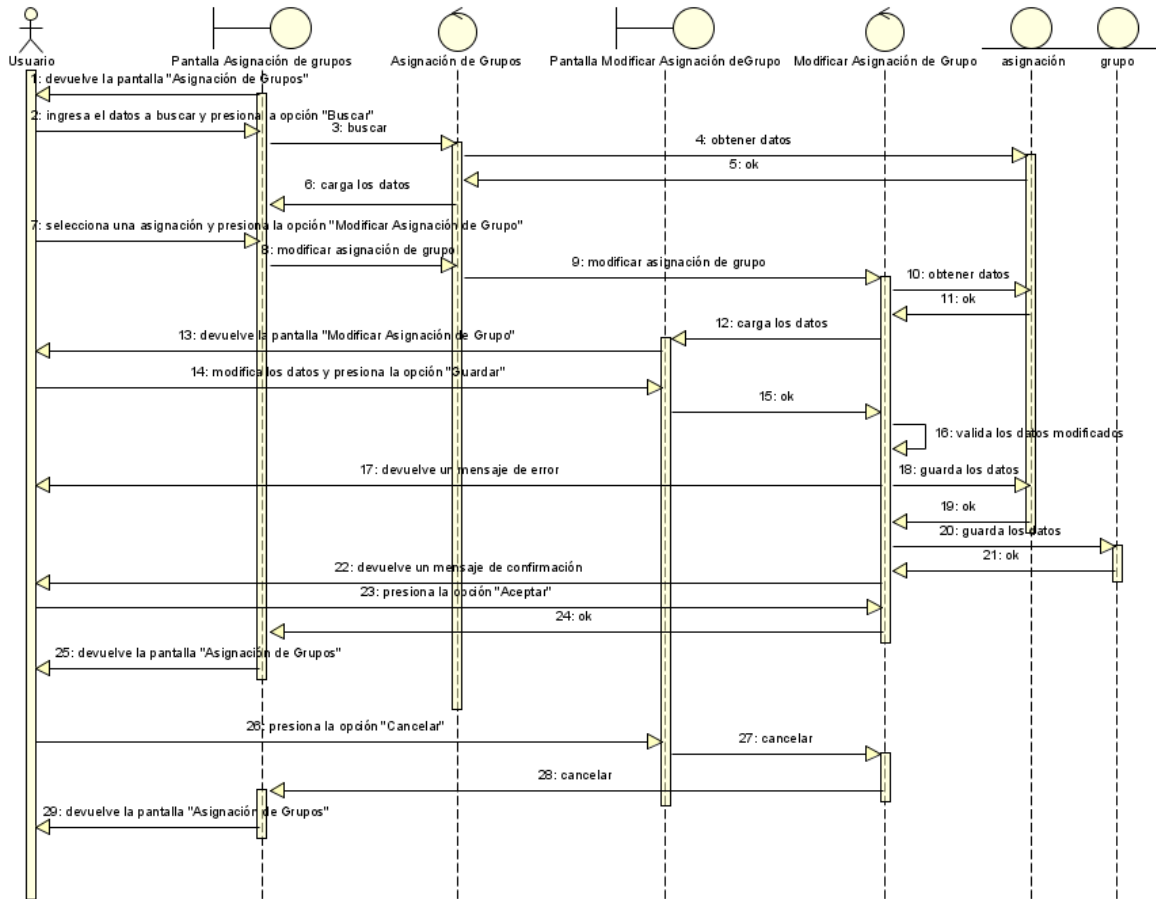
Figura N°100. Diagrama de Secuencia Modificar Asignación de Grupo.
