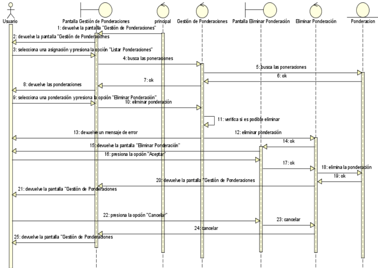
Figura N°112. Diagrama de Secuencia Eliminar Ponderación.
