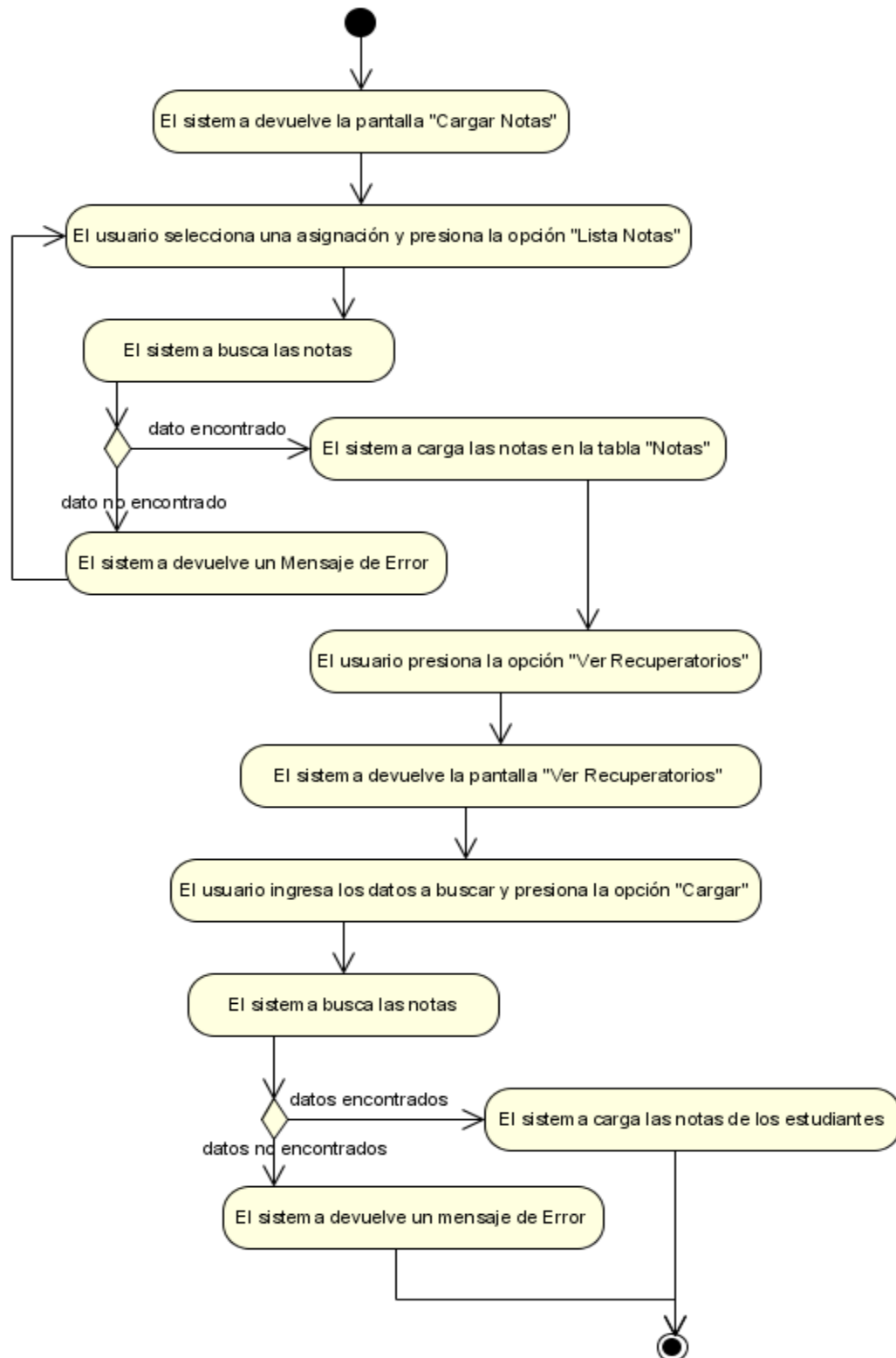
Figura N°71. Diagrama de Actividad Ver Recuperatorios.
