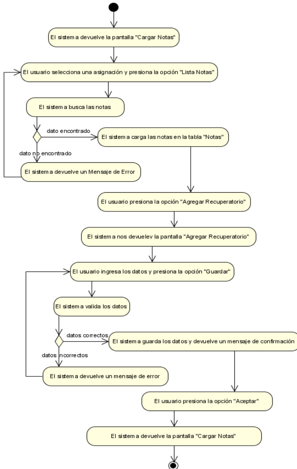
Figura N°67. Diagrama de Actividad Agregar Recuperatorio.
