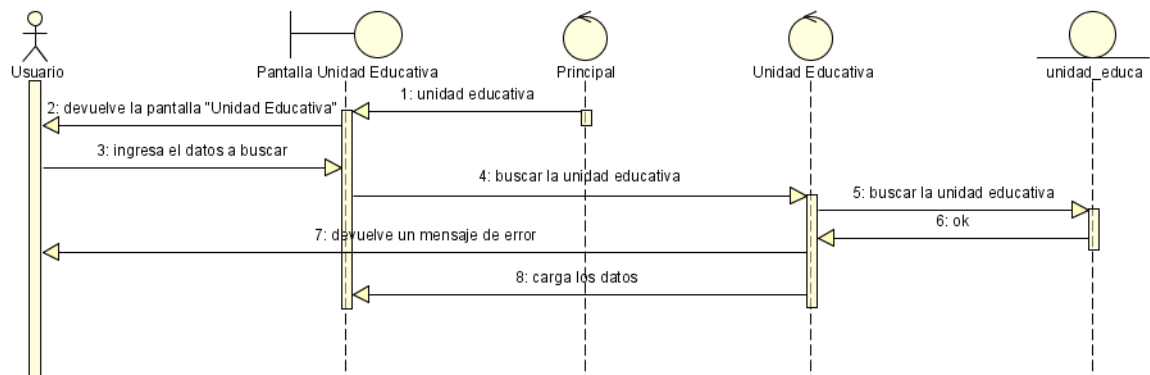
Figura N°84. Diagrama de Secuencia Listar Unidades Educativas.
