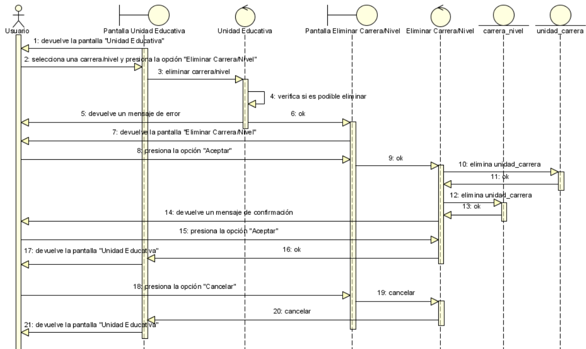
Figura N°91. Diagrama de Secuencia Eliminar Carrera/Nivel.
