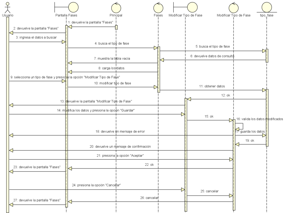
Figura N°76. Diagrama de Secuencia Modificar Modelo Educativo.
