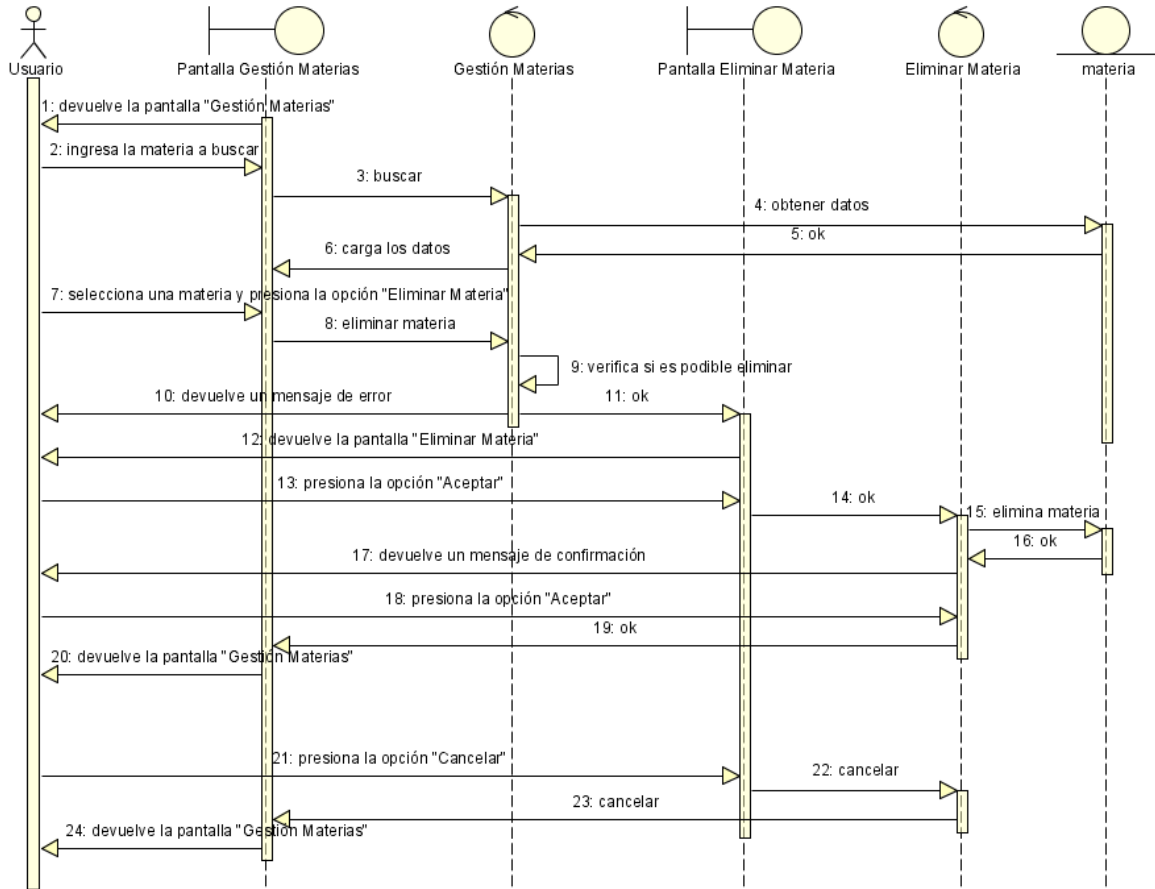
Figura N°96. Diagrama de Secuencia Eliminar Materia.
