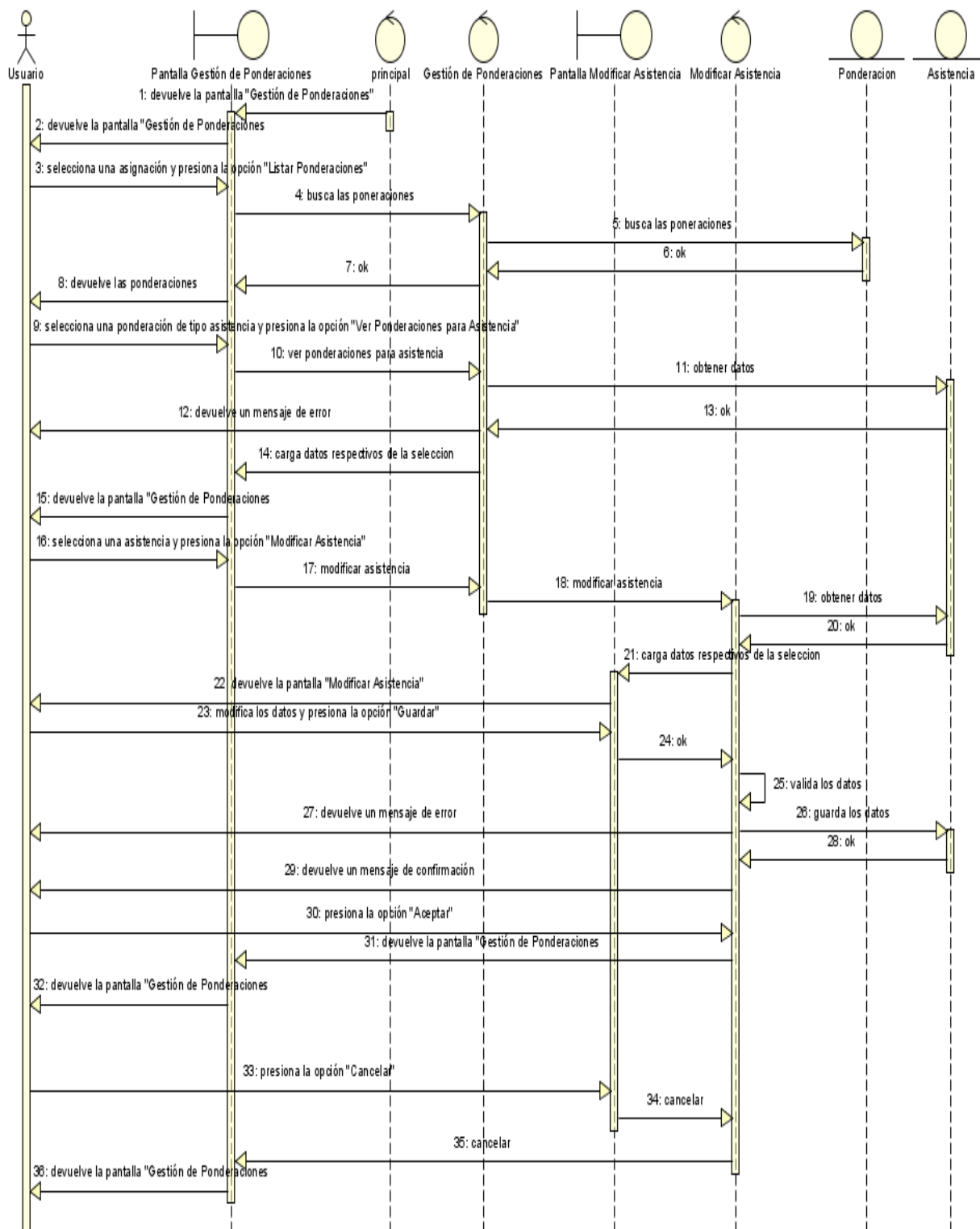
Figura N°116. Diagrama de Secuencia Modificar Asistencia.
