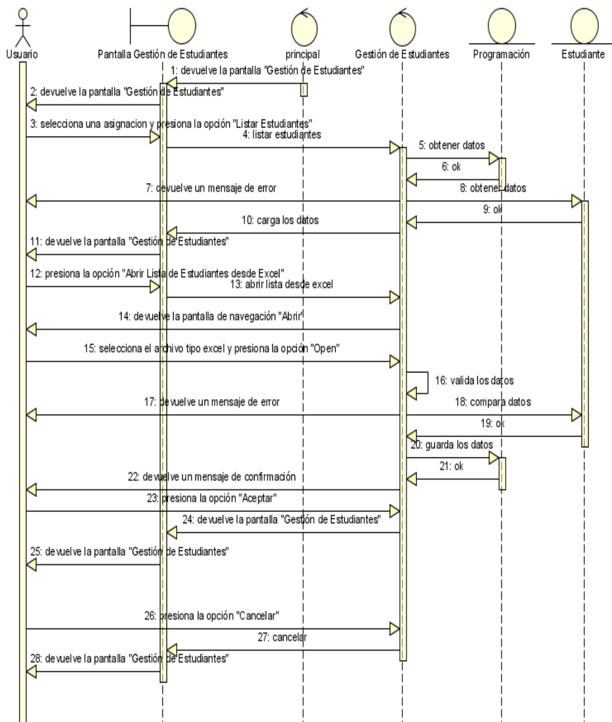
Figura N°119. Diagrama de Secuencia Abrir Lista de Estudiantes.
