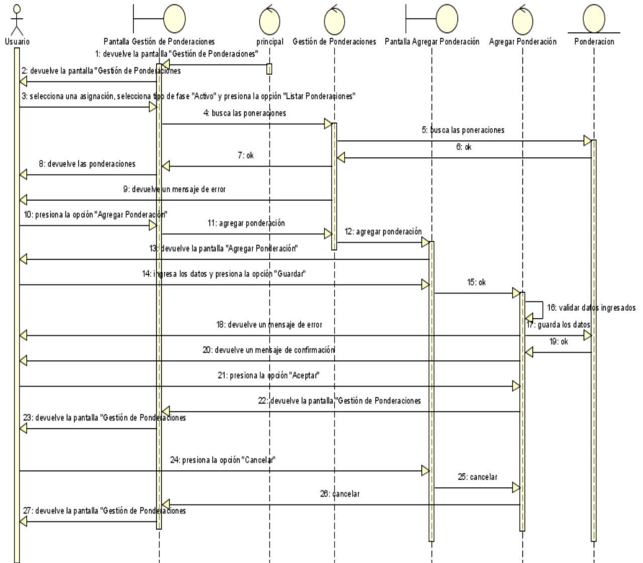
Figura N°109. Diagrama de Secuencia Agregar Ponderación.
