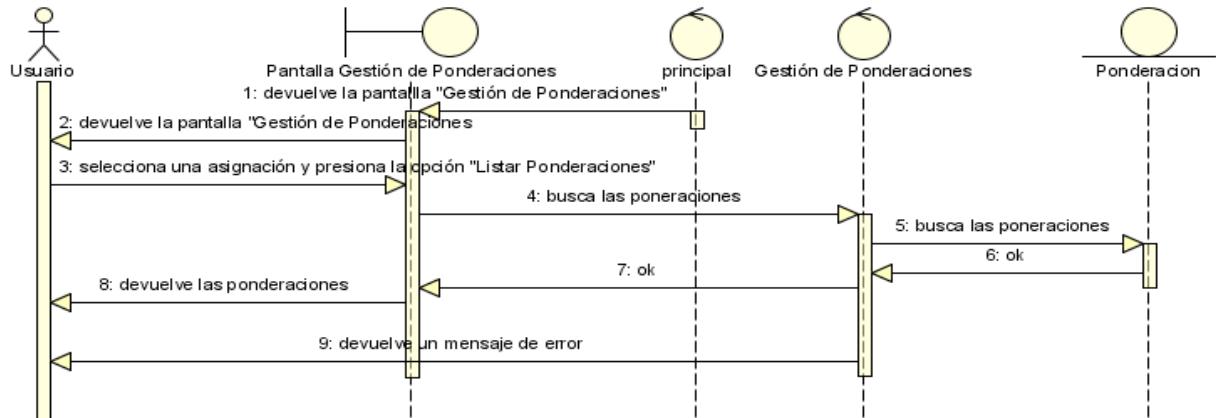
Figura N°110. Diagrama de Secuencia Listar Ponderaciones.
