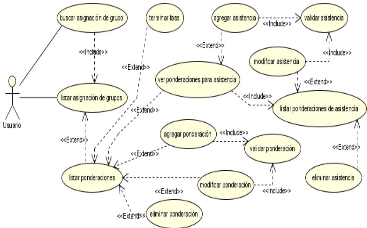
Figura N°9. Diagrama de Caso de Uso Gestionar Ponderaciones.
