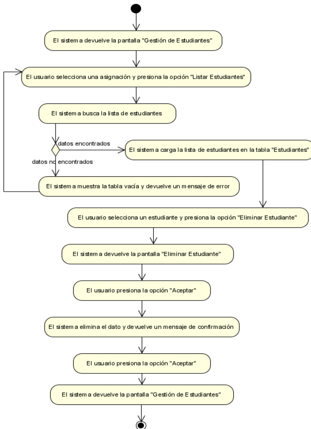
Figura N°62. Diagrama de Actividad Eliminar Estudiante.
