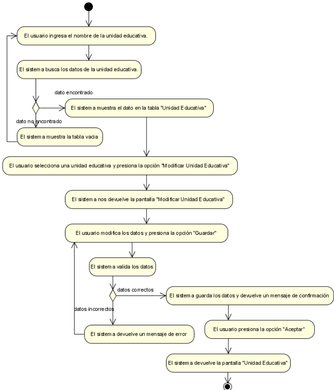
Figura N°25. Diagrama de Actividad Modificar Unidad Educativa.
