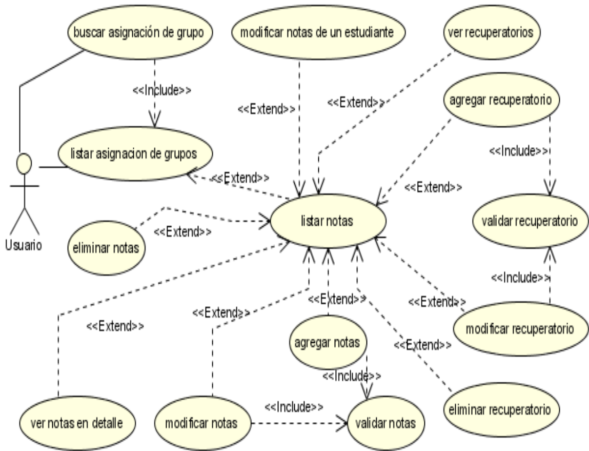
Figura N°11. Diagrama de Caso de Uso Gestionar Cargado de Notas.
