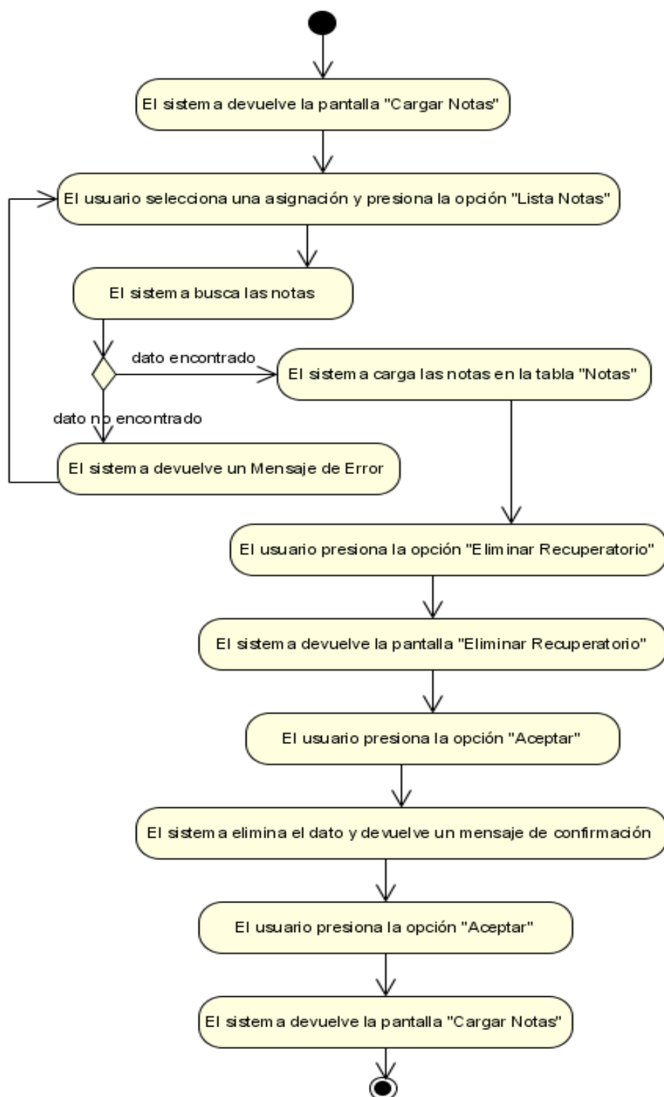
Figura N°69. Diagrama de Actividad Eliminar Recuperatorio.
