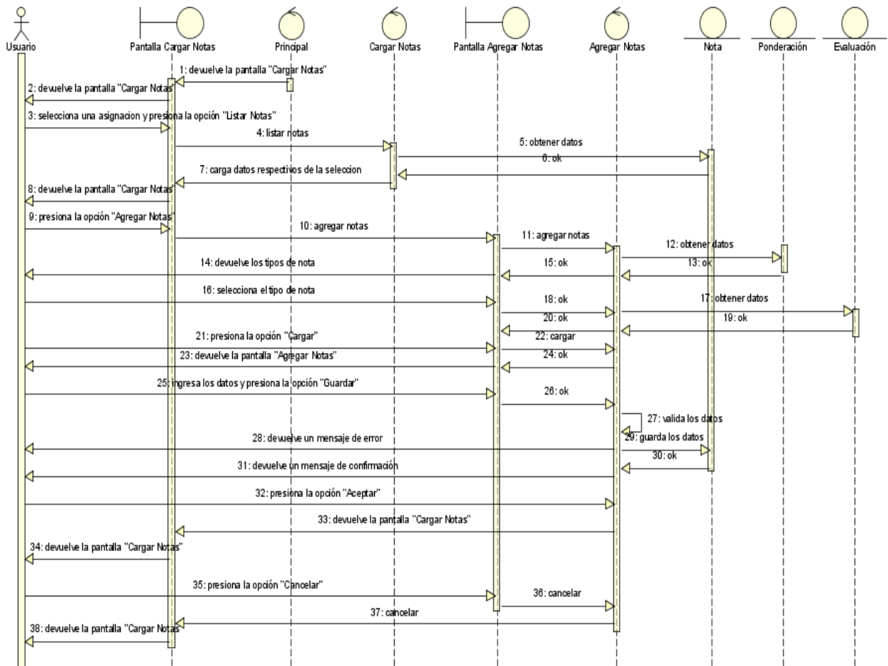
Figura N°124. Diagrama de Secuencia Agregar Notas.
