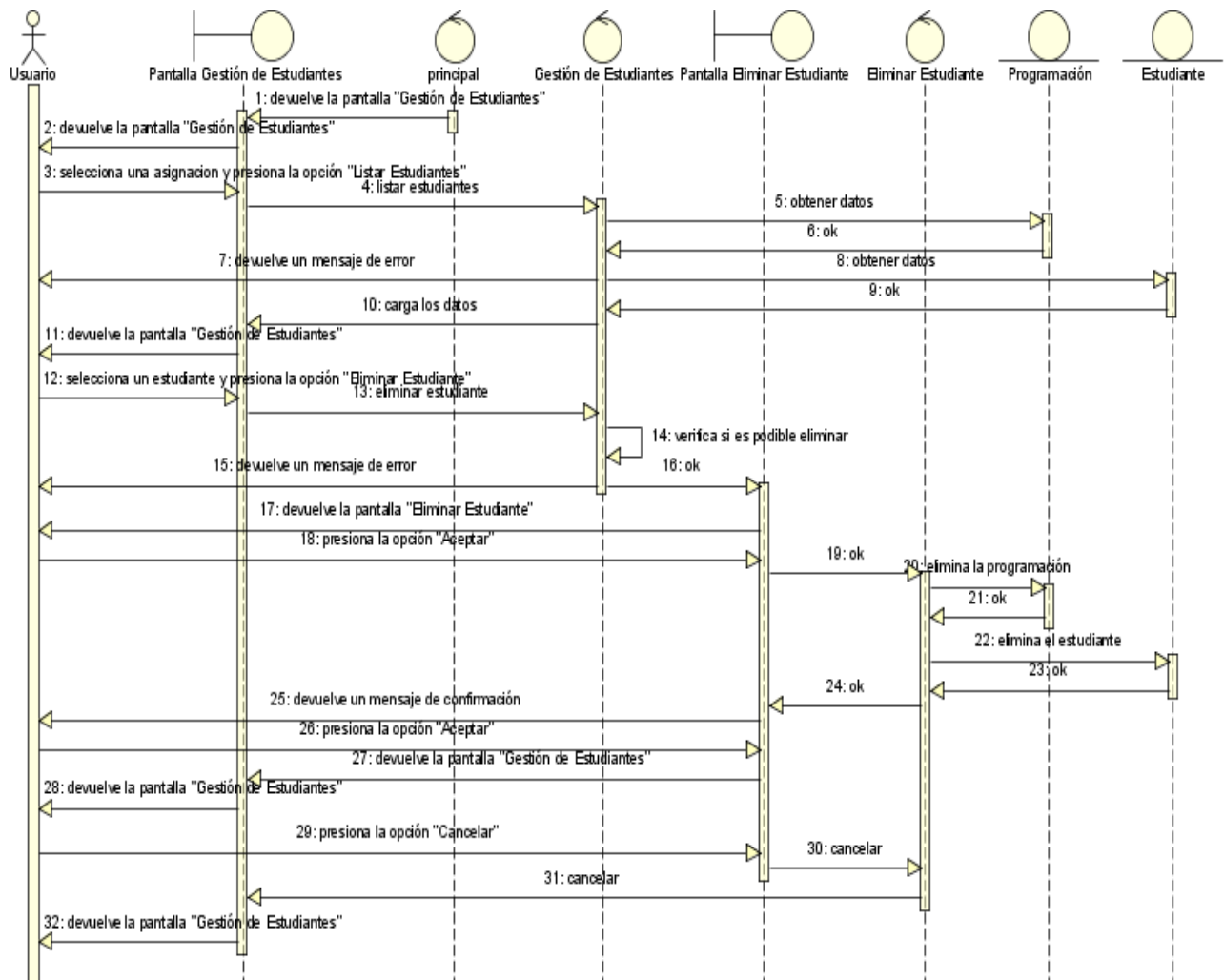
Figura N°122. Diagrama de Secuencia Eliminar Estudiante.
