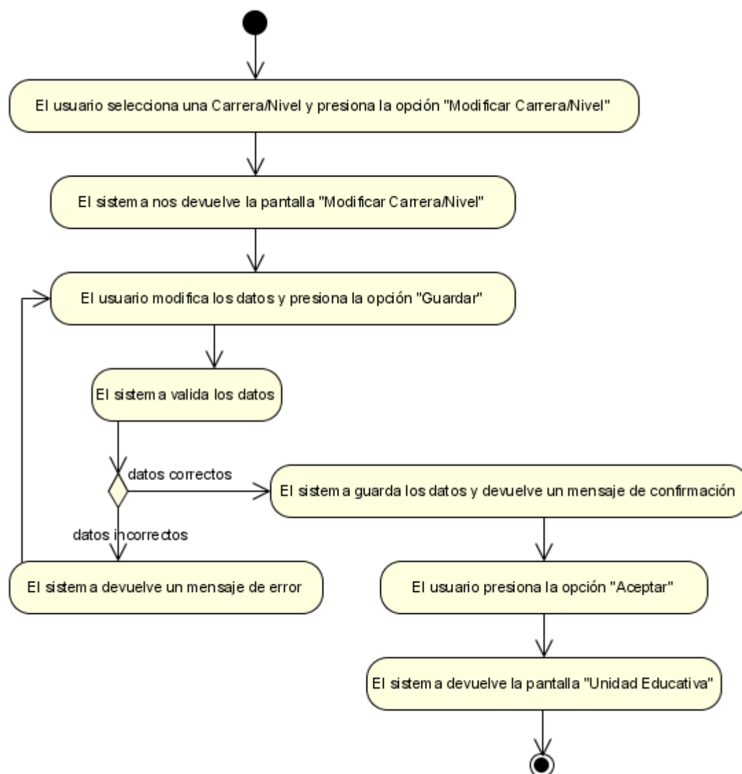
Figura N°30. Diagrama de Actividad Modificar Carrera/Nivel.
