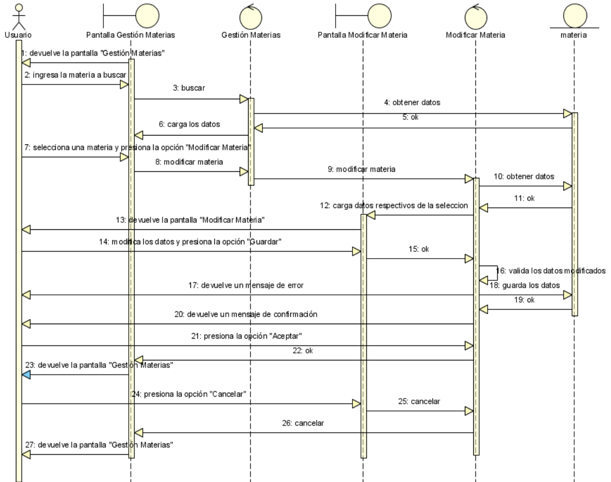
Figura N°95. Diagrama de Secuencia Modificar Materia.
