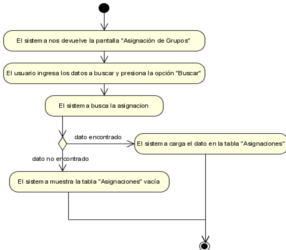
Figura N°38. Diagrama de Actividad Listar Asignación de Grupos.
