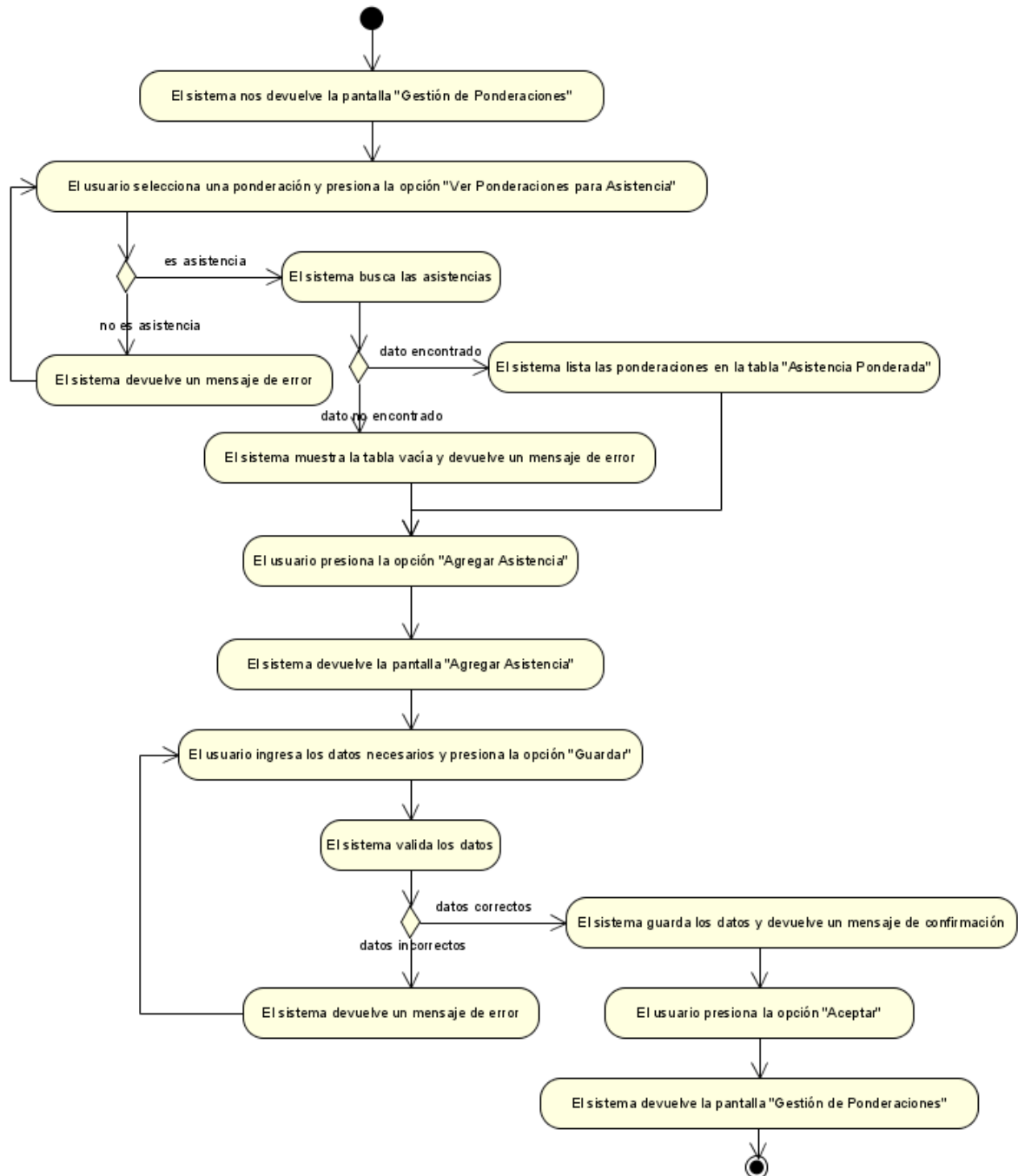
Figura N°54. Diagrama de Actividad Agregar Asistencia.
