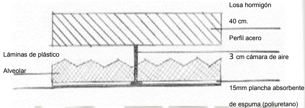
Corte detalle panel para cielo
