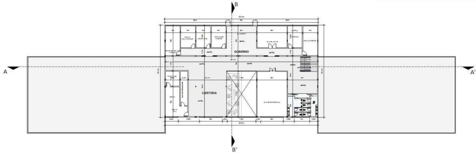
PLANTA ALTA ACOTADA
