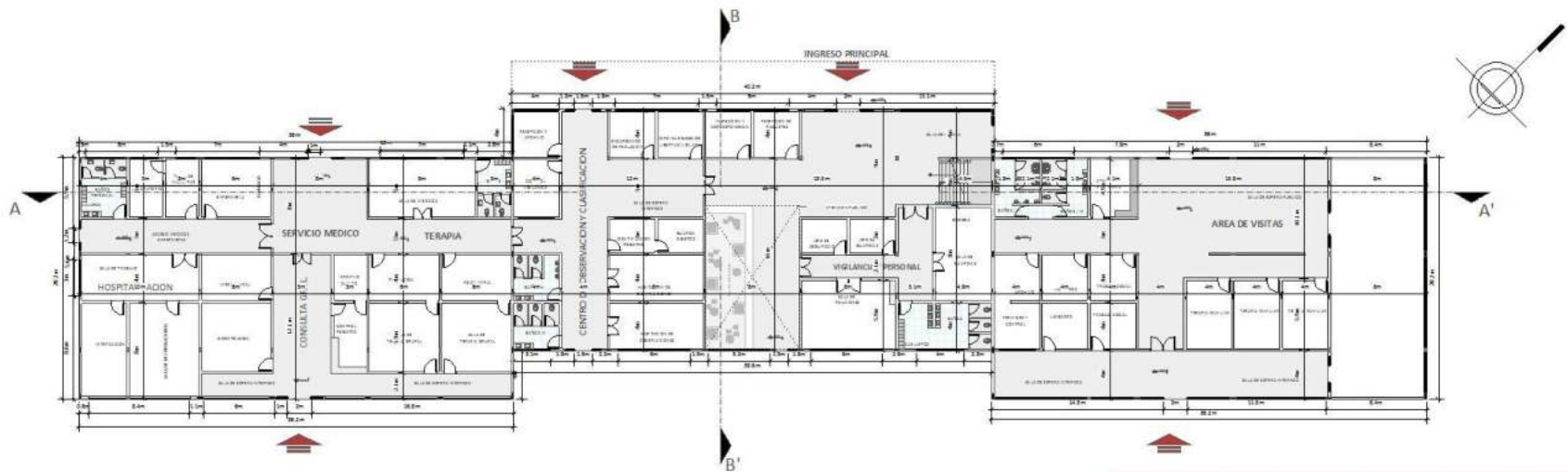
PLANTA BAJA ACOTADA
