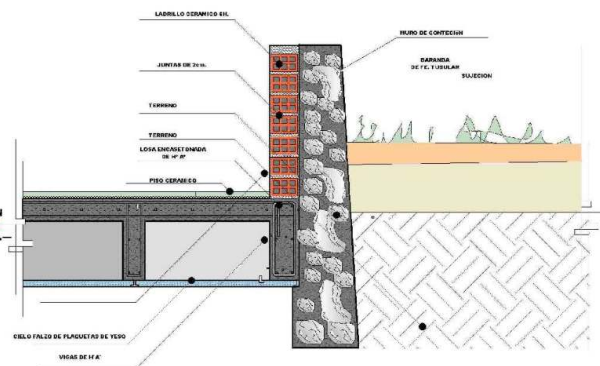
DETALLES CONSTRUCTIVOS
