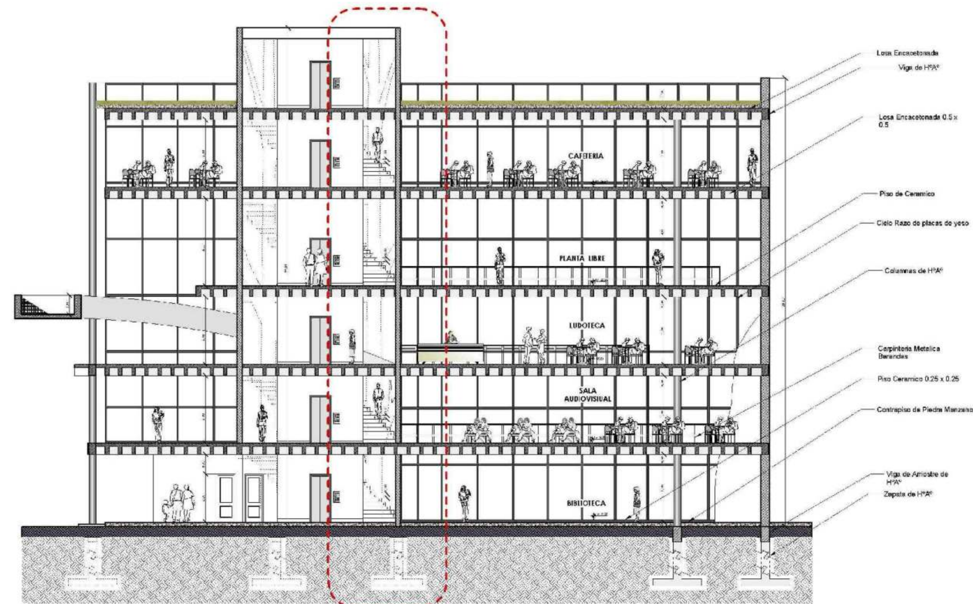
CORTE LONGITUDINAL
