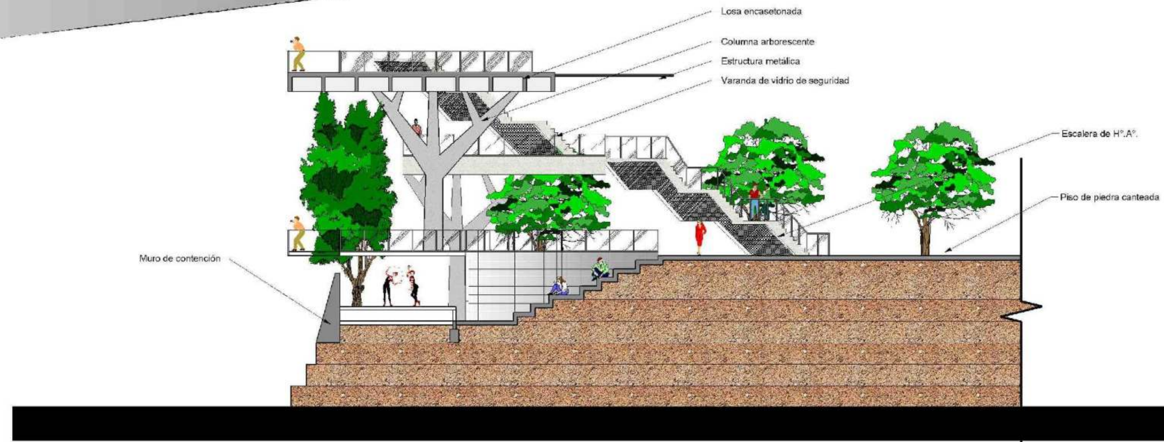
CORTE A-A''
