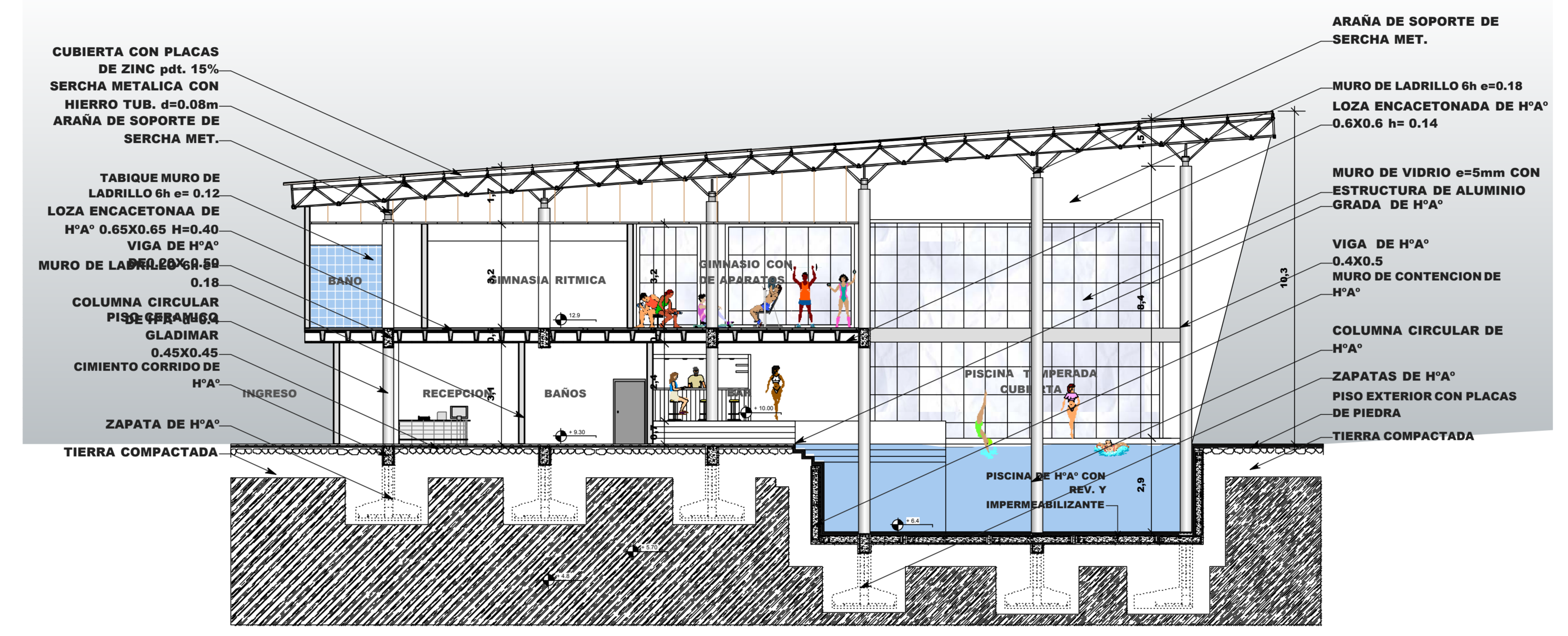
CORTES A-A' ESC. 1:100
