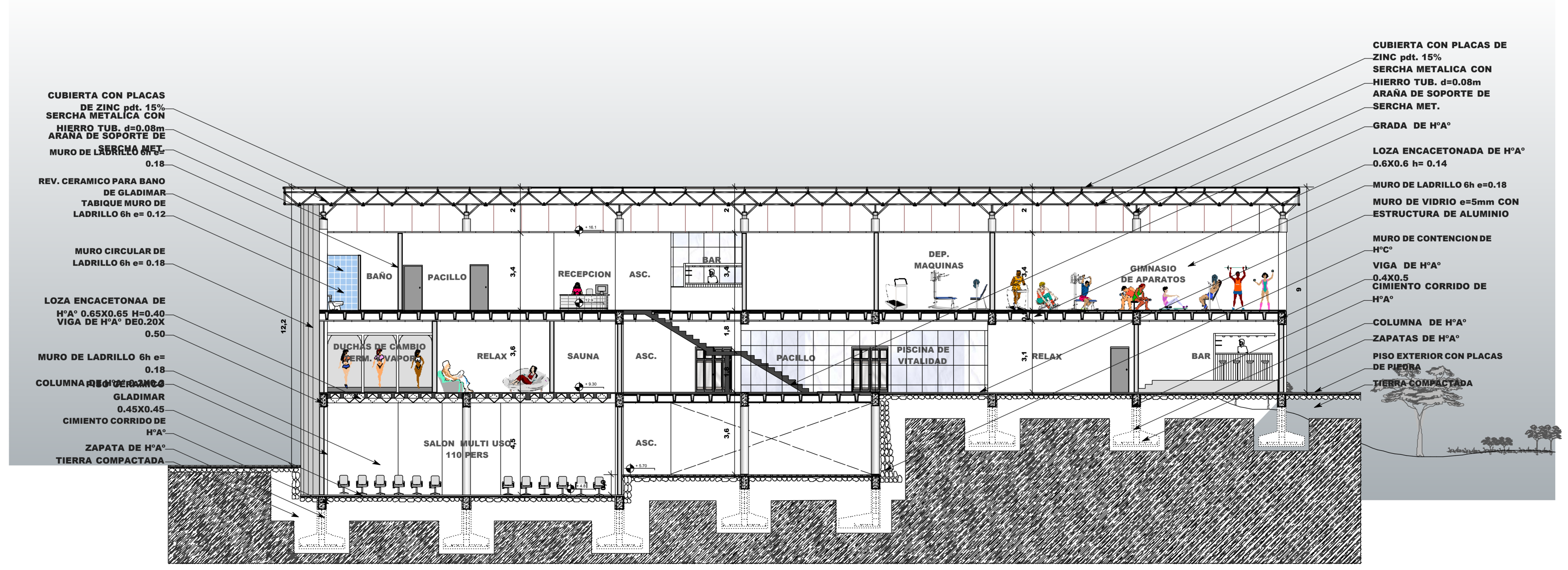
CORTES B-B' ESC. 1:100
