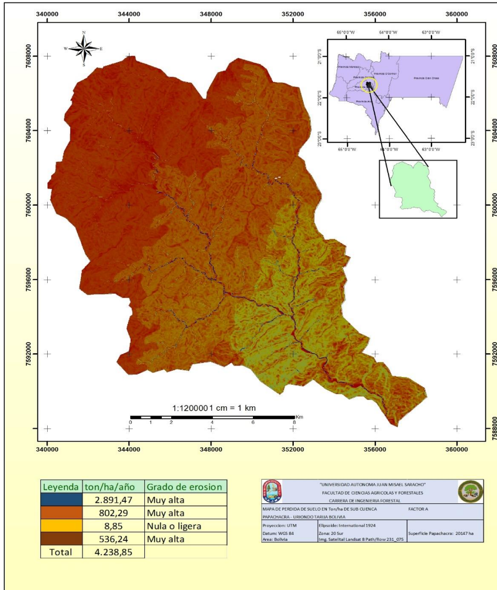
Mapa 5; resultados de perdida de suelo (A)
