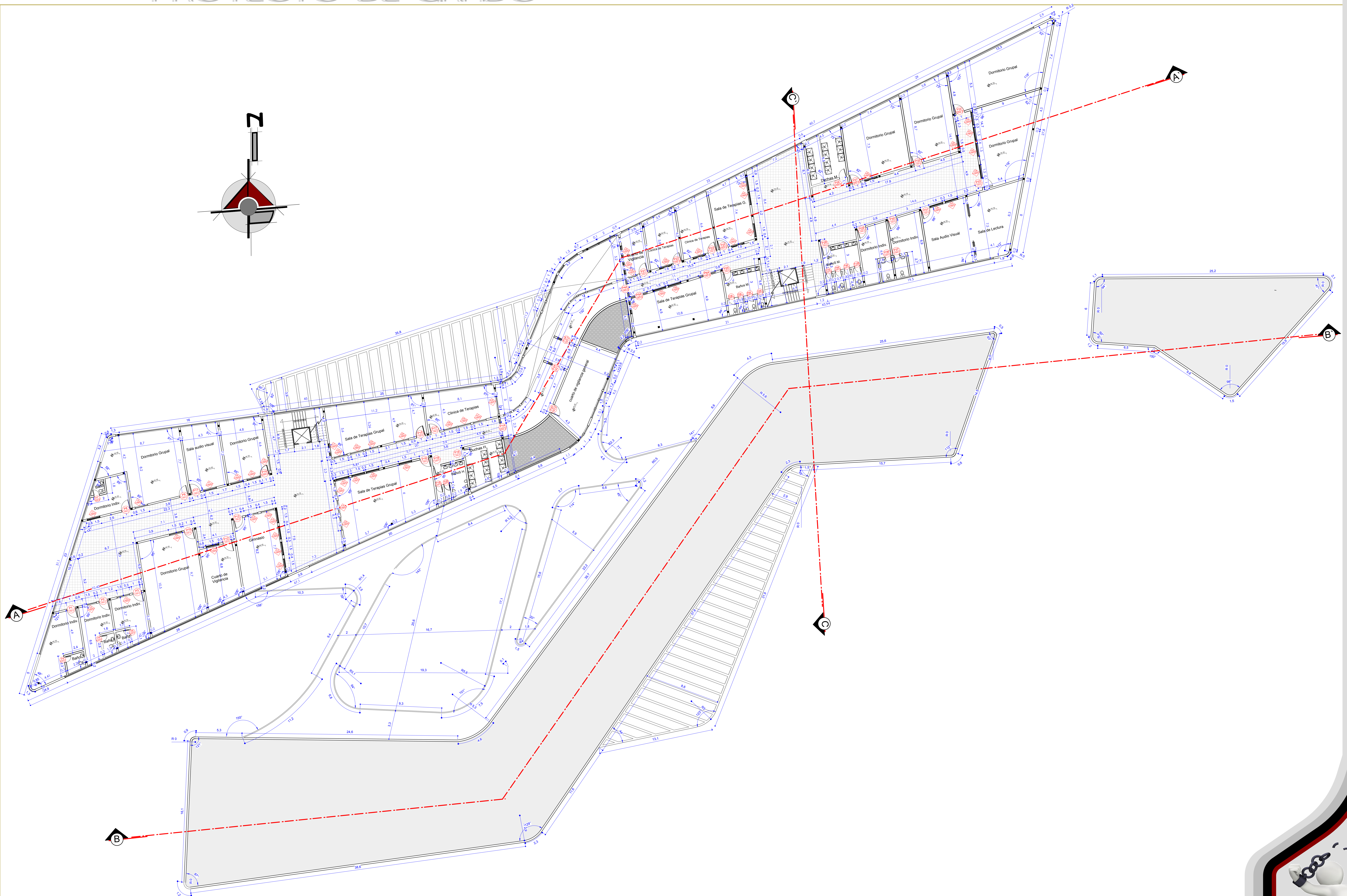
PLANTA ACOTADA PLANTA ALTA (1er Piso) ESC. 1: 150
