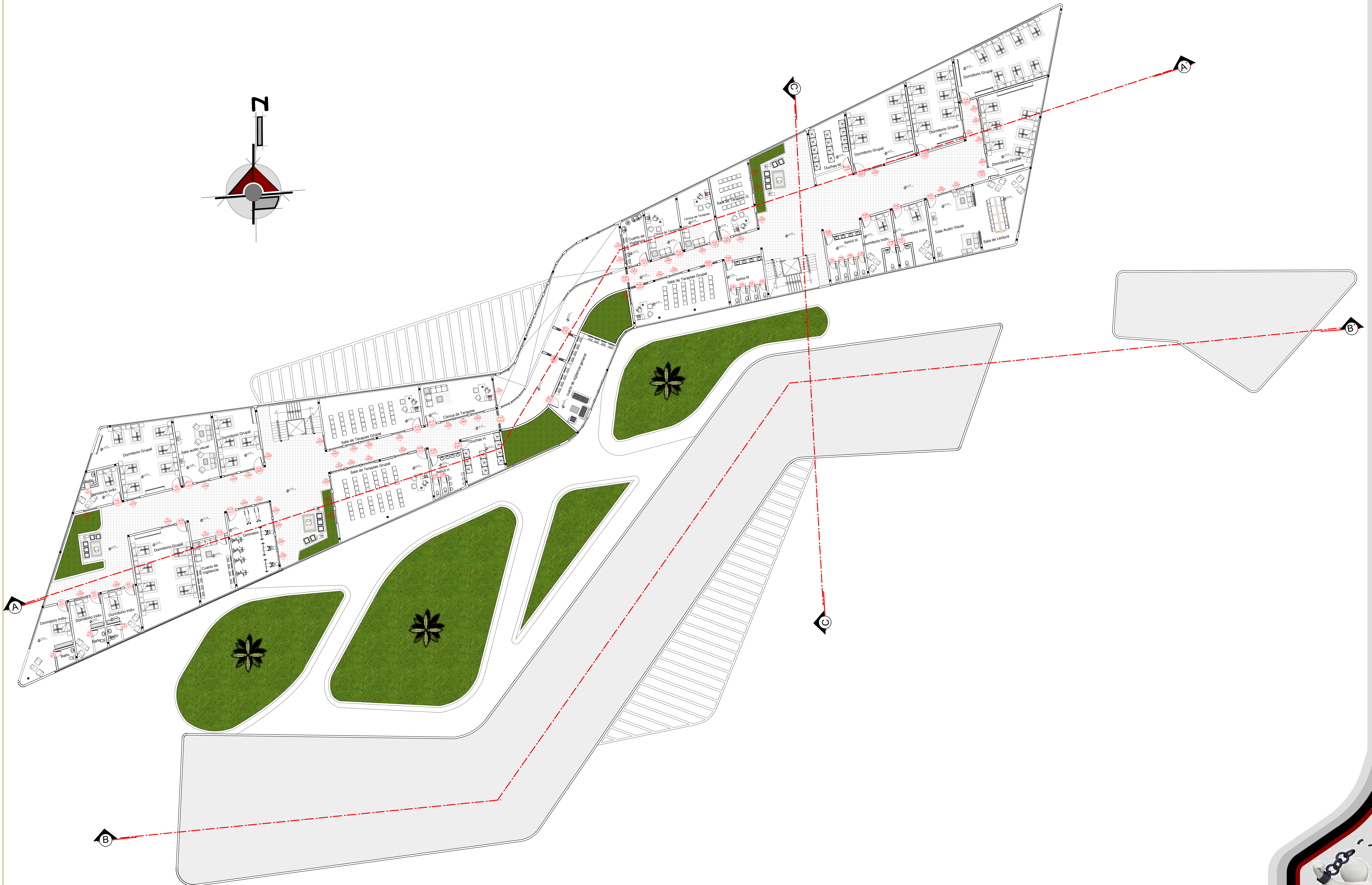
PLANTA AMOBLADA PLANTA ALTA (1er Piso) ESC. 1: 150
