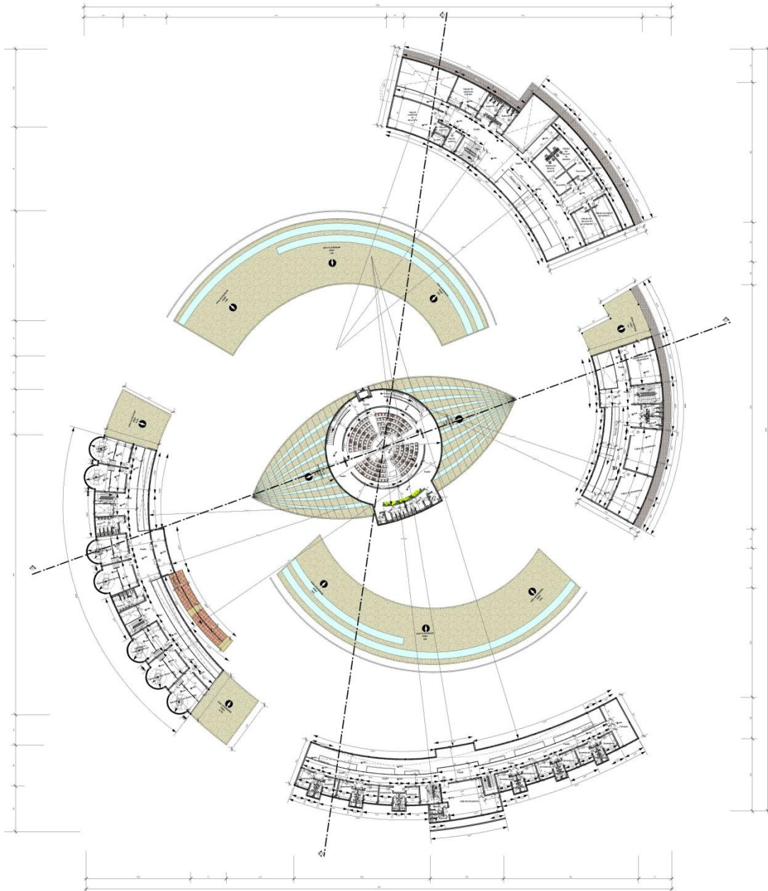
PRIMERA PLANTA ACOTADA ESC.: 1:100
