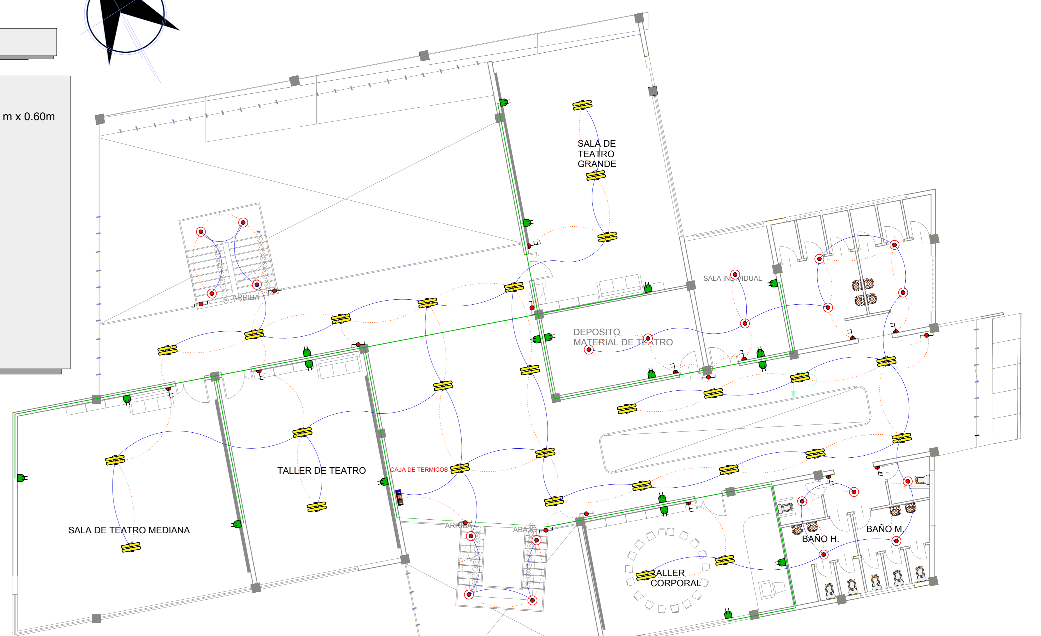
INSTALACION ELECTRICA ESC: 1:100
