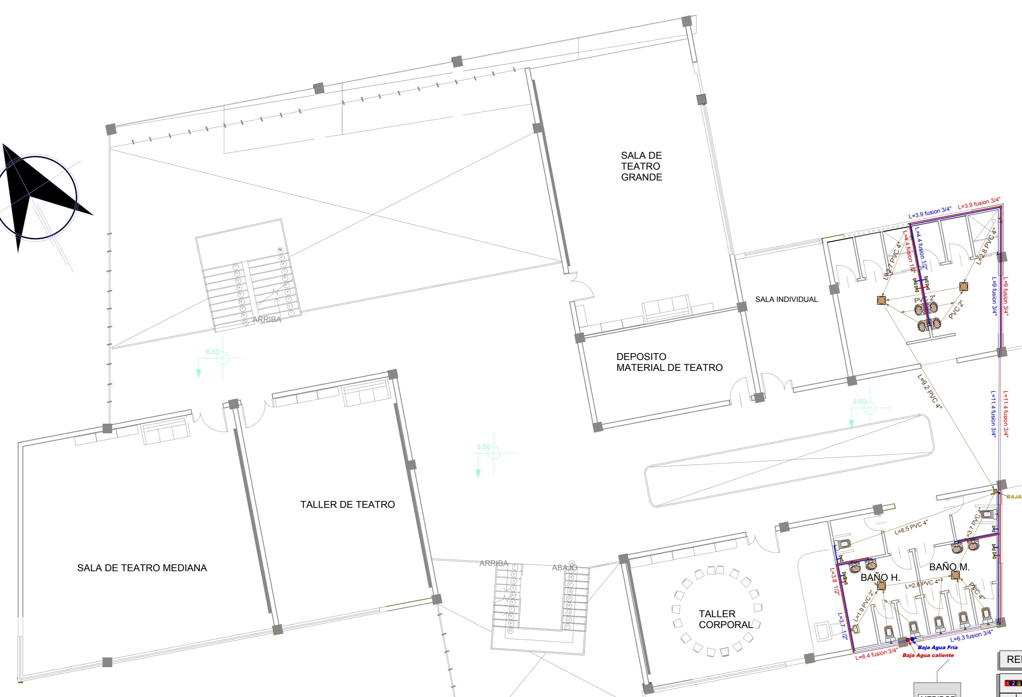
INSTALACION AGUA POTABLE Y INSTALACION SANITARIA SEGUNDA PLANTA ESC: 1:100
