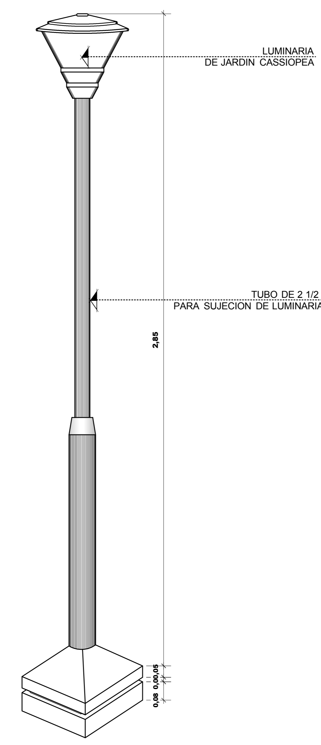
ISOMETRIA LUMINARIA EXTERIOR jardin ESCALA 1 : 10
