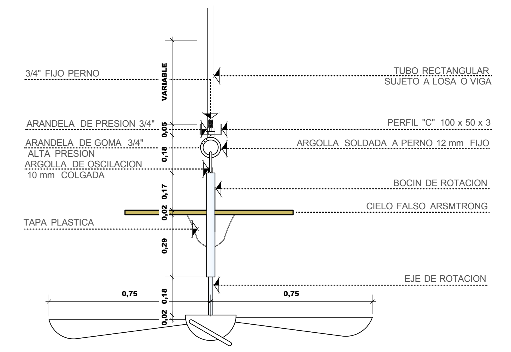
VENTILADOR DE TECHO PANASONIC F - 5609H ESCALA 1 : 10
