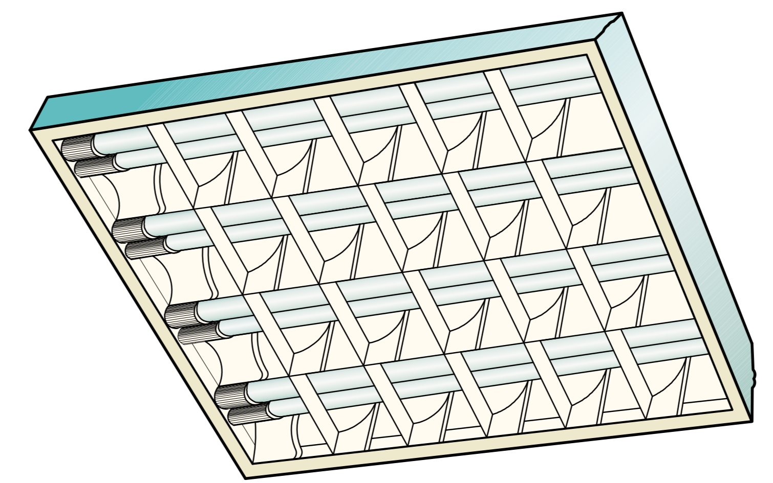
ISOMETRIA ILUMUNACION FLUORESCENTE MODELO EAE 420 MARCA FyK ESCALA 1 : 5
