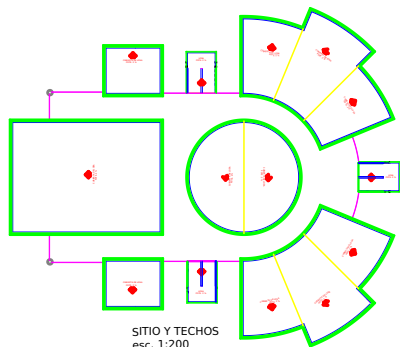
SITIO Y TECHOS esc. 1:200
