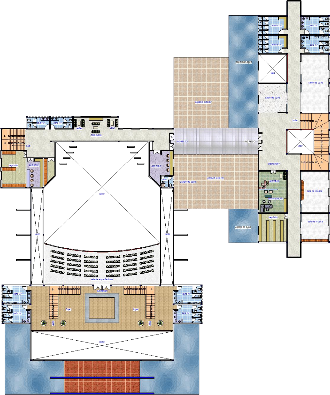
PLANTA ALTA AMOBLADA
