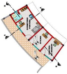
PLANTA AMOBLADA ESC. 1:100
