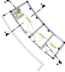
INST. ELÉCTRICA ESC. 1:100
