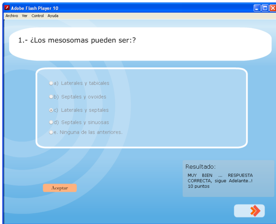
Figura 118: Pantalla evaluación
