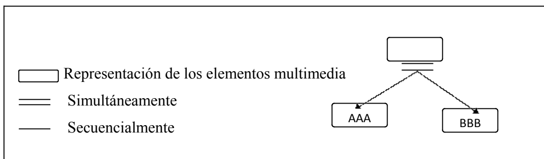
Figura 12: Diseño navegacional
