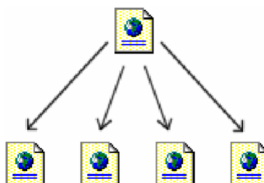
Figura 8: Estructura jerárquica
