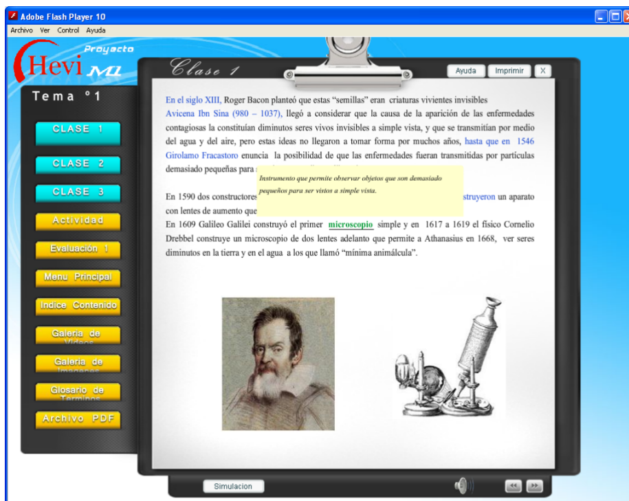
Figura 110: Pantalla clase 1
