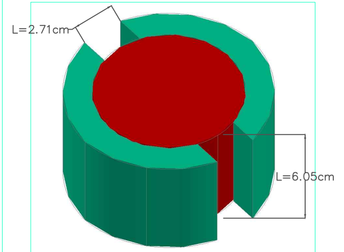
VISTA ISOMETRICA
