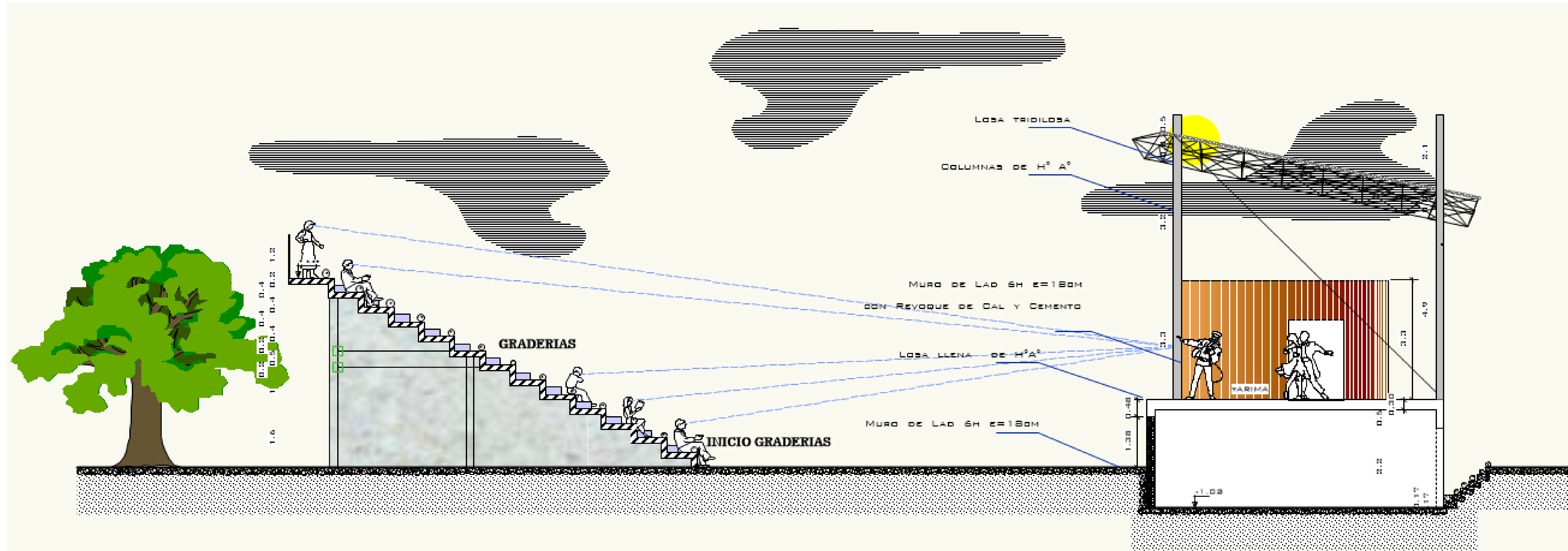
CORTE A-A
