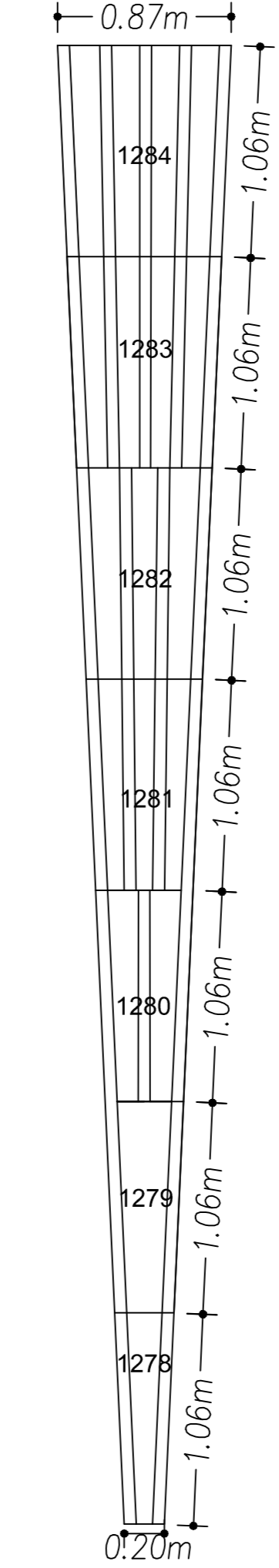
DISTRIBUCION DE COSTILLAS EN LOSA INFERIOR Esc. 1:25
