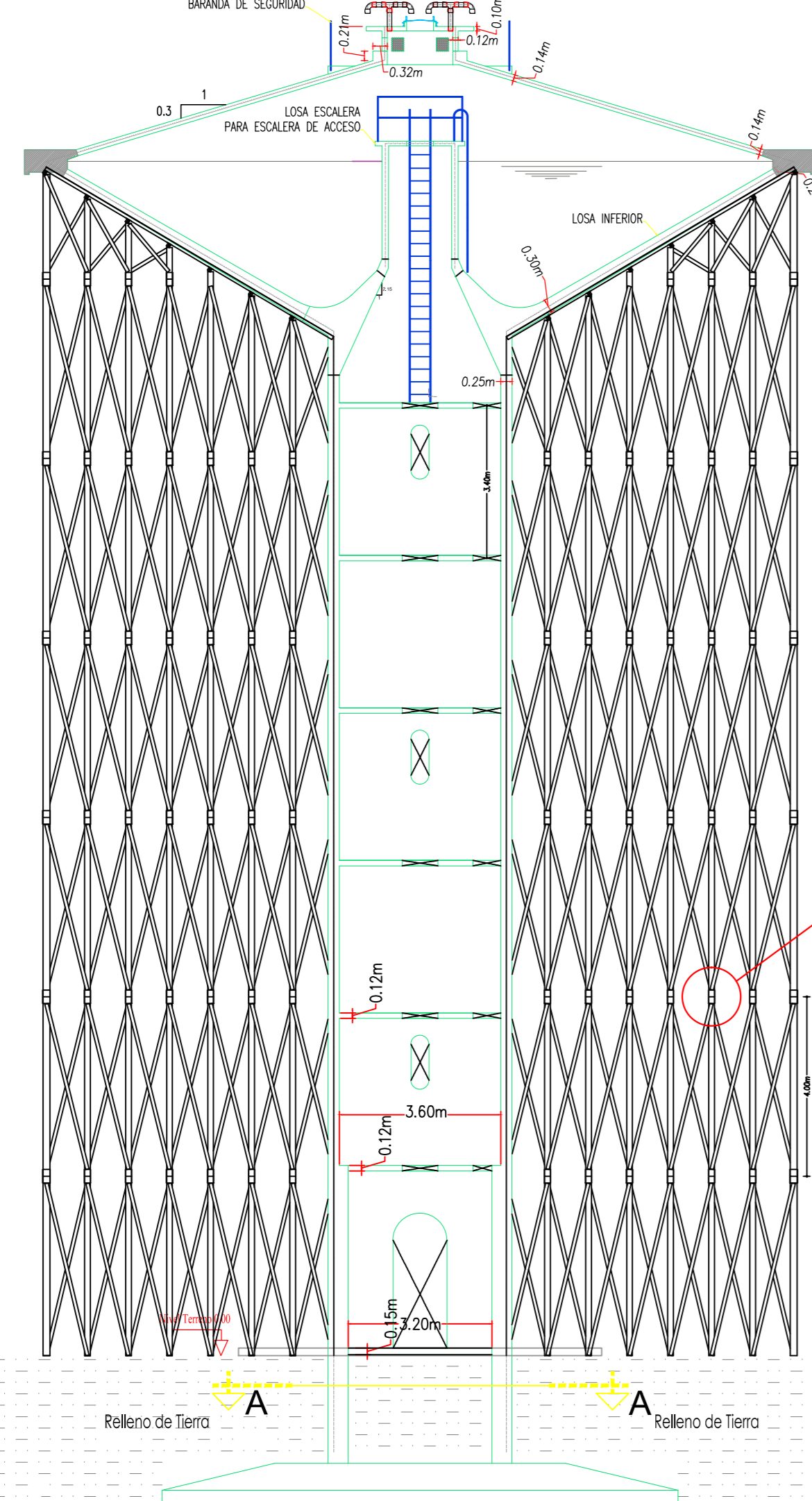
PLANO MODELO DE ENCOFRADO TRADICIONAL APOYADO SOBRE TERRENO NATURAL Esc. 1:100 A-A
