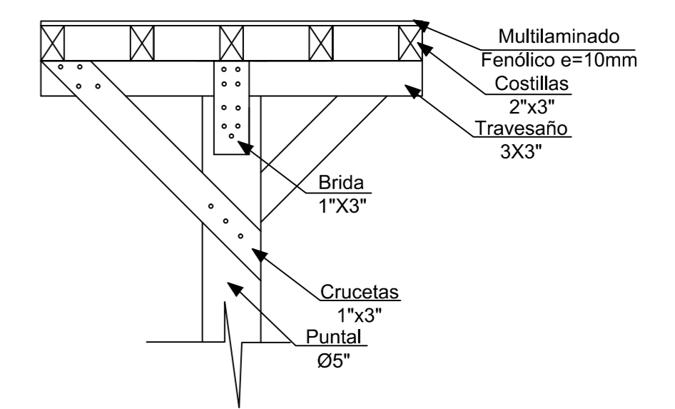
DETALLE DE LOS ELEMENTOS DEL PUNTAL (1284) Esc. 1:10
