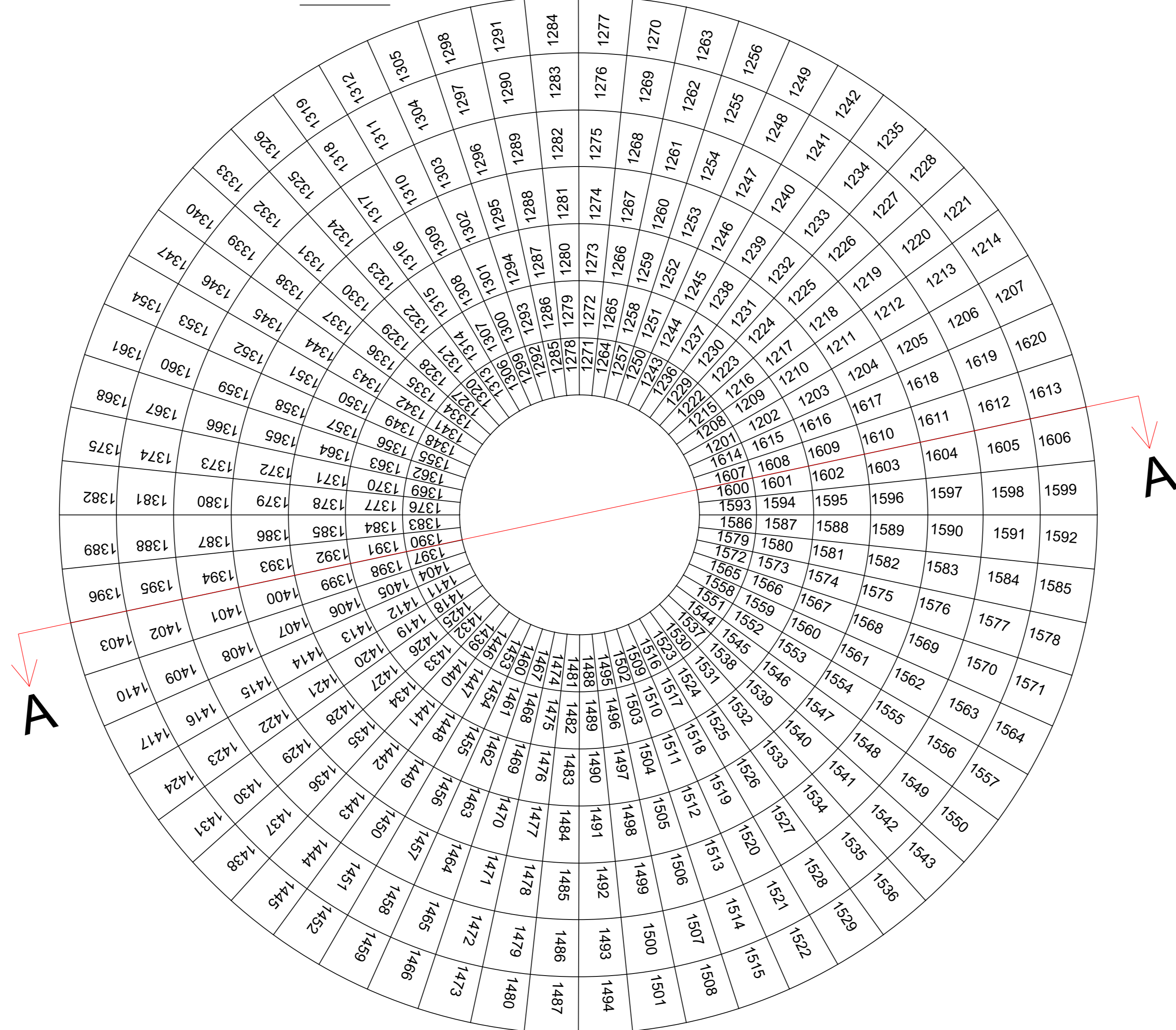
PLANO VISTA EN PLANTA DE LA LOSA INFERIOR Esc. 1:50
