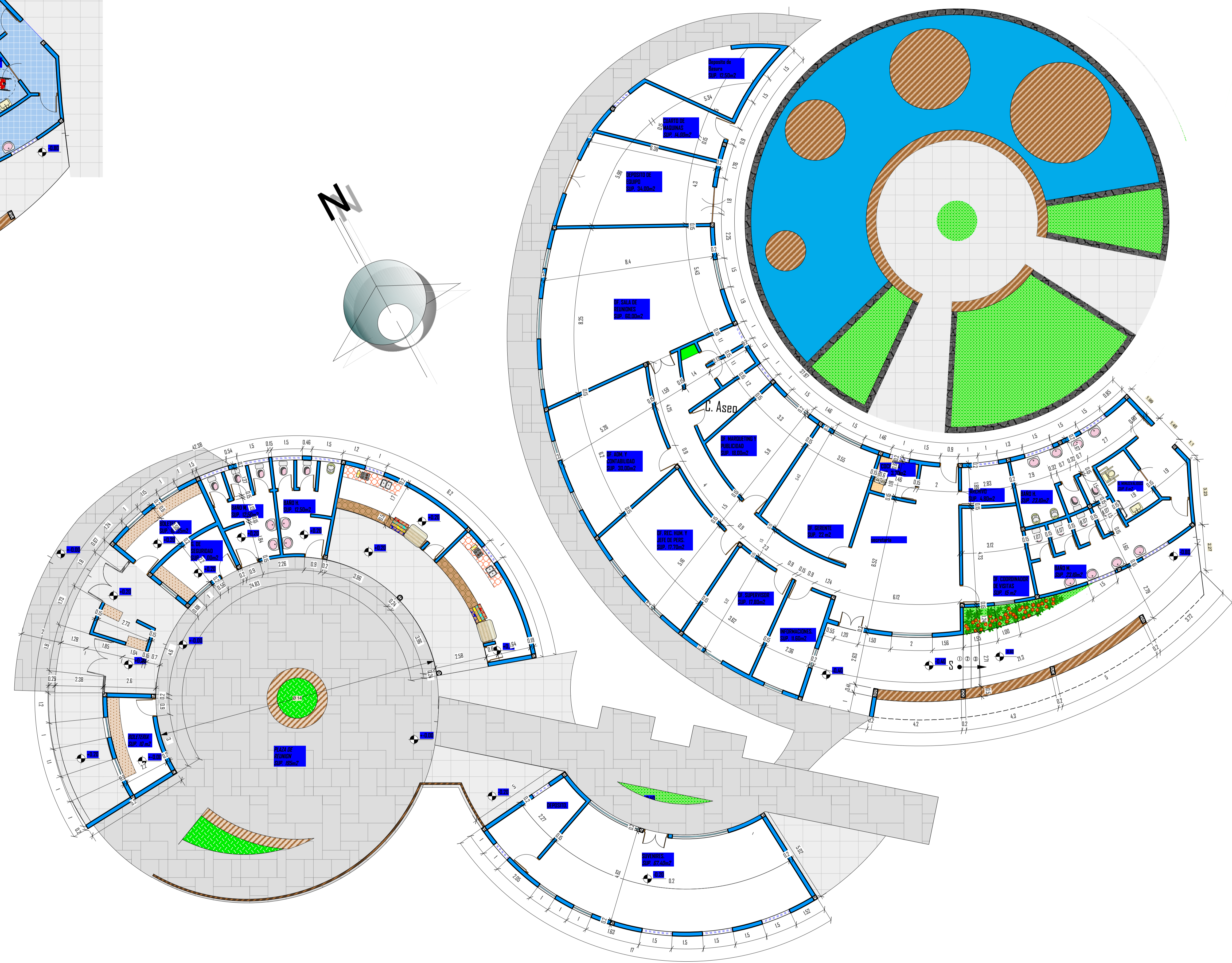
PLANTA AGOTADA (ZONA DE INGRESO Y ADMINISTRACION) ESCALA: 1:100
