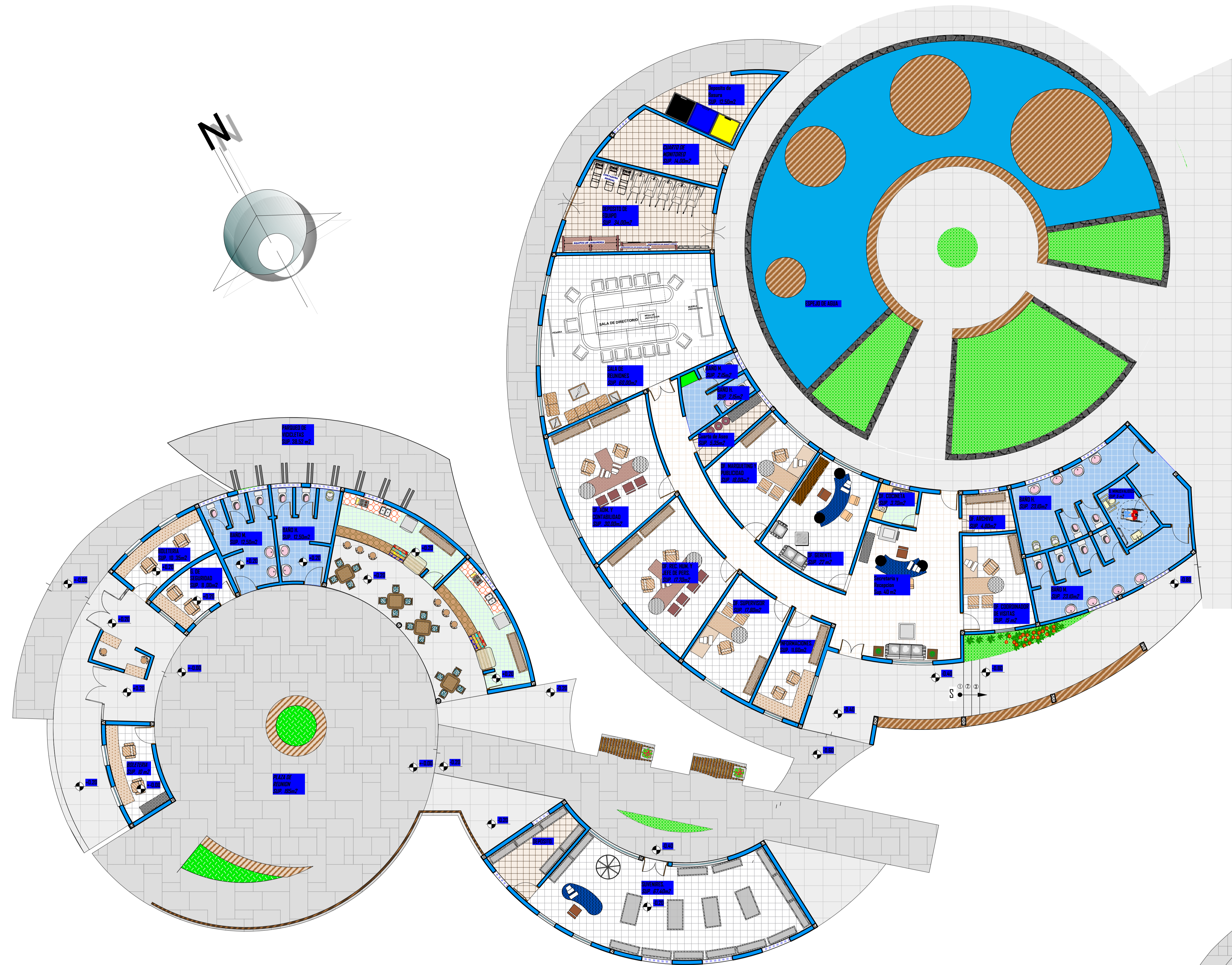
PLANTA AMOBLADA (ZONA DE INGRESO Y ADMINISTRACION) ESCALA: 1:100
