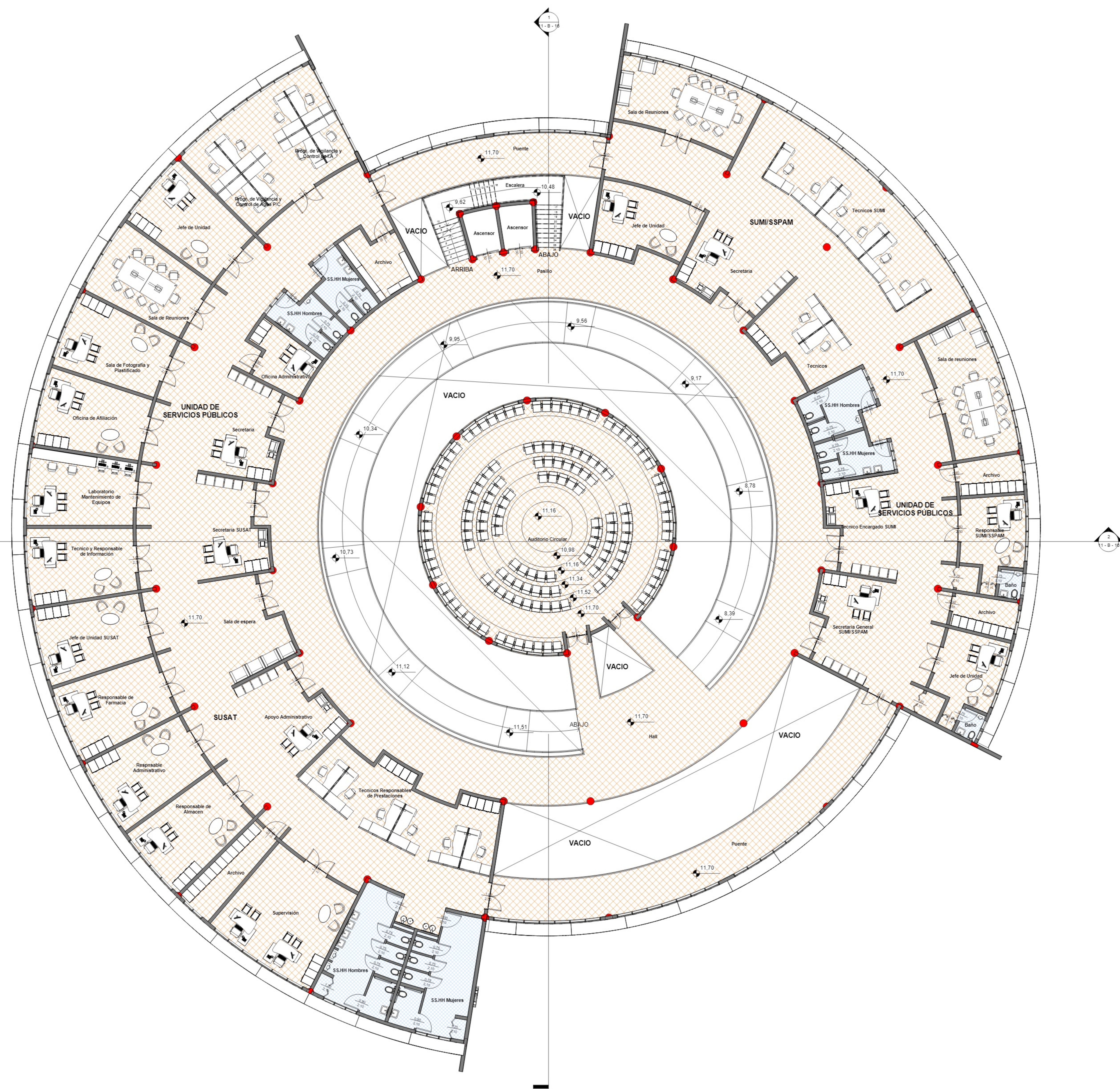
04 - Tercer Piso 1 : 100
