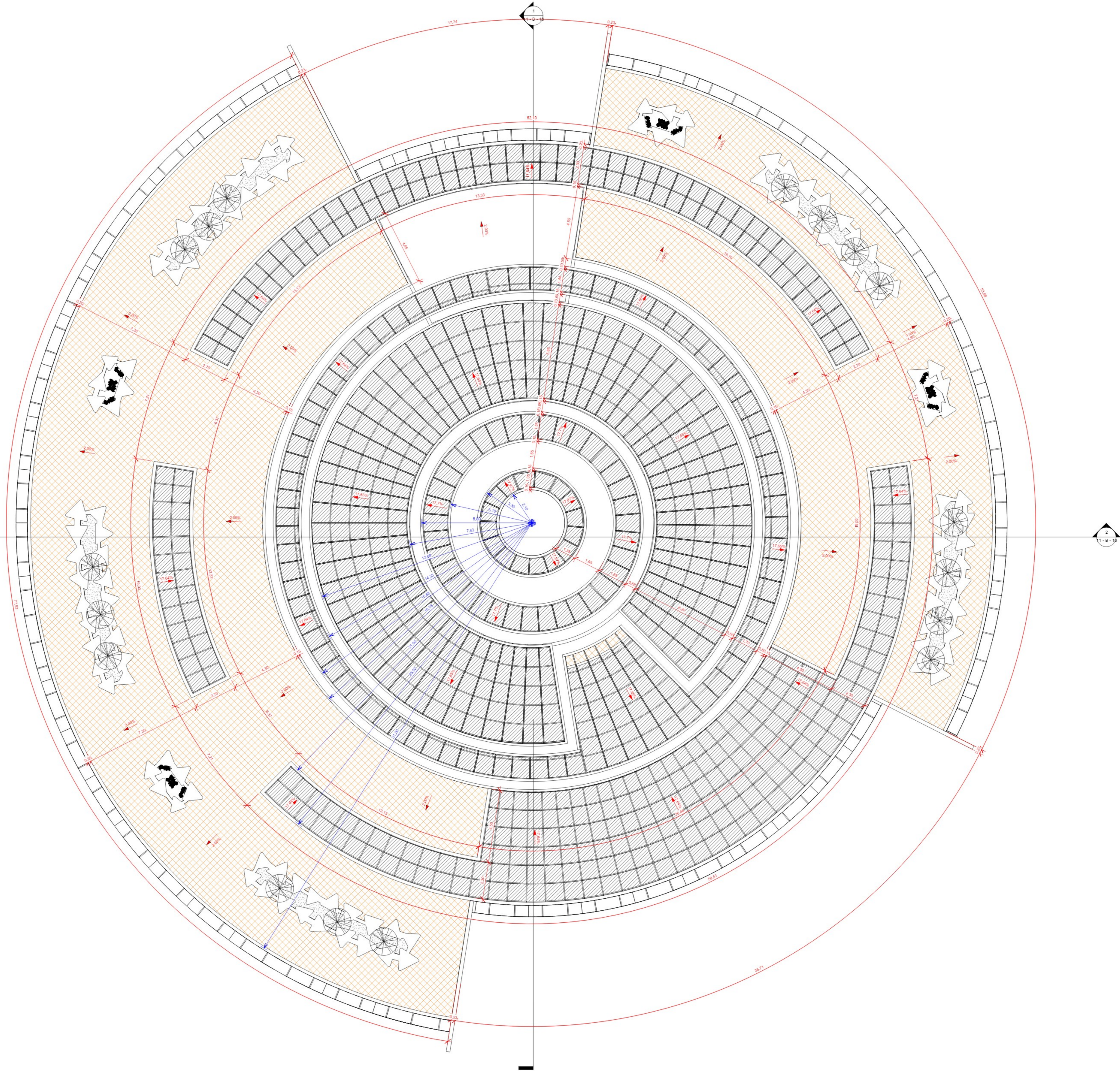
06 - Cubierta 1 : 100
