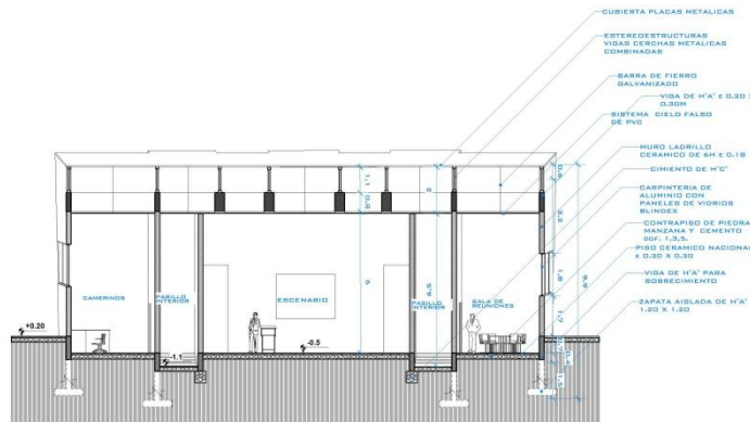
CORTE I-I
