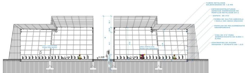
CORTE F-F
