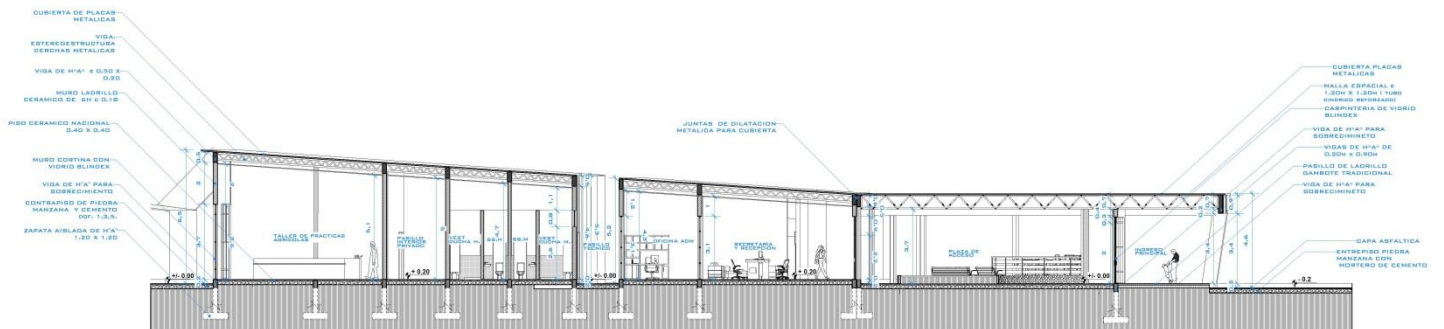
CORTE C-C
