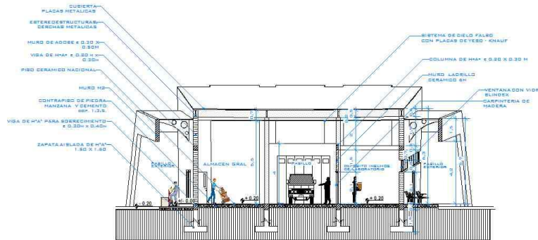
CORTE B-B
