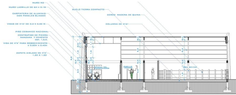
CORTE G-G
