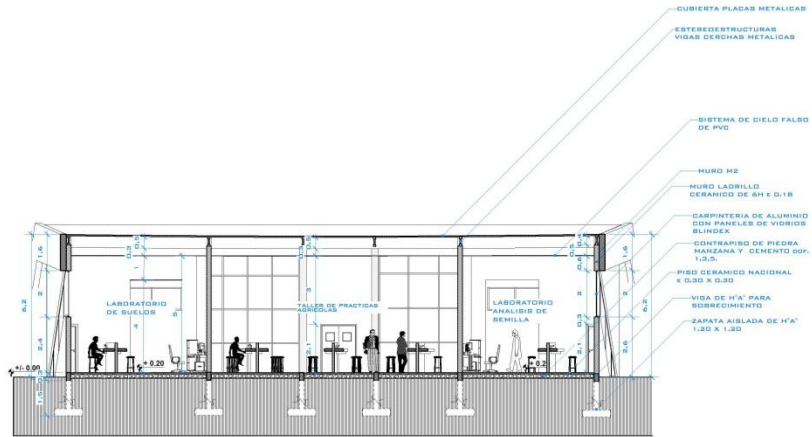
CORTE D-D
