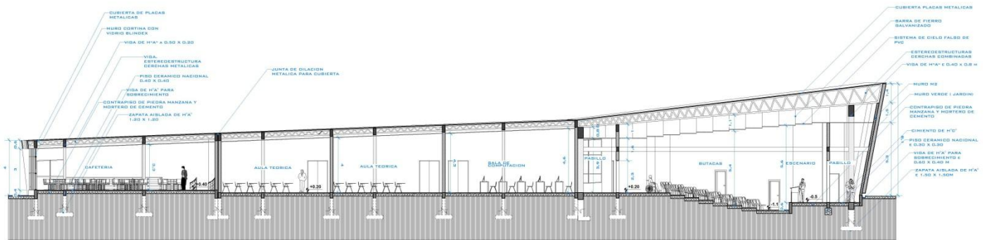
CORTE H-H
