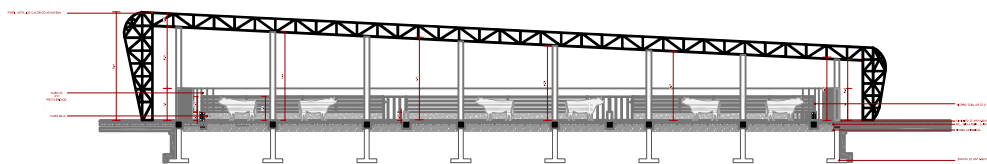
CORTE A-A GANADO MAYOR ESC:1.100
