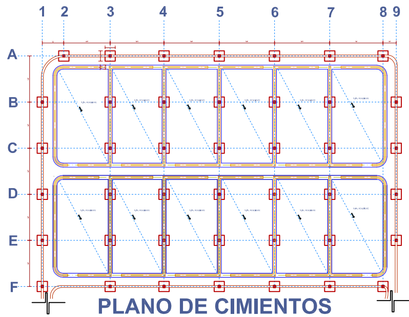
PLANO DE CIMIENTOS ESC:1.100
