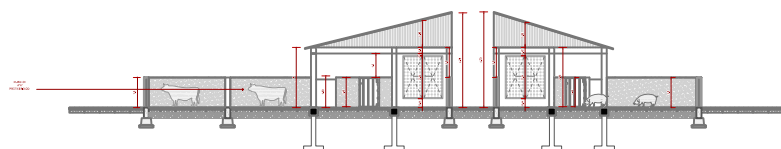
CORTE A-A GANADO MENOR ESC:1.100
