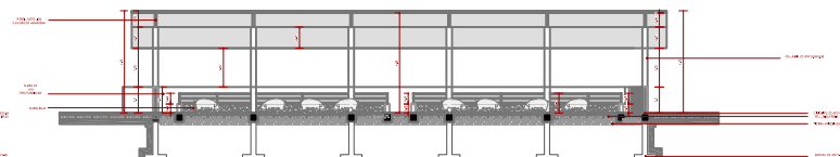
CORTE B-B GANADO MENOR ESC:1.100
