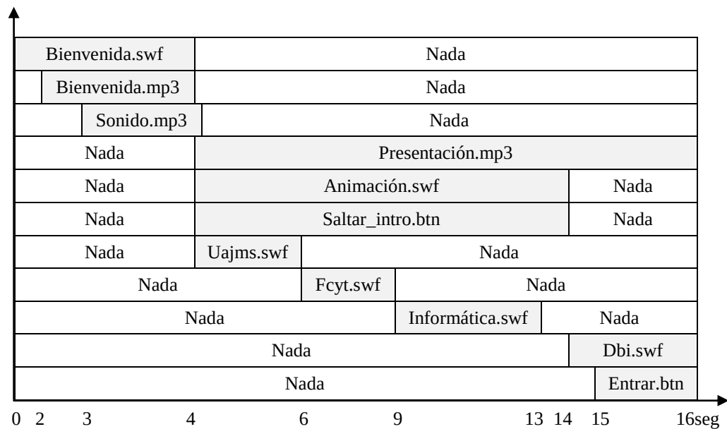
Figura 27: Sincronización Pantalla Presentación
