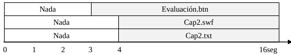
Figura 30: Sincronización Pantalla Capítulo2
