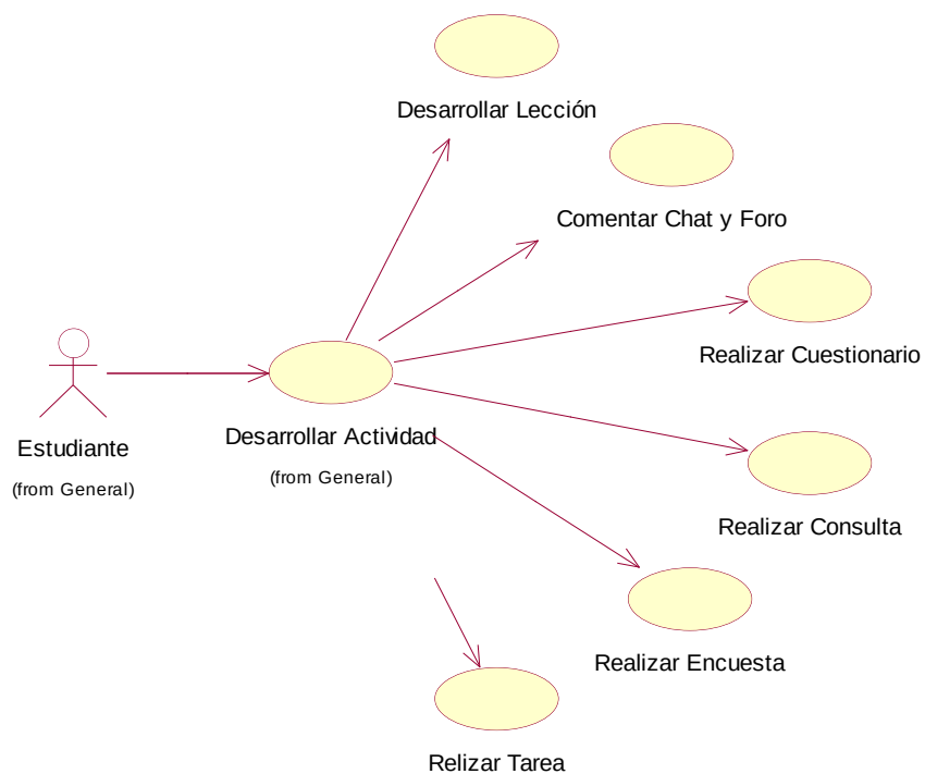
Figura 59: Diagrama de Casos de Uso Desarrollar Actividades
