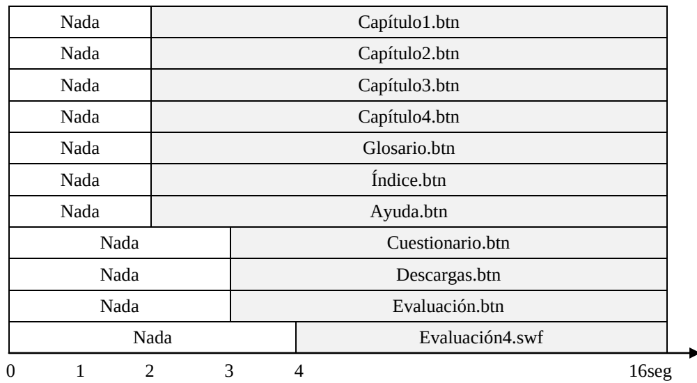
Figura 42: Sincronización Pantalla EvaluaciónCap4
