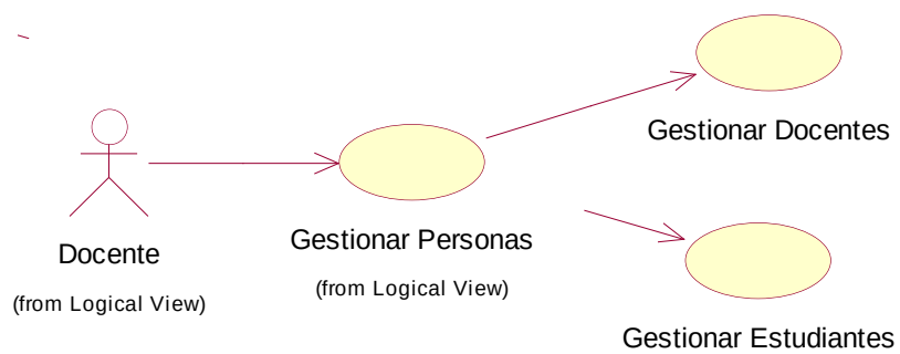
Figura 55: Diagrama de Casos de Uso Gestionar Personas
