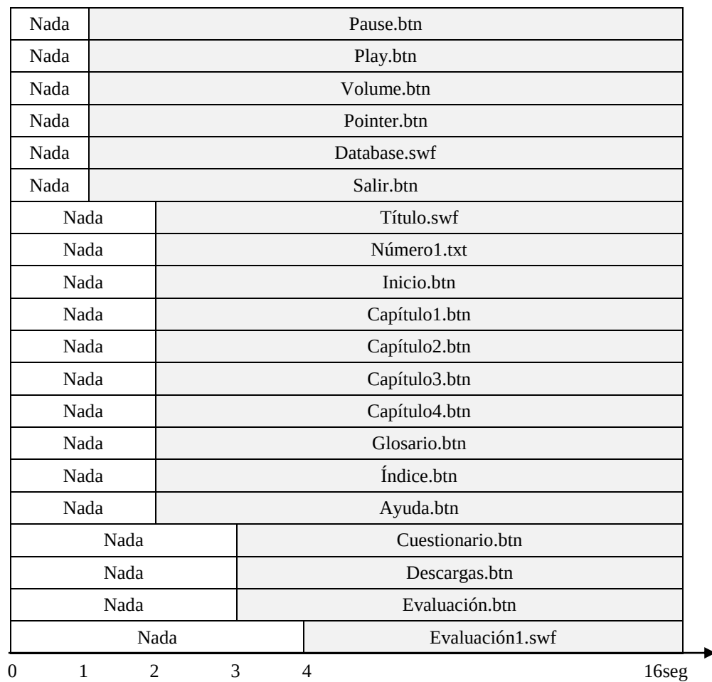
Figura 39: Sincronización Pantalla EvaluaciónCap1
