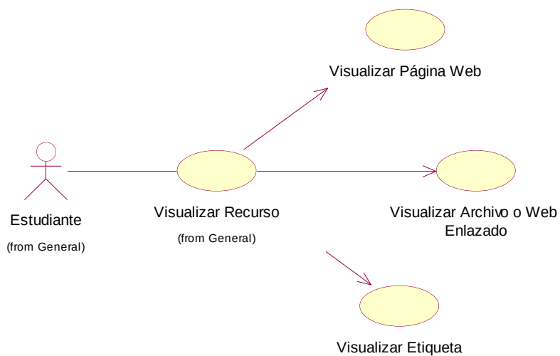
Figura 60: Diagrama de Casos de Uso Visualizar Recursos
