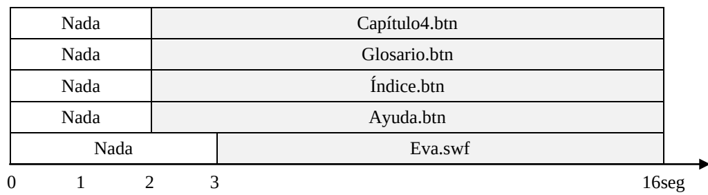
Figura 28: Sincronización Pantalla Inicio
