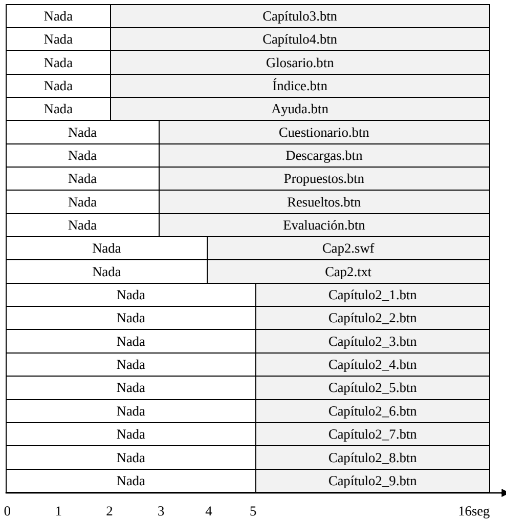
Figura 34: Sincronización Pantalla Capítulo2_N
