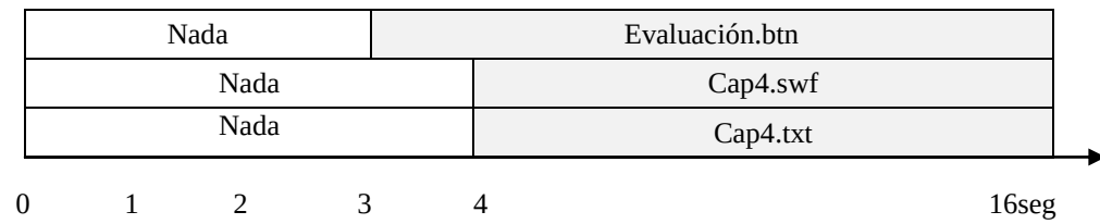
Figura 32: Sincronización Pantalla Capítulo4
