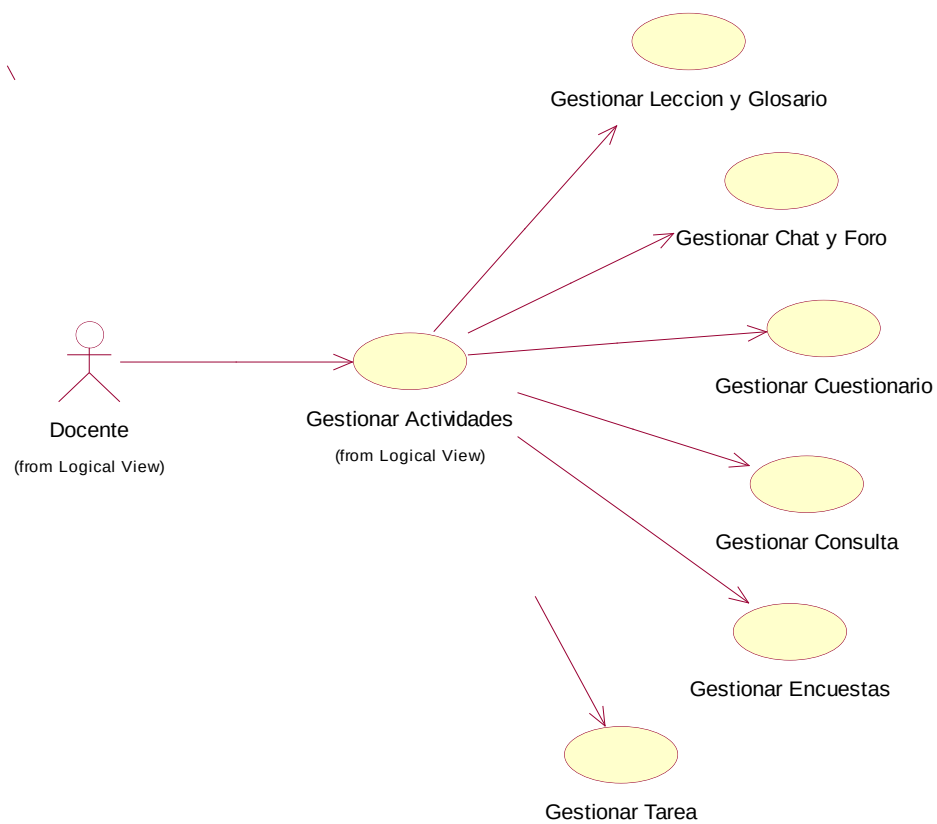
Figura 56: Diagrama de Casos de Uso Gestionar Actividades
