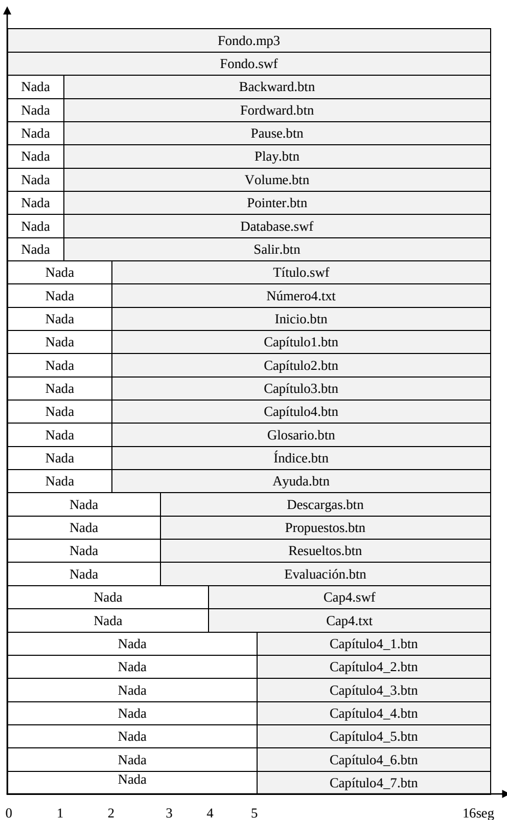
Figura 36: Sincronización Pantalla Capítulo4_N
