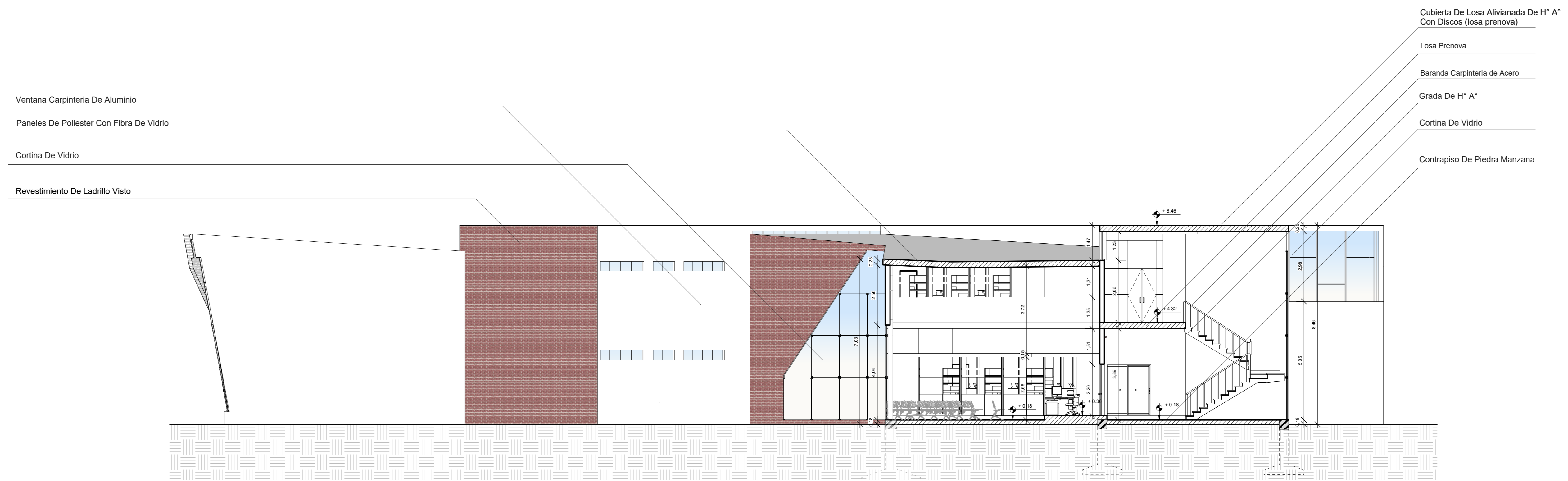
CORTE TRANSVERSAL D - D'
