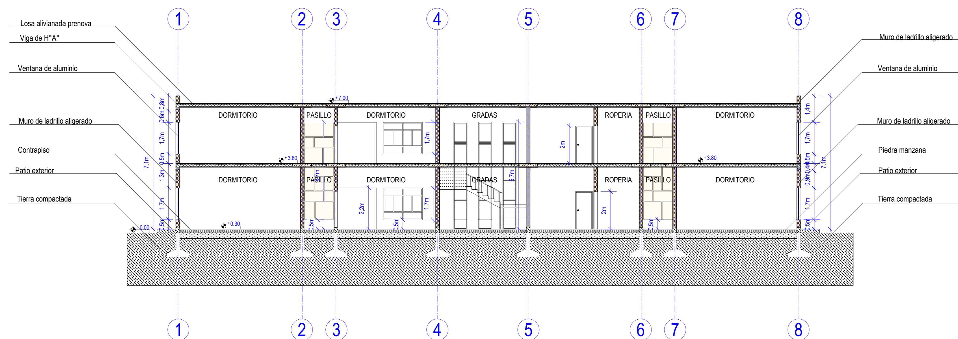
CORTE TRANSVERSAL C-C"
