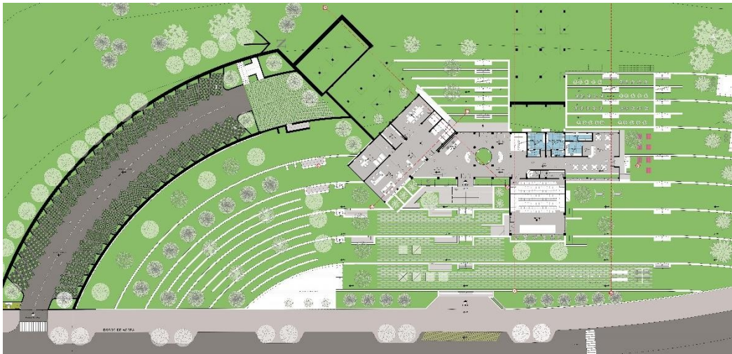
PLANTA BAJA
