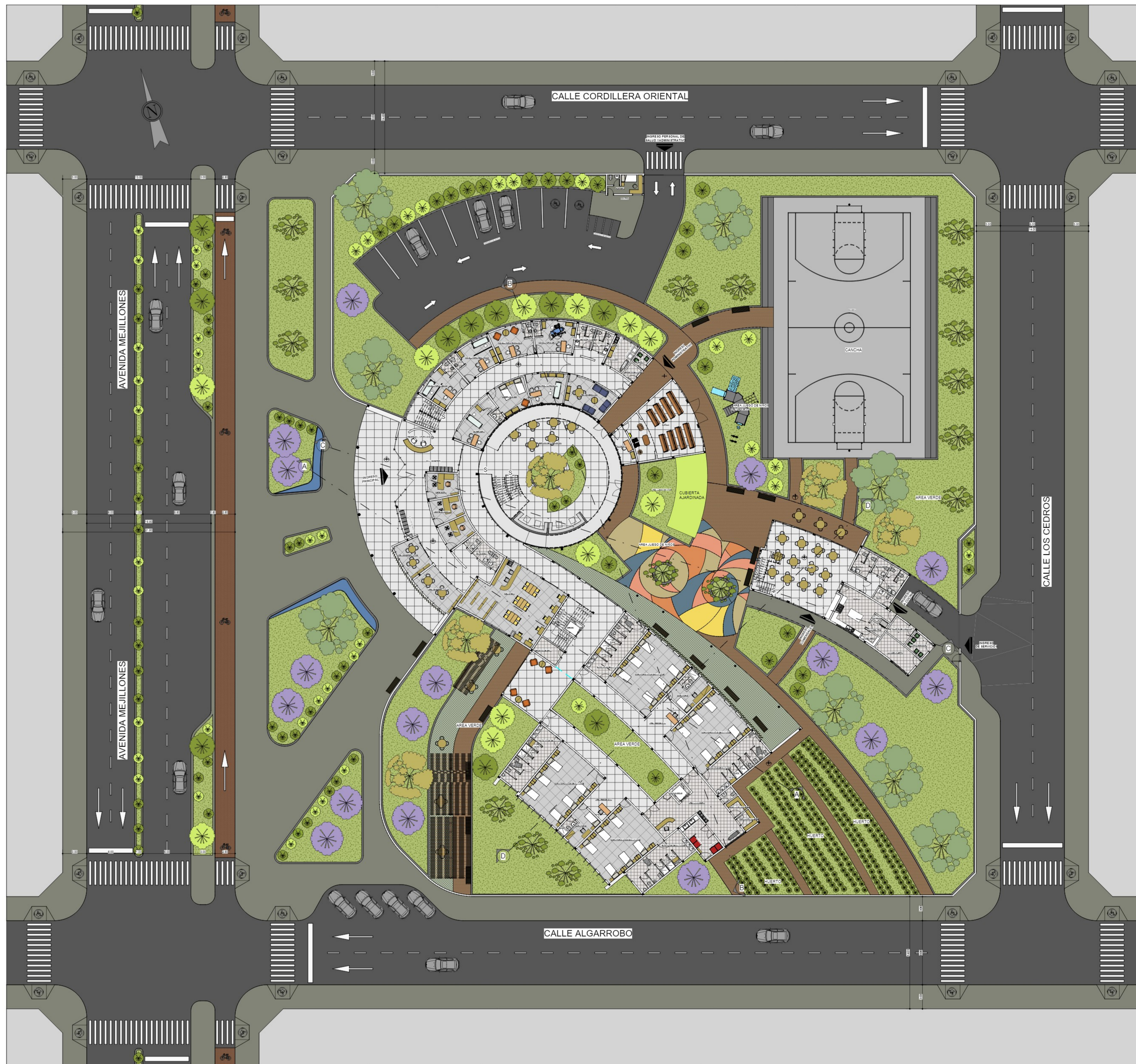
PLANO: PLANO PAISAJISTICO OTOÑO ESC. 1 : 200
