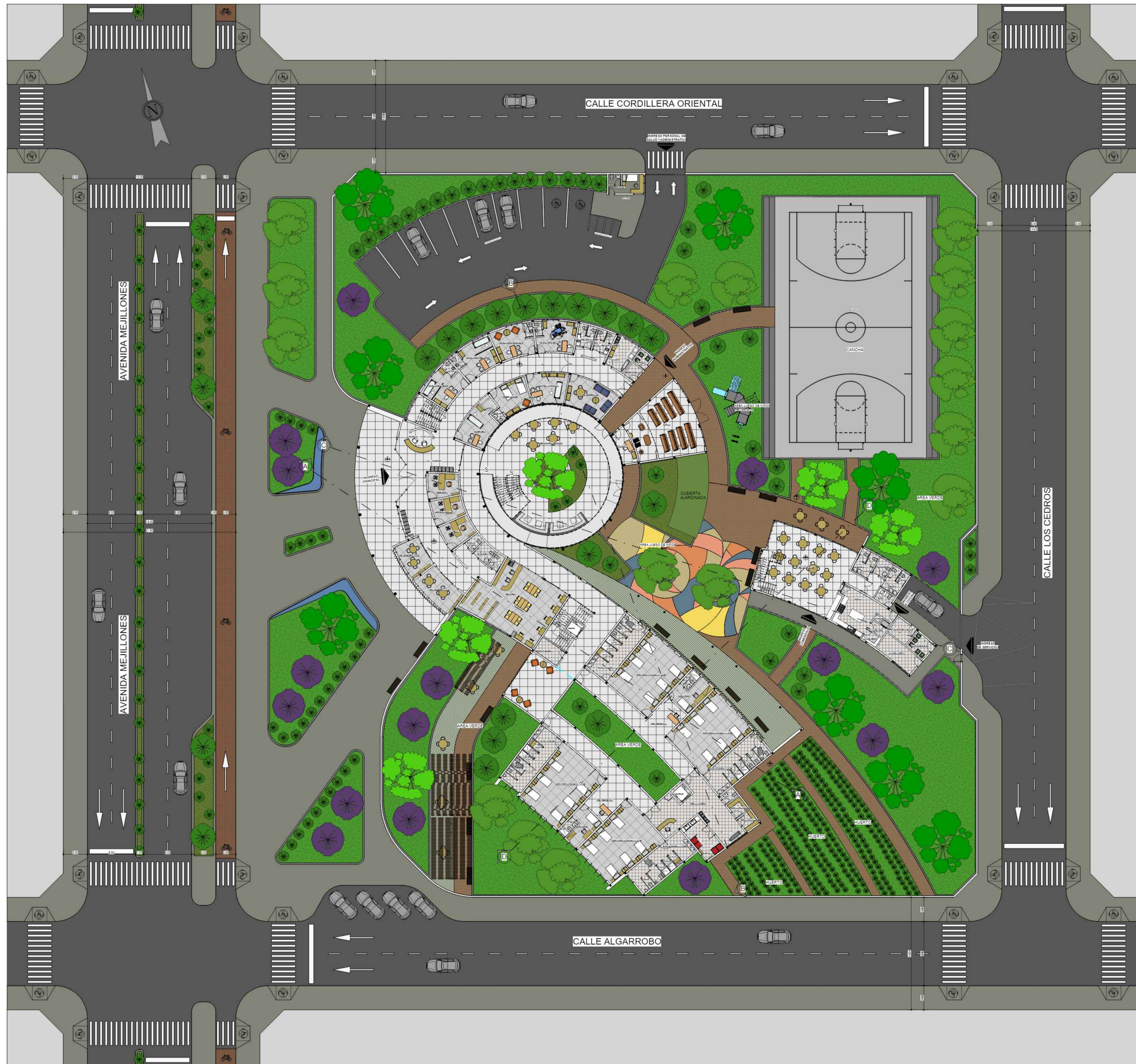
PLANO: PLANO PAISAJISTICO VERANO ESC. 1 : 200
