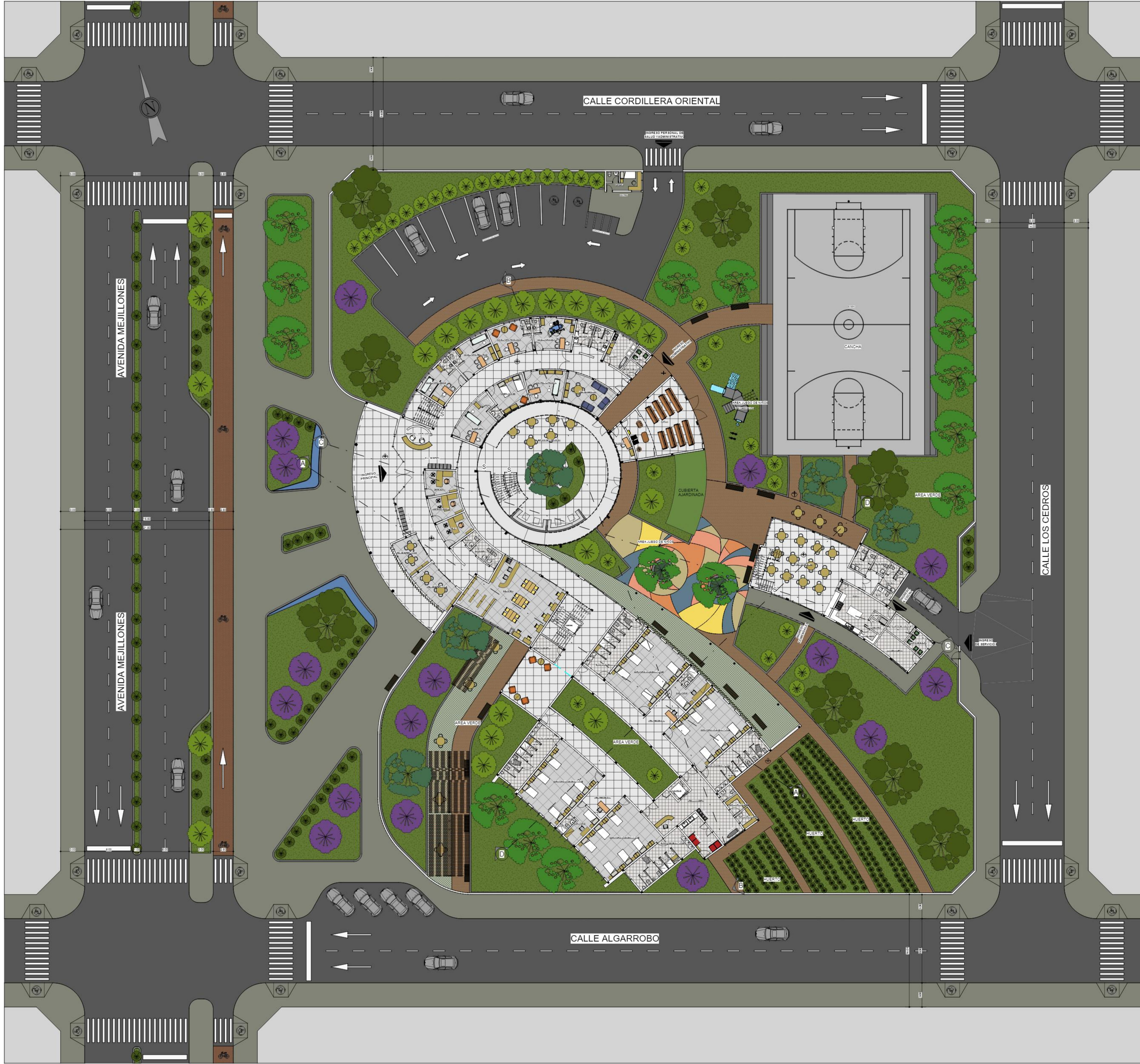
PLANO: PLANIMETRIA GENERAL ESC. 1 : 200
