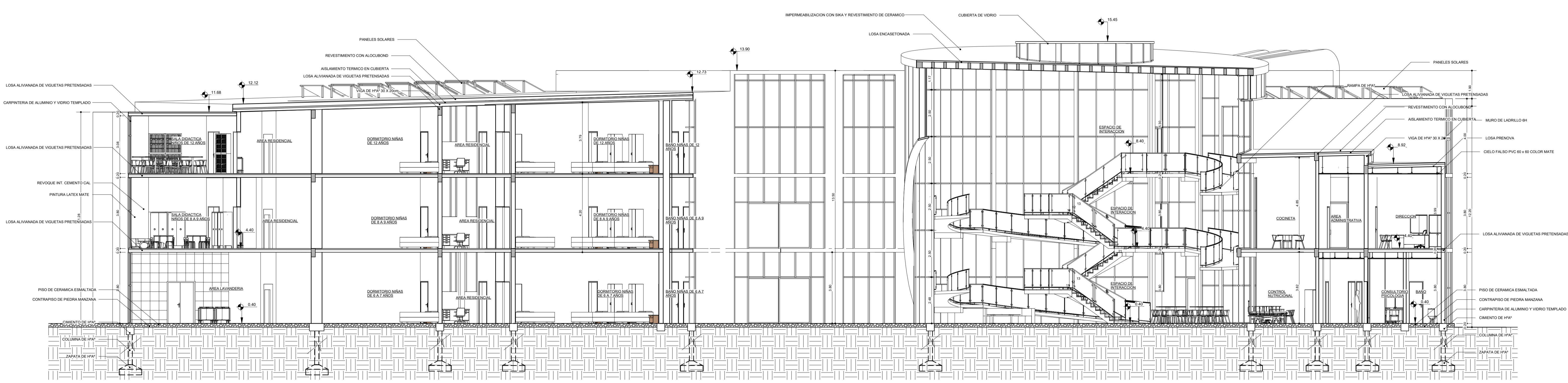
CORTE B - B ESC. 1:100
