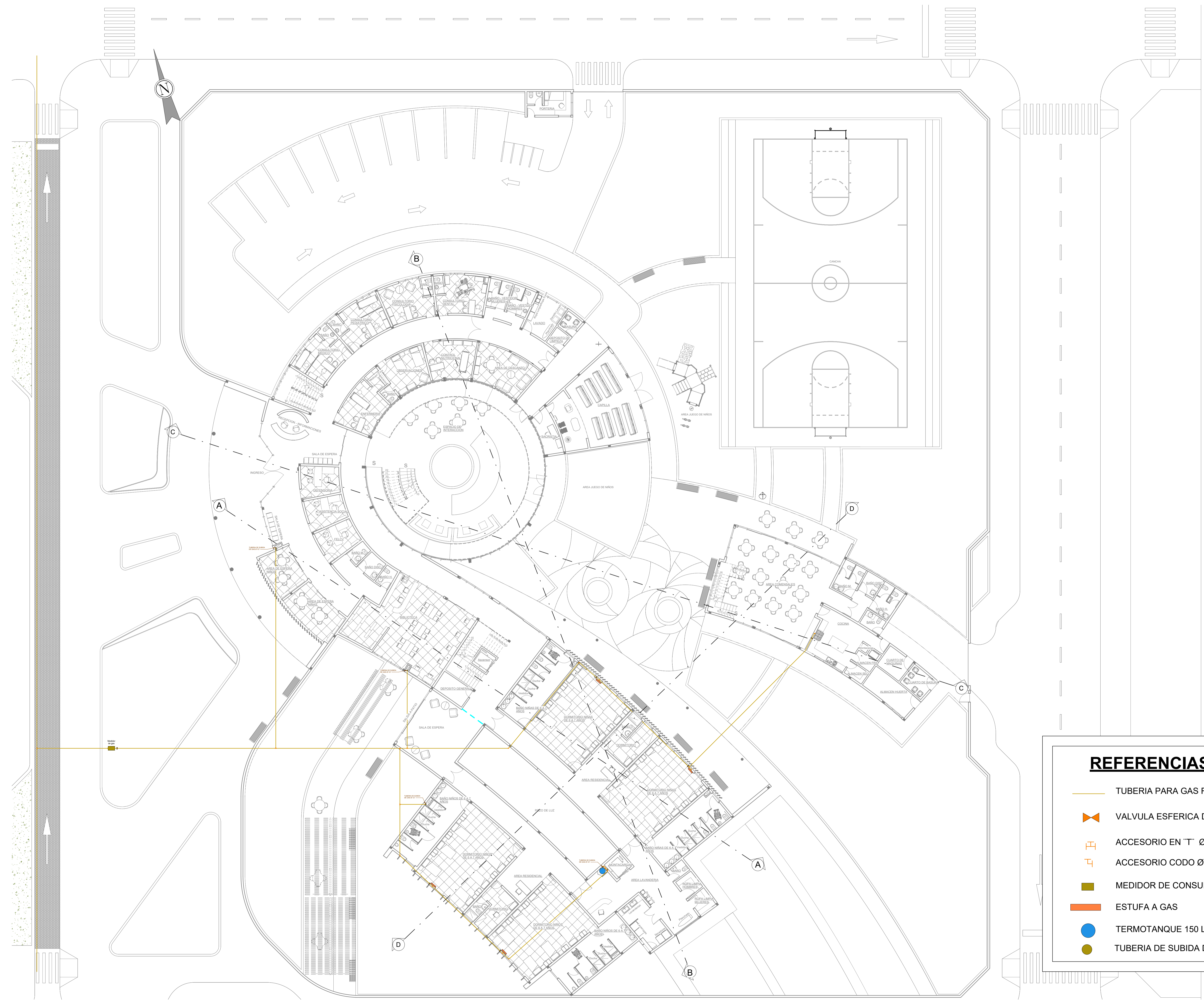
PLANO: PLANO DE INSTALACIONES DE GAS - PLANTA BAJA ESC.1 : 150
