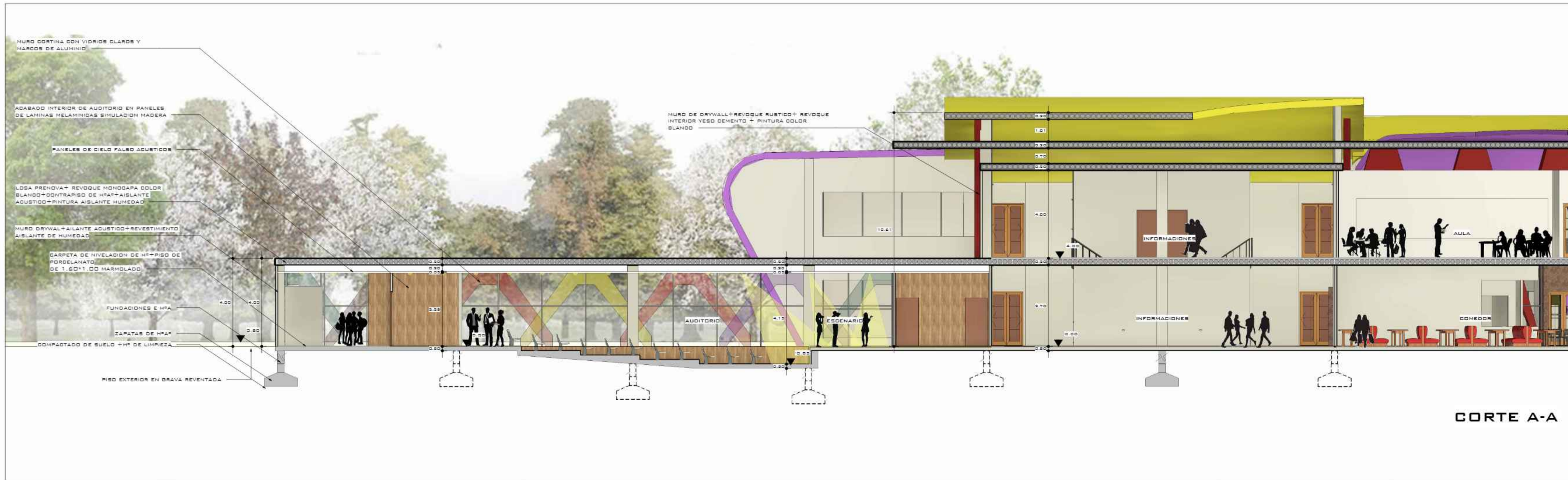
1 CORTE A-A A102 | 1:100
