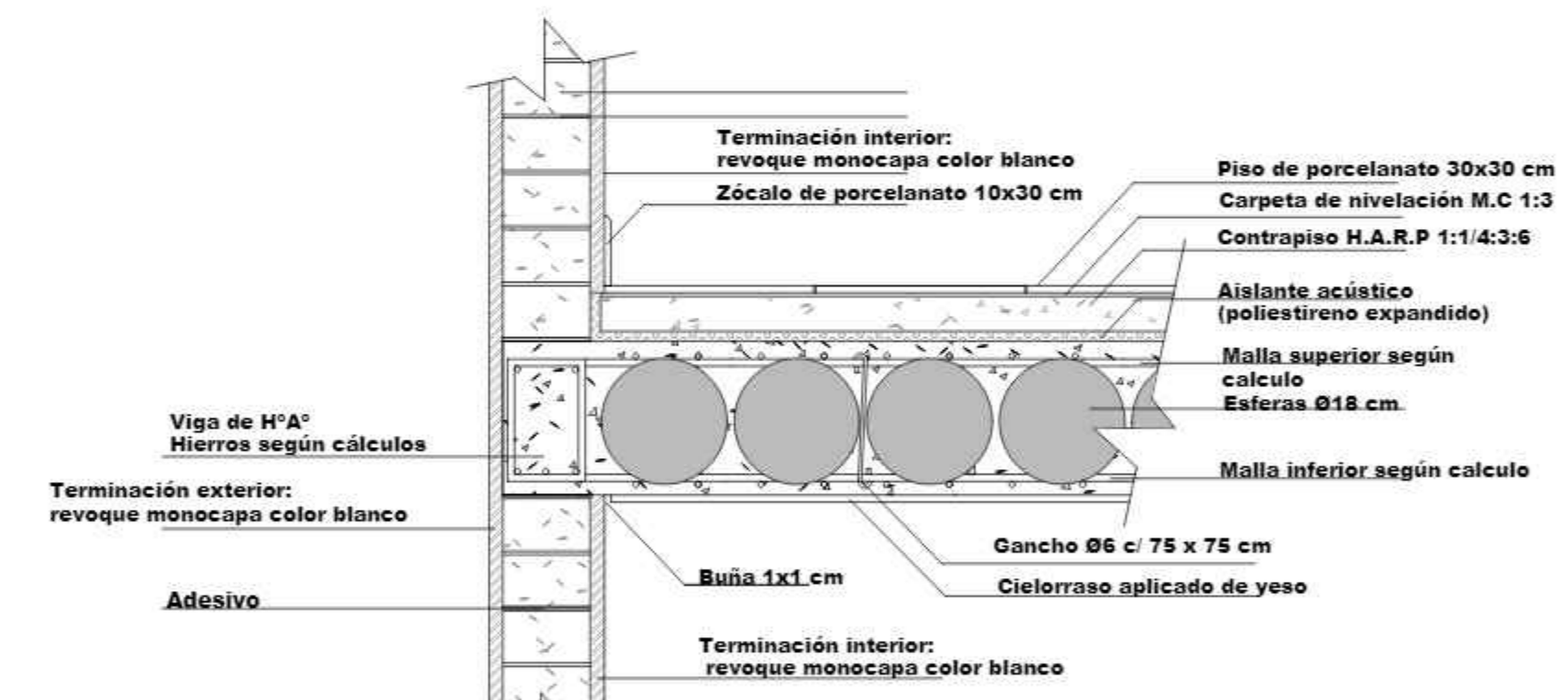
DETALLE LOZA PRENOVA ESC. 1/10
