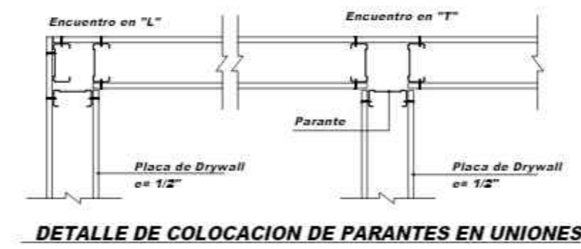
DETALLE DE UNION DE PLANCHAS DRYWALL
