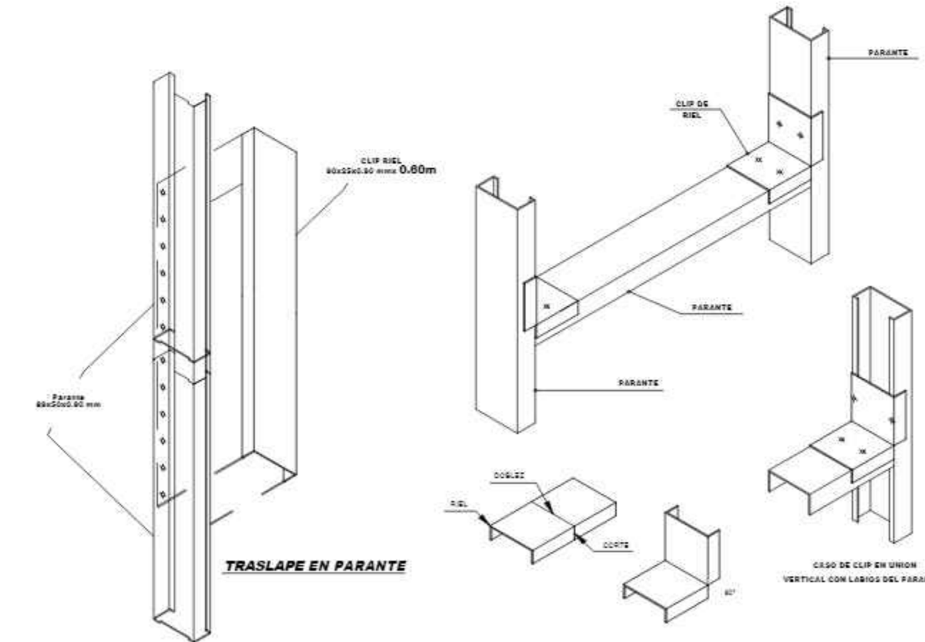
DETALLE HORIZONTAL DE PERFILES ESC. 1/10
