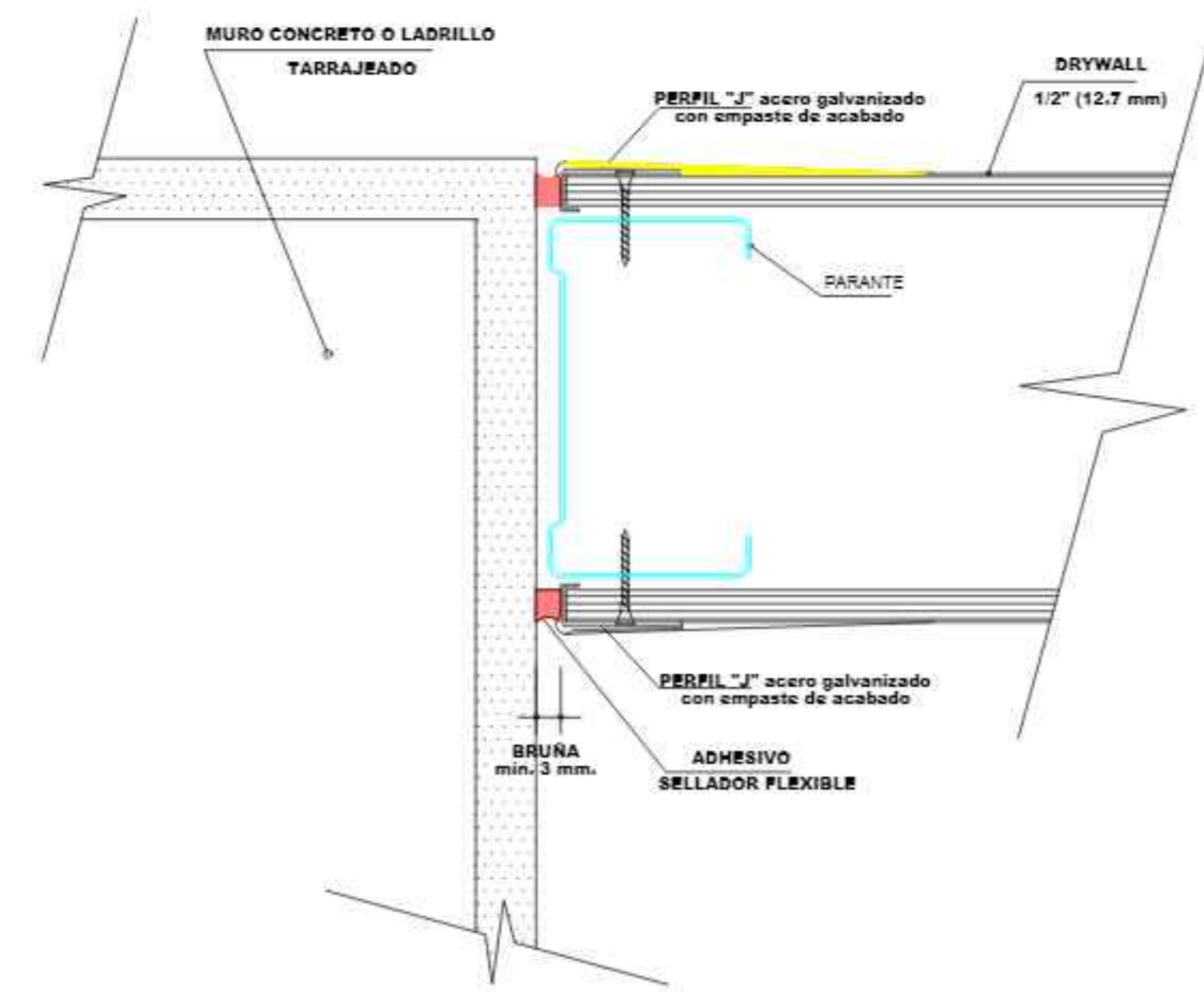
DETALLE ENCUENTRO TABIQUE CONCRETO / TABIQUE DRYWALL
