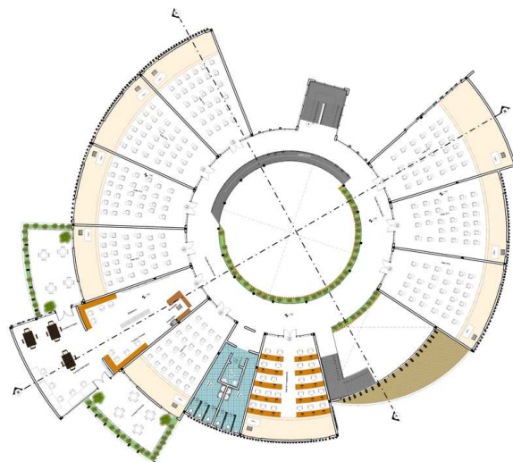
PLANO DE PLANTA ALTA AMOBLADA ESCALA 1:50
