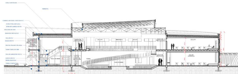
CORTE A-A" (BLOQUE AULAS) ESC. 1/2000
