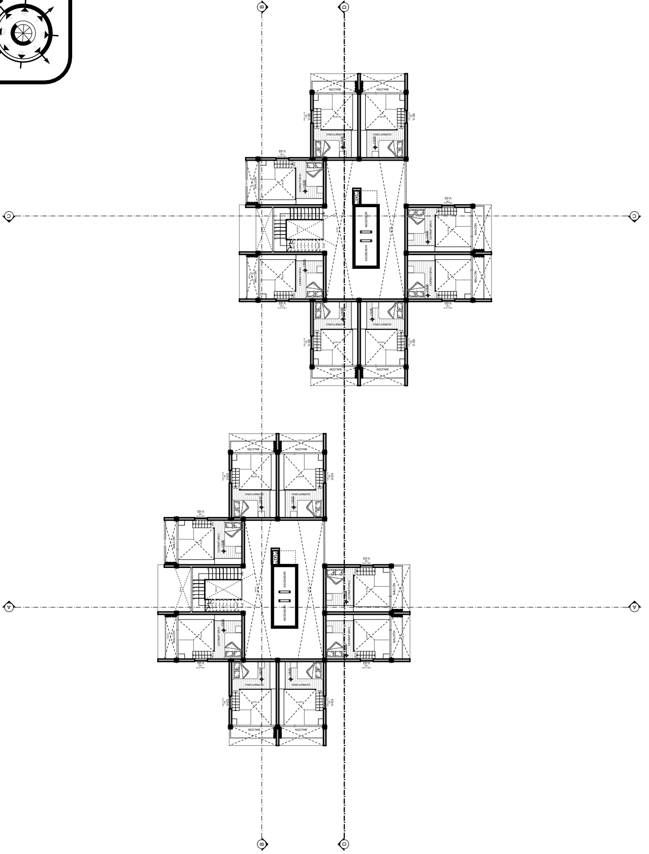
PLANO AMOBLADO MESANINE CUARTO PISO ESC. 1:300
