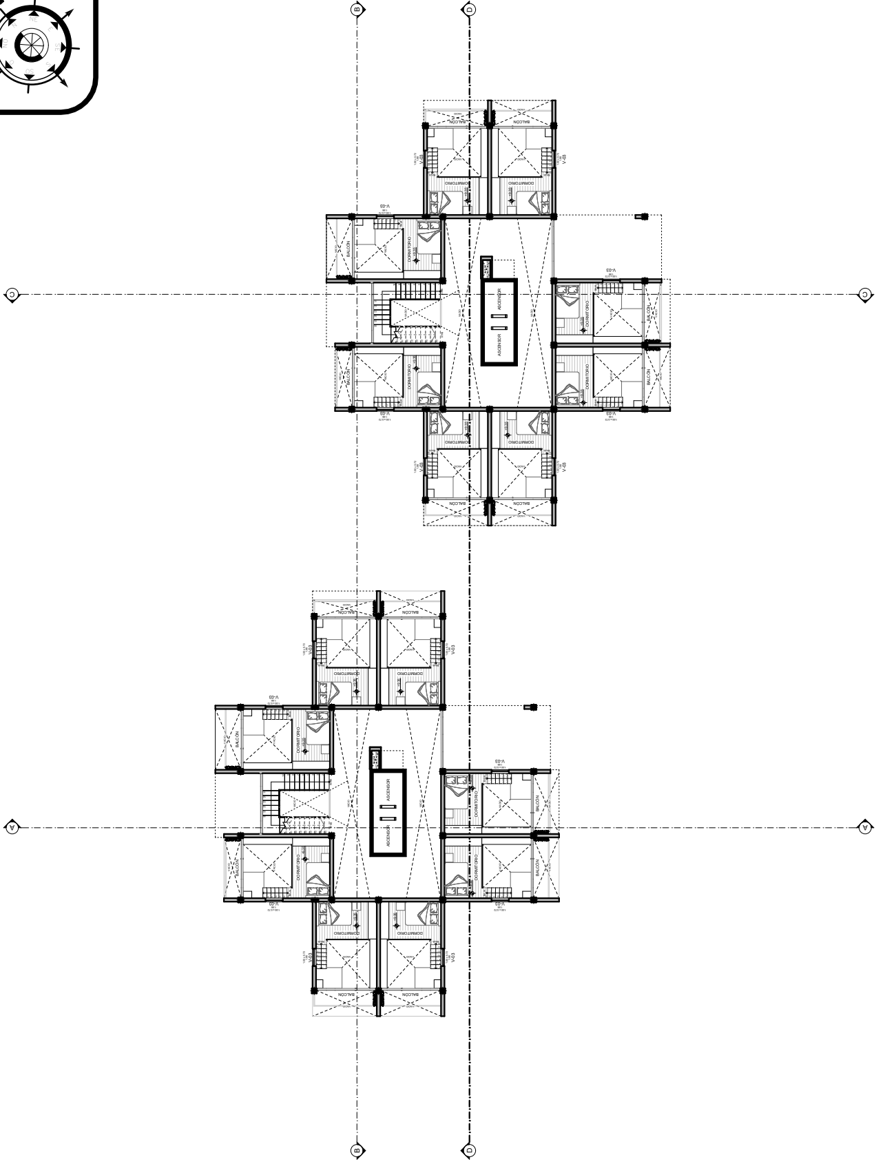
PLANO AMOBLADO MESANINE SEGUNDO PISO ESC. 1:300
