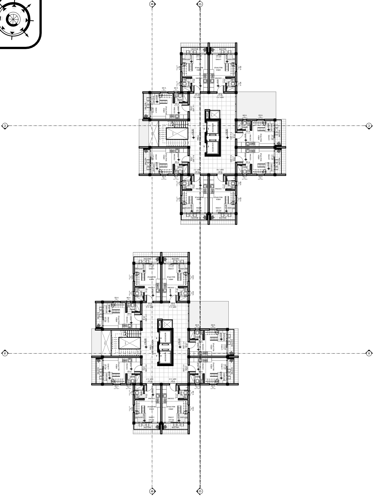
PLANO AMOBLADO CUARTO PISO ESC. 1:300
