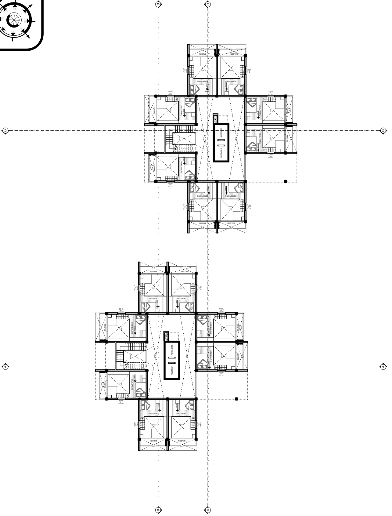
PLANO AMOBLADO MESANINE TERCER PISO ESC. 1:300
