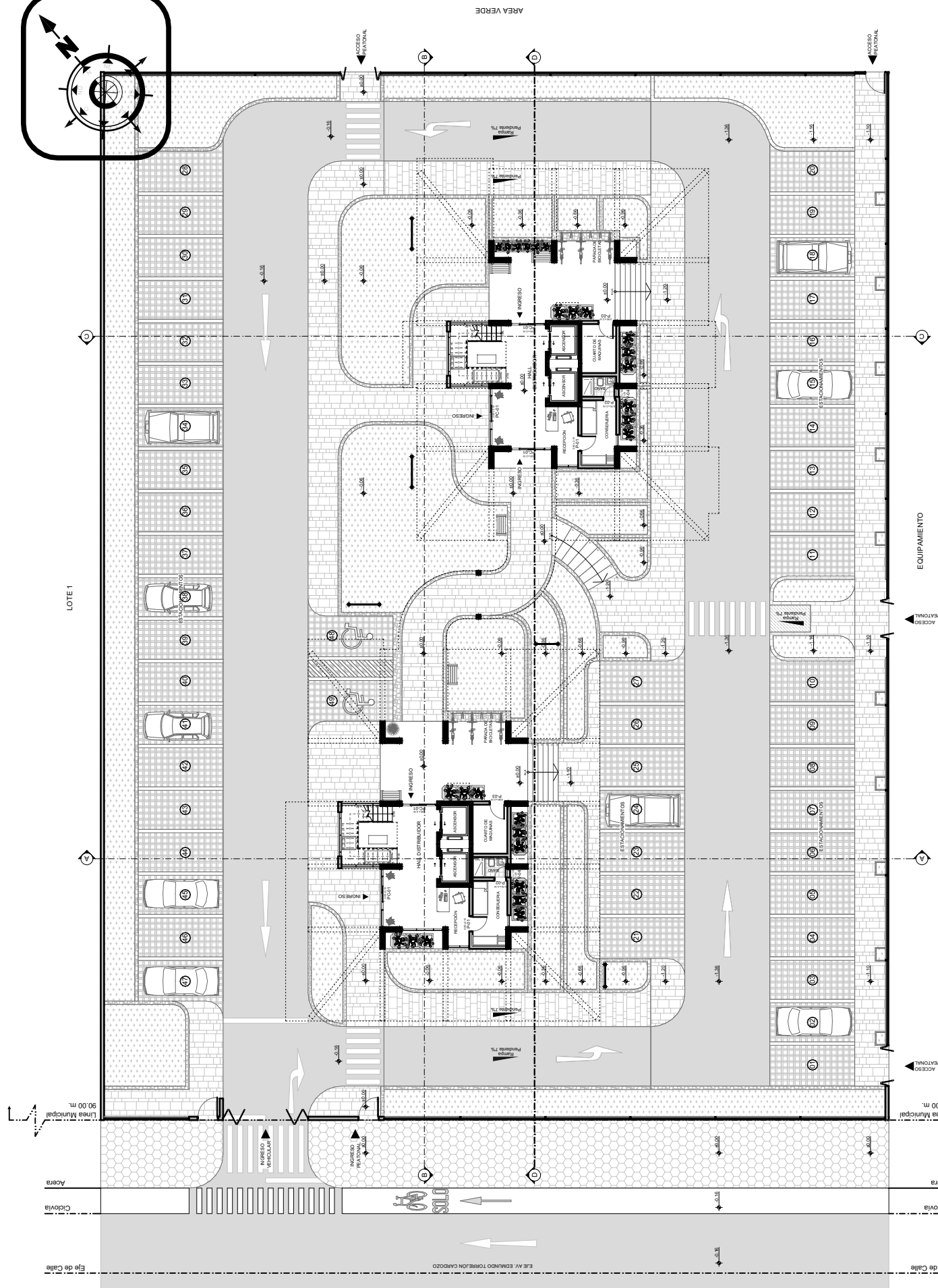
PLANO AMOBLADO PLANTA BAJA ESC. 1:300
