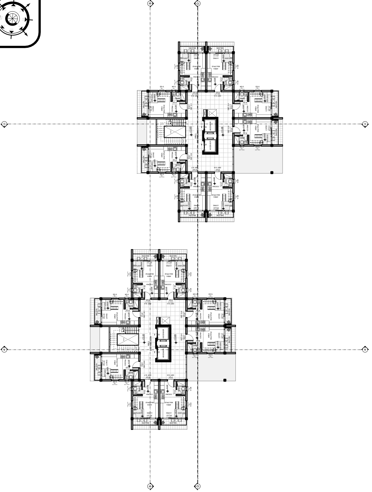
PLANO AMOBLADO TERCER PISO ESC. 1:300
