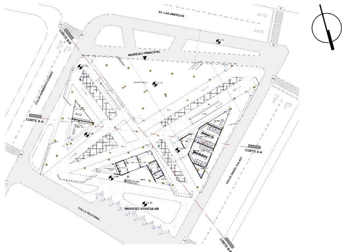
PLANTA BAJA ACOTADA
