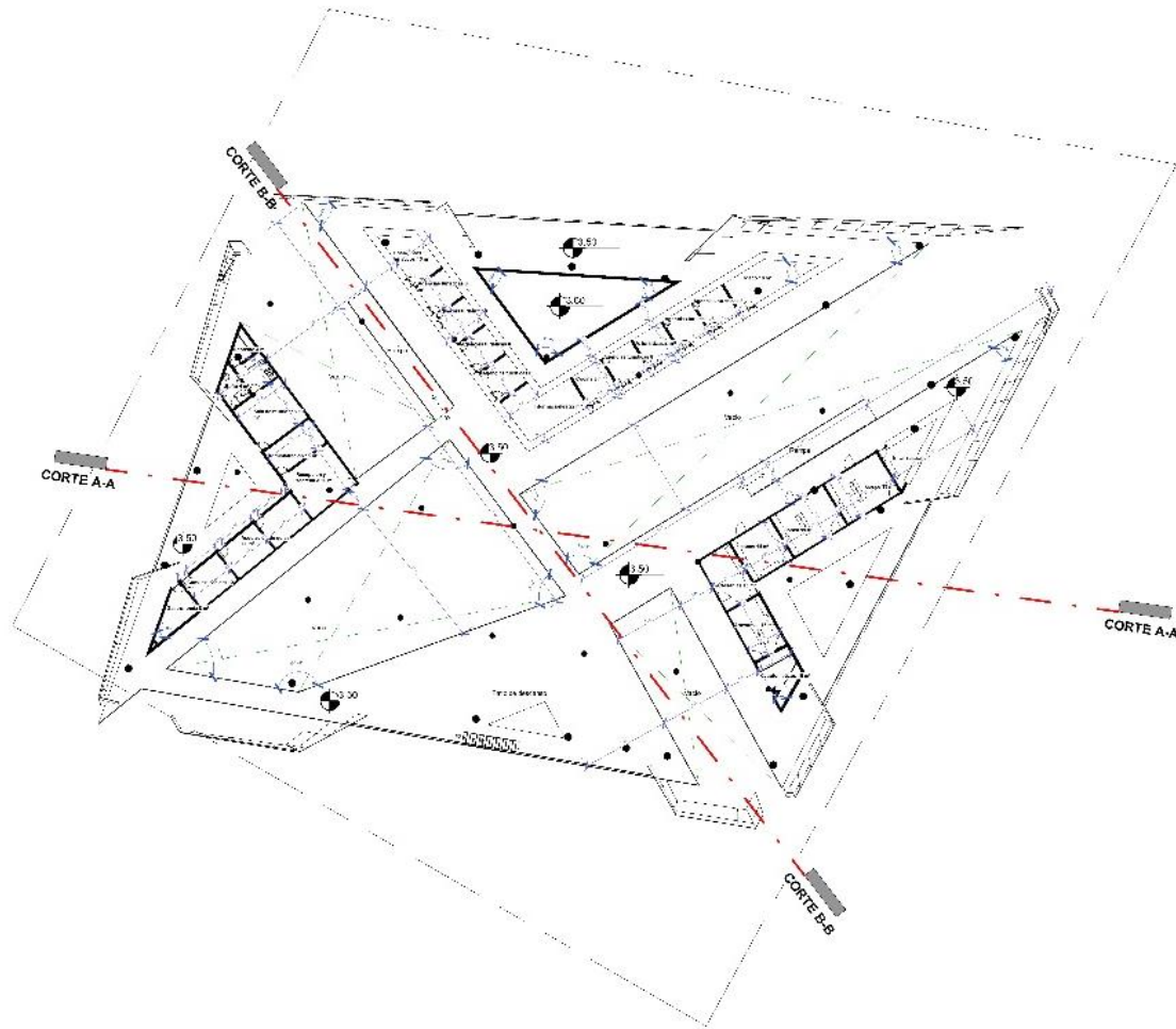
PRIMER PISO ACOTADO
