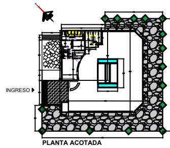
PLANTA ACOTADA
