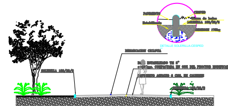
CORTE AA TIPO DEL SENDERO PRINCIPAL CON ASFALTO
