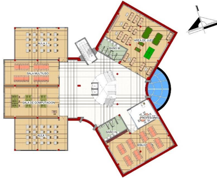
PLANTA MESSANINE BLOQUE DE ADMINISTRACIÓN Y HOSPEDAJE
