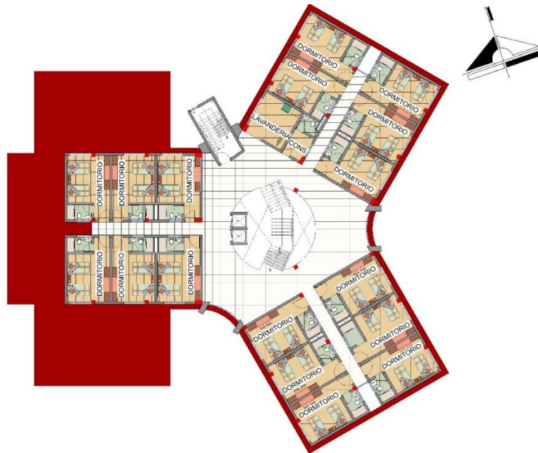
PRIMER PISO BLOQUE DE ADMINISTRACIÓN Y HOSPEDAJE
