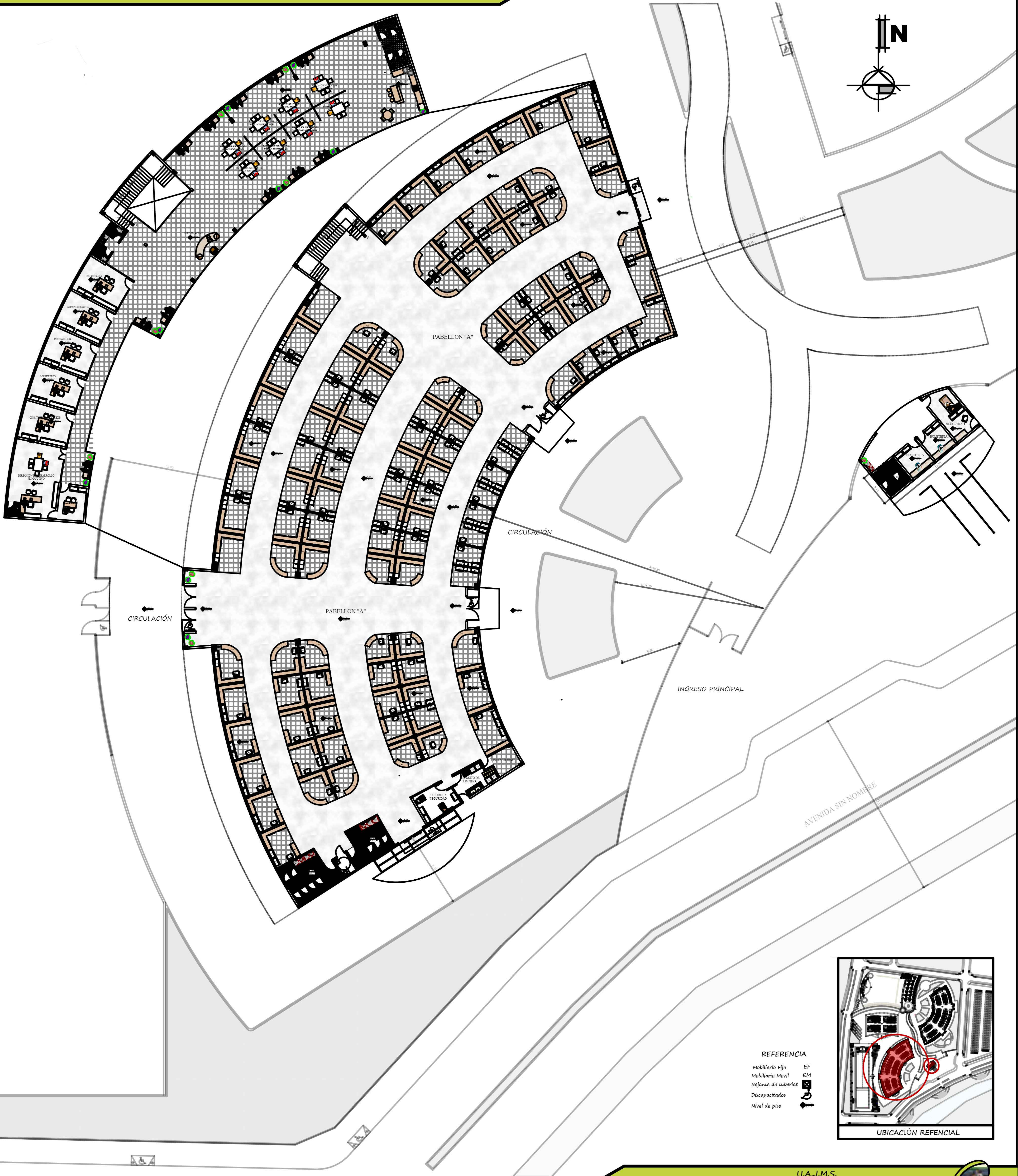
PLANTA BAJA - ALTA AMOBLADA INGRESO - PABELLON "A" ESC: 1:100
