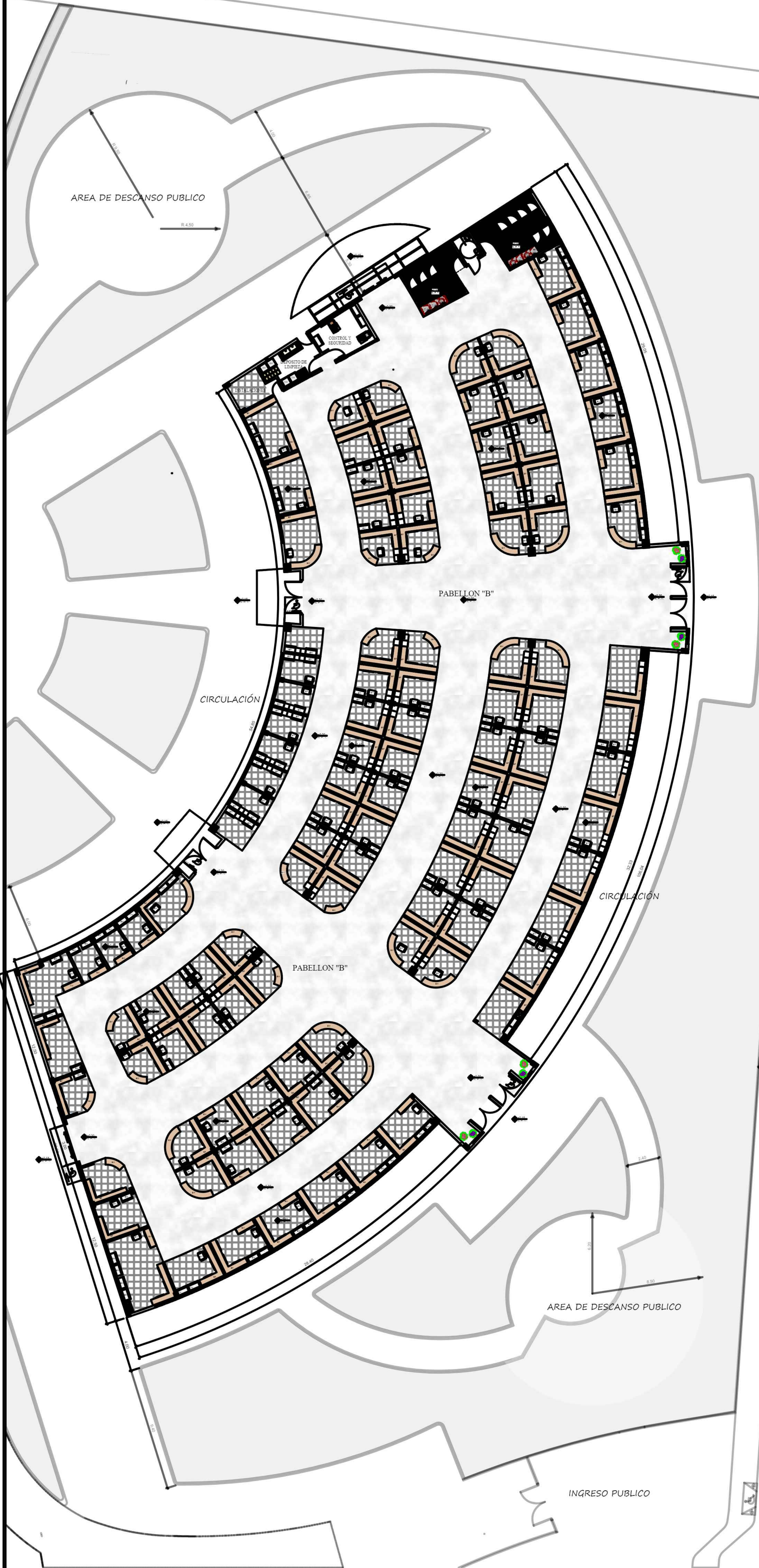
PLANTA AMOBLADA PABELLON "B" ESC: 1:100
