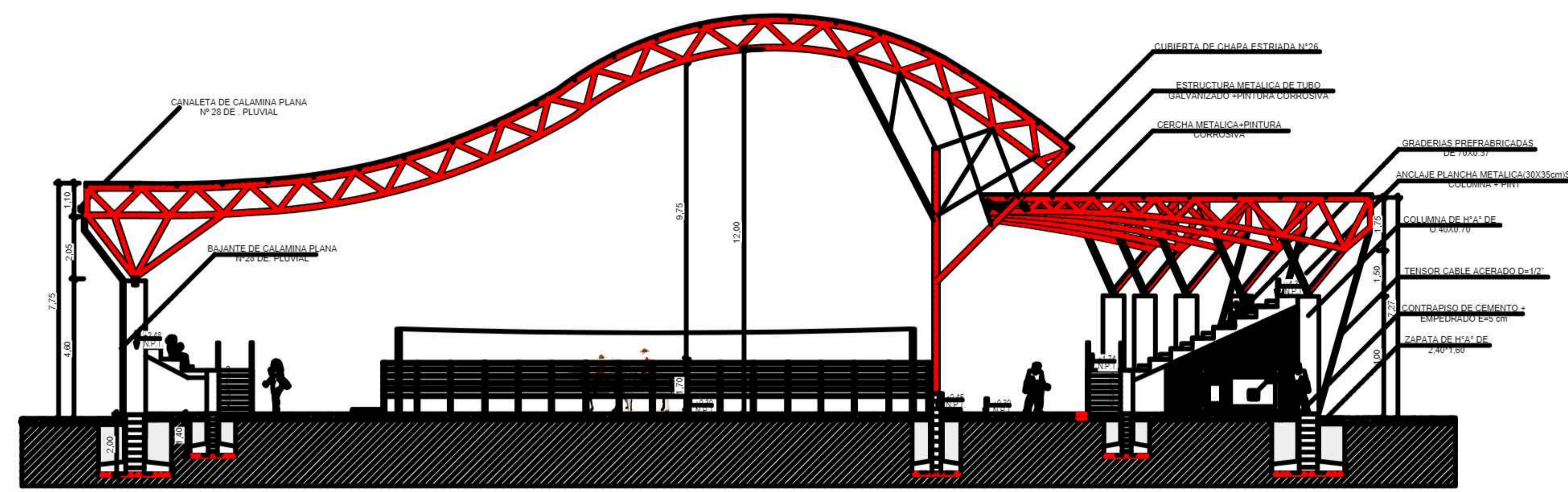
CORTE C-C'
