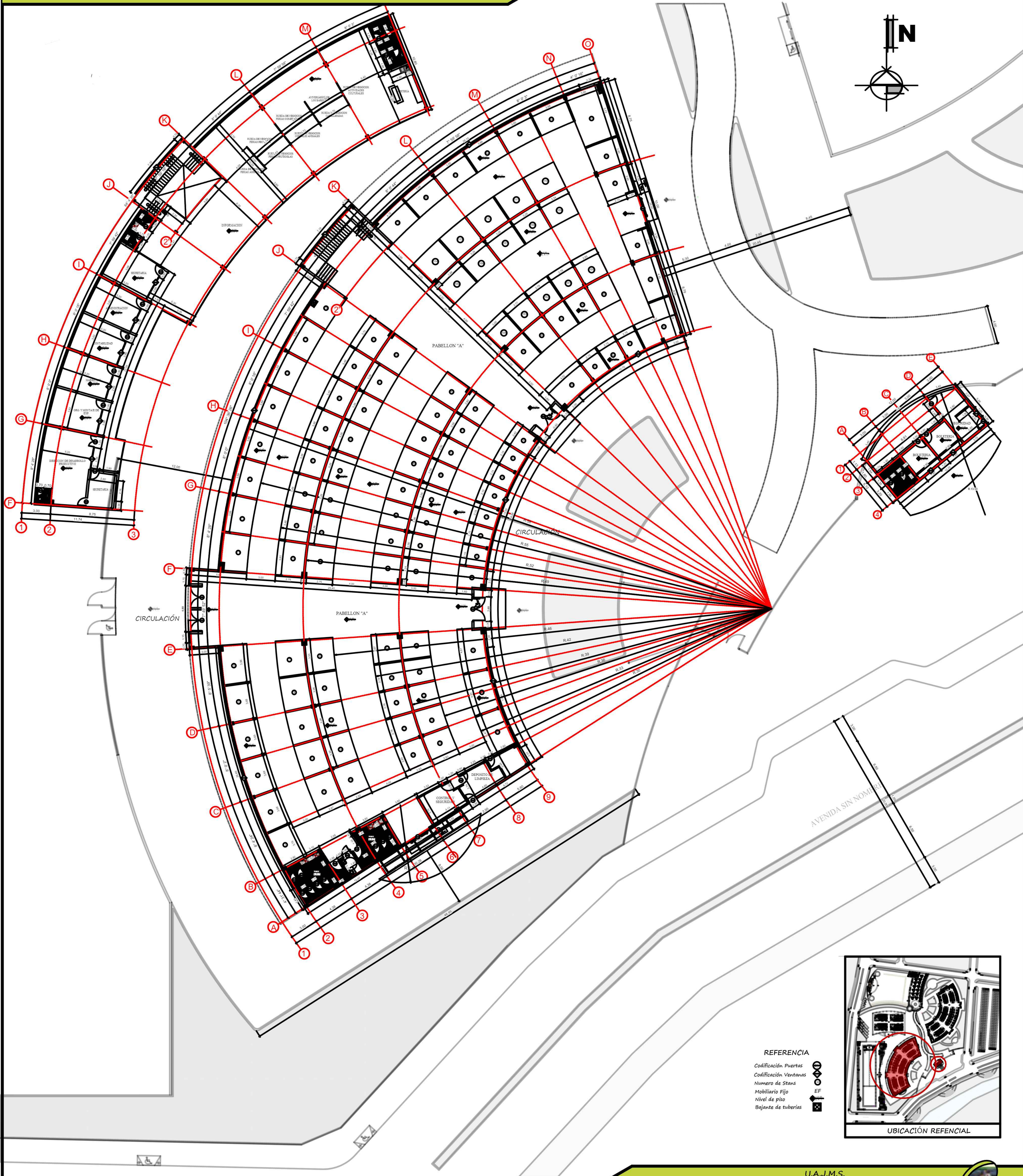
PLANTA BAJA - ALTA ACOTADA INGRESO - PABELLON "A" ESC: 1:100
