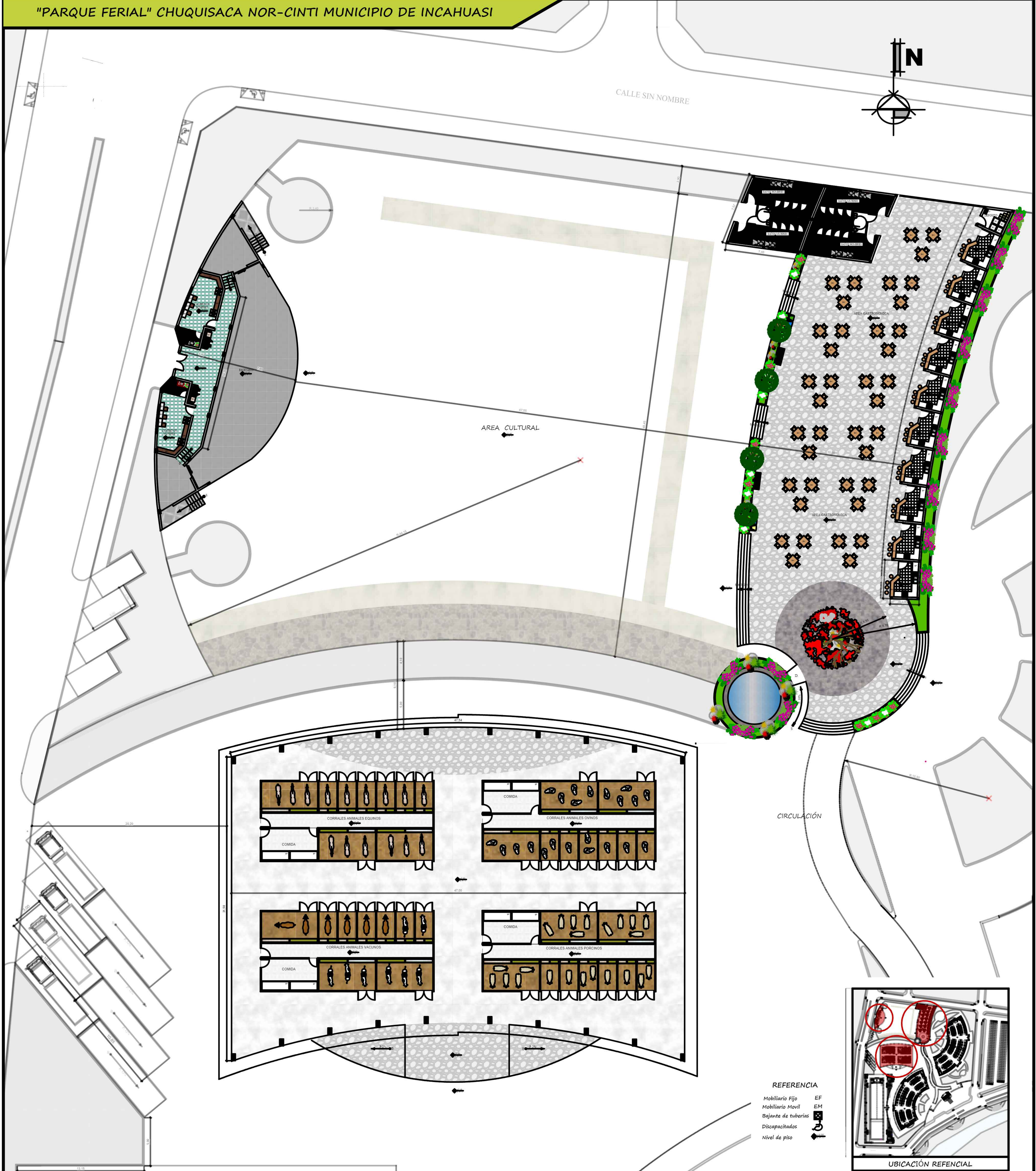
PLANTA AMOBLADA AREA CULTURAL-GASTRONOMICA Y CORRALES ESC: 1:100
