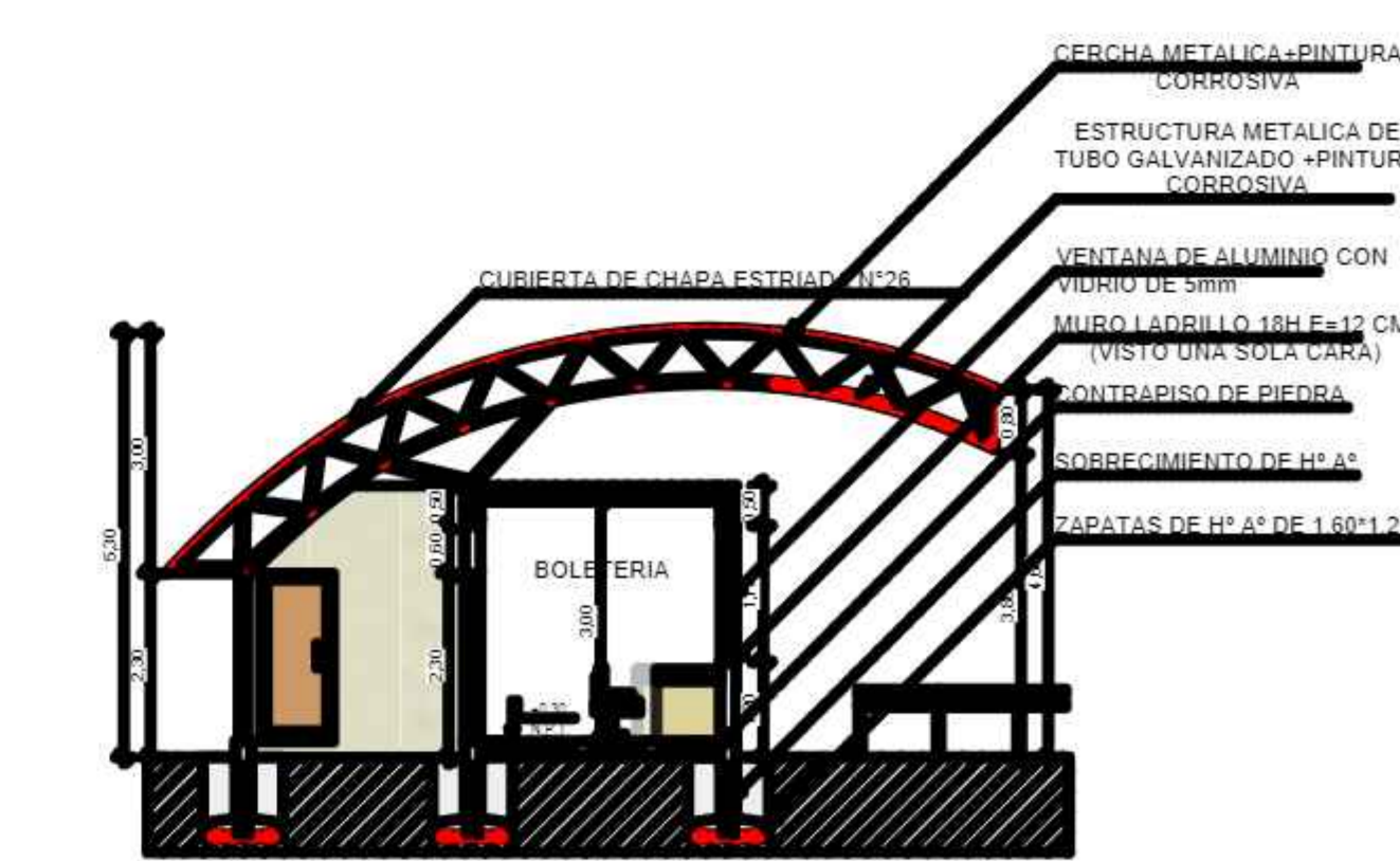
CORTE E-E'
