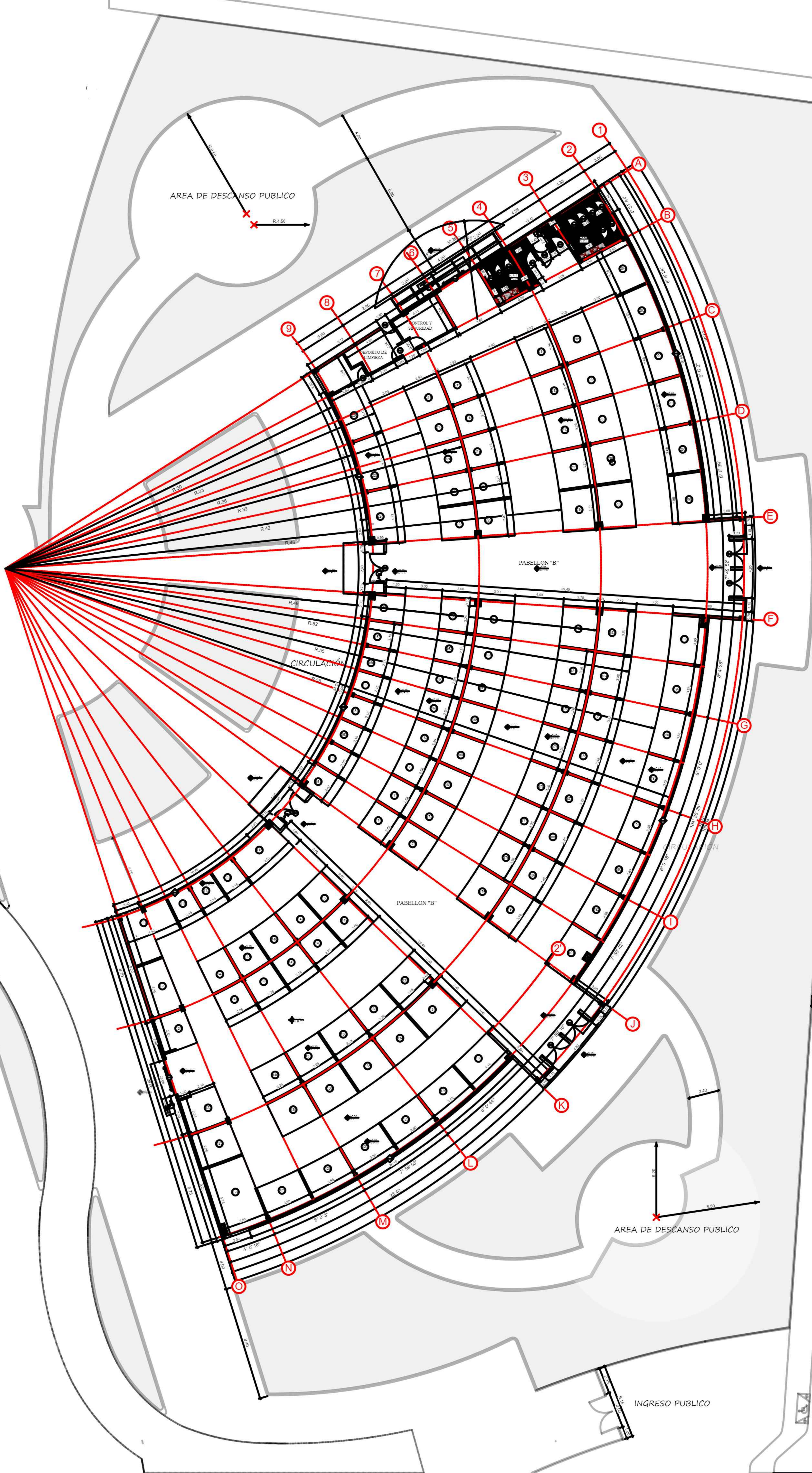
PLANTA ACOTADA PABELLON "B" ESC: 1:100
