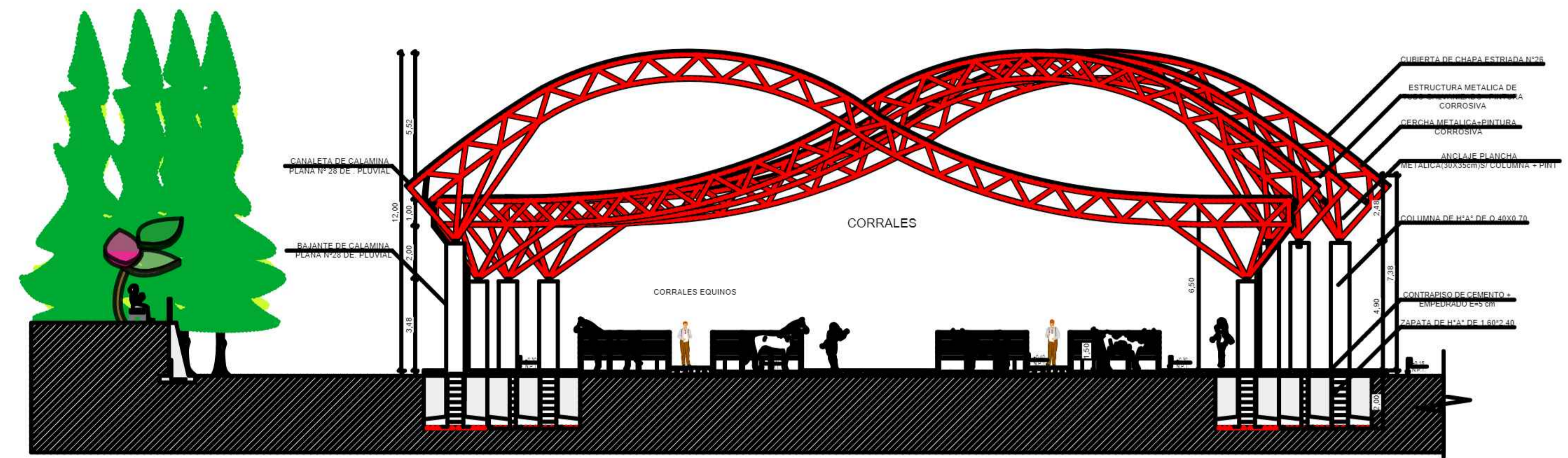
CORTE B-B'
