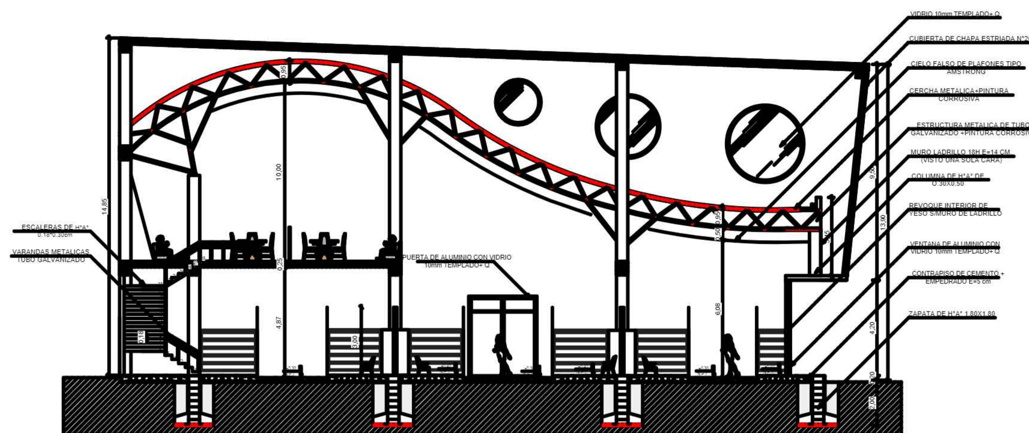
CORTE D-D'
