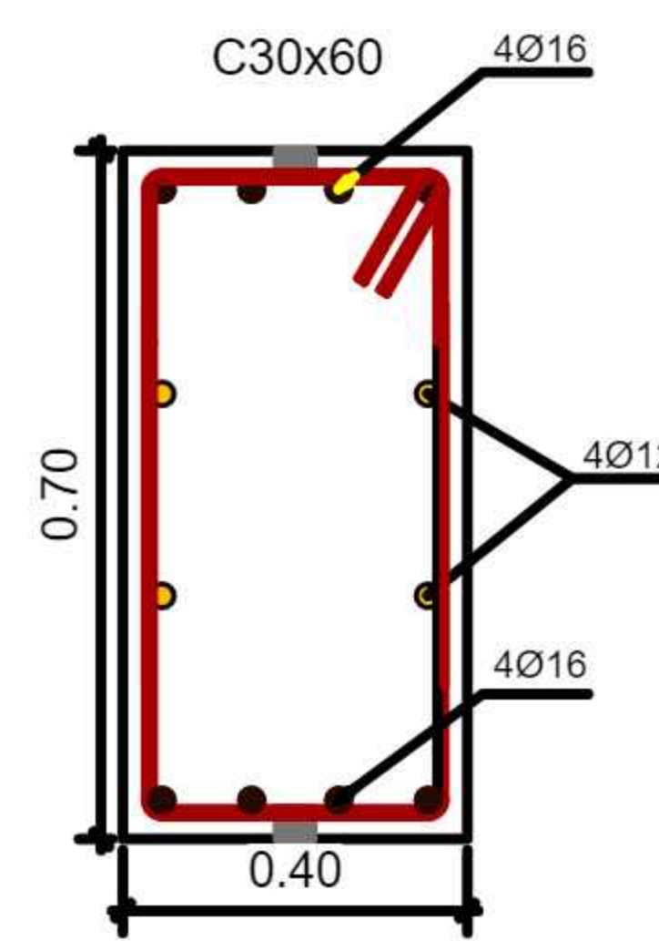
COLUMNA ESC. 1:50
