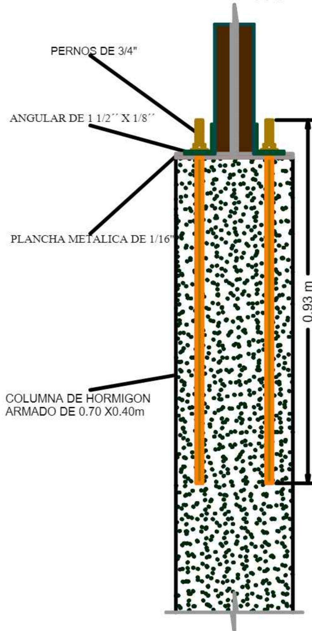
DETALLE DE ANCLAJE ESC. 1:10
