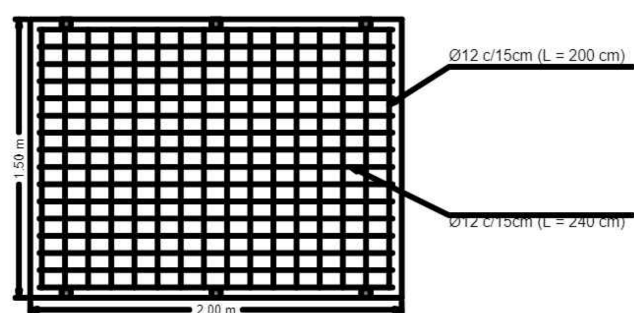
DETALLE CONSTRUCTIVO DE ZAPATA
