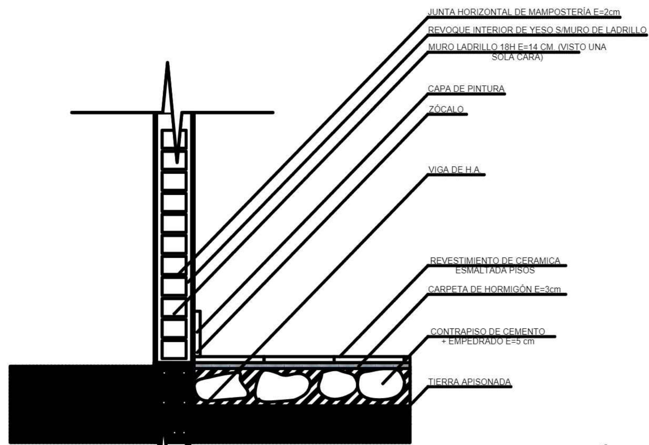
DETALLE CONSTRUCTIVO DE MURO ESC. 1:10
