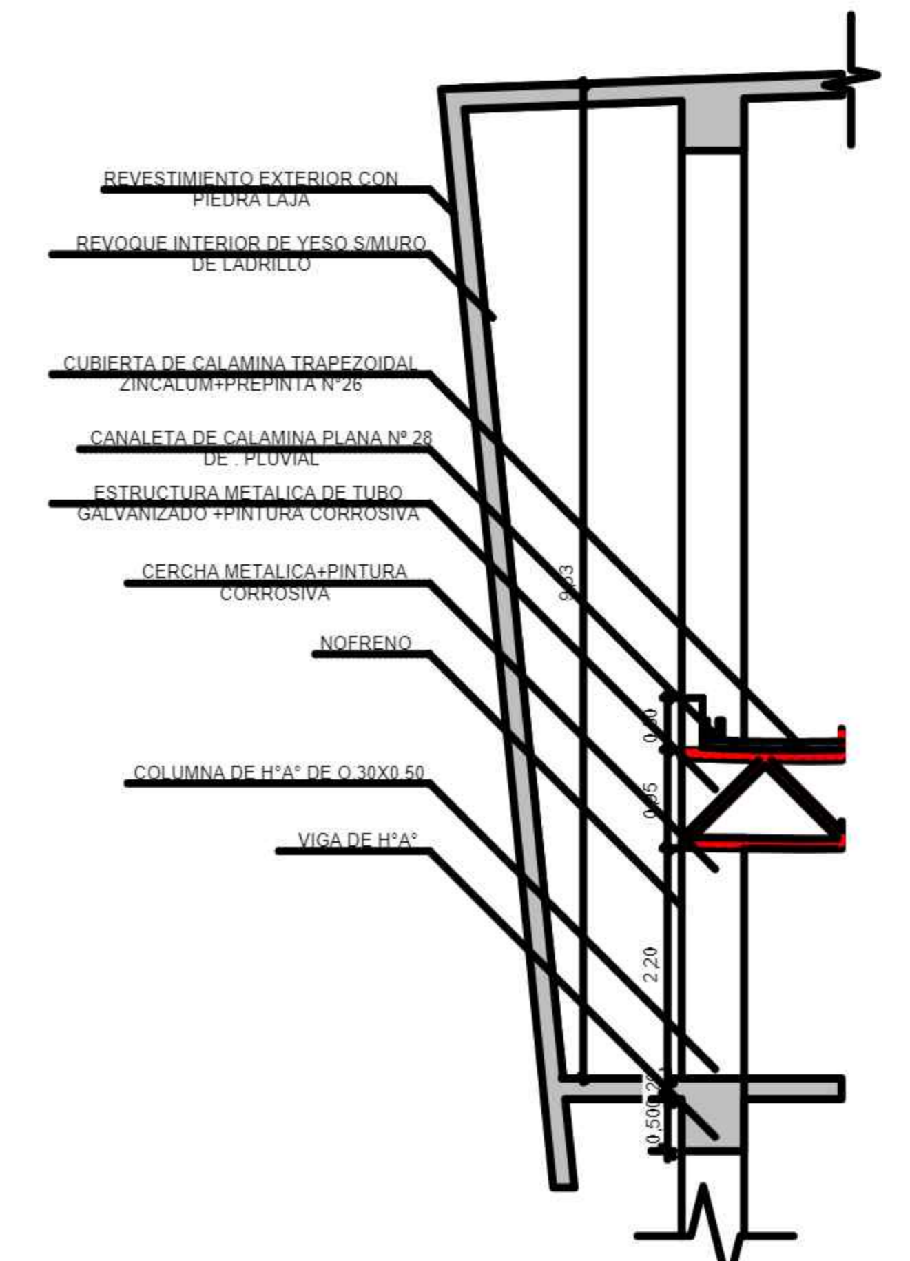
DETALLE CONSTRUCTIVO UNION JUNTAS ESC. 1:50
