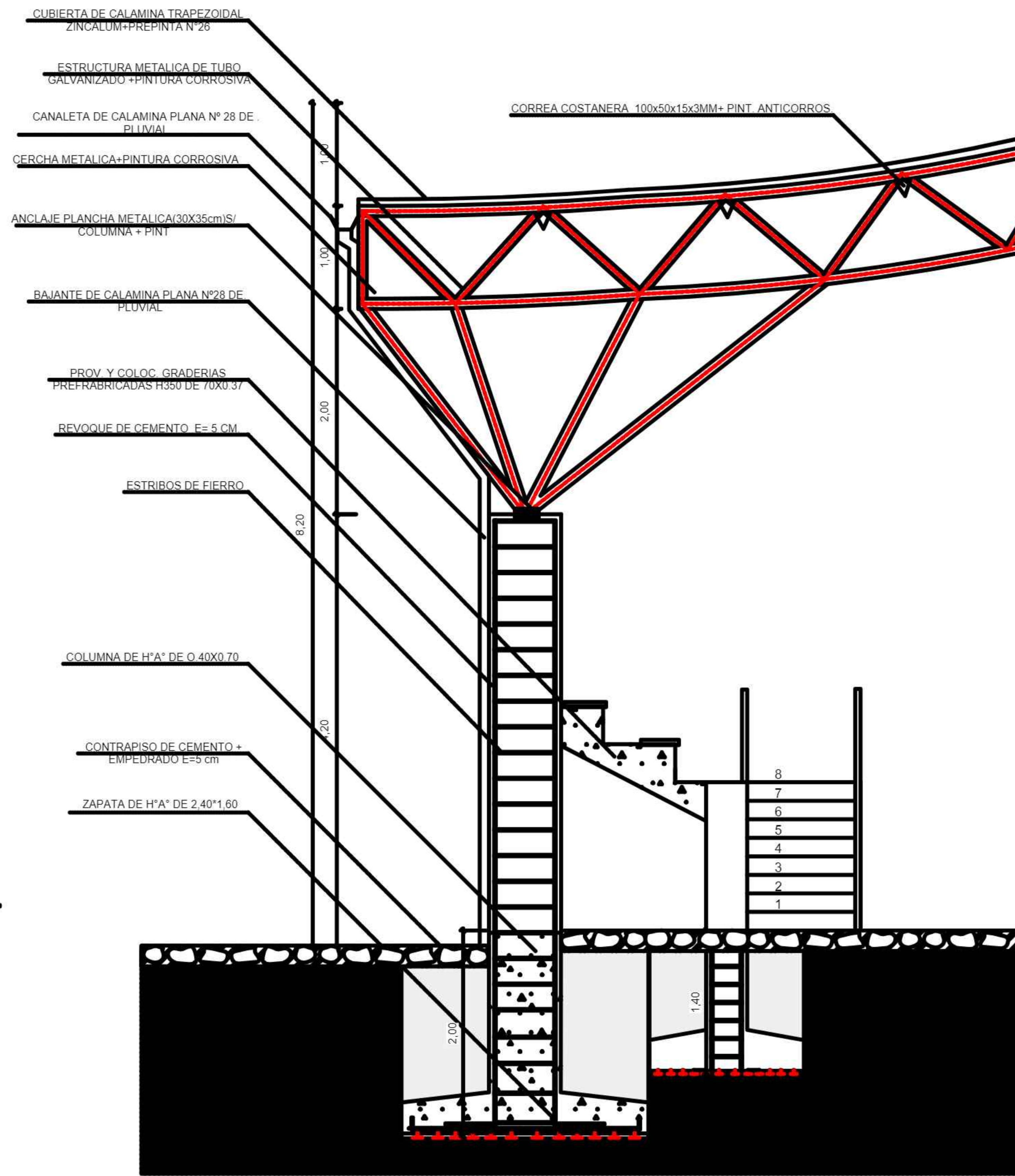
CORTE DE BORDE C-C" ESC. 1:25
