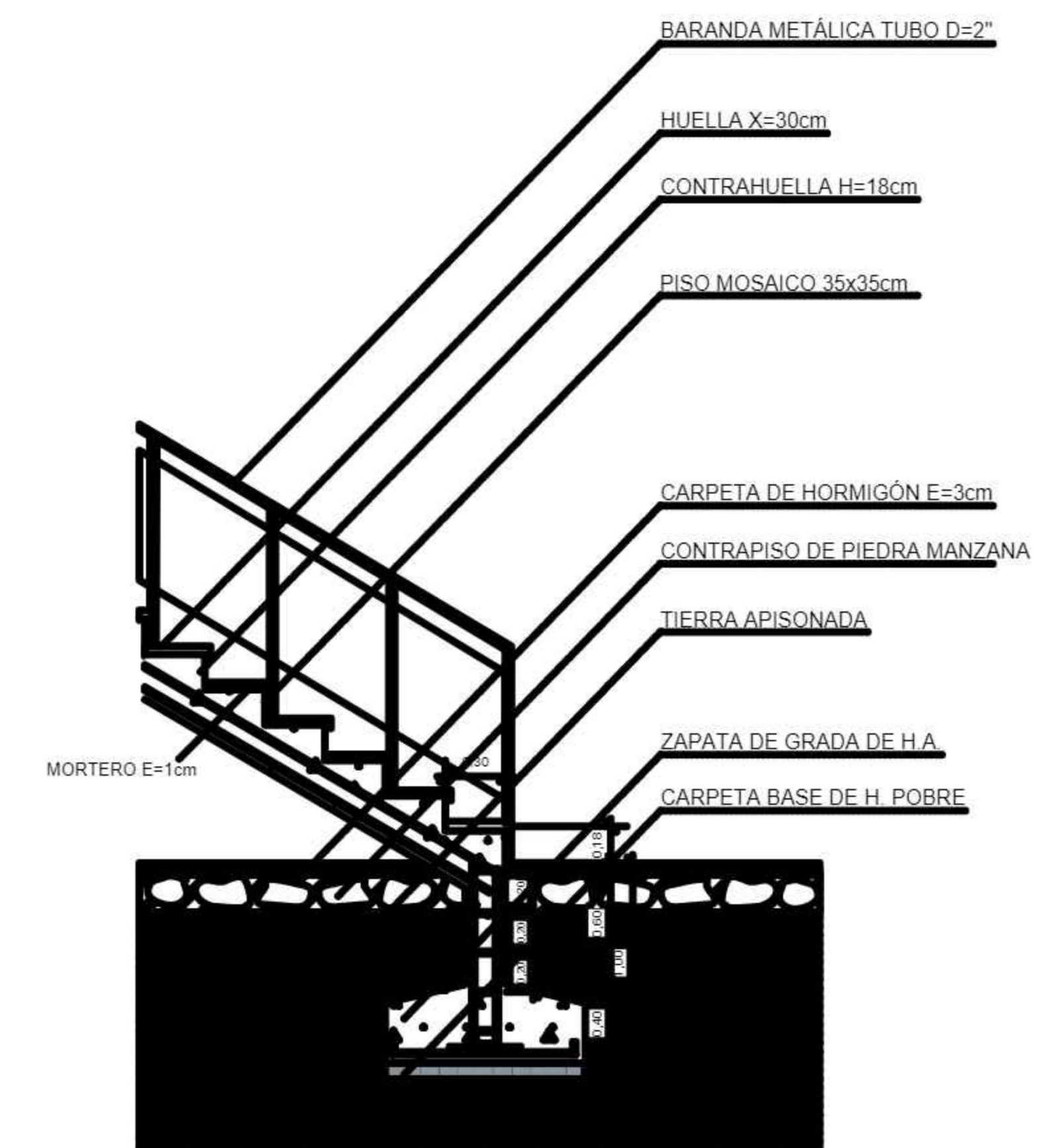
DETALLE CONSTRUCTIVO DE ESCALERA ESC. 1:25
