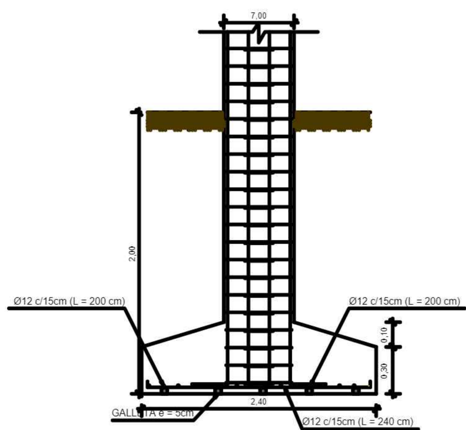
DETALLE CONSTRUCTIVO DE MURO ESC. 1:10
