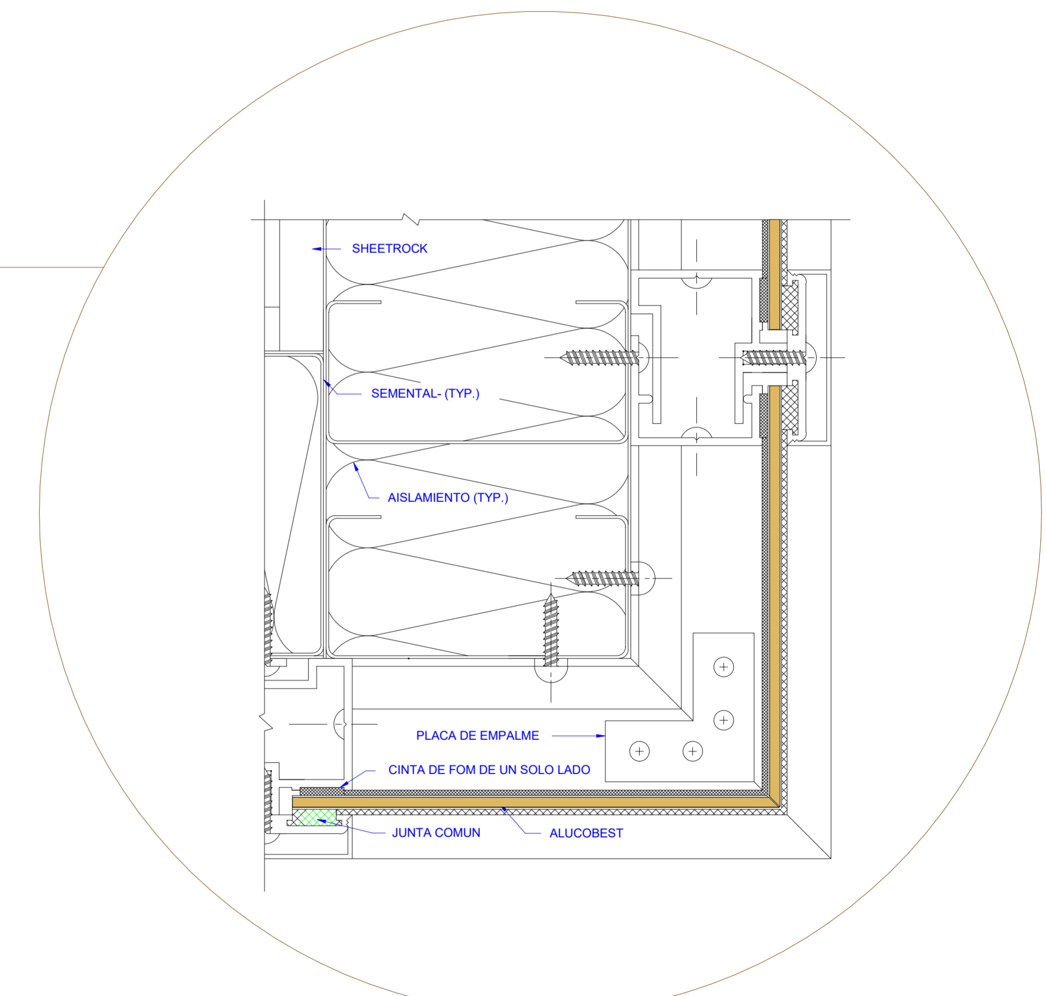
DETALLE DE ESQUINA PLACA DE ALUMINIO ESCALA 1.100
