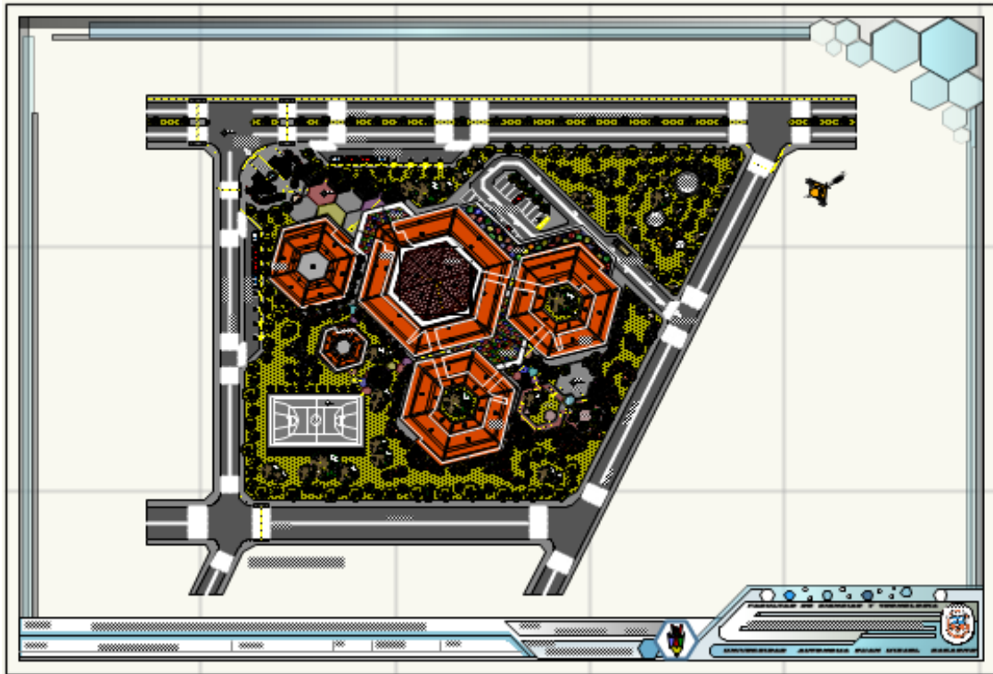
PLANO PAISAJISTICO OTOÑO
