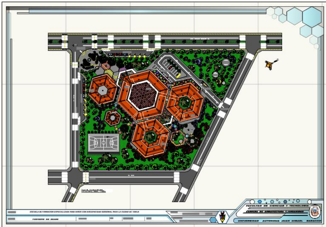
PLANO PAISAJISTICO PRIMAVERA
