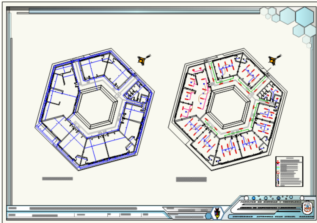
AREA DE ACADEMICA III PLANTA ACOTADA - INSTALACION ELECTRICA
