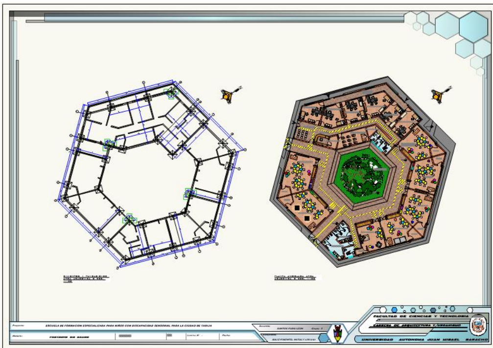
AREA DE ACADEMICA II PLANO DE CIMIENTOS - PLANTA AMOBLADA
