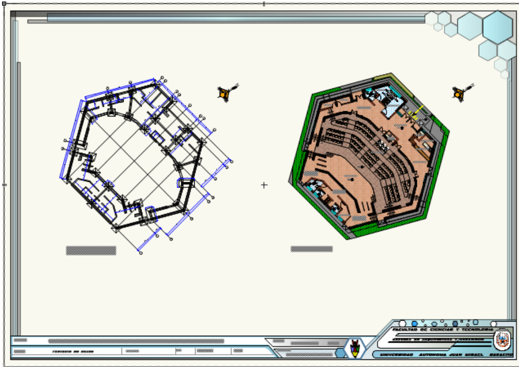
AREA DE SERVICIO PLANO DE CIMENTOS – PLANTA AMOBLADA
