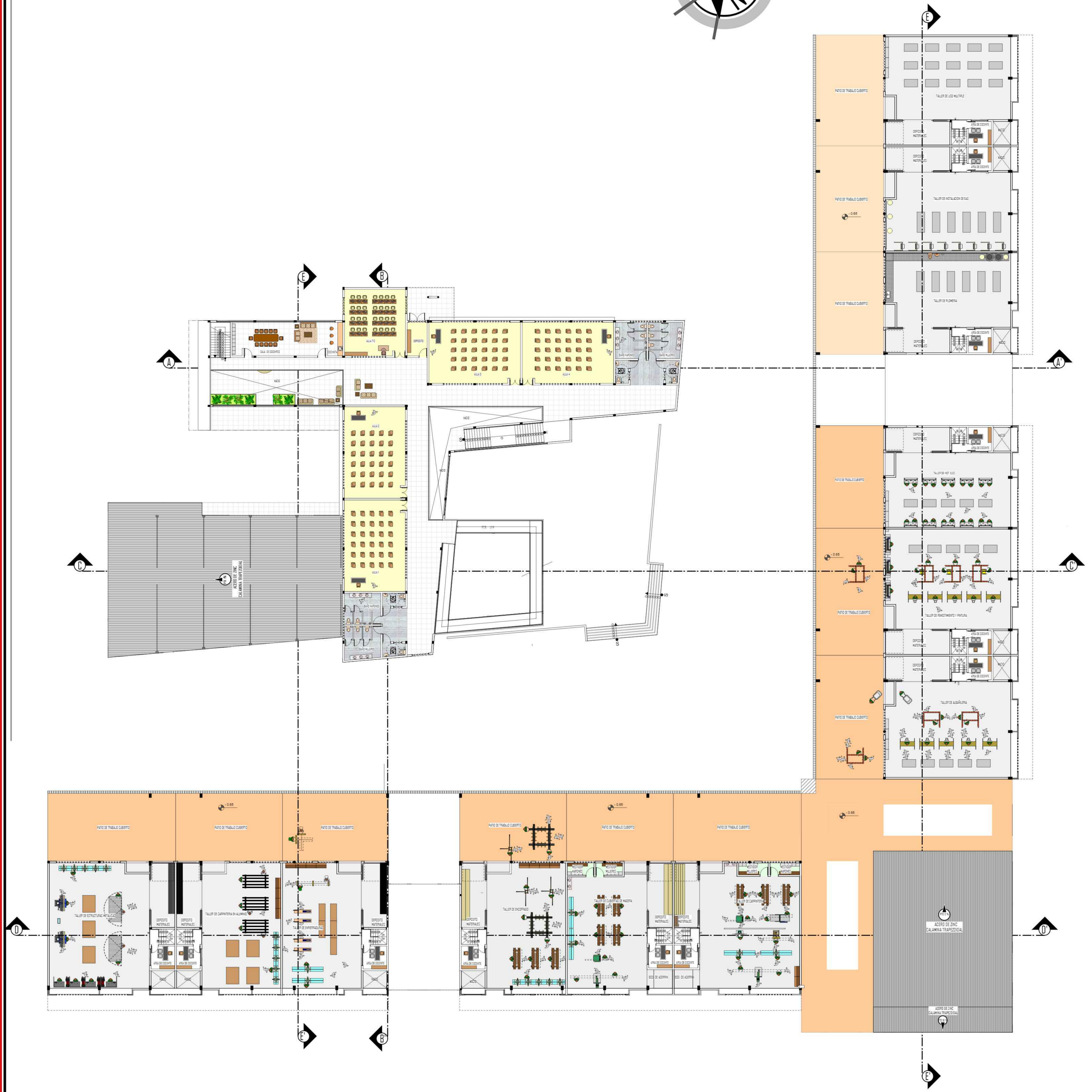
PLANTA ALTA
