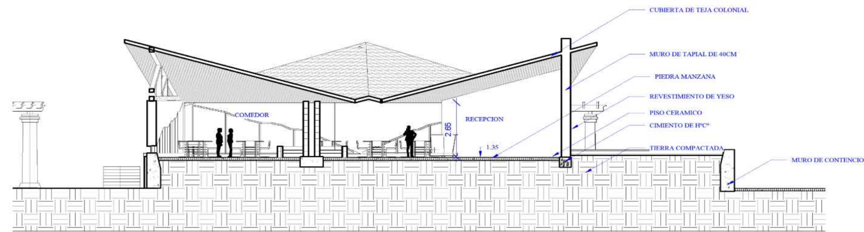
CORTE C-C'' (AREA DE COMEDOR)
