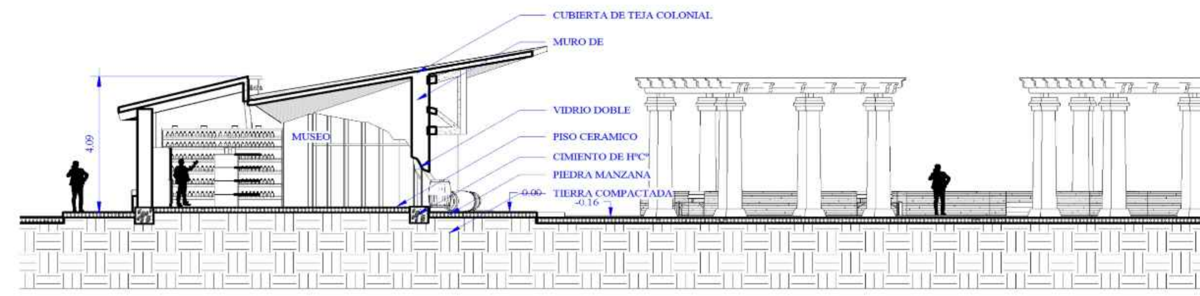
CORTE B-B'' (AREA DE MUSEO)
