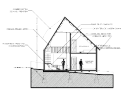
CORTE TRANSVERSAL A-A1 CABAÑA 1
