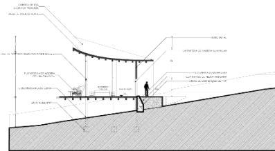
CORTE LONGITUDINAL B-B1 CABAÑA 3
