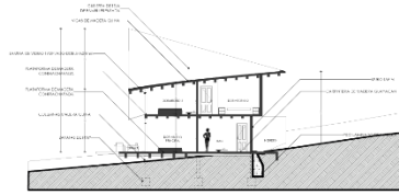
CORTE LONGITUDINAL B-B1 CABAÑA 1
