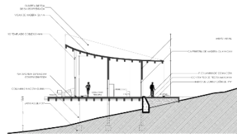
CORTE LONGITUDINAL B-B1 CABAÑA 2
