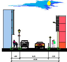
PERFIL DE VIA E-E DE LA CALLE GENERAL TRIGO ENTRE DOMINGO PAZ Y CORRADO
