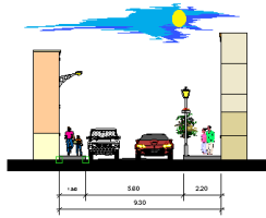
PERFIL DE VIA D-D DE LA CALLE GENERAL TRIGO ENTRE BOLIVAR Y DOMINGO PAZ
