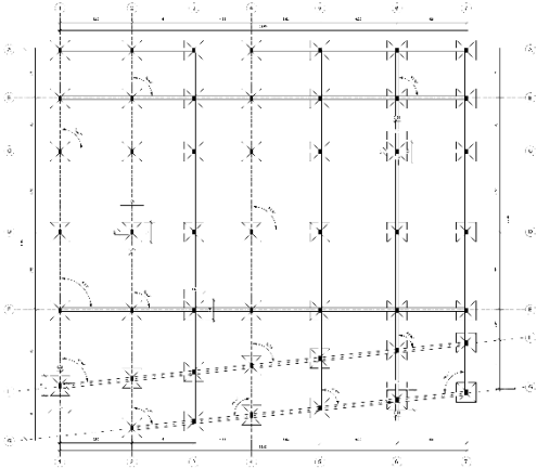
CIMENTOS ESC. 1:100
