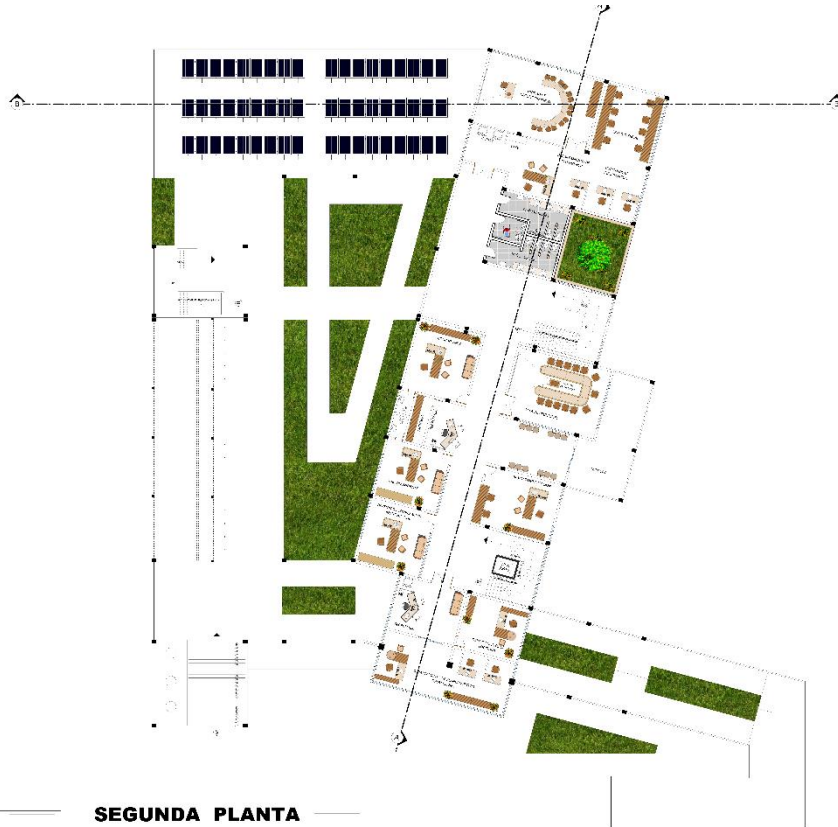
SEGUNDA PLANTA
