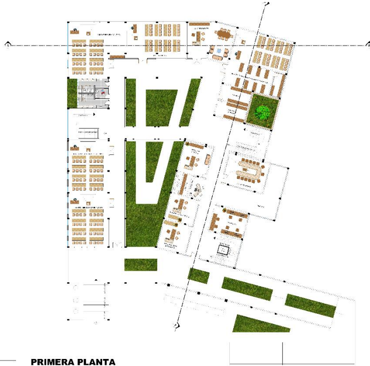
PRIMERA PLANTA
